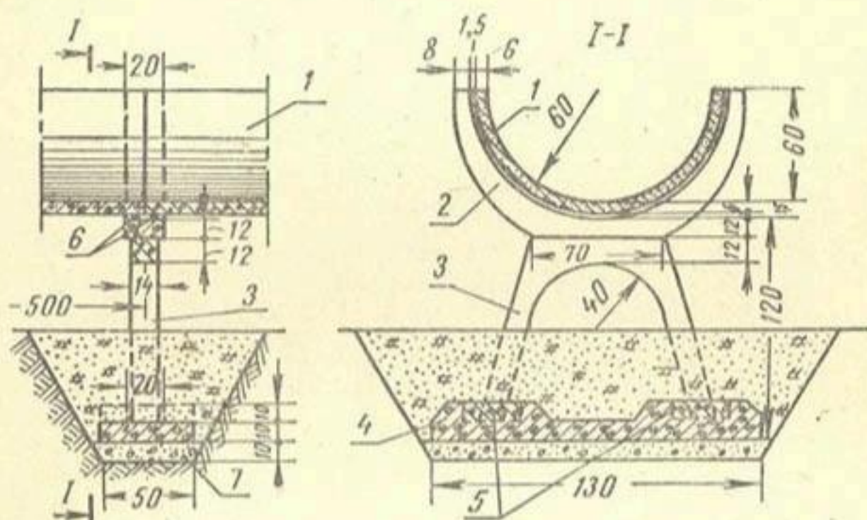
Рис. 18. Конструкция полукруглых лотков, соединяемых с помощью седла на рамной стойке:
