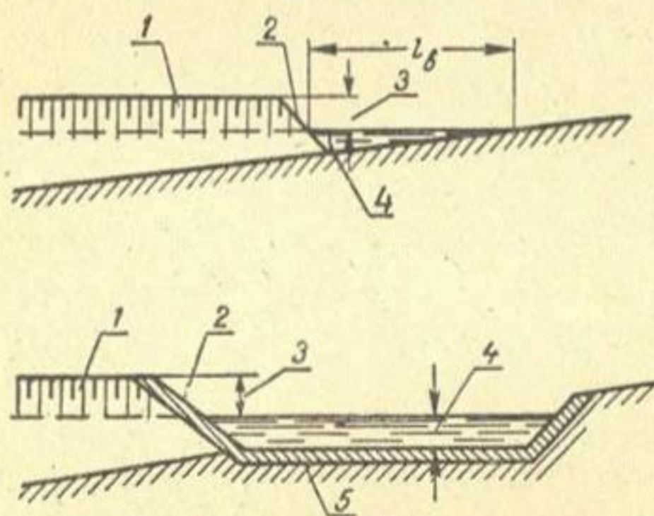
Рис. 47. Водообход у шпоры для пропуска воды (вверху — треугольного сечения без крепления; внизу — трапецидального сечения с креплением):
