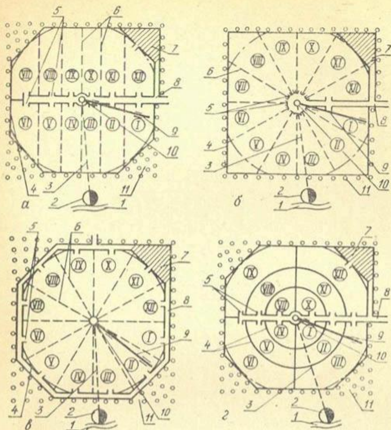
Рис. 14. Схемы организации территории участка культурного пастбища, орошаемого дождевальная установка «Фрегат» с одной позиции с загонами:
