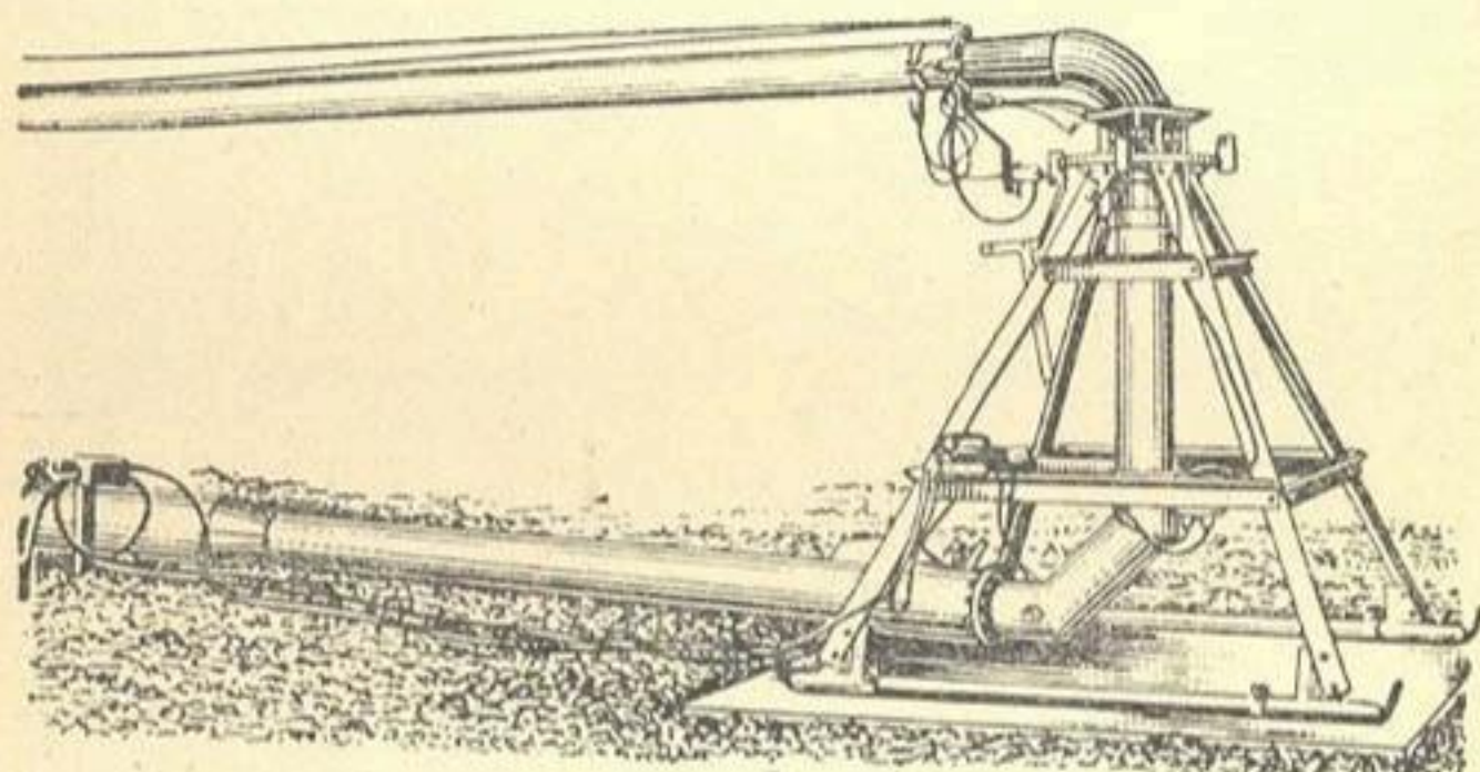
Рис. 9. «Фрегат» на поливе:
