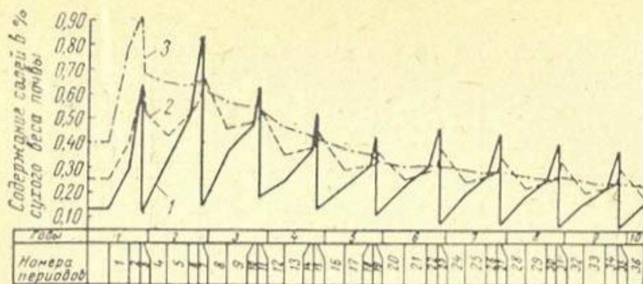
Рис. 34. Динамика засоленности в % сухого веса почв: 1 — на глубине 0,2 м; 2 — на глубине 1 м; 3 — на глубине 2 м.
