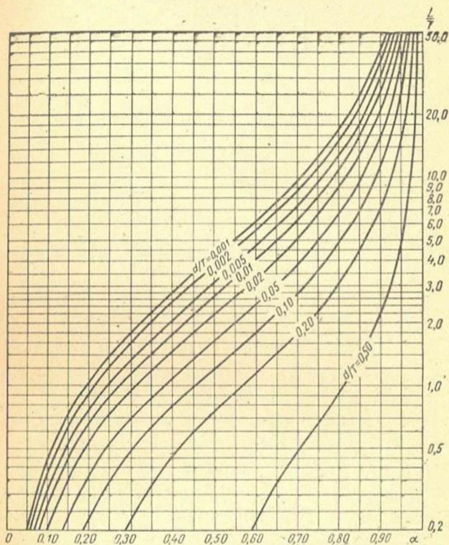
Рис. 40. График для определения коэффициента всячести дренажа:
