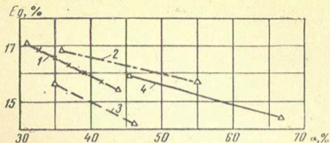
Рис. 2. Потери на испарение ( E_g ) в зависимости от относительной влажности воздуха ( a ):
