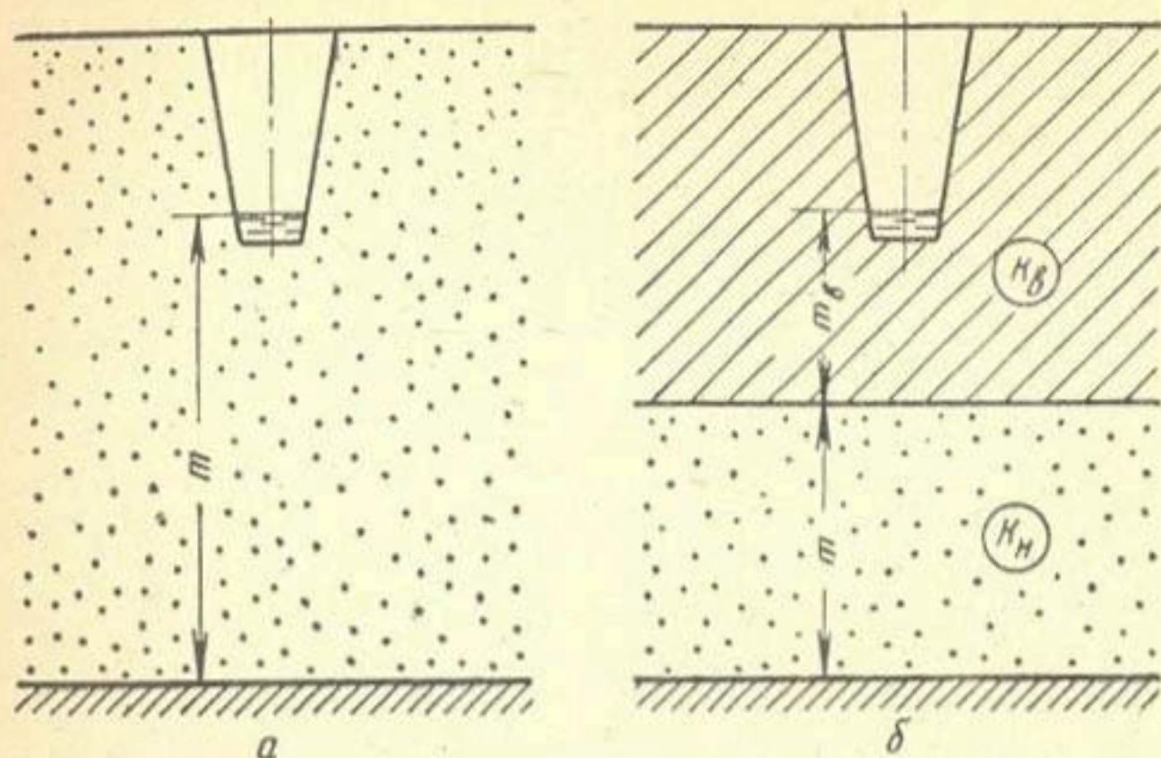
Рис. 41. Типовые схемы строения придренной области: а — однослойное; б — двухслойное с дренаем в верхнем слое.
