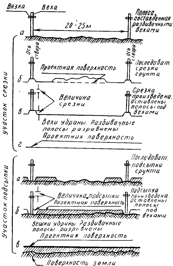
Рис. 38. Последовательность разработки полосы при ее планировке (по схеме „Узгипровхоза“)
