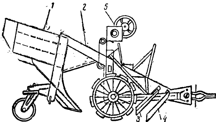
Рис. 68. Канавокопатель КМ-80У:
