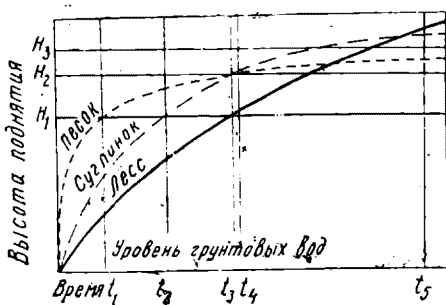
Рис. 28. Схематические кривые капиллярного подъема грунтовой воды разными грунтами (по С. И. Тюремову)
