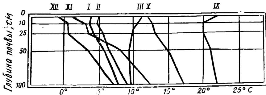
Рис. 52. Температуры почвы Голодностепской опытной станции (средние за месяц)
