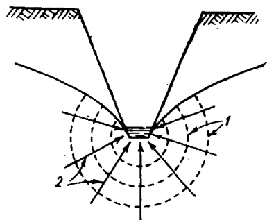
Рис. 63. Схема движения грунтовых вод к дренаю:
