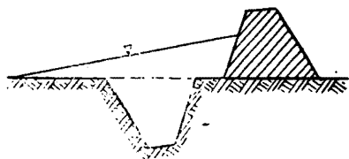
Рис. 101. Поперечное сечение канала и вала
