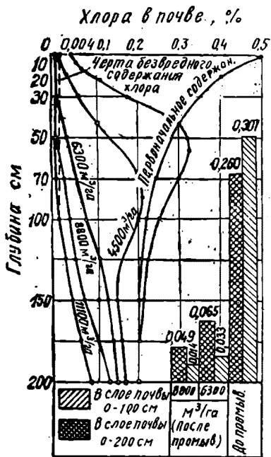
Рис. 90. Динамика вымыва хлора из почвы при промывках (М. С. Есипов)
