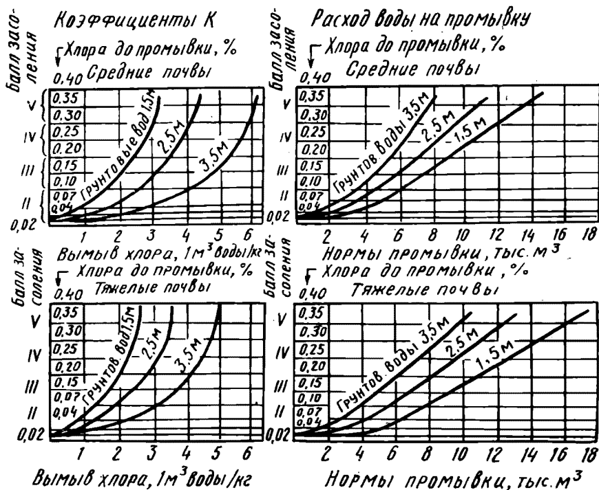
Рис. 57. Коэффициенты промывного действия воды (коэффициенты K) и затраты воды на вытеснение солей при слабом действии искусственного дренажа (А. Е. Нерозин, 1948)
