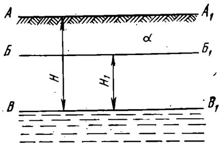
Рис. 27. Схема условий критического уровня минерализованных грунтовых вод (по Б. Б. Полюпову):
