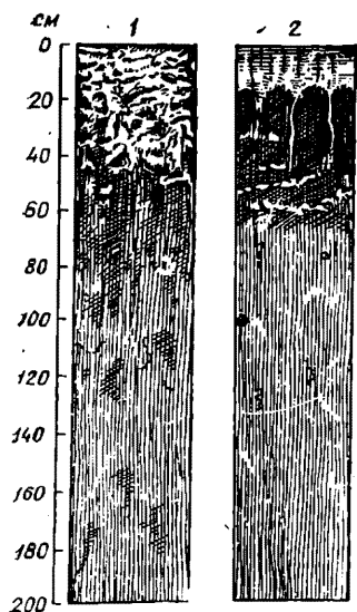
Рис. 13. Профили засоленных почв (по Г. Н. Самбур):
