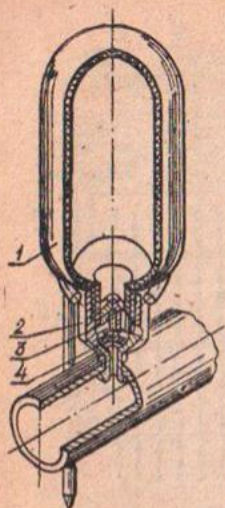
Рис. 42. Капельница-водовыпуск импульсного действия:
