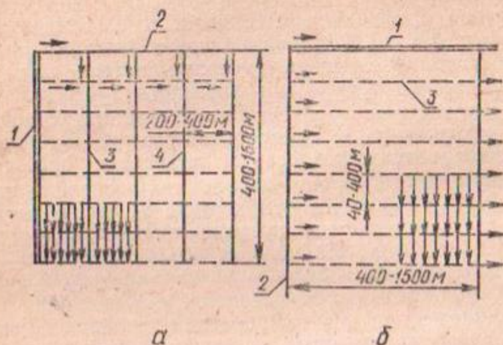
Рис. 6. Схема расположения временной оросительной сети:
