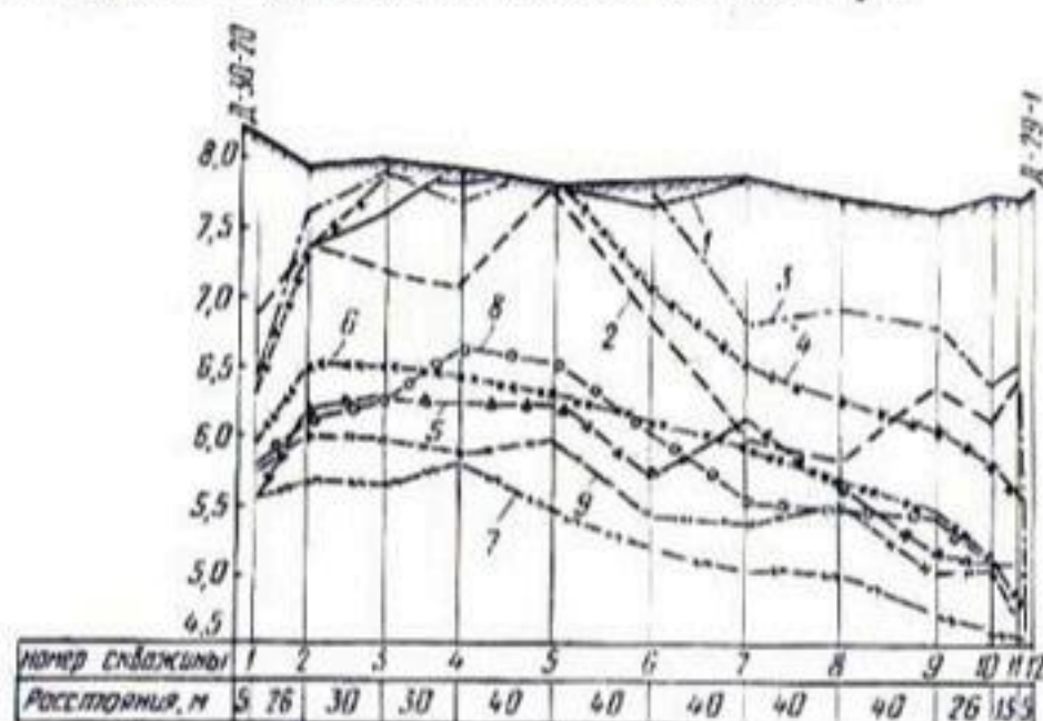
Рис. 23. Депрессионные кривые на промываемом поле в межденье Д-29-1—Д-30-20 в совхозе «Чалдовар»:
