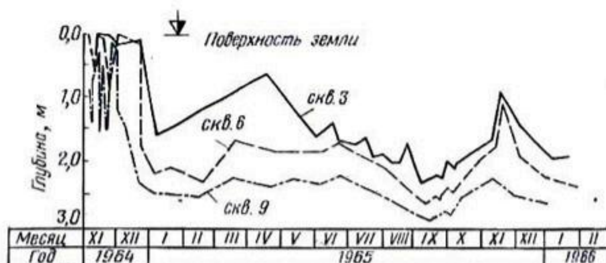
Рис. 22. Динамика уровня грунтовых вод по скважинам 3, 6, 9 в межденье Д-29-1 — Д-30-20 в совхозе «Чалдовар».
