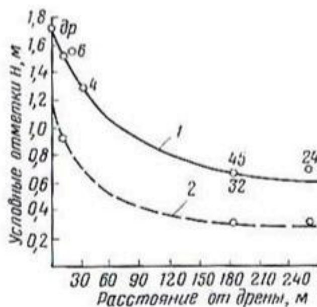
Рис. 13. Кривые снижения уровня грунтовых вод после строительства дрены, считая от первоначального уровня:
