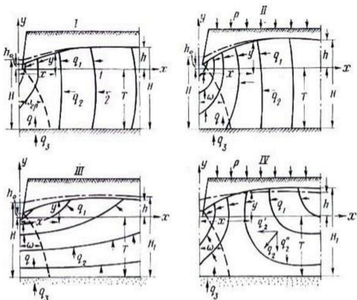
Рис. 9. Основные схемы питания горизонтального дренажа в условиях Чуйской долины:
