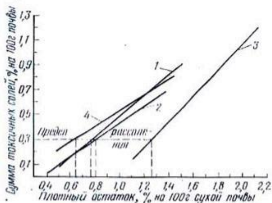
Рис. 35. Связь плотного остатка с суммой токсичных солей в метровом слое сероземно-луговых почв сульфатного типа засоления по анионам и катионам:
