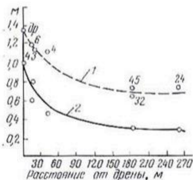
Рис. 14. Кривые снижения пьезометрического напора на глубине 8 м от поверхности земли после строительства дрены:
