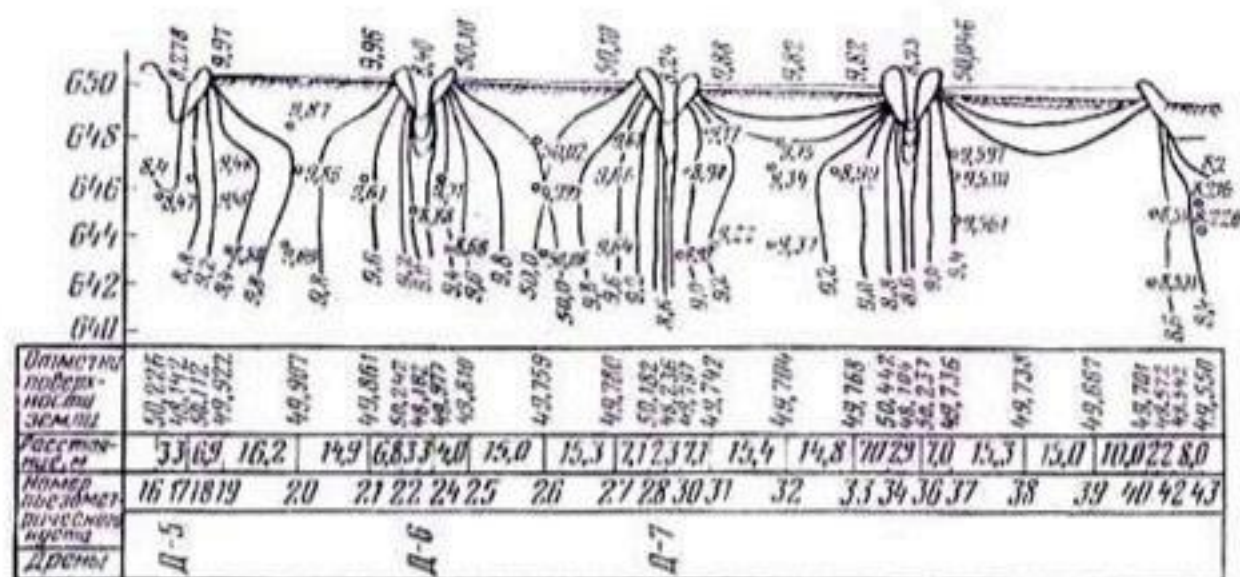
Рис. 8. Линии равных напоров в сфере действия временных дрен на опытном участке в колхозе «Победа».
