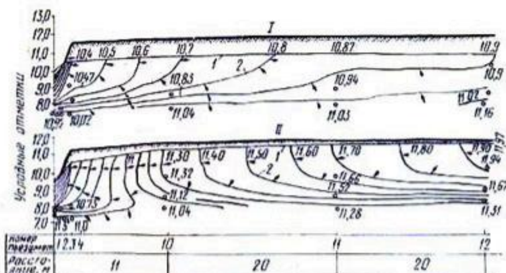
Рис. 6. Распределение напоров в сфере действия дрены:
