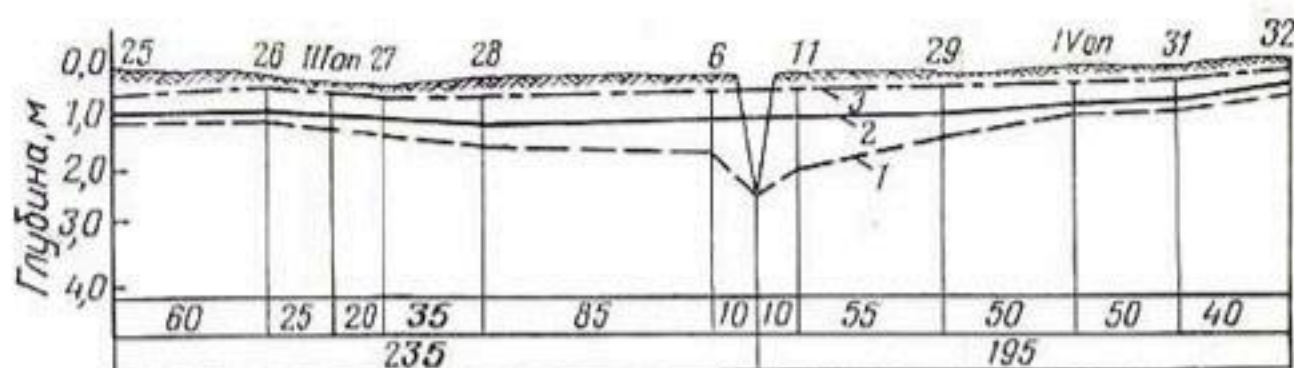
Рис. 16. Уровень грунтовых вод по створу наблюдательных скважин перпендикулярно дрене:
