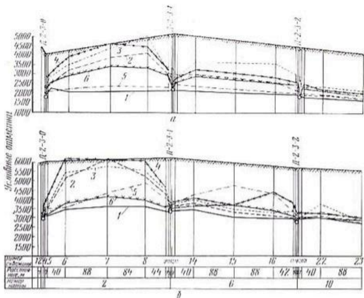
Рис. 39. Динамика уровня грунтовых вод в междуренье Д-2-3-0—Д-2-3-1 (при промывках засоленных земель) и в соседнем междуренье Д-2-3-1—Д-2-3-2 (при отсутствии промывок):
