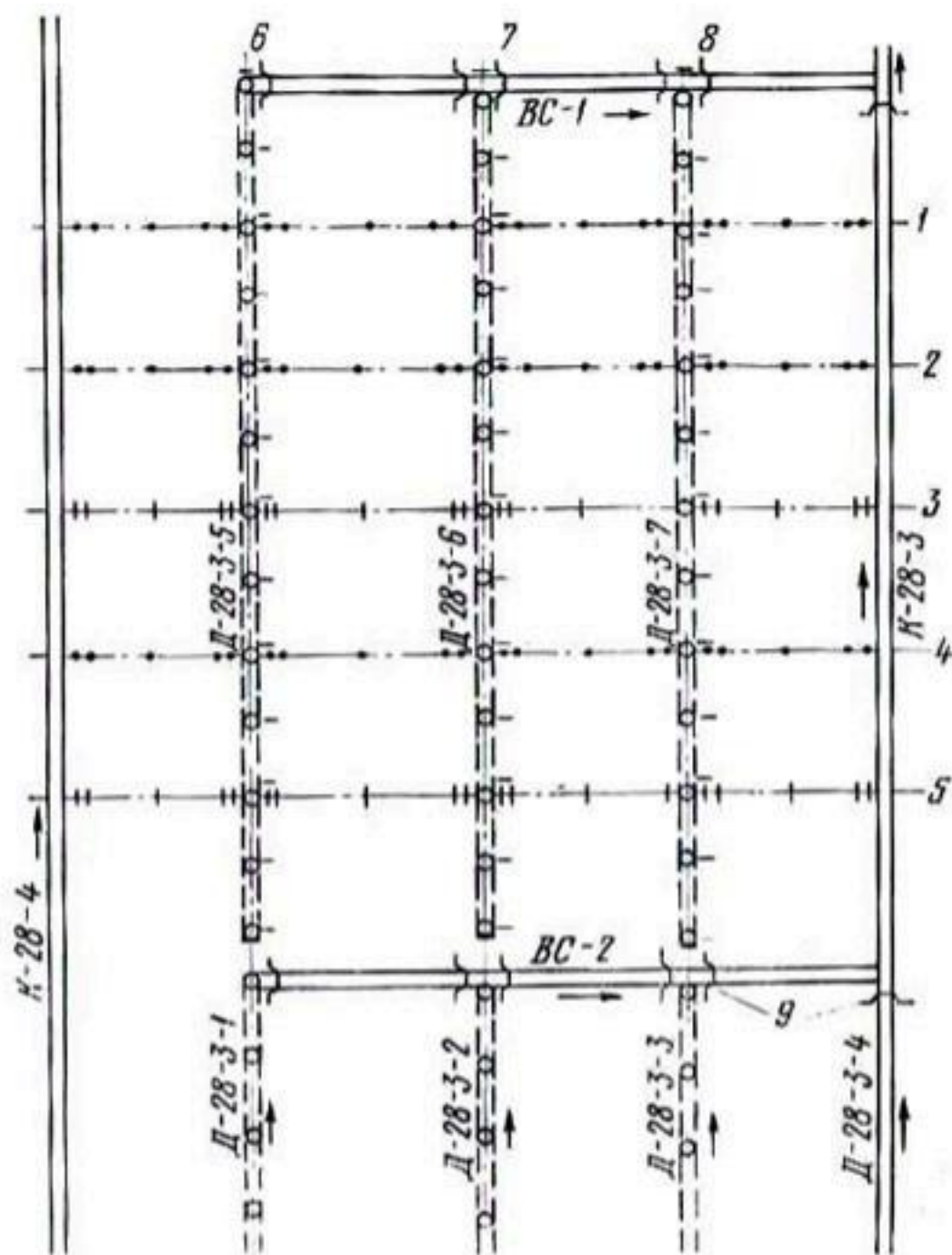
Рис. 4. Схема опытного участка закрытого горизонтального дренажа в колхозе «Победа»:
