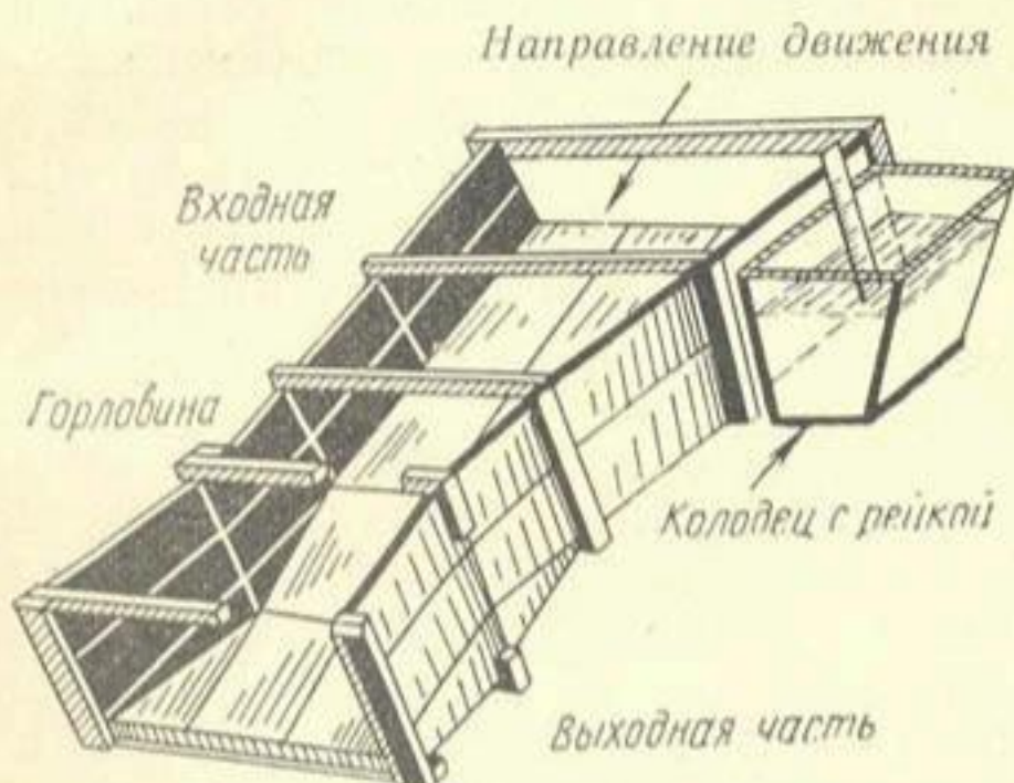
Рис. 23. Открытый водомерный лоток со сжатой горловиной.
