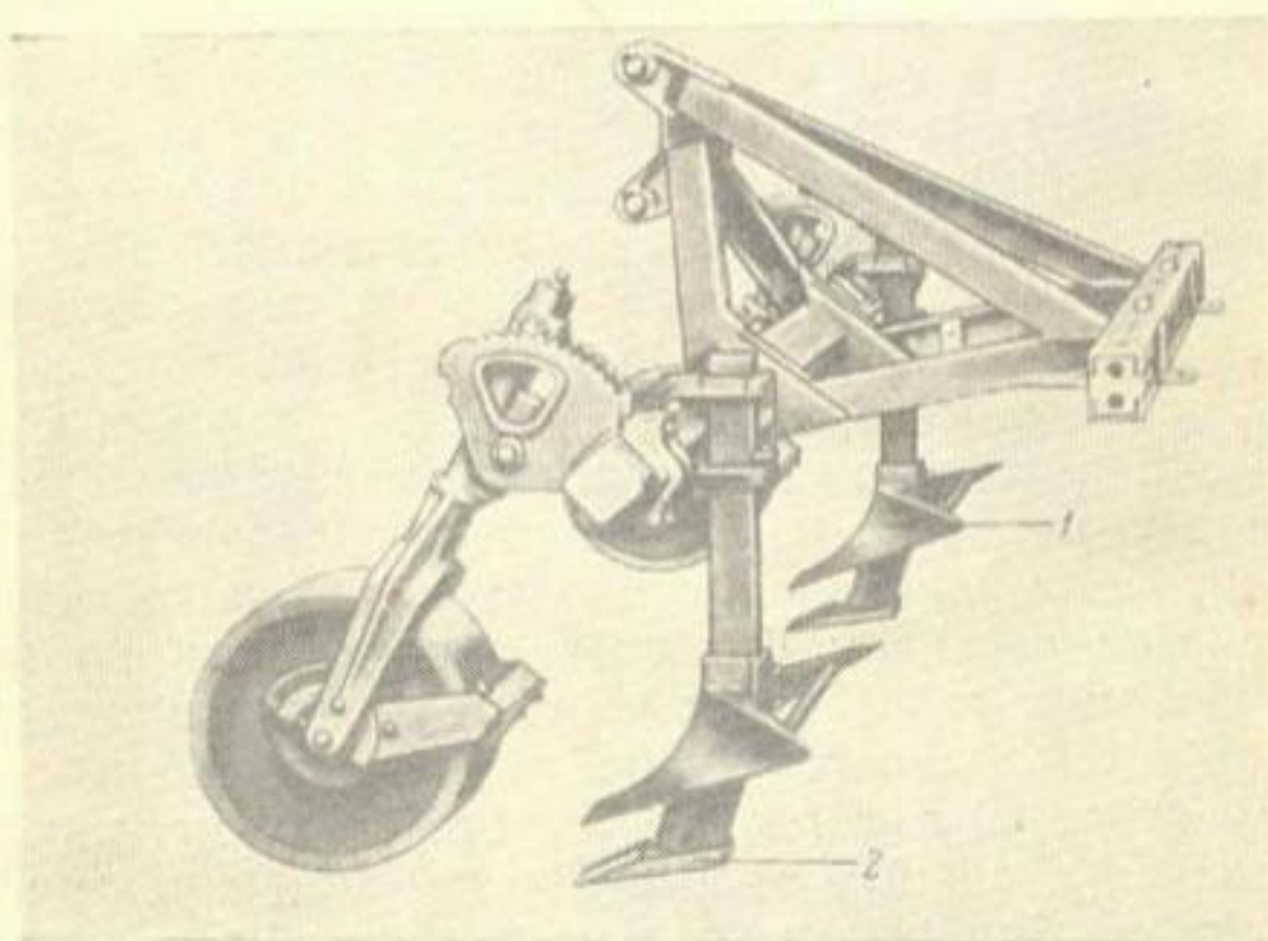
Рис. 30. Бороздодел-щелерез: 1 — двухотвальный бороздорез; 2 — долотообразный лемех.
