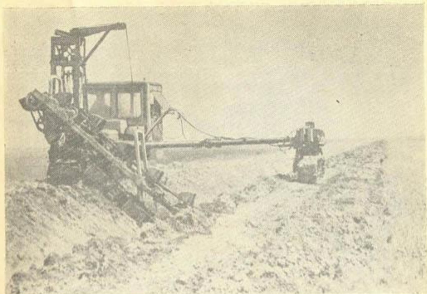
Рис. 13. Многоковшовый экскаватор ЭМ-152А в работе (Генераловская оросительная система).
