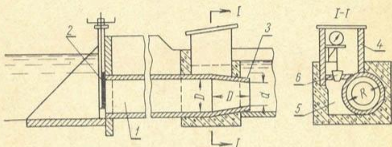
Рис. 19. Трубчатый водомер-регулятор с насадком:
