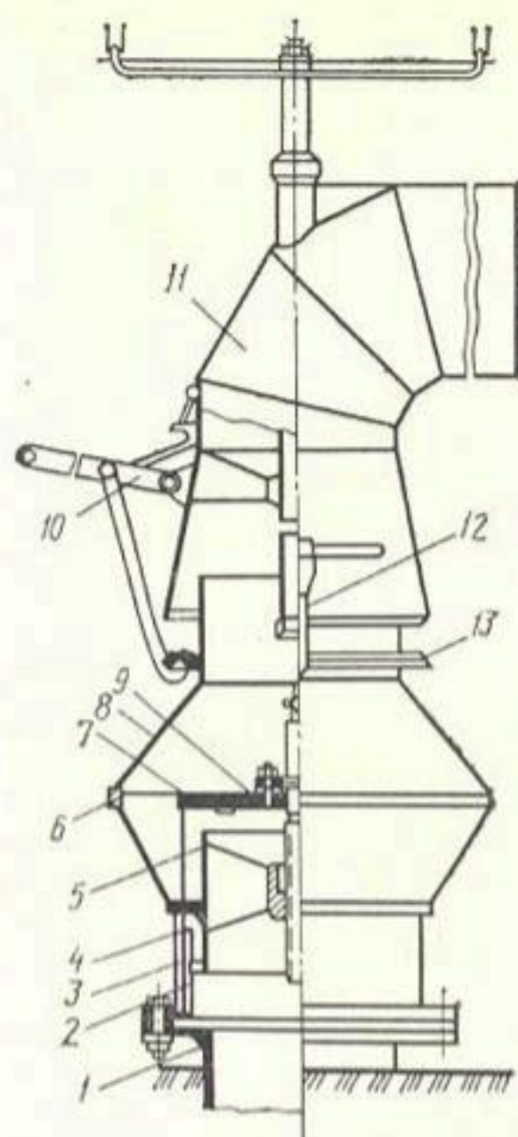
Рис. 4.15. Гидрант-водовыпуск ГВ-3:
