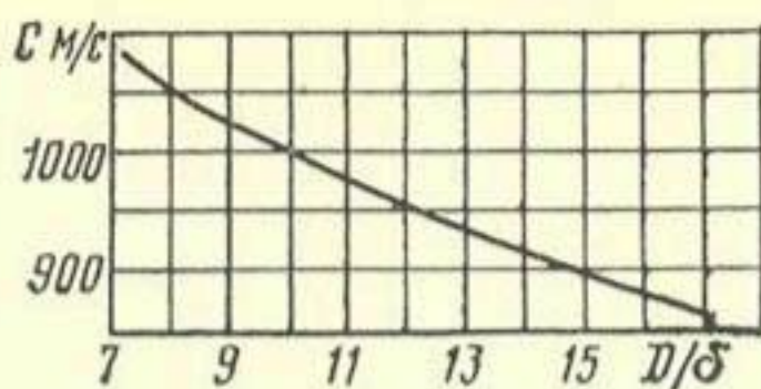
Рис. 5.2. Зависимость скорости распространения ударных волн c вдоль трубопровода от отношения D/\delta для асбестоцементных труб.
