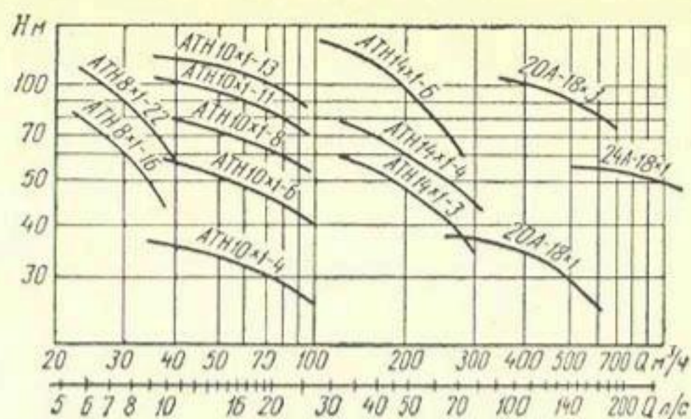
Рис. 2.20. Сводные характеристики насосов типа АТН и А.
