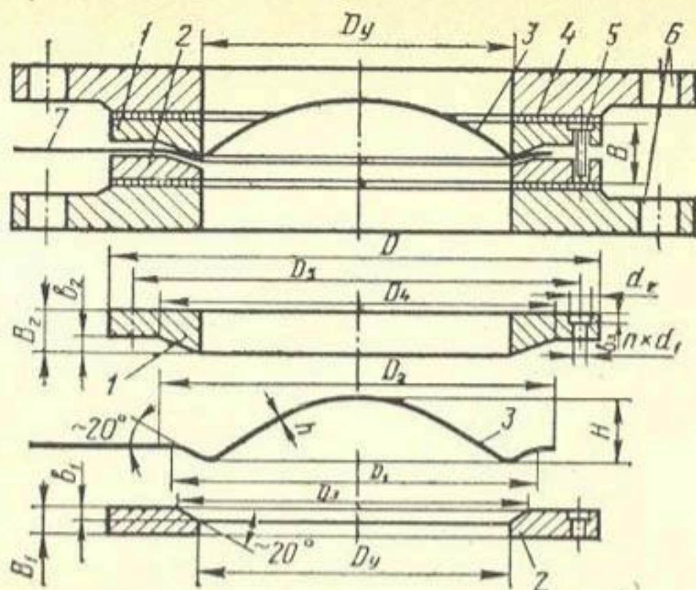
Рис. 5.17. Предохранительное устройство с разрывной мембраной:
