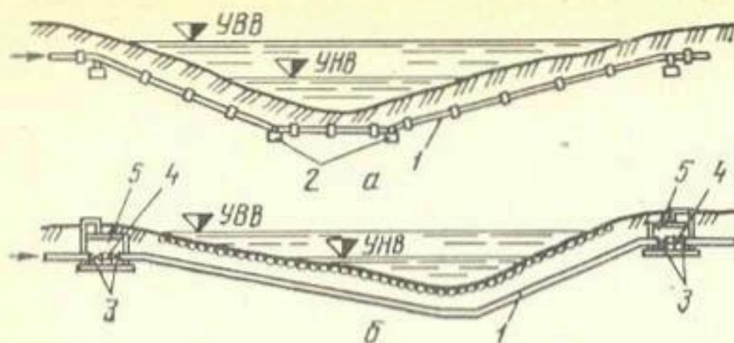
Рис. 6.1. Схемы дюкеров:
