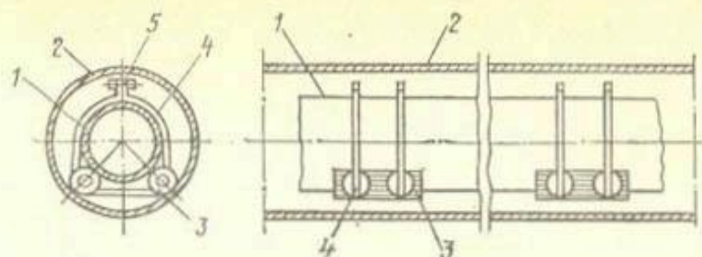
Рис. 6.9. Деревянные опоры под трубы:
