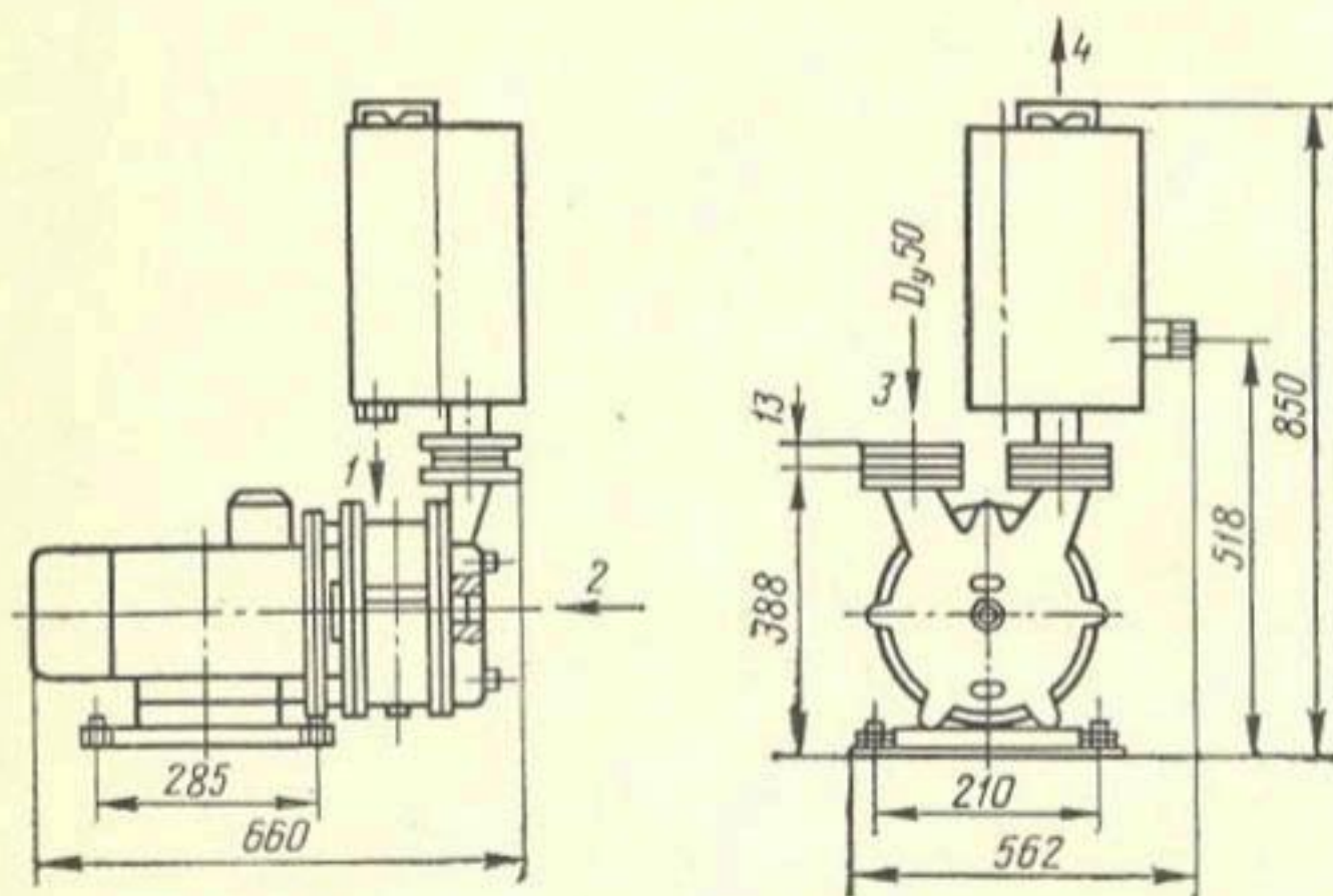
Рис. 2.23. Водокольцевой вакуум-насос ВВН-1,5:
