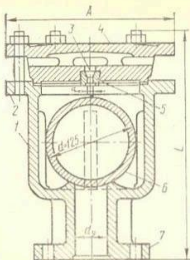
Рис. 5.20. Вантуз ВМТ-50:
