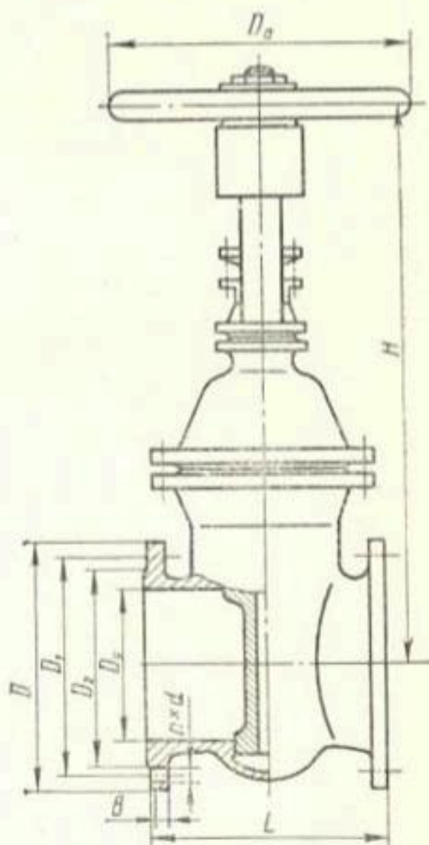
Рис. 4.2. Клиновая задвижка с невыдвижным шпинделем с ручным приводом (30ч476р).
