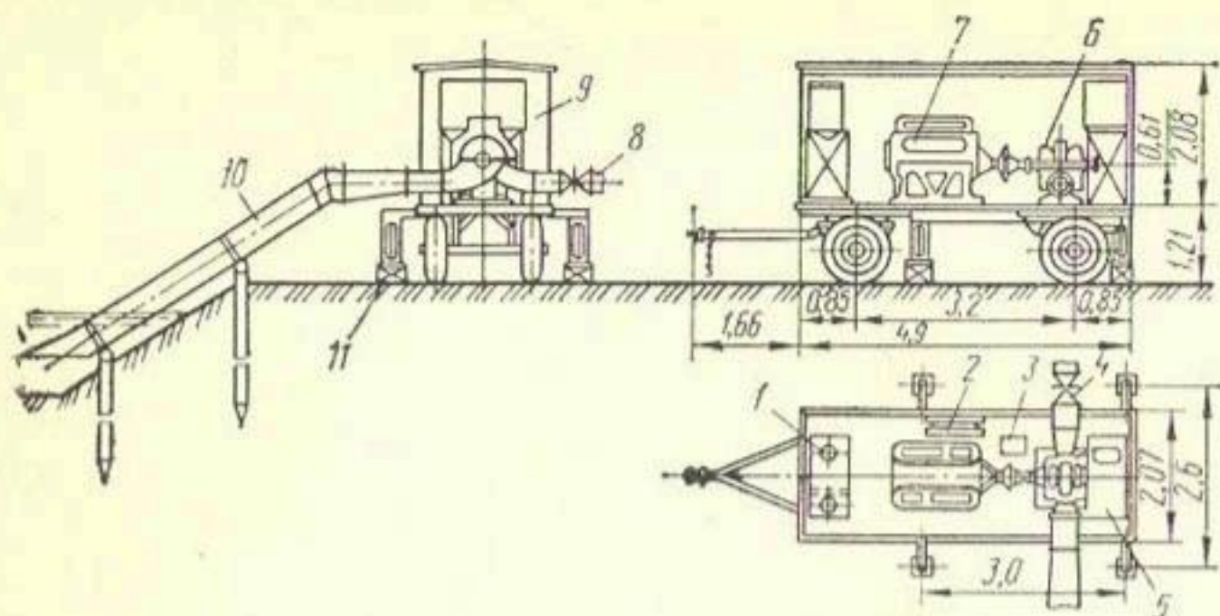
Рис. 2.31. Прицепная насосная станция:
