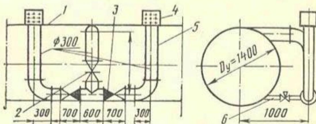
Рис. 5.13. Установка обратных клапанов для впуска и защемления воздуха при гидравлических ударах:
