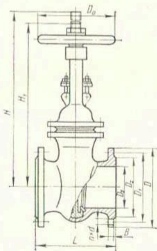
Рис. 4.1. Клиновая задвижка с выдвижным шпинделем с ручным приводом 31чбнж).
