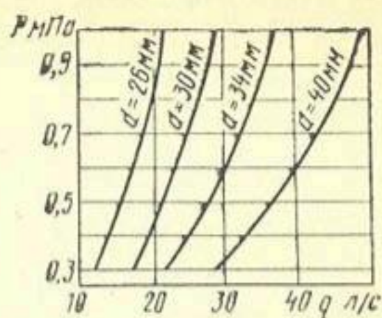
Рис. 5.7. Расходно-напорные характеристики ПСУ-100.
