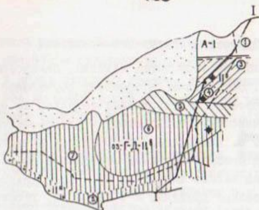
Рис. 53. Карта гидрогеологического районирования Кресоазовианского орошаемого массива в связи с оценкой условий применения вертикального дренажа
