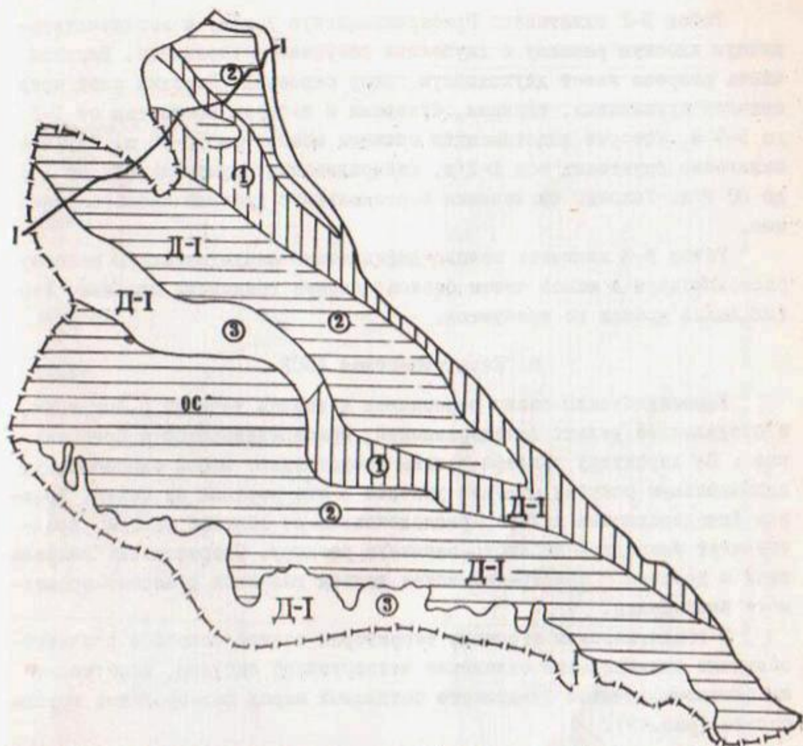
Рис.48. Карта гидрогеологического районирования Хорезмского оазиса в связи с оценкой условий применения вертикального дренажа (Условные обозначения см. по рис.37)
