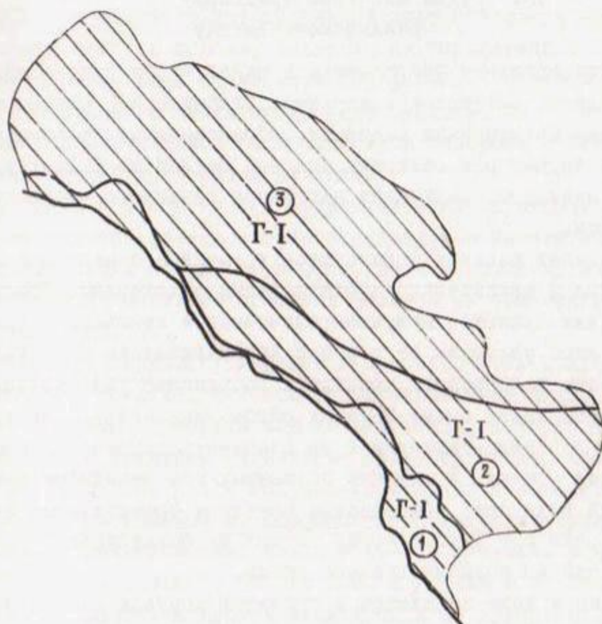
Рис.15. Схематическая карта гидрогеологического районирования Баканасского массива орошения в связи с оценкой условий применения вертикального дренажа (Условные обозначения см. по рис.1)
