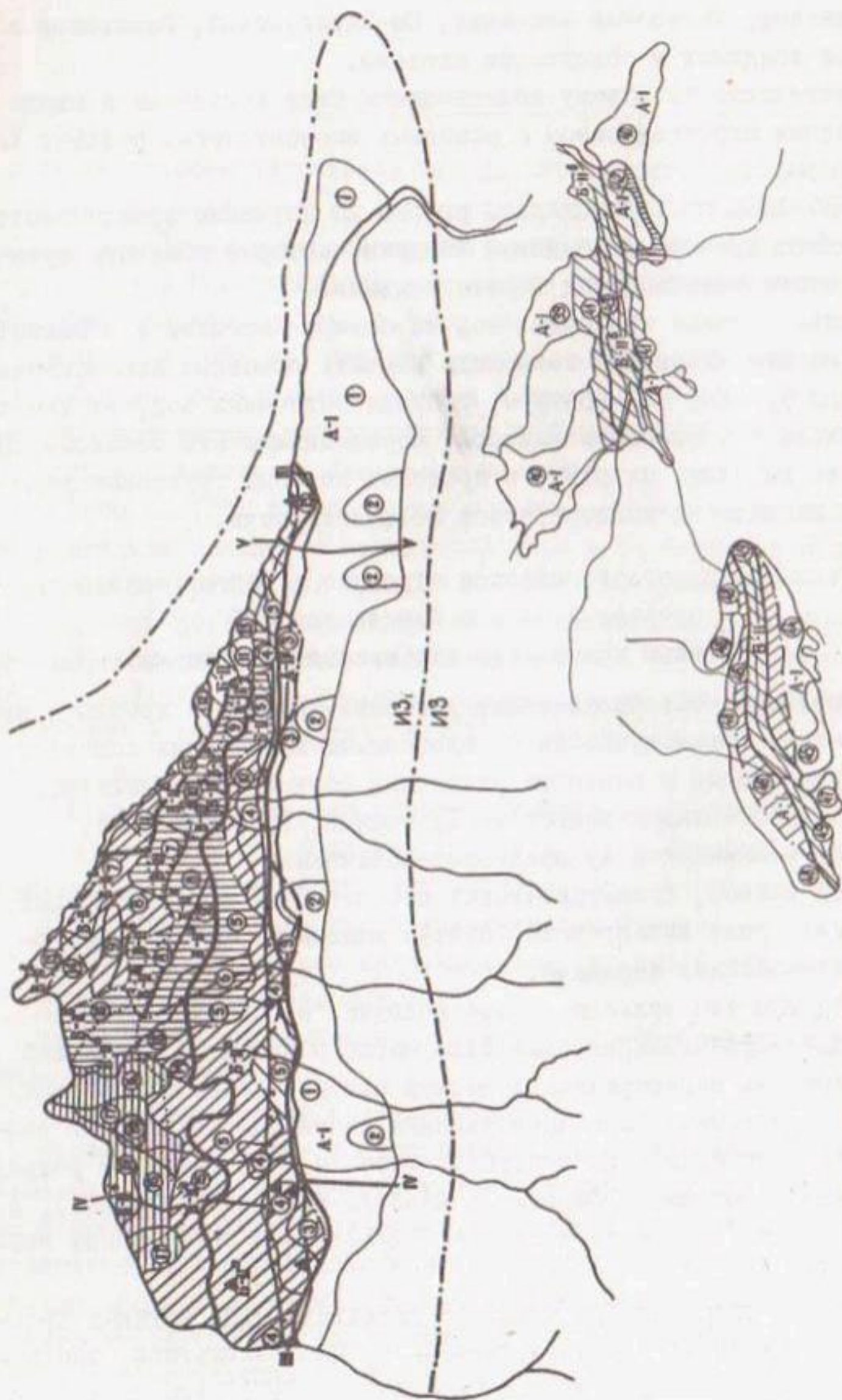
Рис. 18а. Схематическая карта гидрогеологического района северной Киргизии в связи с оценкой условий применения вертикального дренажа (Условные обозначения см. по рис. 18в)
