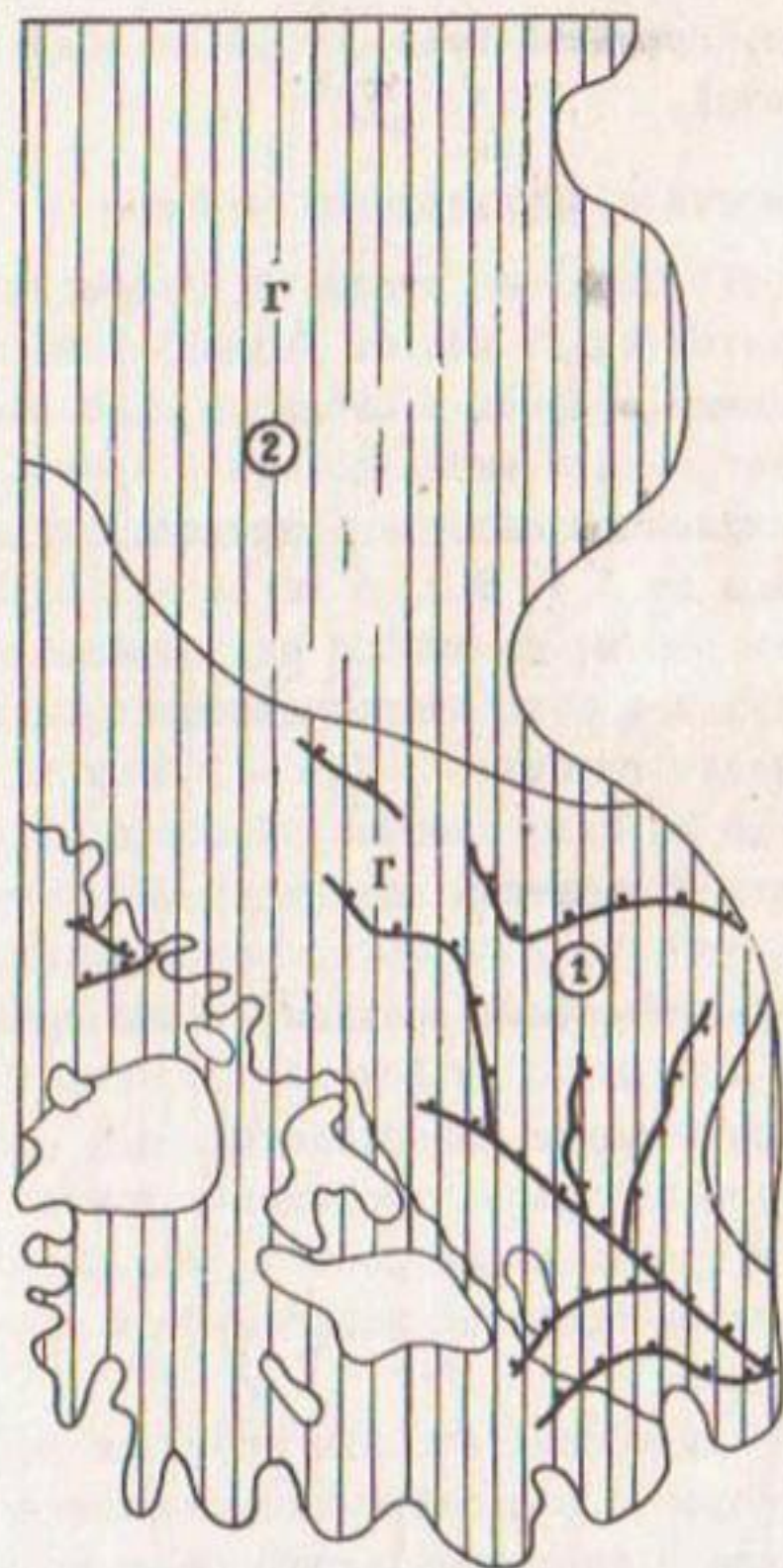
Рис.3. Схематическая карта гидрогеологического районирования Чиилийского массива орошения в связи с оценкой условий применения вертикального дренажа (Условные обозначения см. по рис. I)
