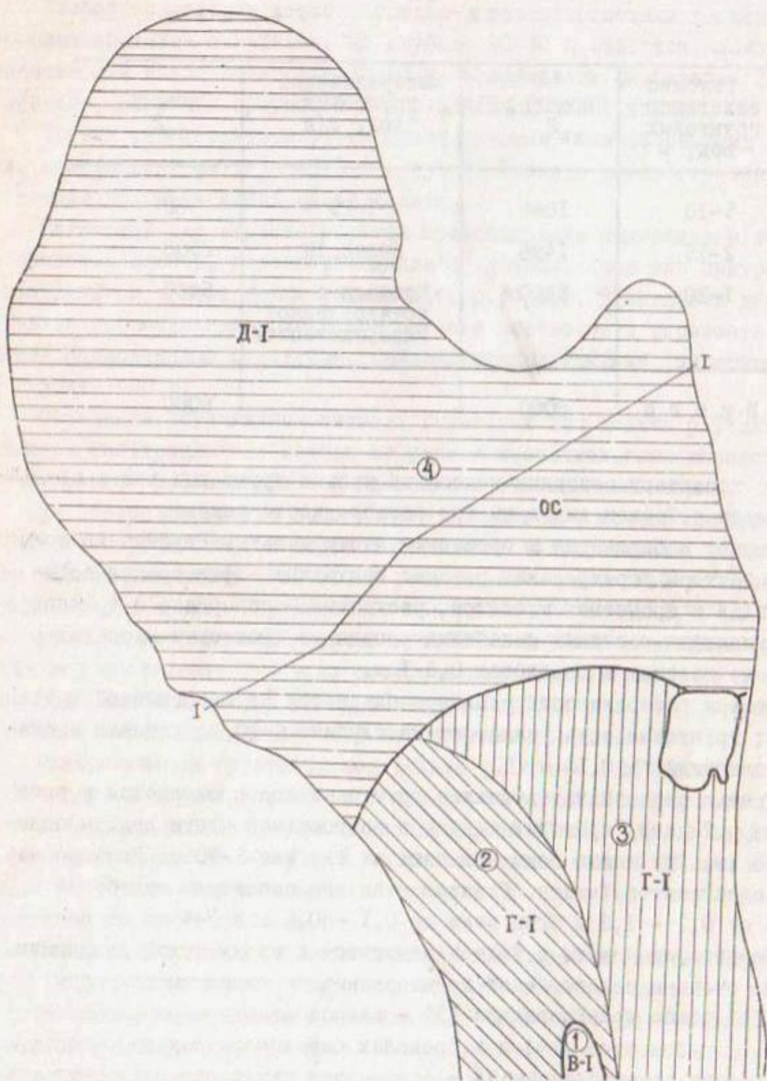
Рис.32. Карта гидрогеологического районирования субэвэральной дельты р.Тсджен в связи с оценкой условий применения вертикального дренажа (Условные обозначения см.по рис.28)
