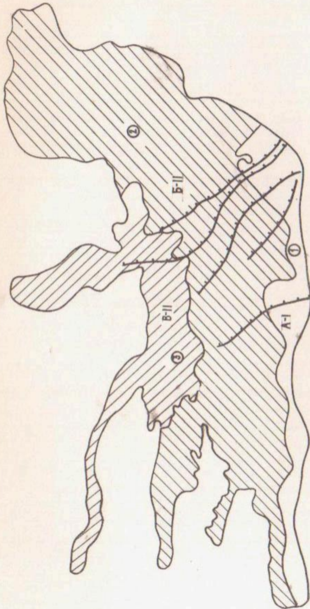
Рис. 13. Схематическая карта гидрогеологического районирования Аксуйского массива орошения в связи с оценкой условий применения вертикального дренажа (Условные обозначения см. по рис. I)
