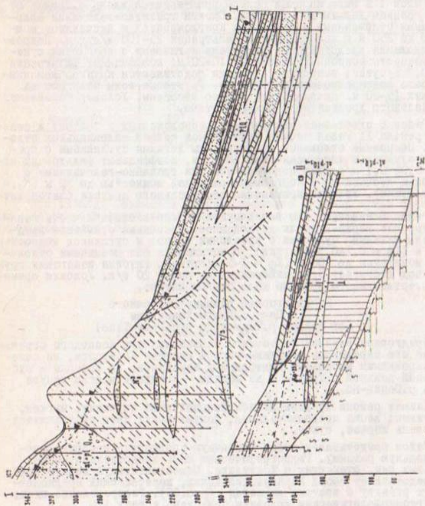
Рис. 25. Геологические разрез предгорной равнины Восточного и Центрального Копетдага по линиям I-I и II-II (Условные обозначения см. по рис. 26)
