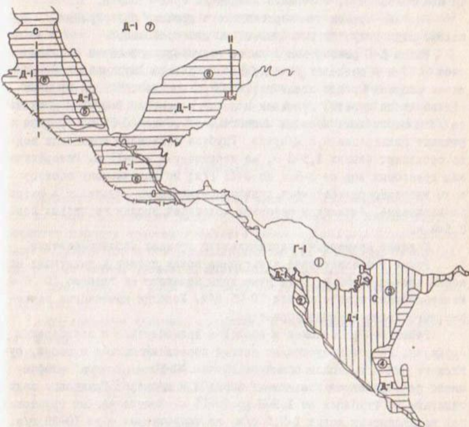
Рис.50. Карта гидрогеологического районирования Керекенлакской АССР в связи с оценкой условий применения вертикального дренажа (Условные обозначения см. по рис.87)
