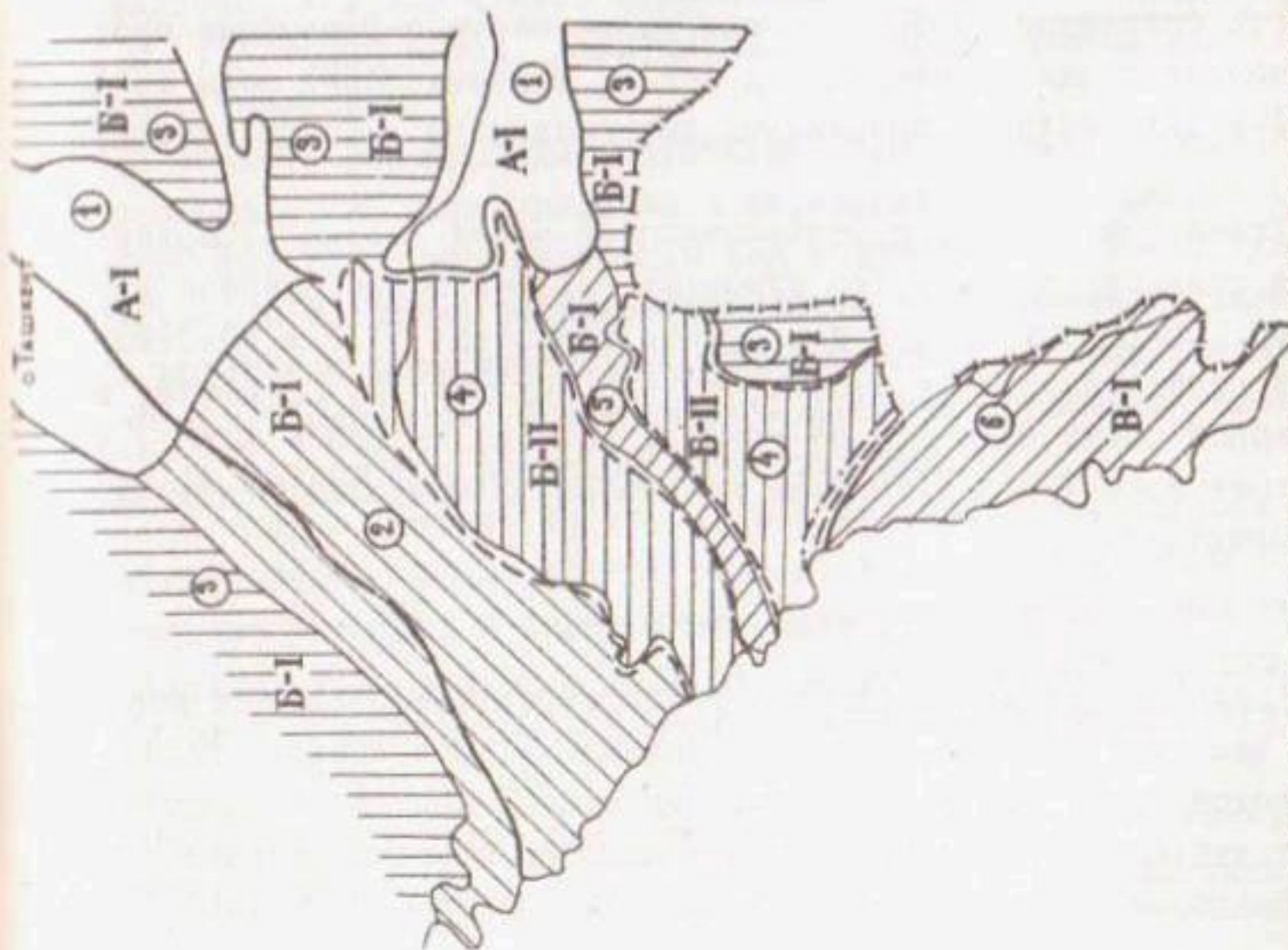
Рис. 37. Карта гидрогеологического районирования Притяженского оазиса в связи с оценкой условий применения вертикального дренажа
