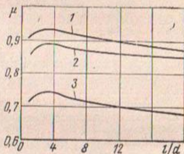
Рис. 5.17. Зависимость \mu от l/d при Re_T=10^4 : 1...3 — \alpha=10^\circ ; 30^\circ ; 90^\circ .
