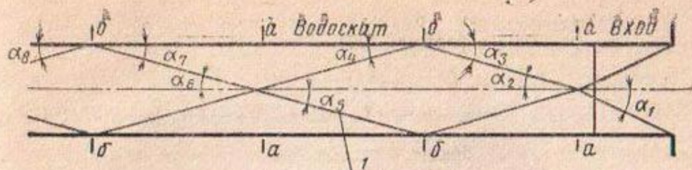
Рис. 8.9. Расчетная схема быстротока прямоугольного сечения при косых стоячих волнах.
