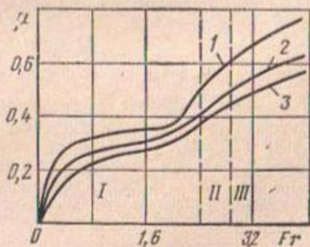
Рис. 9.6. Зависимость коэффициента расхода труб от критерия Фруда: I, II, III — соответственно безнапорная область, полунанпорная, напорная; 1...3 — l/d = 3,01; 5,91; 29,85 .
