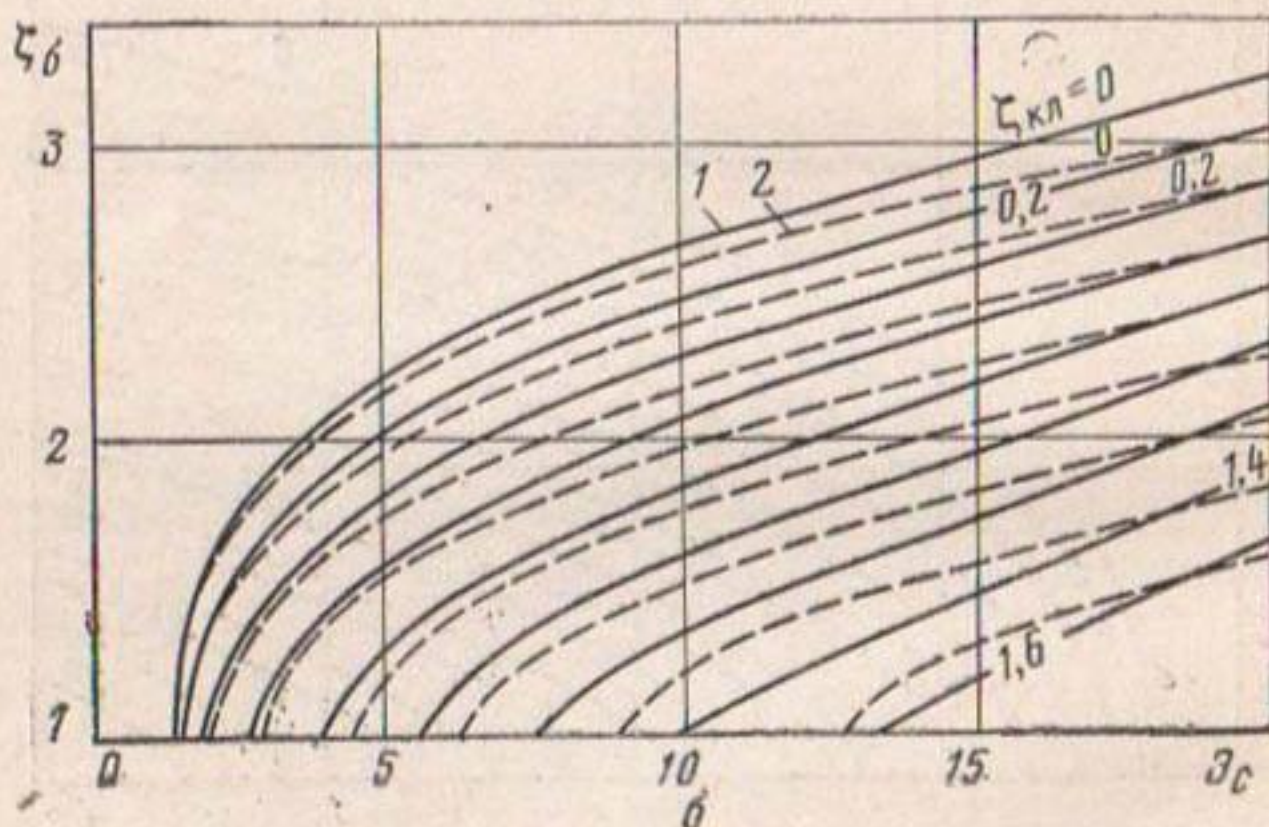
Рис. 8.8. Зависимость |\zeta_\delta| от \alpha и \zeta_{\kappa\lambda} для призматических русл трапециевидального сечения: а — y_\kappa = 0,05 и 0,1 ; б — y_\kappa = 0,15 и 0,25 (кривые даны через 0,2 ).
