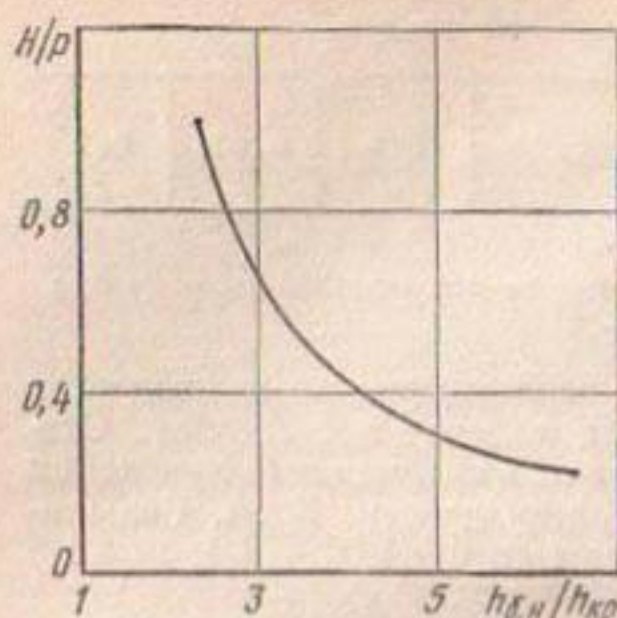
Рис. 7.7. Зависимость H/p от h_{б.н}/h_{кр} .
