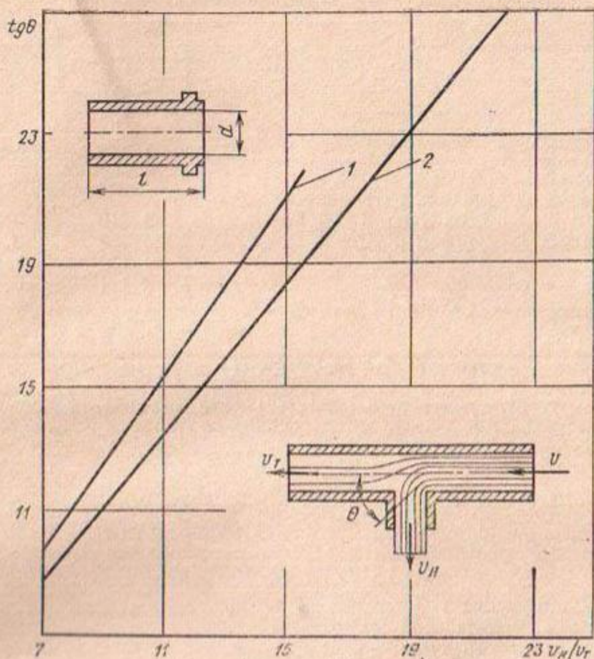
Рис. 5.23. Зависимость \theta для внешних цилиндрических насадков от v/v_T при l/d=3 : 1, 2= d —0,002 м, 0,004...0,016 м.
