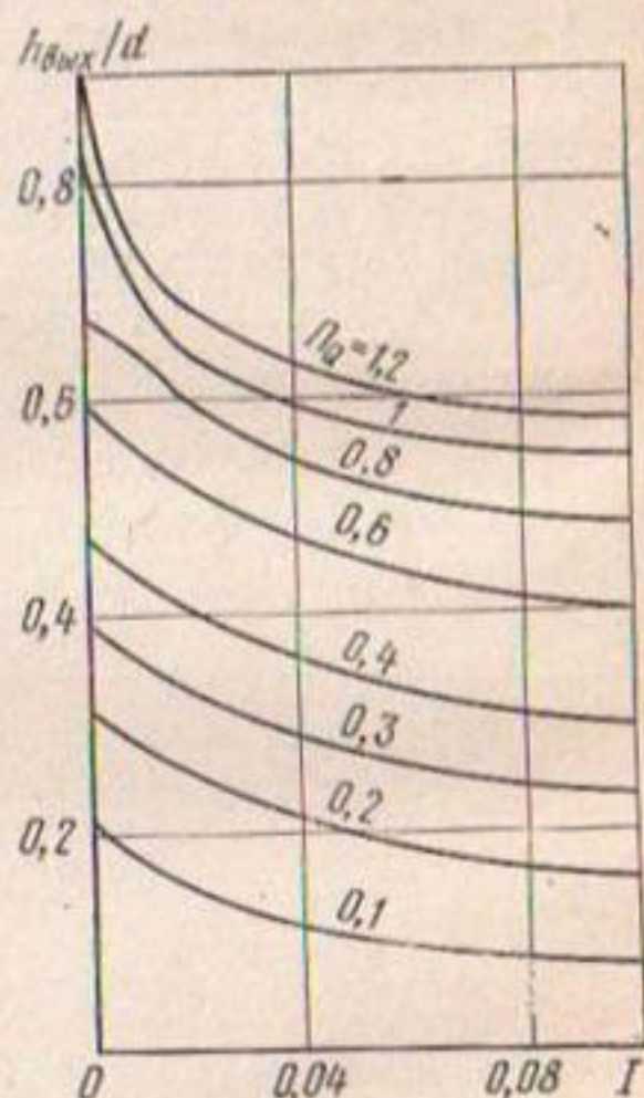
Рис. 9.3. Зависимость h_{\text{вых}}/a от P_Q и i для водопропускной трубы прямоугольного или квадратного сечения: P_Q = Q/(d \sqrt{ag}) .
