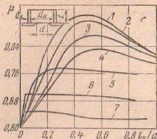
Рис. 5.2. Зависимость \mu для круглых отверстий от l_k/d и d_k/d : 1...7 — d_k/d = 1,226; 1,254; 1,306; 1,386; 1,117; 1,057; 1,008 .
