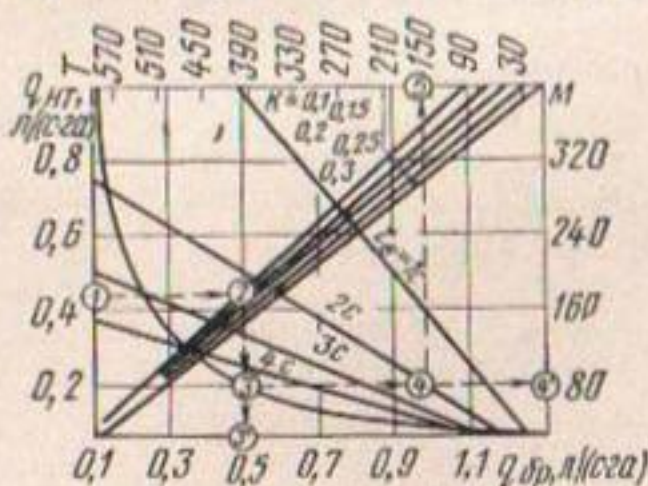
Рис. 10.8. Режим работы импульсных дождевателей ( M = (t_v + t_n) / t_n ; цифрами обозначен порядок расчета).
