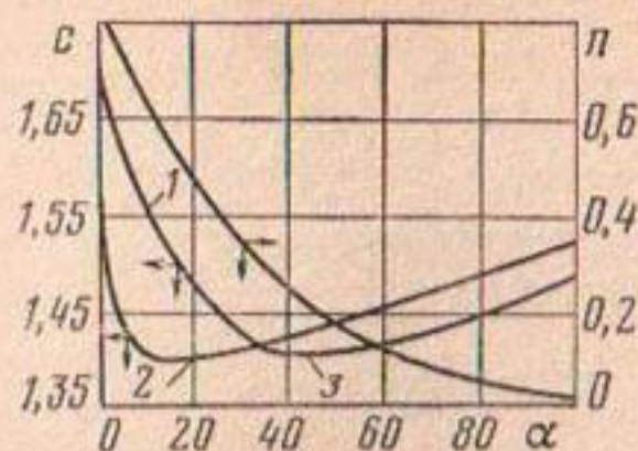
Рис. 5.5. Зависимость c и n от \alpha : 1 — l_u/d > 0,05 ; 2 — l_u \leq 0,5 ; 3 — \alpha = f(n) .
