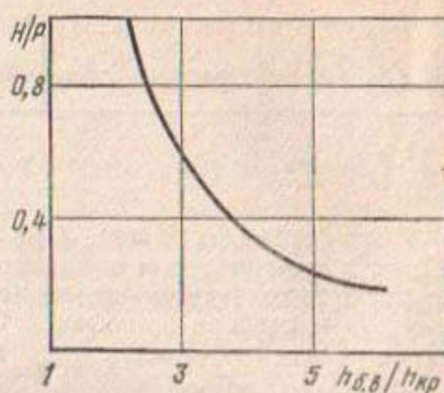
Рис. 7.8. Зависимость H/p от h_{ов}/h_{кр} .
