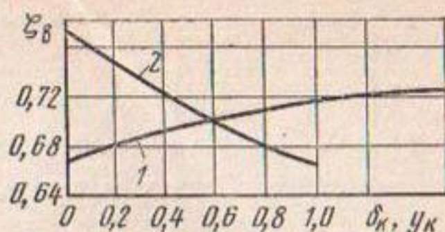
Рис. 8.4. Зависимость \zeta_b от y_k и \delta_k : 1 — \zeta_b = f_1(y_k) ; 2 — \zeta_b = f_2(\delta_k) .
