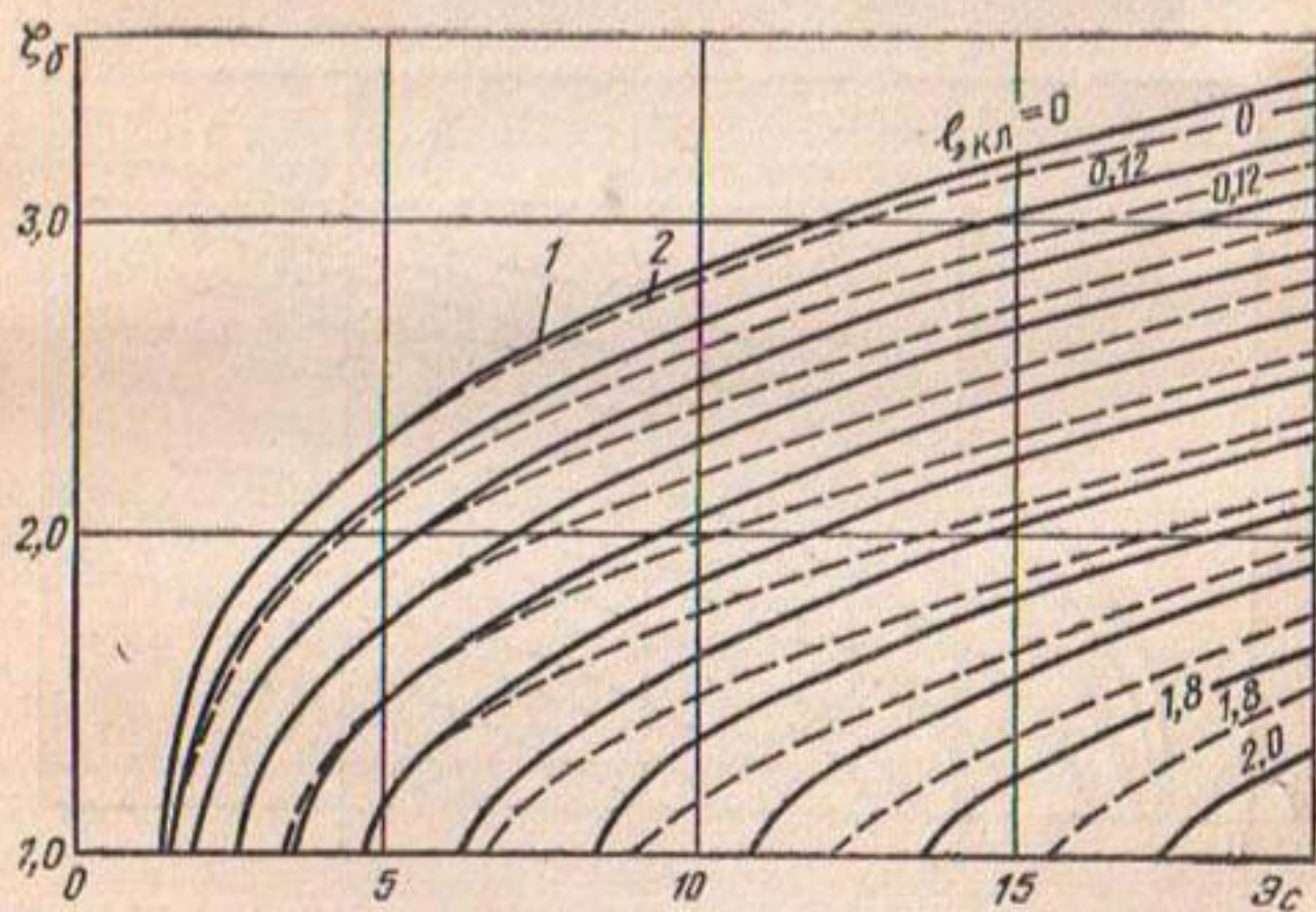
Рис. 8.7. Зависимость \zeta_{\delta} от \mathcal{E}_c и \zeta_{кп} призматических русл прямоугольного и трапецидального сечений: 1 — y_k = 0 ; 2 — y_k = 0,025 (кривые даны через 0,2).
