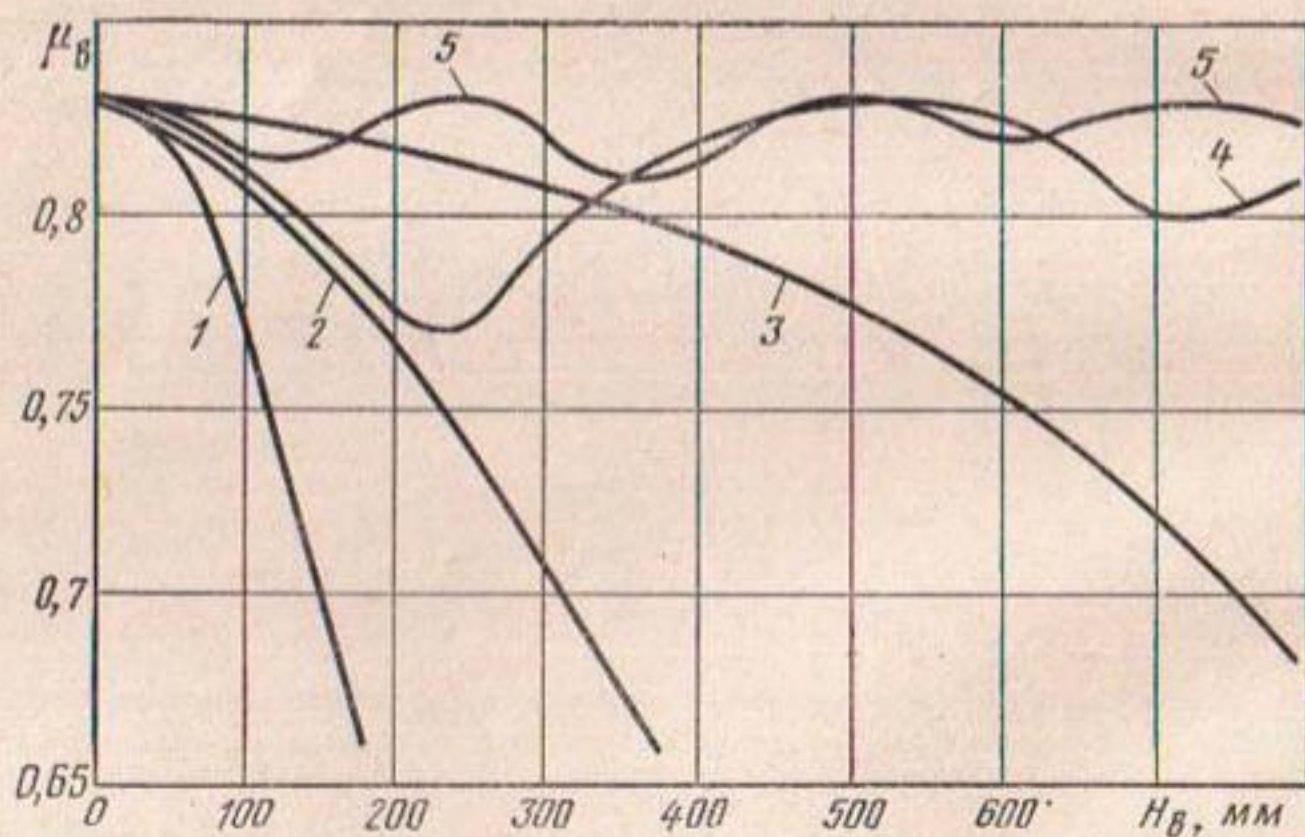
Рис. 5.28. Влияние f и вибрируемого уровня жидкости H_{\text{ж}} на \mu при d=1 мм, l/d=3 , p_2=7,85 кПа, \text{Re}_\tau=4\,300 \dots 6\,000 : 1...5— f=800 Гц; 400; 40; 40; n соответственно 2; 2; 1; 2; 4.
