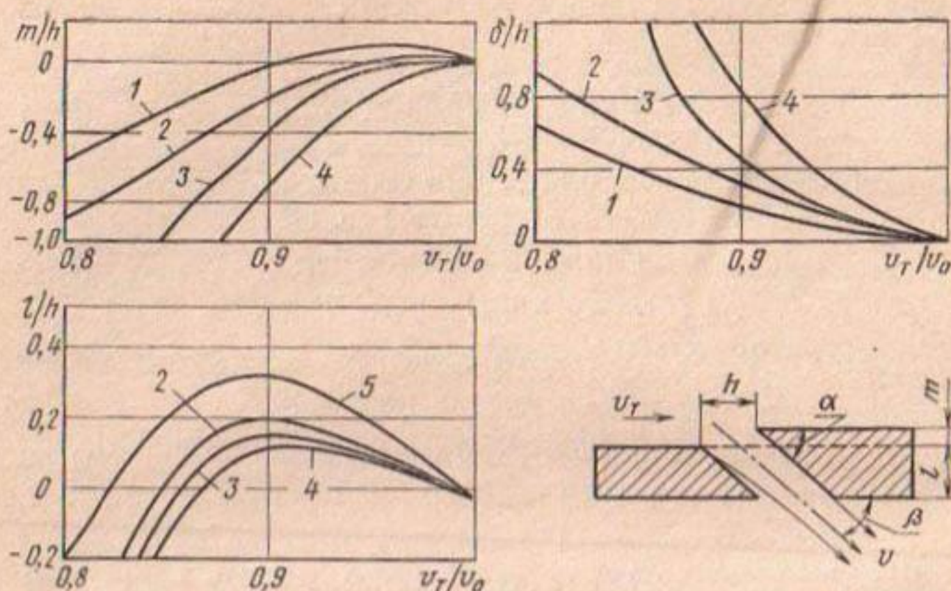
Рис. 5.19. Зависимость l/h , \delta/h , m/h от v_r/v для \alpha = 30^\circ : 1...5 — \pi/6 ; \pi/10 ; \pi/12 ; \pi/18 ; 3\pi/20 .
