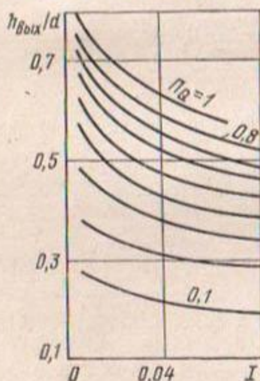
Рис. 9.2. Зависимость h_{\text{вых}}/d от P_Q и i для водопропускной трубы круглого выходного сечения: P_Q = Q/(d^2 \sqrt{dg}) (кривые даны через 0,1).
