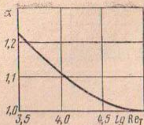
Рис. 5.4. Зависимость \alpha от Re_T .
