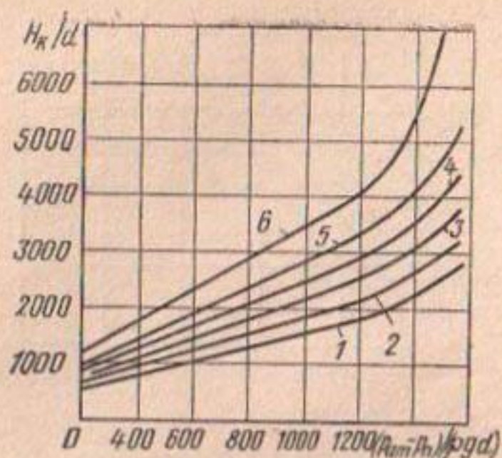
Рис. 5.10. Зависимость H_k/d от (p_{at} - p_n)/(\rho g d) : 1...6 — l/d = 10 ; 15; 20; 25; 30; 40.
