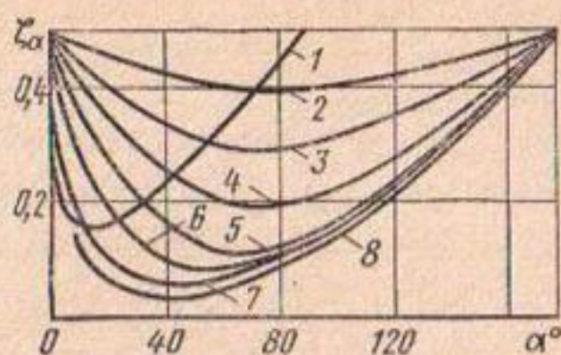
Рис. 5.6. Зависимость \zeta_\alpha от \alpha : 1 — l_u/d \leq 0,05 ; 2...8 — l_k/d = 0,025; 0,05; 0,075; 0,1; 0,15; 0,2 \dots 1,5; 2 \dots 2,5 .
