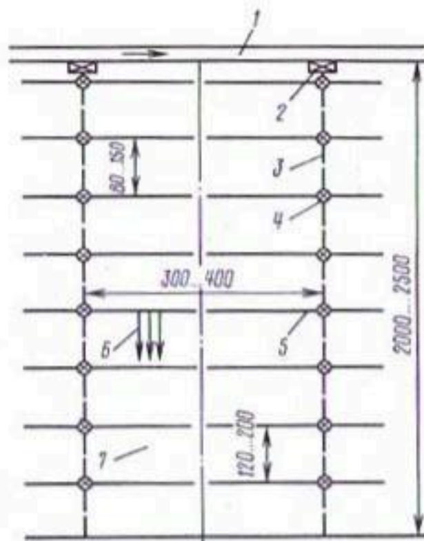
Рис. 2.7. Схема оросительной сети с применением гибких трубопроводов для уклонов 0,01...0,03:
