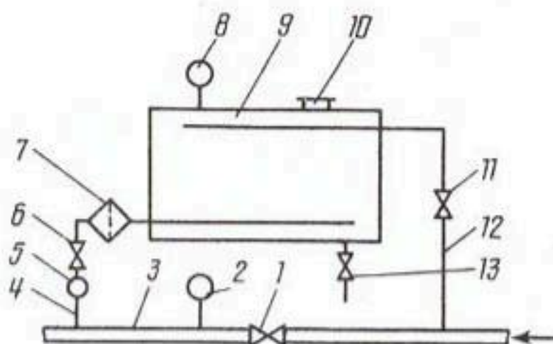
Рис. 4.10. Установка для внесения удобрений:
