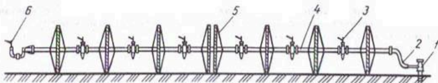
Рис. 3.13. Дождевальный колесный трубопровод ДКН-80:
