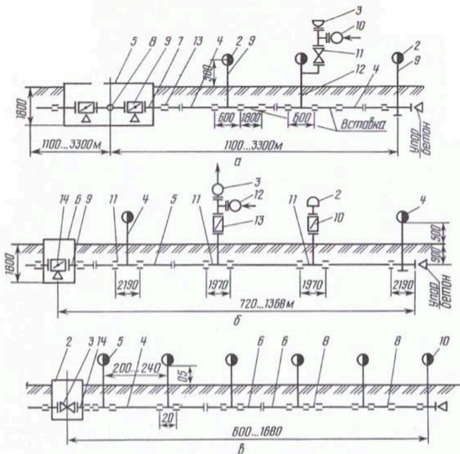
Рис. 2.18. Схема монтажа элементов поливных модулей:
