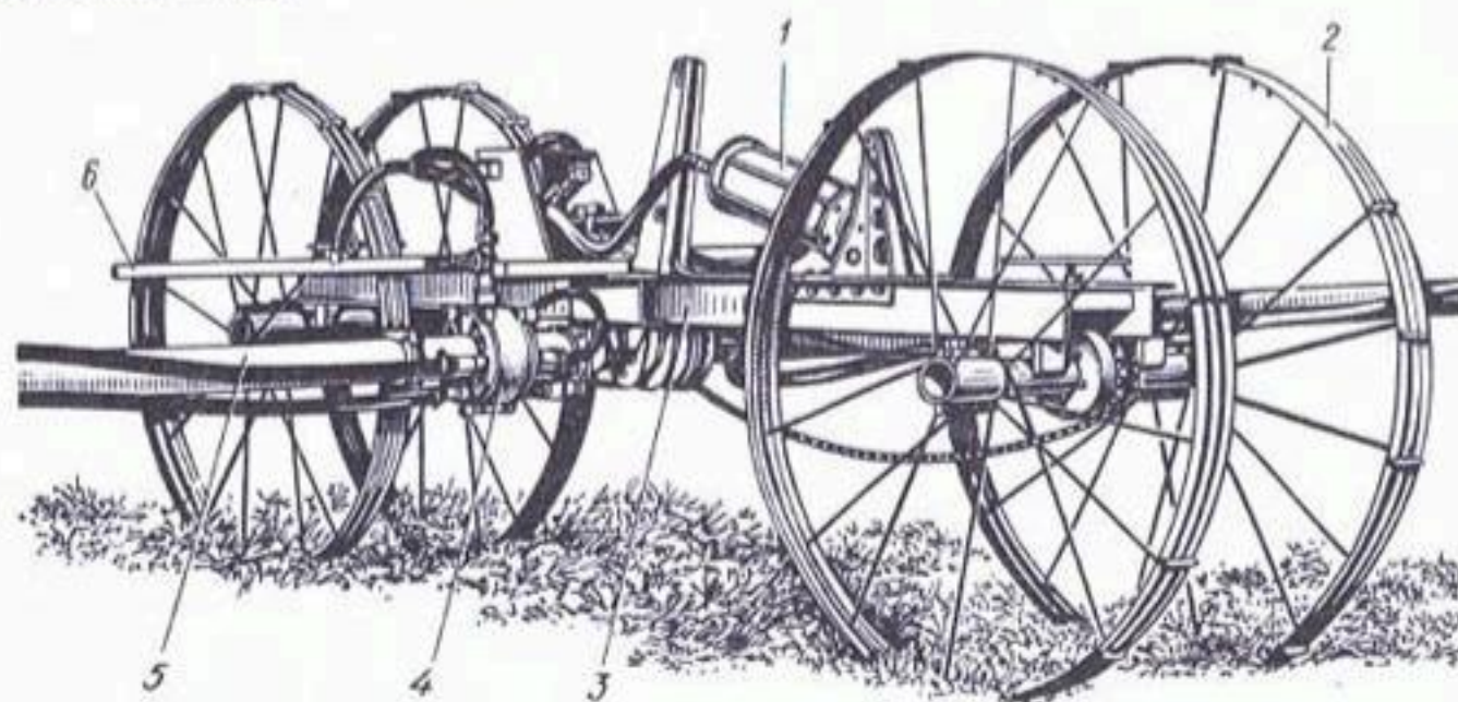
Рис. 3.10. Центральная тележка колесного трубопровода ДКГ-80 «Ока» с гидроприводом: 1 — гидродвигатель; 2 — колесо ведущее; 3 — рама; 4 — муфта обводная; 5 — трубопровод управляющий; 6 — трубка сливная
