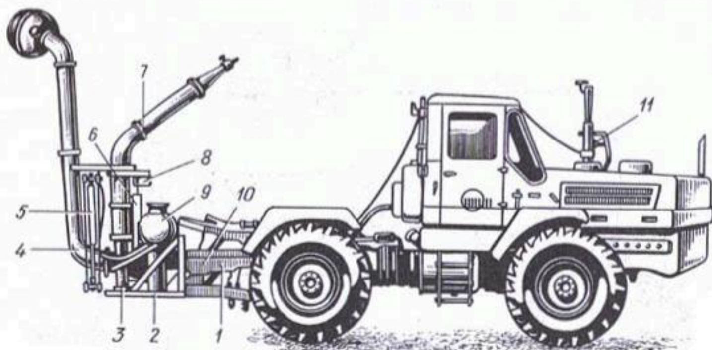
Рис. 3.23. Дальнеструйная дождевальная машина ДДН-100 навесная на трактор:
