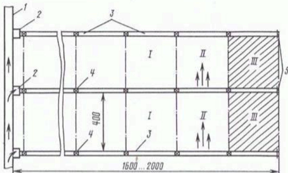
Рис. 2.19. Схема оросительной сети с автоматизированными поливными лотками:
