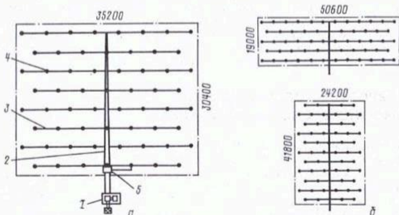
Рис. 3.60. Комплект оборудования импульсного дождевания КСИД-10А:
