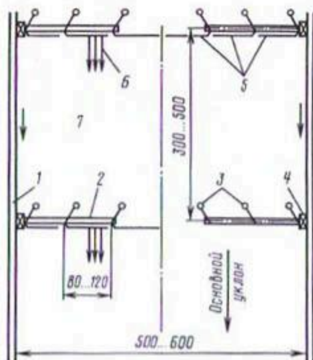
Рис. 2.6. Схема оросительной сети с применением гибких трубопроводов (продольная схема, i = 0,03...0,07 ):
