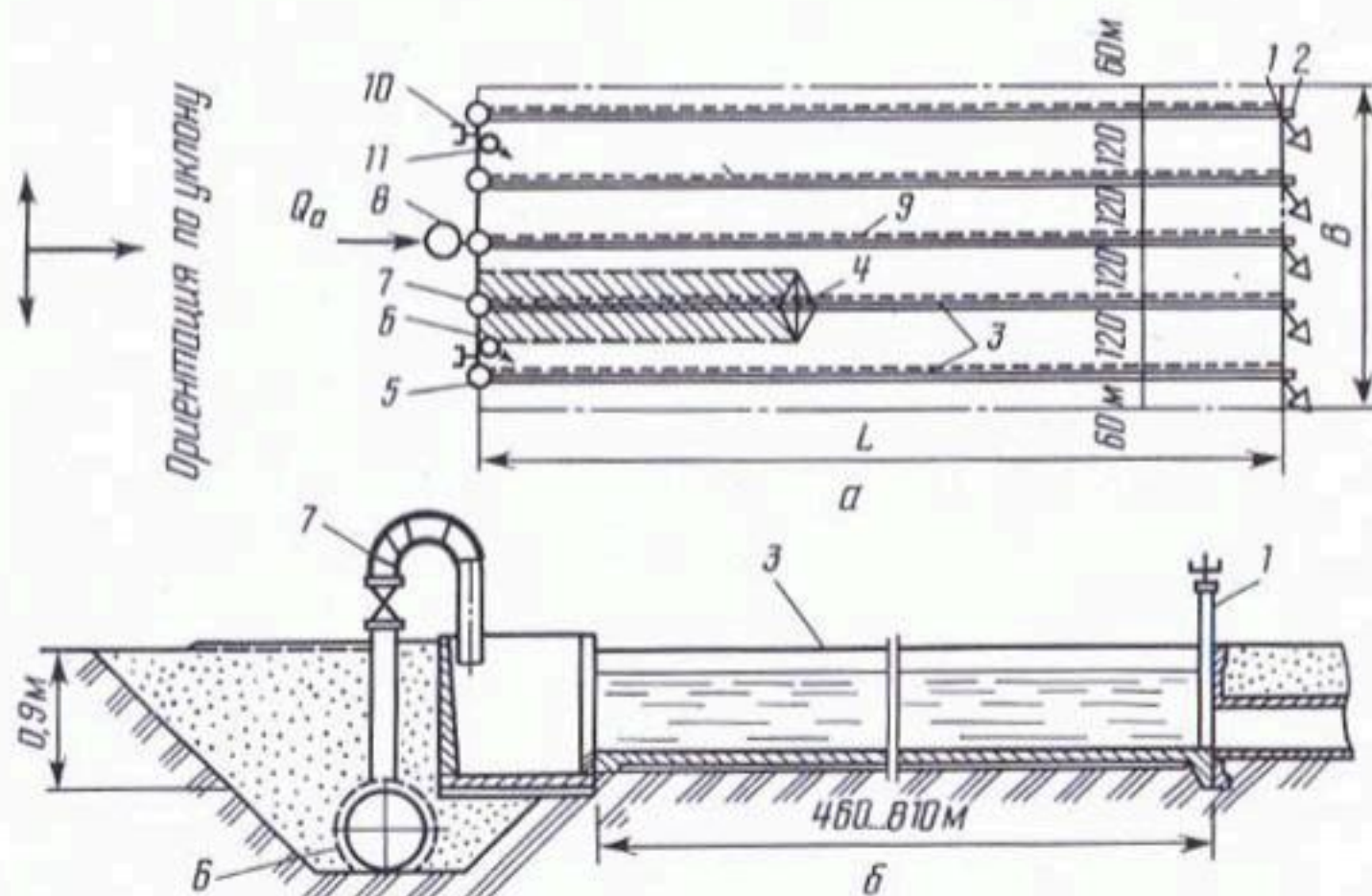
Рис. 3.52. Схема поливного модуля с двухконсольным дождевальным агрегатом ДДА-100МА, сетью из асбестоцементных труб, открытыми оросителями с монолитной бетонной облицовкой, подводом воды к торцу модульного участка (а) и его монтажа (б) (условные обозначения по табл. 3.63)
