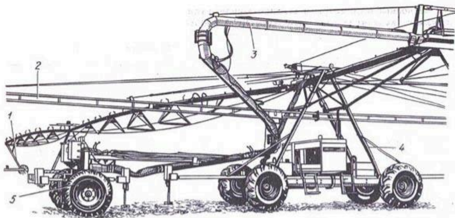
Рис. 3.53. Дождевальная машина «Таврия»:
