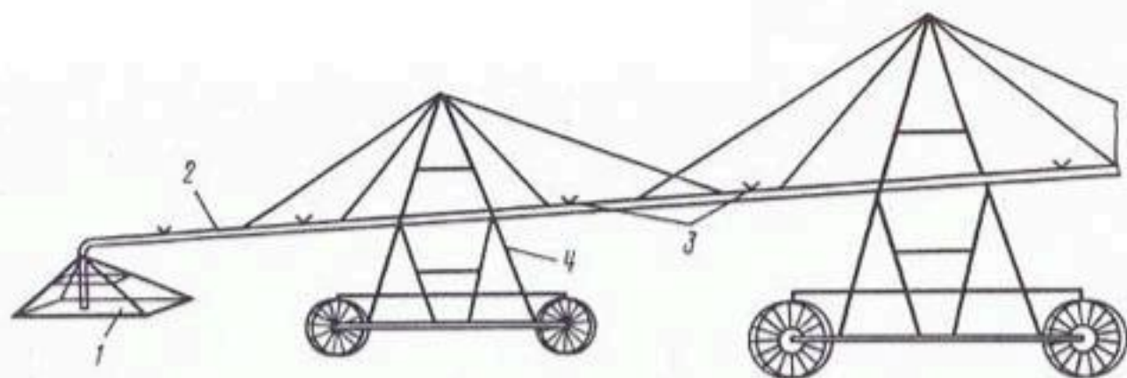
Рис. 3.33. Схема дождевальной машины ДМУ «Фрегат»: 1 — неподвижная опора; 2 — водопроводящий пояс; 3 — дождевальные аппараты; 4 — самоходная опорная тележка
