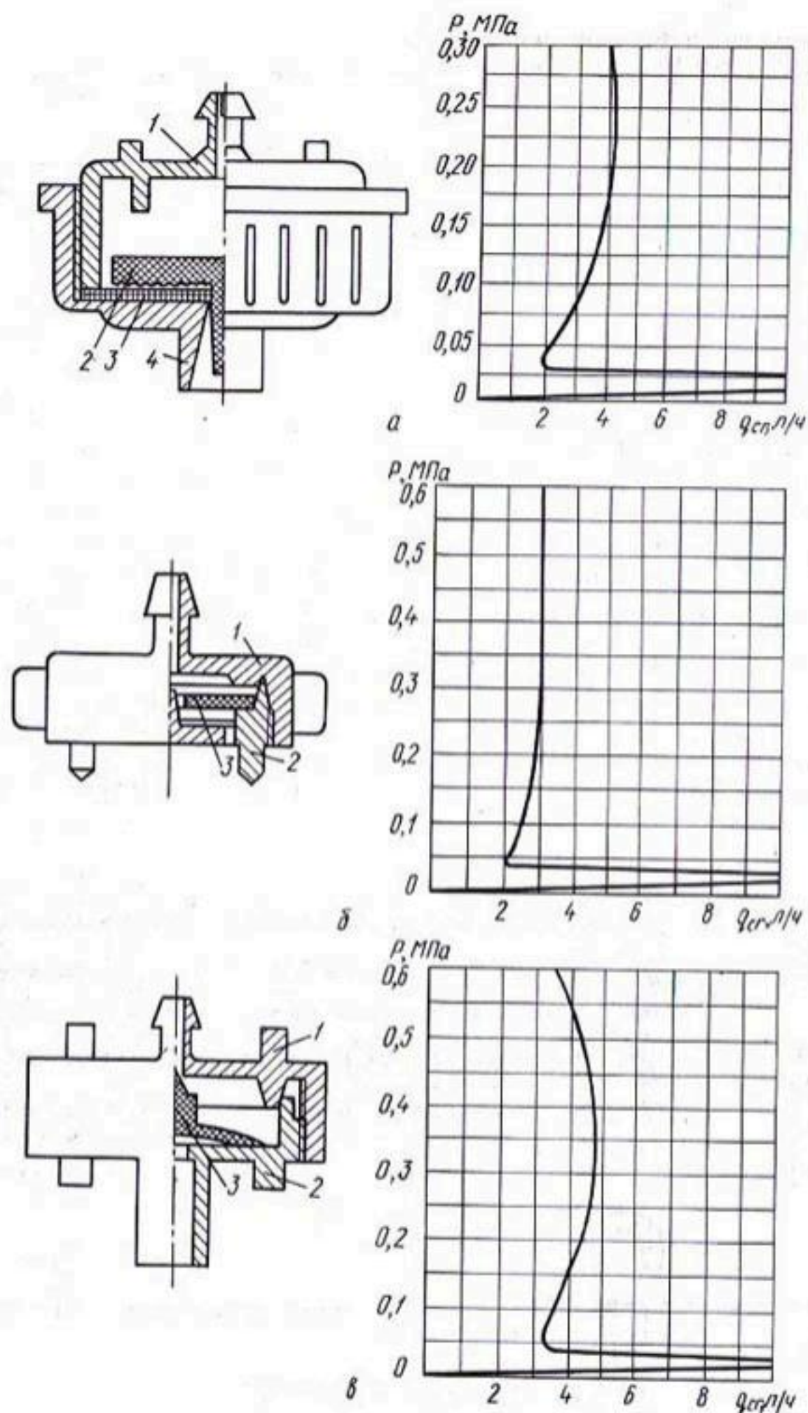
Рис. 4.2. Конструктивные схемы и расходно-напорные характеристики капельниц: а — «Молдавия-1А»: 1 — корпус; 2 — дроссель; 3 — шайба-прокладка; 4 — крышка с выходным отверстием; б — «Горная»: 1 — корпус; 2 — крышка; 3 — мембрана; в — КУ-1: 1 — корпус; 2 — крышка; 3 — диафрагма резиновая;
