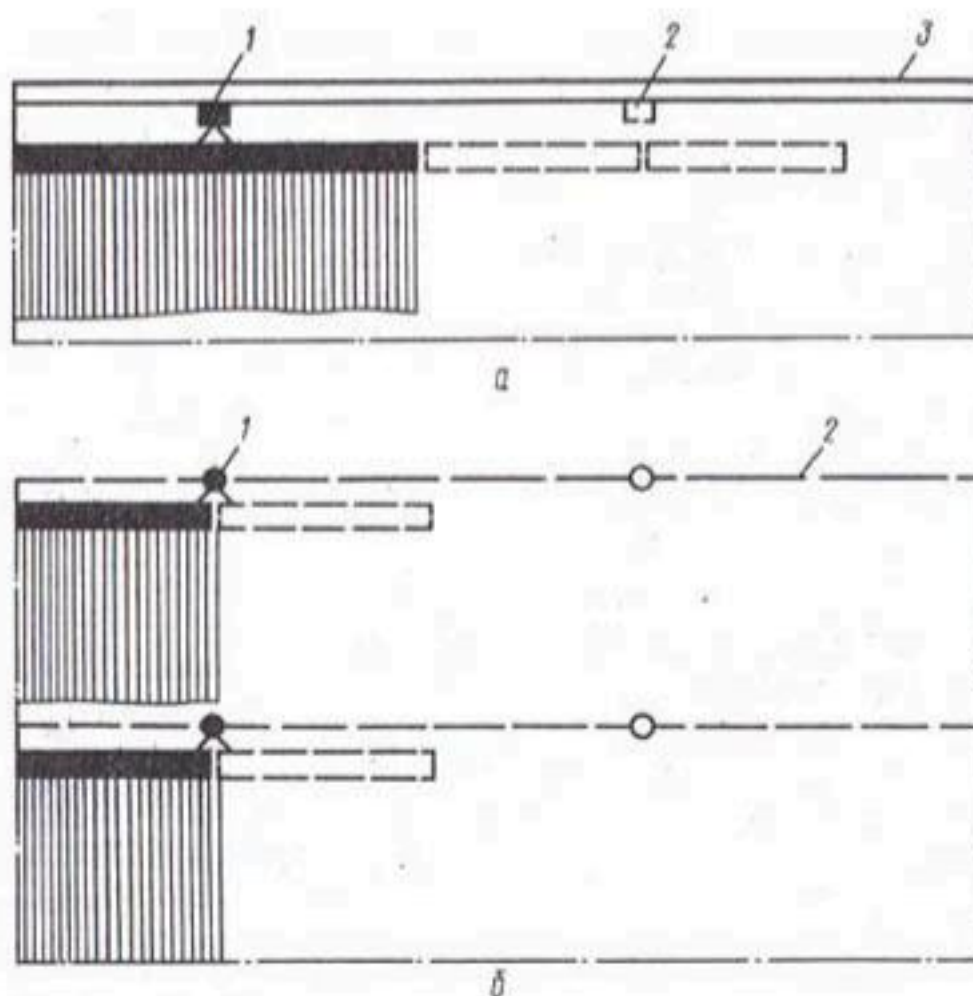
Рис. 2.12. Технологические схемы полива АПШ-1:
