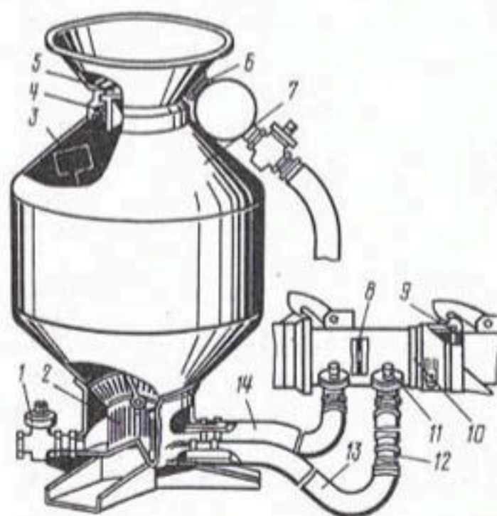
Рис. 3.7. Гидроподкормщик ГПД-50:
