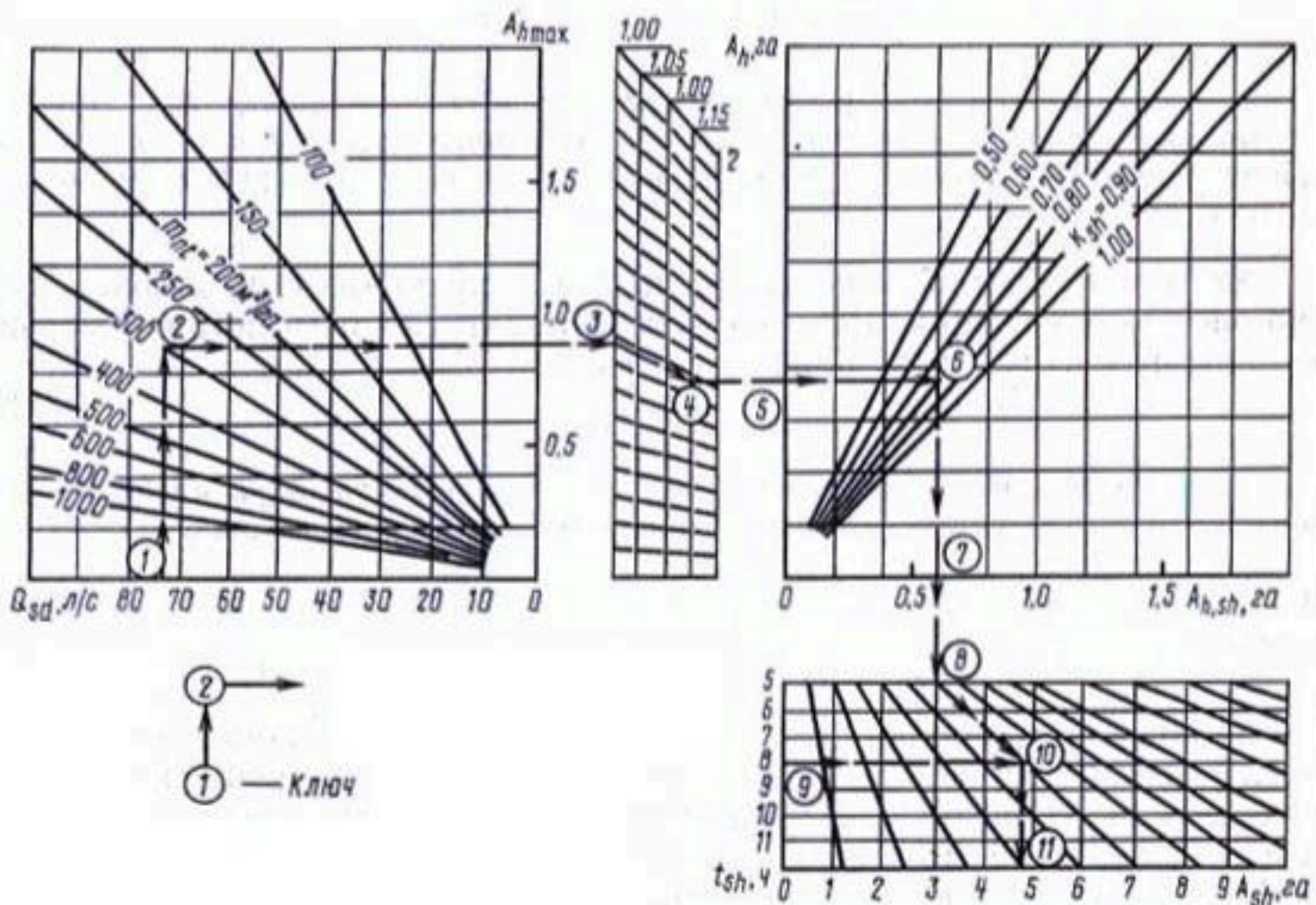
Рис. 3.56. Номограмма для определения сменной выработки дождевальных машин и установок:
