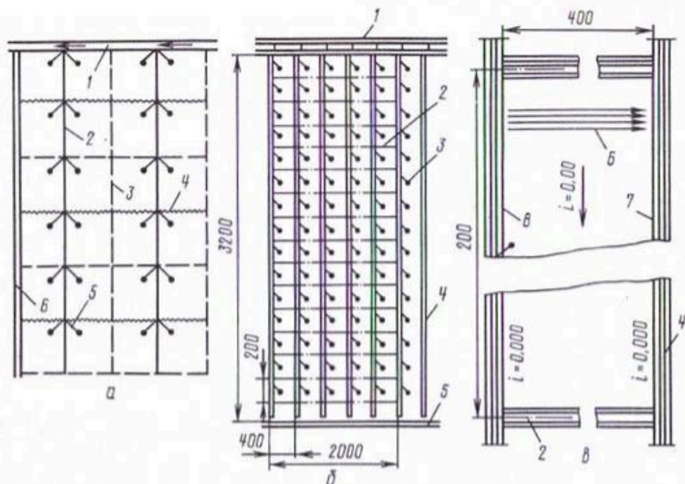
Рис. 2.8. Схема сети для полива по постоянным поливным участкам на очень малых уклонах (0,0005...0,0003):
