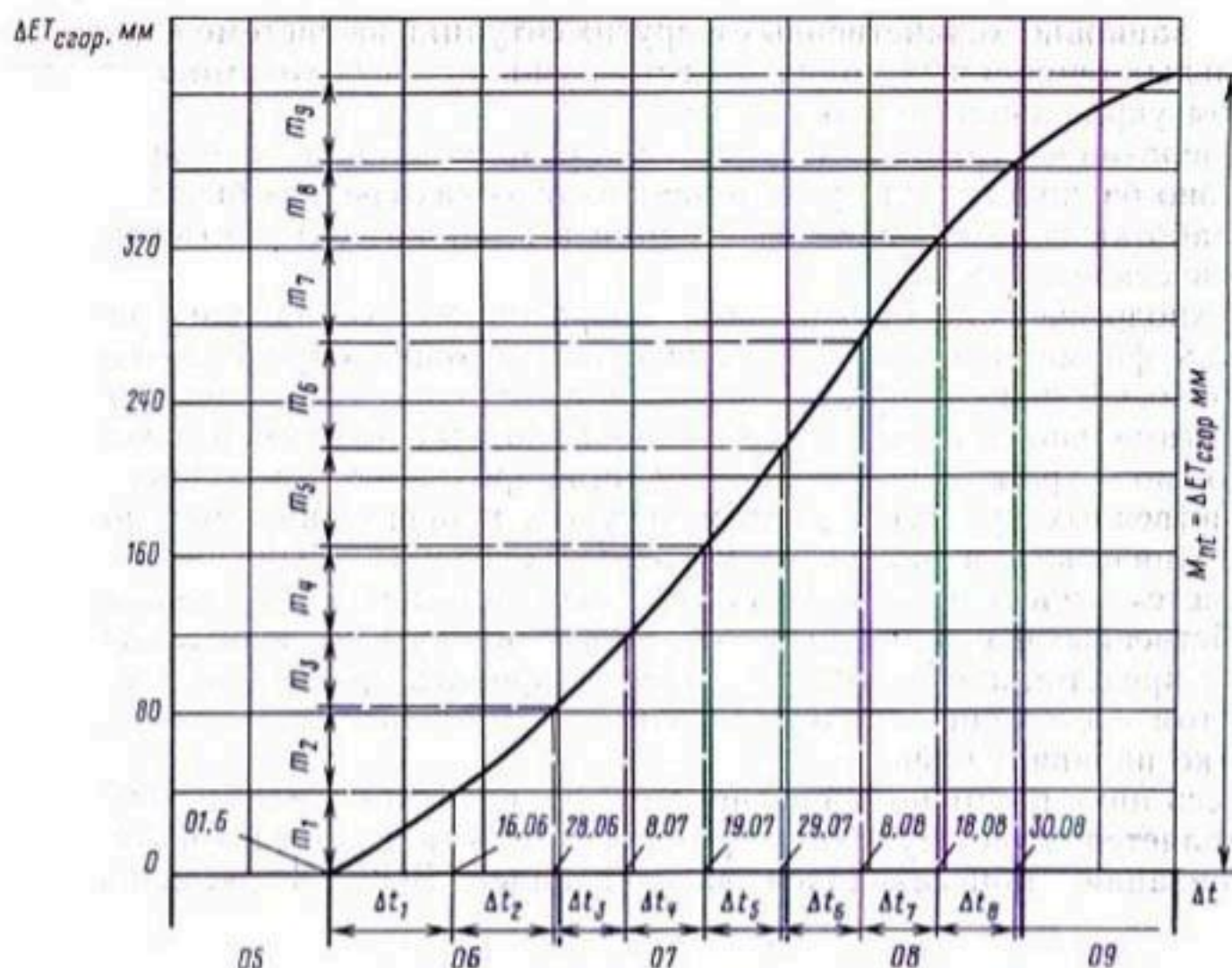
Рис. 1.25. Графоаналитический расчет поливного режима по интегральной кривой дефицита водопотребления: m — поливная норма; \Delta ET_{сгор} — дефицит водопотребления; M_{ит} — оросительная норма, нетто; \Delta t — межполивной период, 16.06... 30.08 — средние даты поливов
