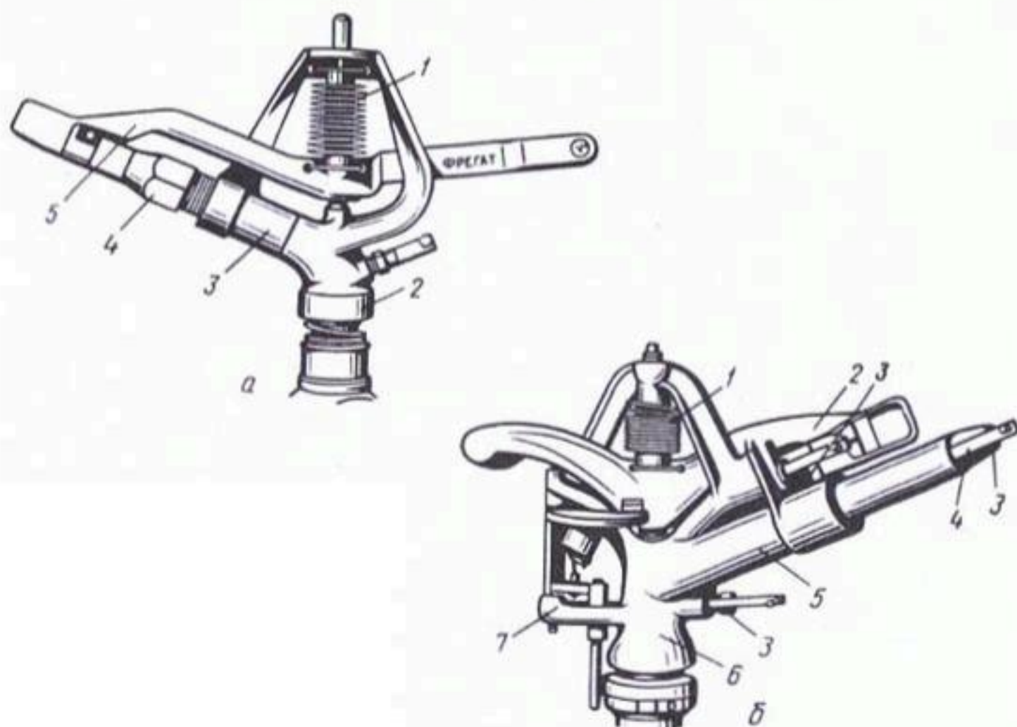
Рис. 3.4. Дождевальные аппараты «Фрегат» и их напорно-расходные характеристики:
