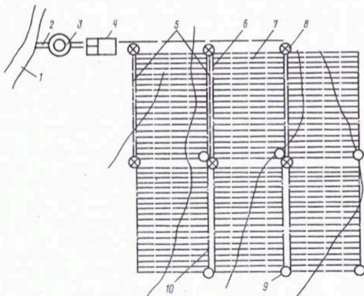
Рис. 4.11. Схема системы ВПО:
