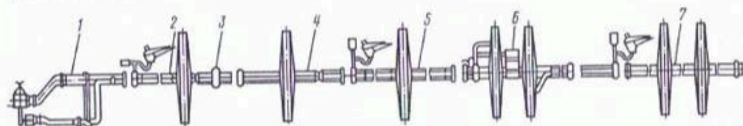
Рис. 3.9. Схема компоновки дождевального крыла машины ДКГ-80 «Ока»: 1 — узел присоединения к гидранту телескопический; 2 — секция с дождевальным аппаратом (нормально открытый); 3 — программное устройство; 4 — секция без аппарата; 5 — секция с дождевальным аппаратом (нормально закрытый); 6 — тележка с гидроприводом; 7 — концевая секция
