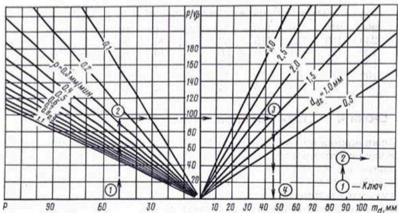
Рис. 1.24. Номограмма для определения достокровой поливной нормы:
