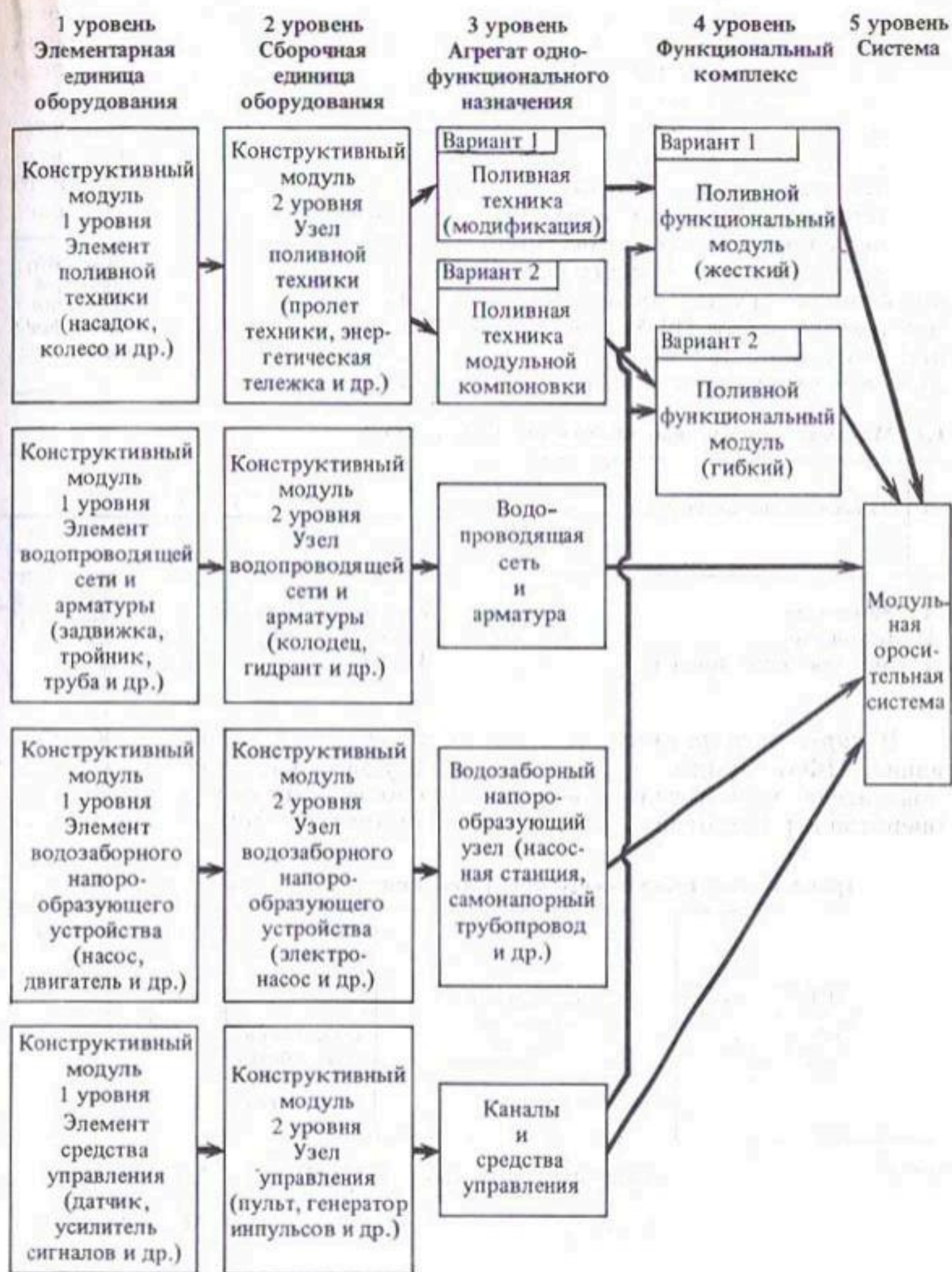
Рис. 1.7. Иерархия модулей оросительной системы
