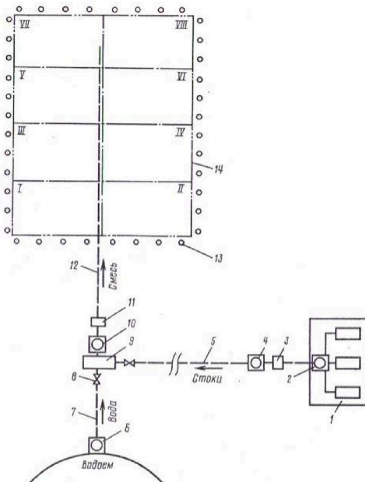
Рис. 4.12. Схема системы ВПО при подаче стоков (воды) в оросительную сеть: 1 — прифермское или полевое хранилище стоков; 2, 4 — насосные станции сточных вод; 3 — приемный резервуар насосной станции сточных вод; 5 — напорный трубопровод стоков; 6 — насосная станция воды; 7 — напорный трубопровод воды; 8 — задвижка; 9 — смесительная камера; 10 — насосная станция смеси; 11 — узел приготовления минеральных удобрений; 12 — напорный трубопровод смеси; 13 — лесополоса; 14 — поле севооборота; I...VIII — номера полей
