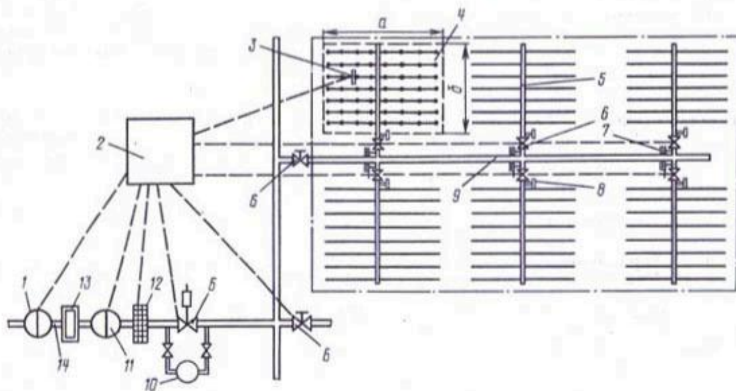
Рис. 4.1. Принципиальная схема системы капельного орошения:
