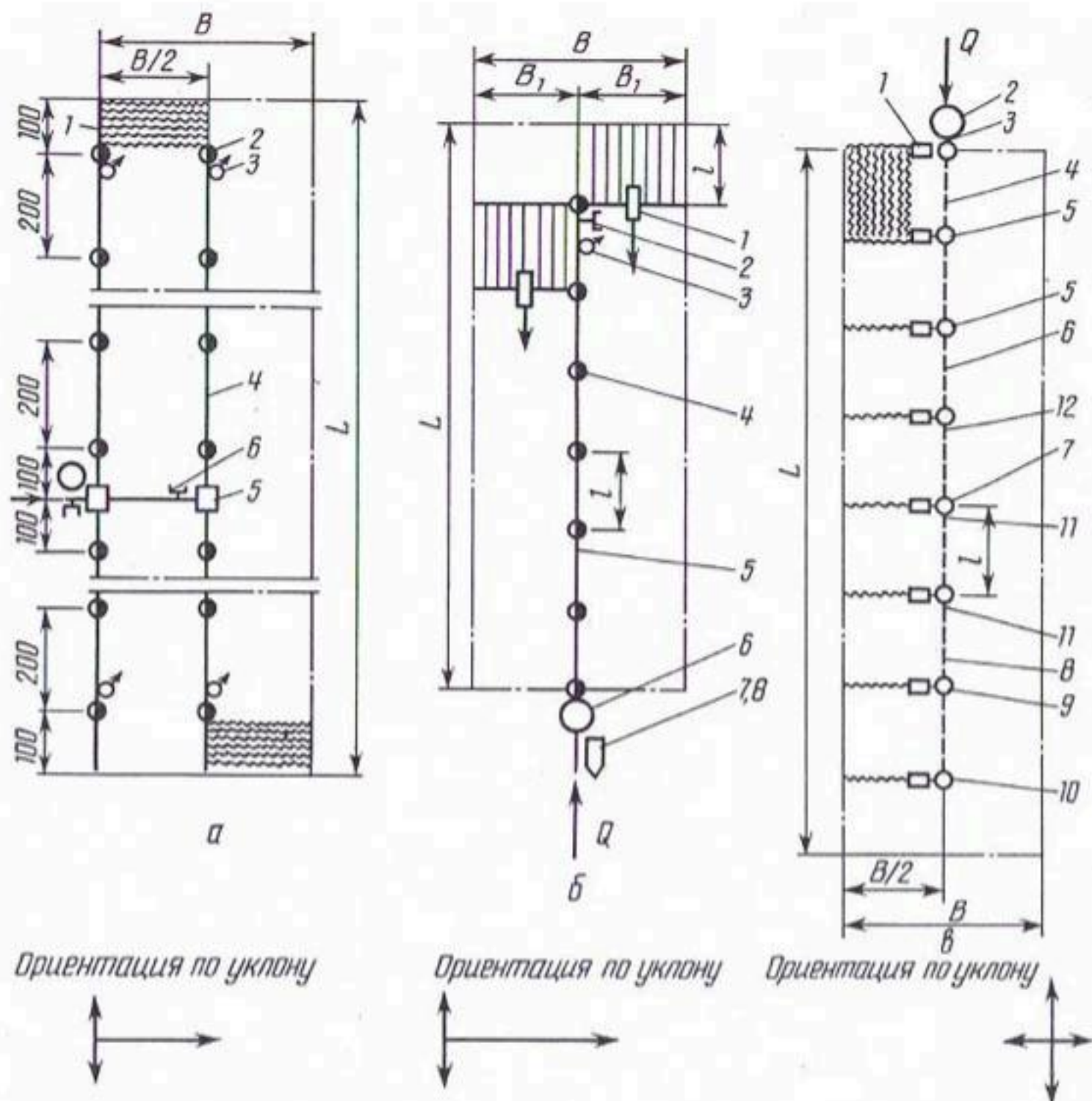
Рис. 2.17. Схема модульного участка с поливом: а — АПШ-1 (обозначения см. табл. 2.13); б — ТКП-90 (обозначения см. табл. 2.14); в — АШУ-32 (обозначения см. табл. 2.15) (размеры в м)
