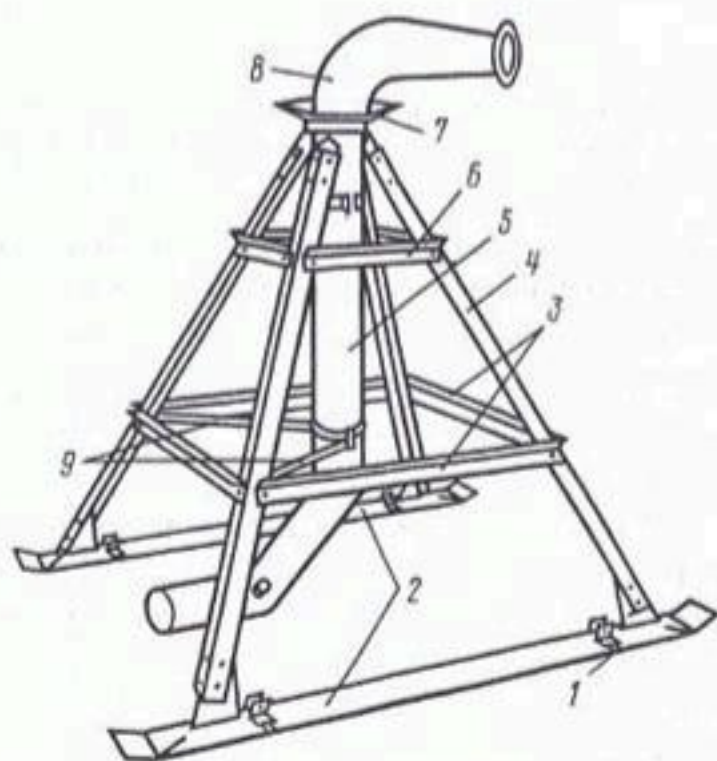
Рис. 3.34. Центральная неподвижная опора машины «Фрегат»:
