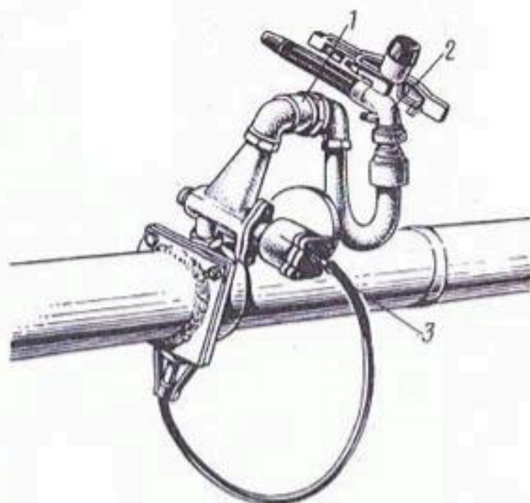
Рис. 3.11. Механизм самоустановки и гидравлический управляющий клапан дождевального аппарата ДКГ-80 «Ока»:
