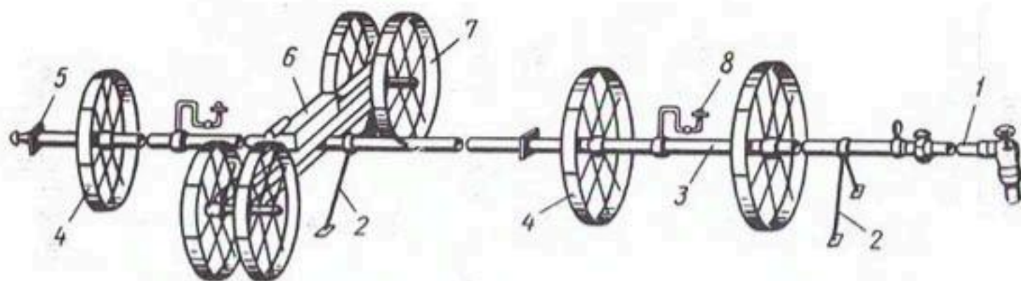
Рис. 3.6. Дождевальная машина «Волжанка»:
