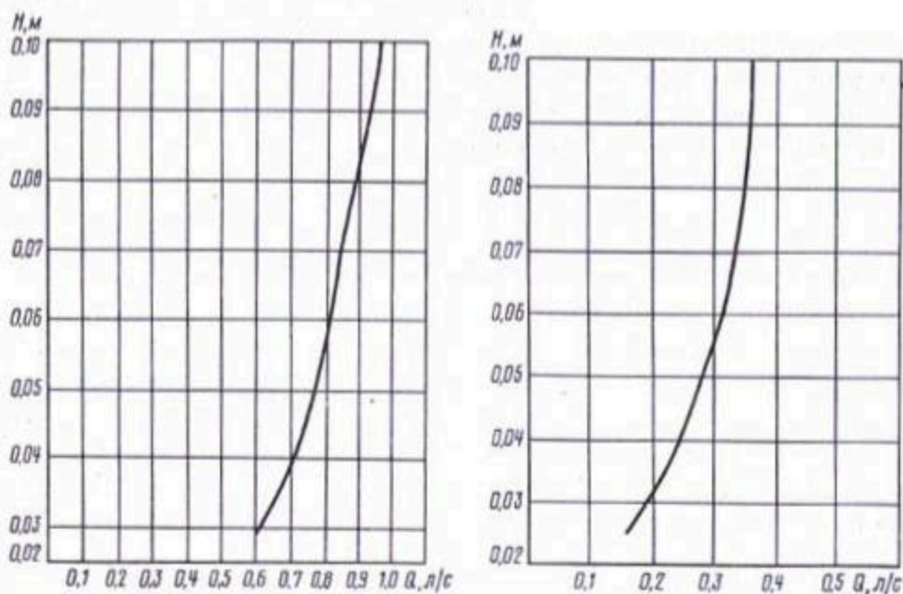
Рис. 2.4. Расходно-напорные характеристики сифонов пластмассового неразряжающегося с внутренним диаметром 35,4 мм и 25 мм
