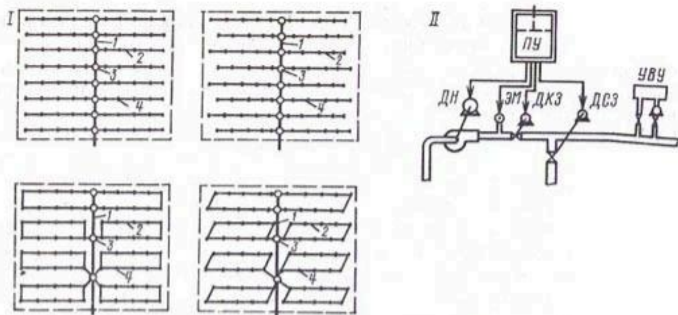
Рис. 3.58. Типовые схемы (I) закрытой оросительной сети и оборудование (II) для гидроимпульсного управления поливом на системе:
