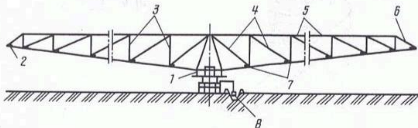
Рис. 3.47. Двухконсольный дождевальная агрегат ДДА-100МА:
