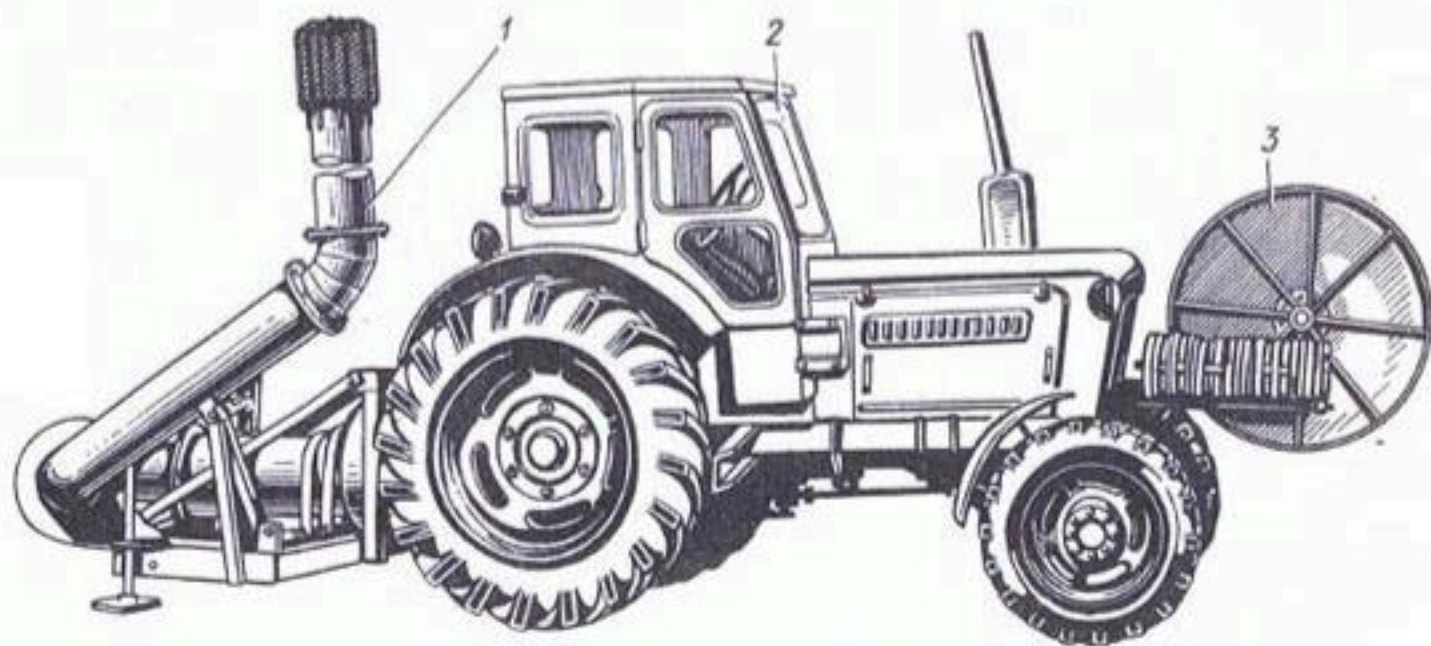
Рис. 2.10. Поливальщик передвижной агрегатный (универсальный) ППА-165У: 1 — всасывающая линия; 2 — трактор; 3 — барабан-контейнер
