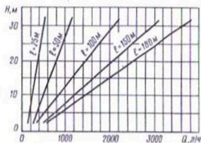
Рис. 4.4. График для определения водопдачи трубопровода «Аква-Дроп» в зависимости от длины и напора в номинальном сечении
