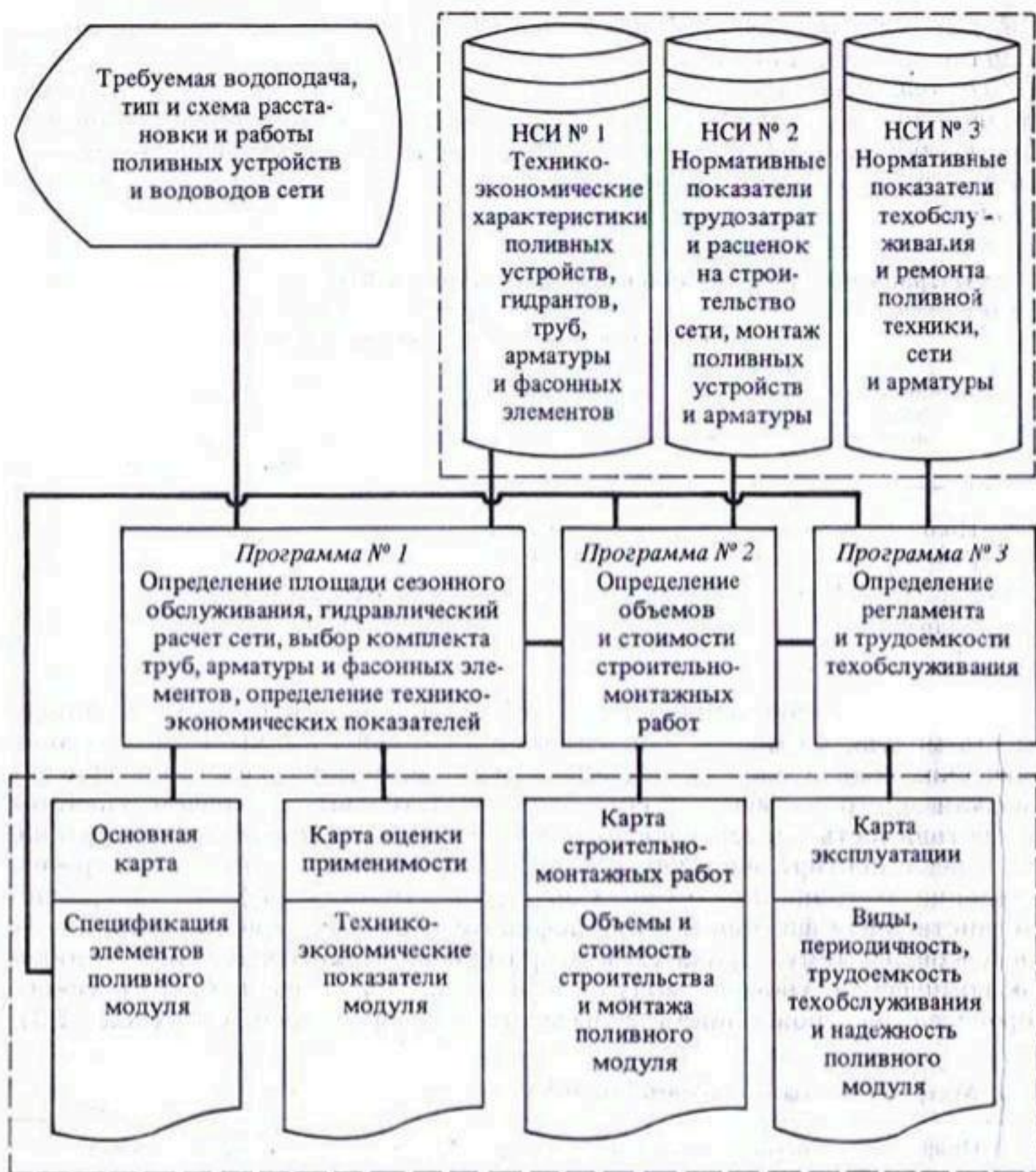
Рис. 1.6. Схема автоматизированного проектирования поливного функционального модуля
