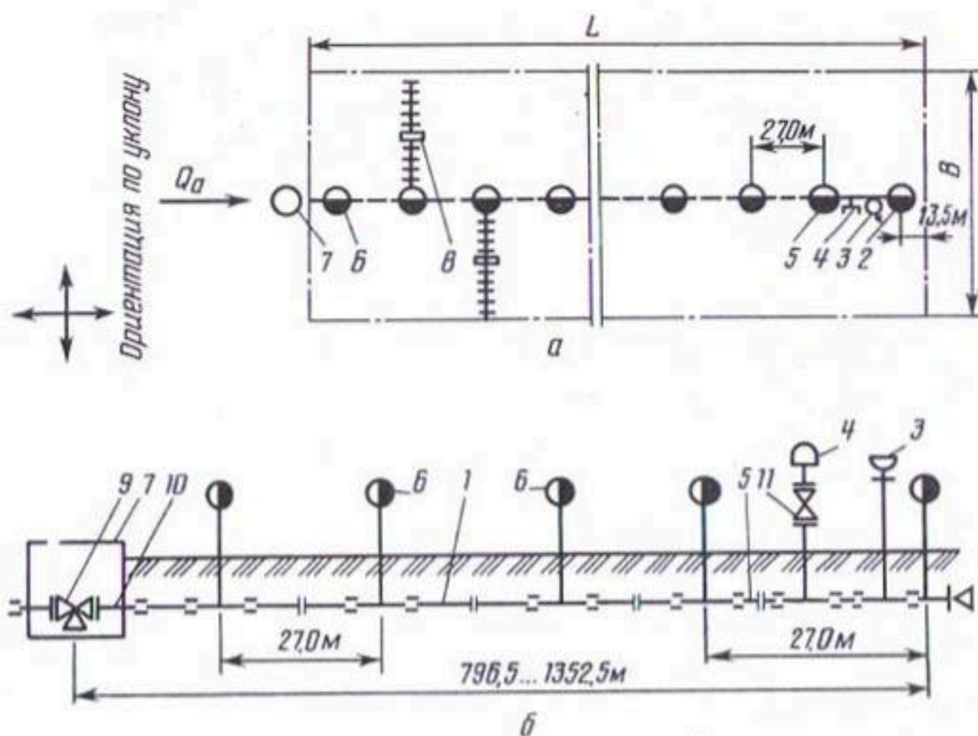
Рис. 3.16. Схема поливного модуля с машиной ДКН-80 (а) и его монтажа (б) (условные обозначения см. табл. 3.25)
