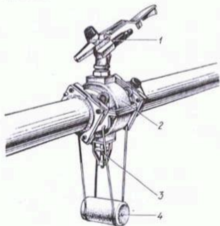
Рис. 3.14. Механизм самоустановки дождевального аппарата ДКН-80.05.00:
