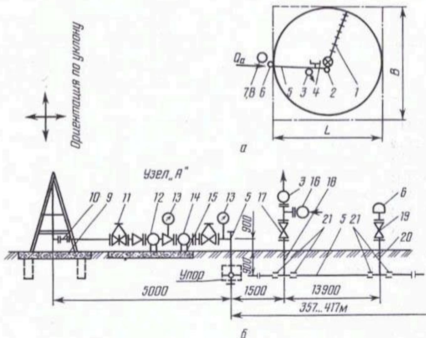
Рис. 3.38. Схема модульного участка с машиной ДМУ «Фрегат», сетью из асбестоцементных труб и подводом воды к торцу модульного участка (а) и его монтажа (б) (условные обозначения см. табл. 3.53)
