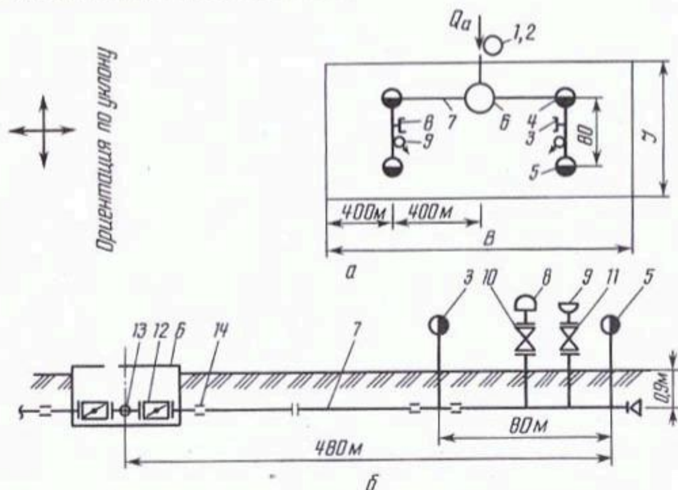
Рис. 3.30. Схема поливного модуля с машиной ДШ-30 (а) и его монтажа (б) (условные обозначения см. табл. 3.44)
