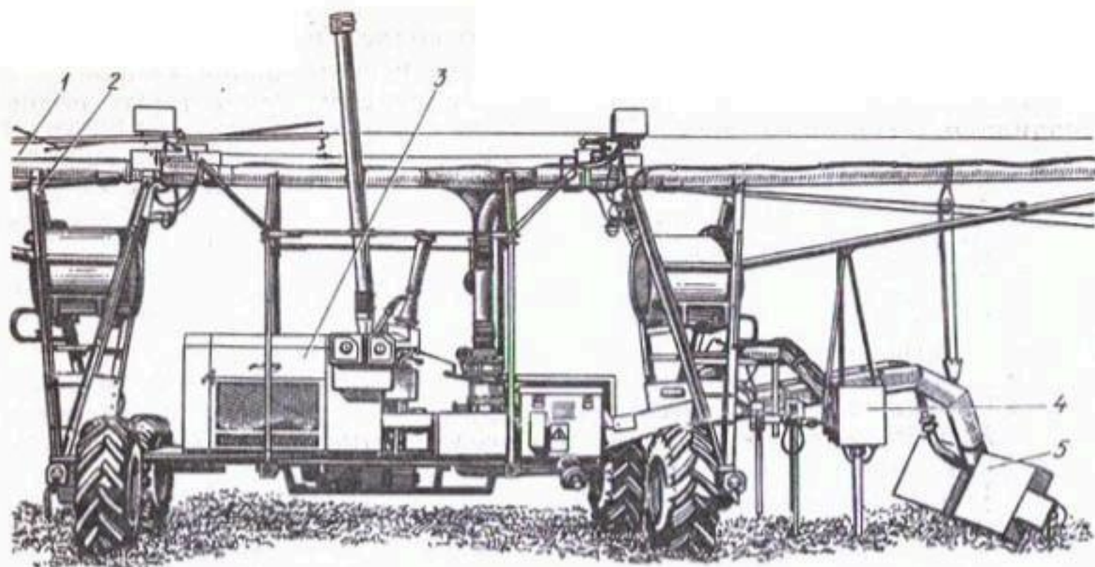
Рис. 3.43. Центральная часть дождевальной машины «Кубань-Л»:
