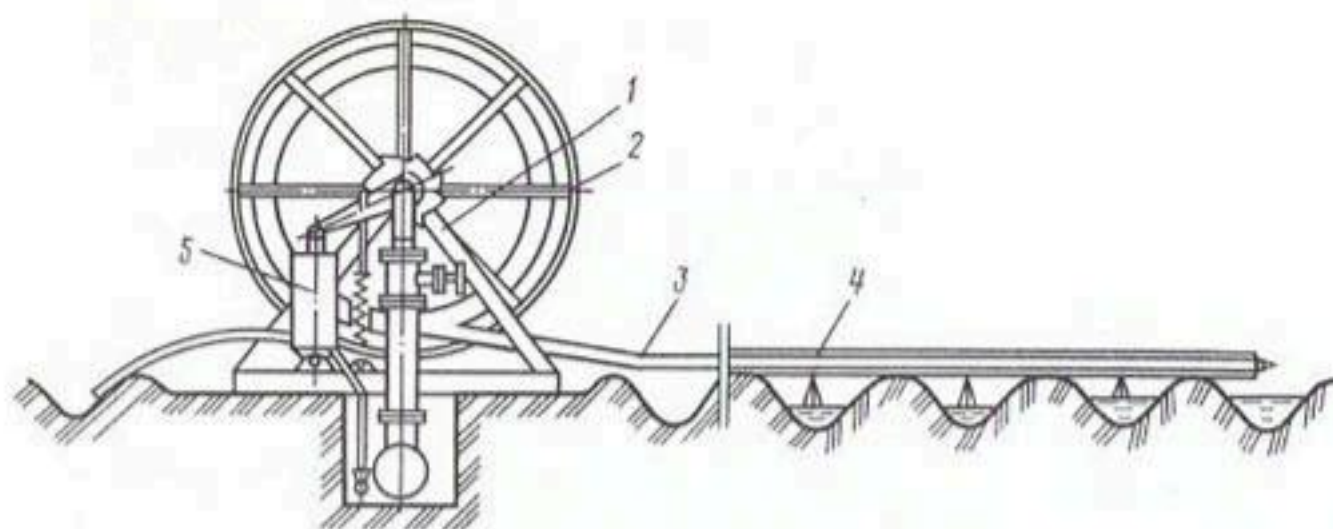
Рис. 2.15. Схема шлангового поливного устройства АШУ-32: 1 — рама; 2 — барабан; 3 — шланг поливной; 4 — водовыпускные отверстия; 5 — гидроцилиндр
