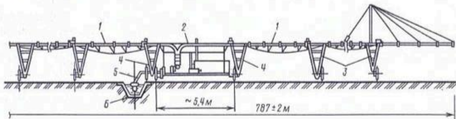
Рис. 3.42. Дождевальная машина «Кубань-Л»:
