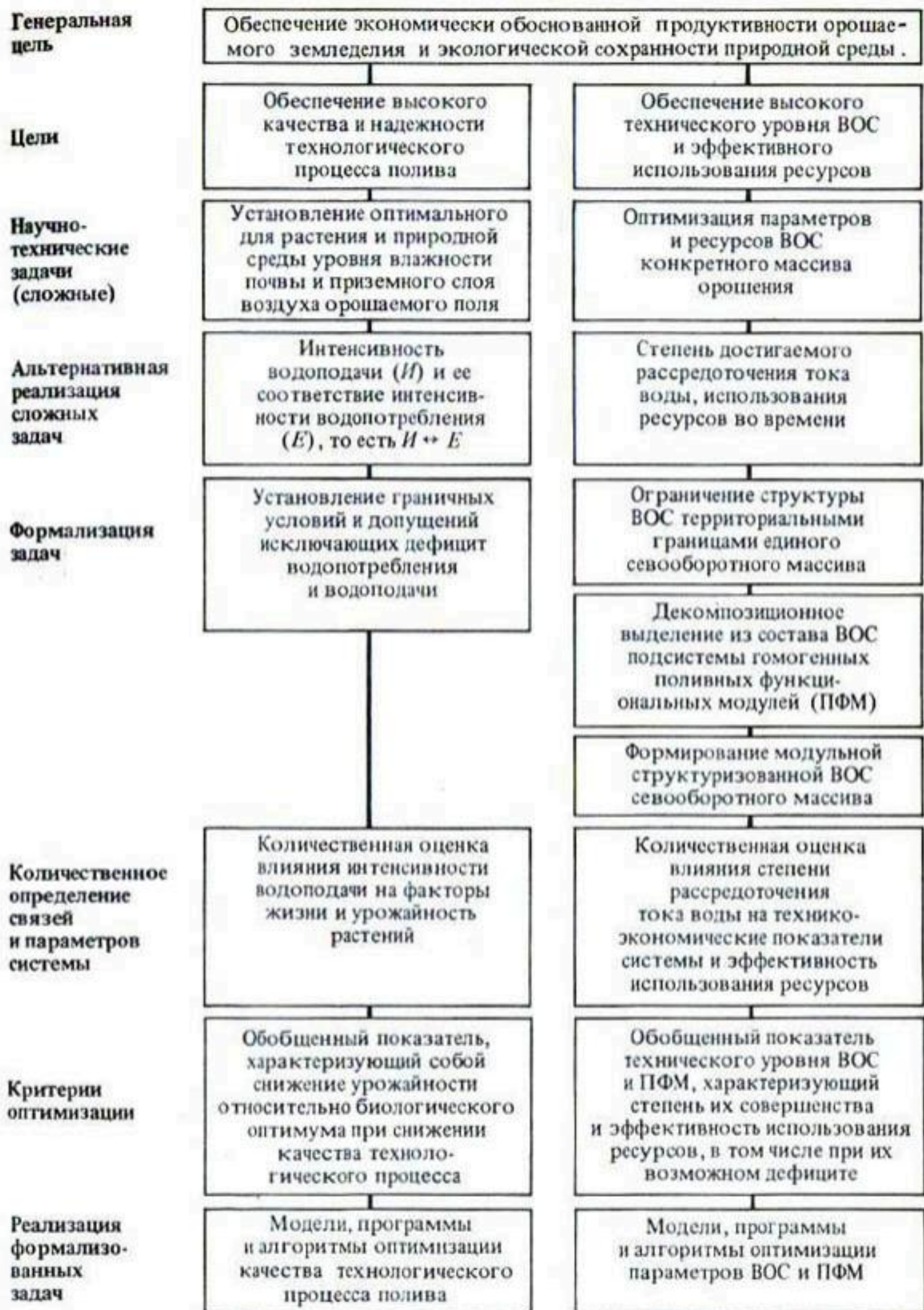
Рис. 1.4. Задачи оптимизации поливной техники в составе внутрихозяйственной оросительной системы
