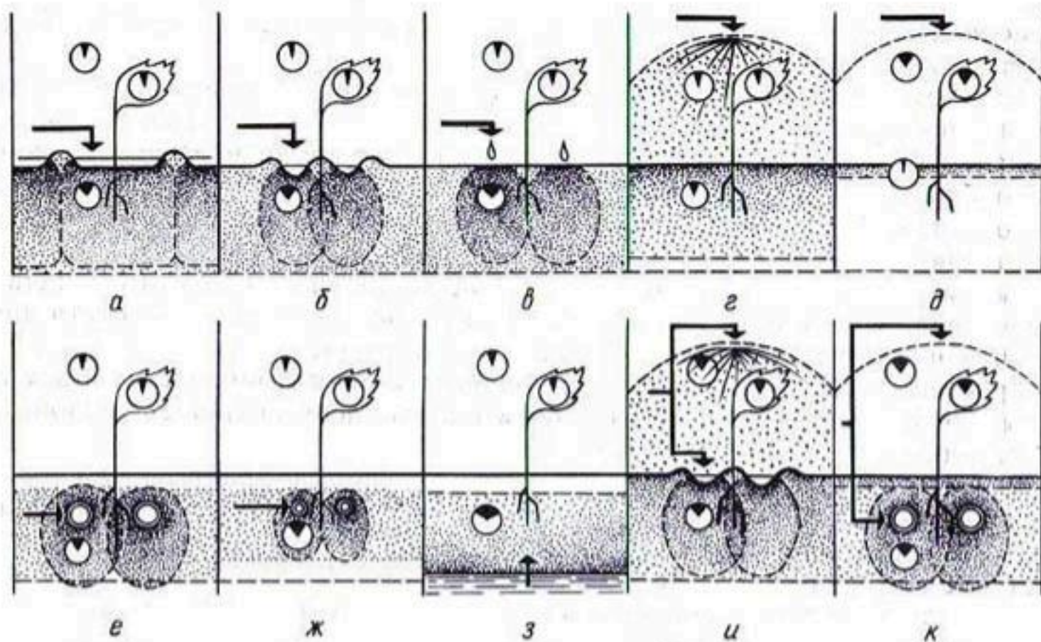
Рис. 1.2. Способы полива (классификационная схема):
