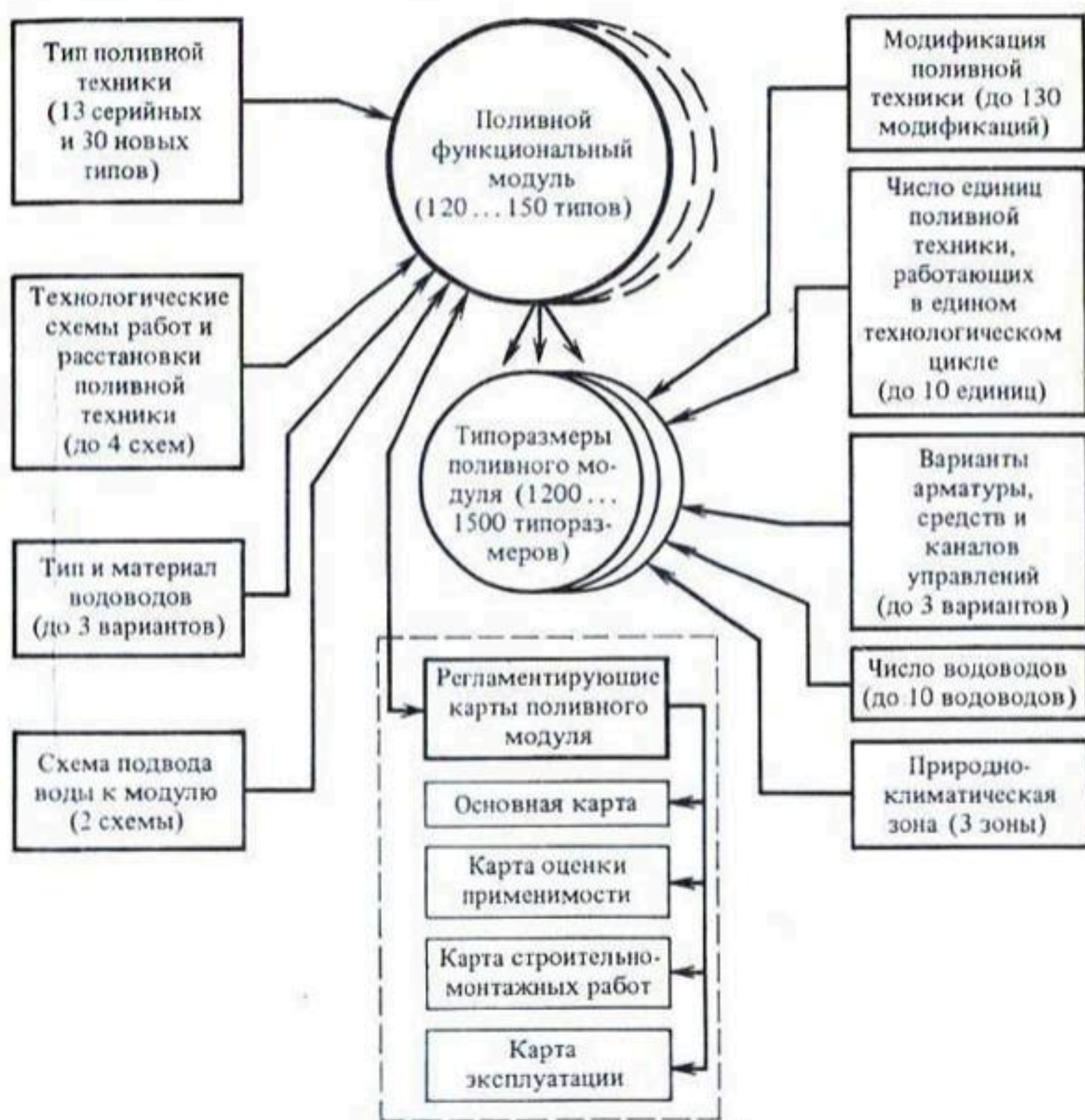
Рис. 1.5. Принципиальная схема оптимизации поливной техники на основе модульного принципа
