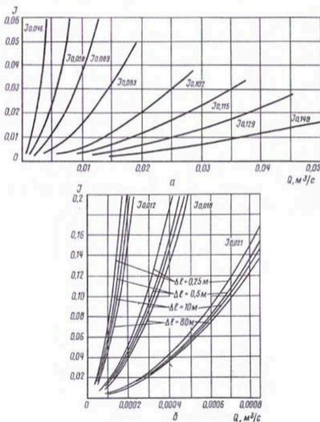
Рис. 4.5. Графики для определения удельных потерь давления в трубопроводах:
