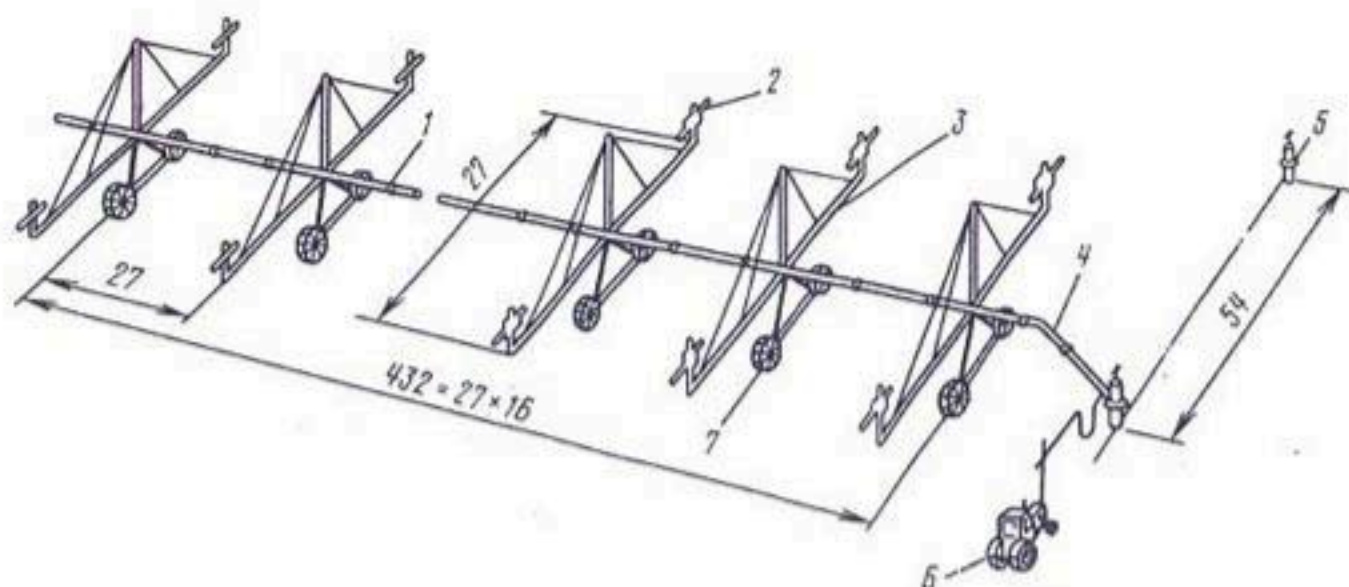
Рис. 3.19. Общий вид дождевальной машины «Днепр» ДФ-120: 1 — водопроводящий пояс; 2 — дождевальный аппарат «Роса-3»; 3 — открывок; 4 — соединительное устройство; 5 — гидрант; 6 — навесная тракторная электростанция; 7 — самоходная тележка (размеры в м)
