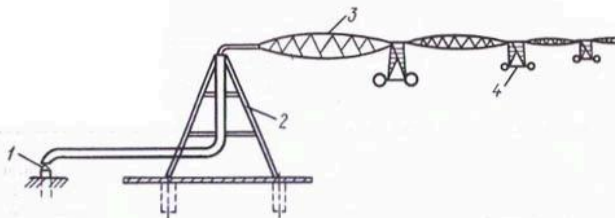
Рис. 3.39. Машина «Кубань-ЛК-1»:
