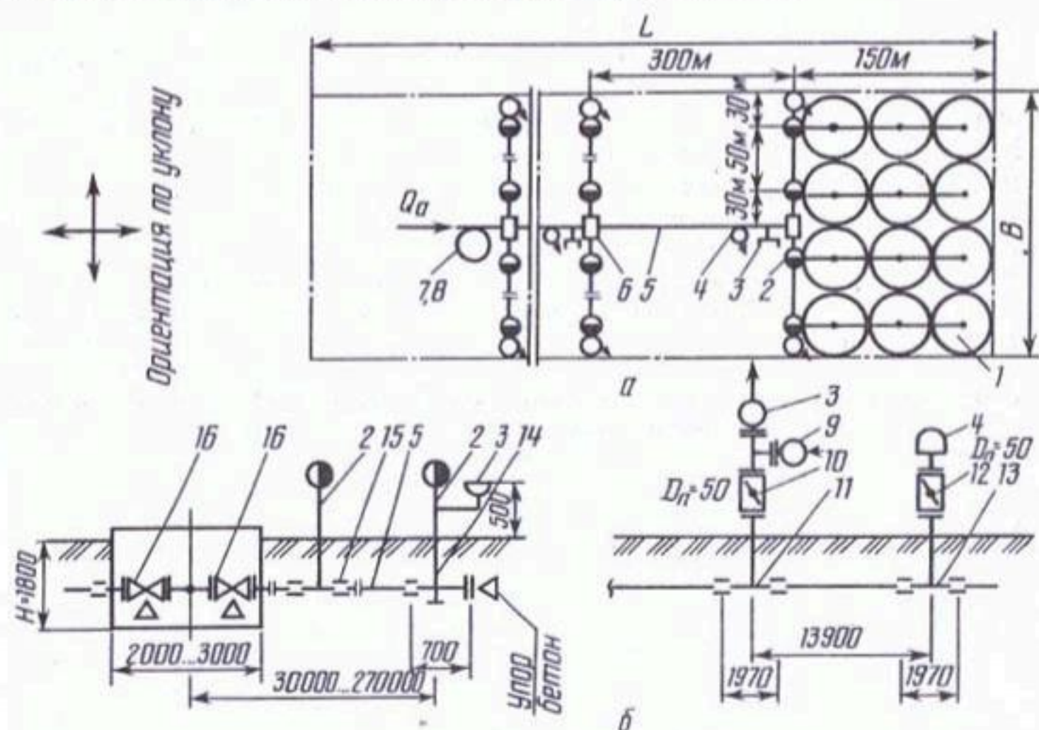
Рис. 3.18. Схема поливного модуля с машиной ДШ-25/300 (а) и его монтажа (б) (подвод воды к торцу участка, условные обозначения см. табл. 3.29)
