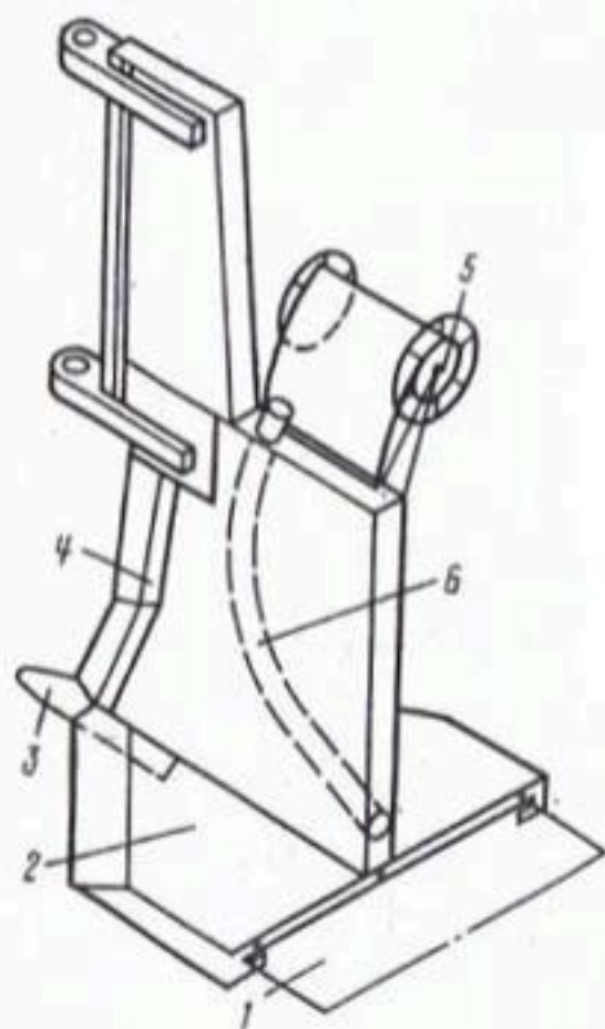
Рис. 4.14. Рабочий орган трубоукладчика НБУ-ПТЭ:
