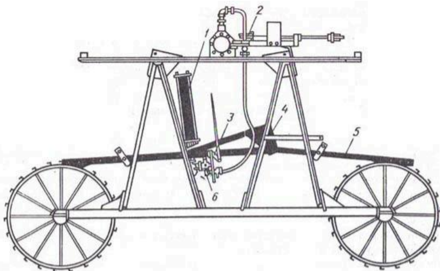
Рис. 3.35. Тележка самоходной опоры машины «Фрегат»:
