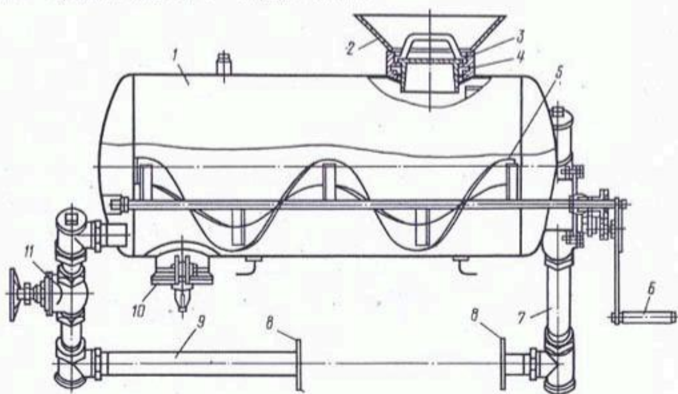
Рис. 3.25. Гидроподкормщик навесных дождевальных машин ДДН-70 и ДДН-100:
