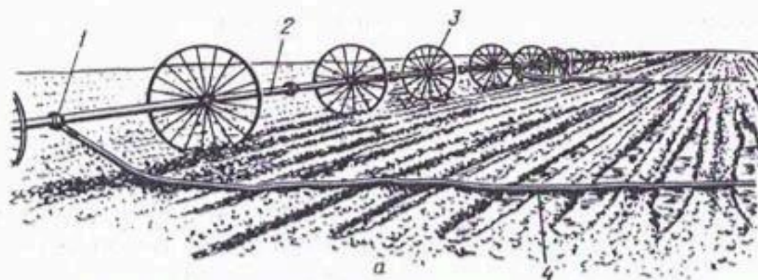
Рис. 2.13. Поливной трубопровод ТКП-90: a — общий вид; 1 — муфта; 2 — водопроводящий пояс; 3 — опорное колесо; 4 — гибкий поливной шлейф; b — муфта со шлейфом для полива по бороздам; 1 — муфта; 2 — диафрагма; 3 — гибкий шланг; 4 — водовыпускные отверстия (20 шт.); 5 — заглушка-зажим для промывки шлейфа
