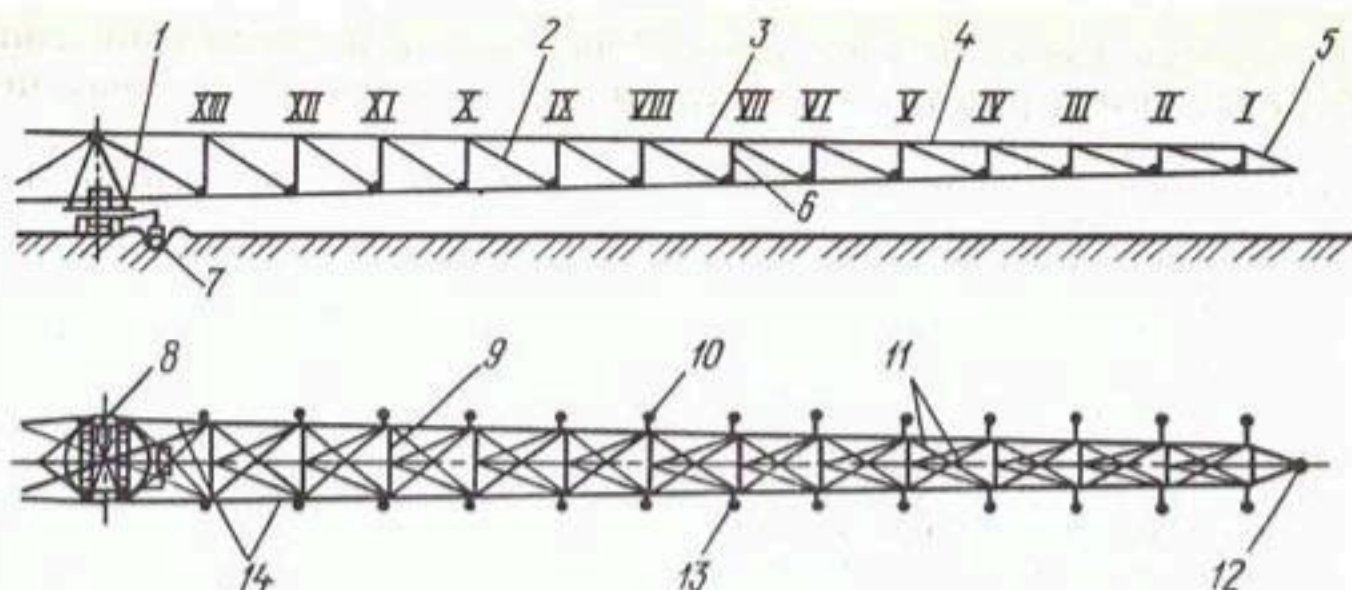
Рис. 3.48. Схема консоли дождевального агрегата ДДА-100МА:
