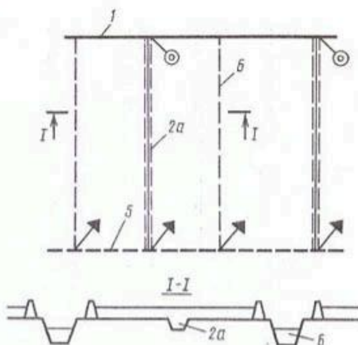
Рис. 2.23. Схема карты-чека с оросителем-сбросом двустороннего действия (условные обозначения см. рис. 2.22)
