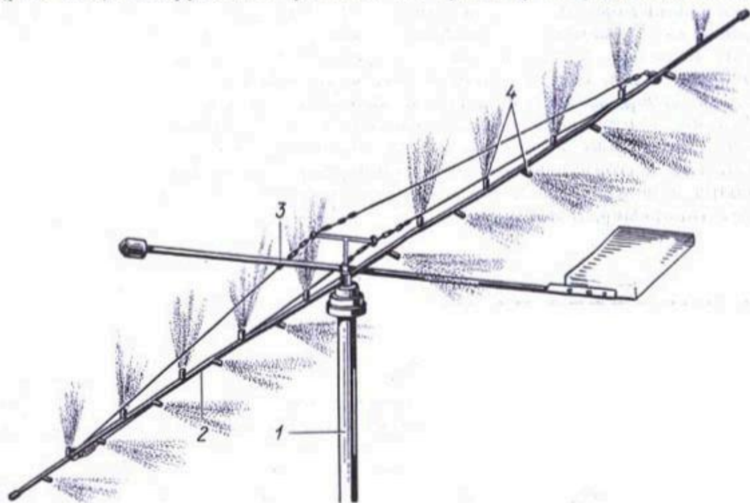
Рис. 3.62. Штанга системы аэрозольного орошения: 1 — мачта; 2 — штанга поворотная; 3 — флюгер; 4 — диспергаторы
