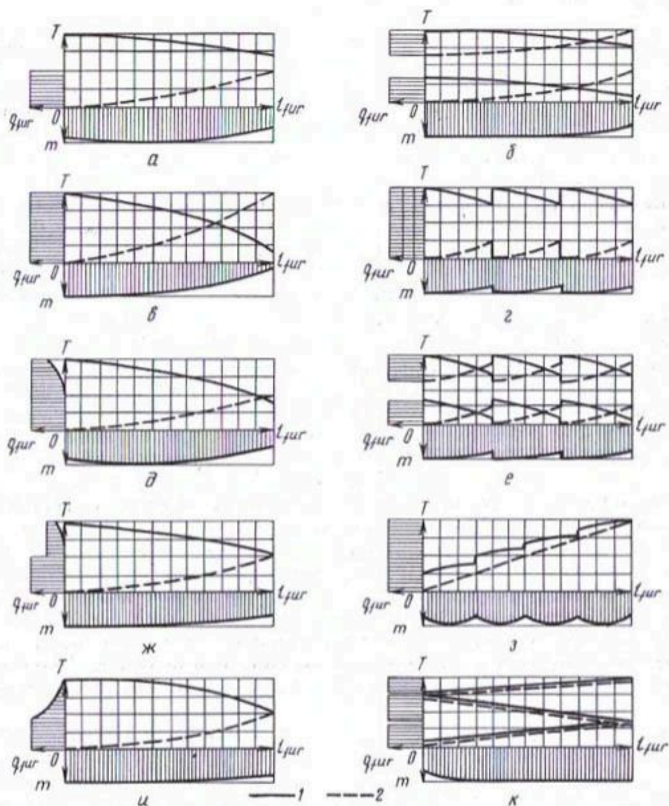
Рис. 2.1. Циклограммы технологий водораспределения по тупым и проточным бороздам:
