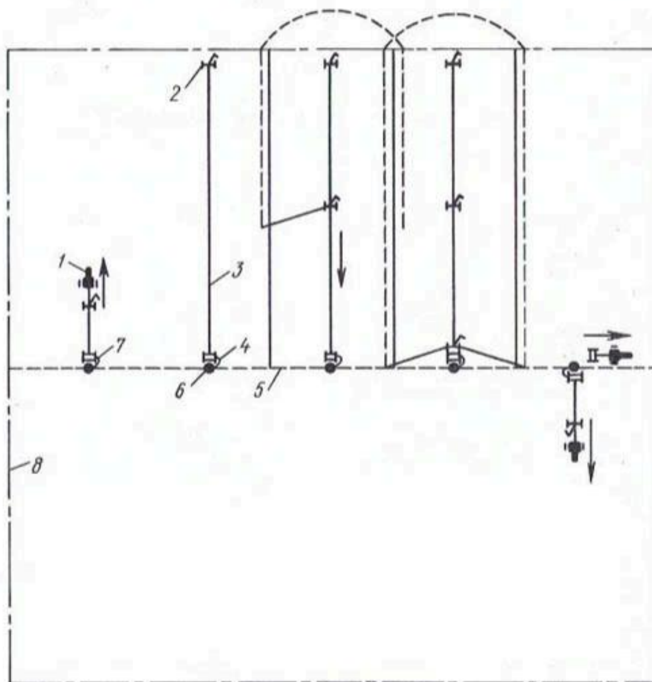
Рис. 3.32. Технологическая схема полива дождевальным оборудованием PZT-75: 1 — трактор; 2 — дождевальный аппарат; 3 — полиэтиленовый шланг; 4 — соединительный рукав; 5 — оросительная сеть; 6 — гидрант на оросительной сети; 7 — шасси с намоточным устройством; 8 — граница орошаемого участка
