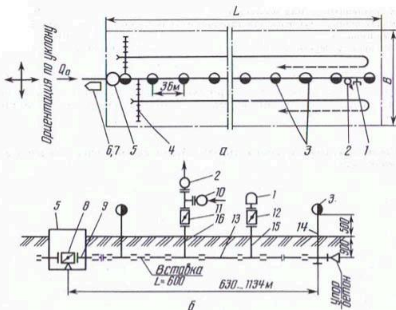
Рис. 3.12. Схема поливного модуля с машиной ДКГ-80 «Ока» (а) и его монтажа (б) (условные обозначения см. табл. 3.21)
