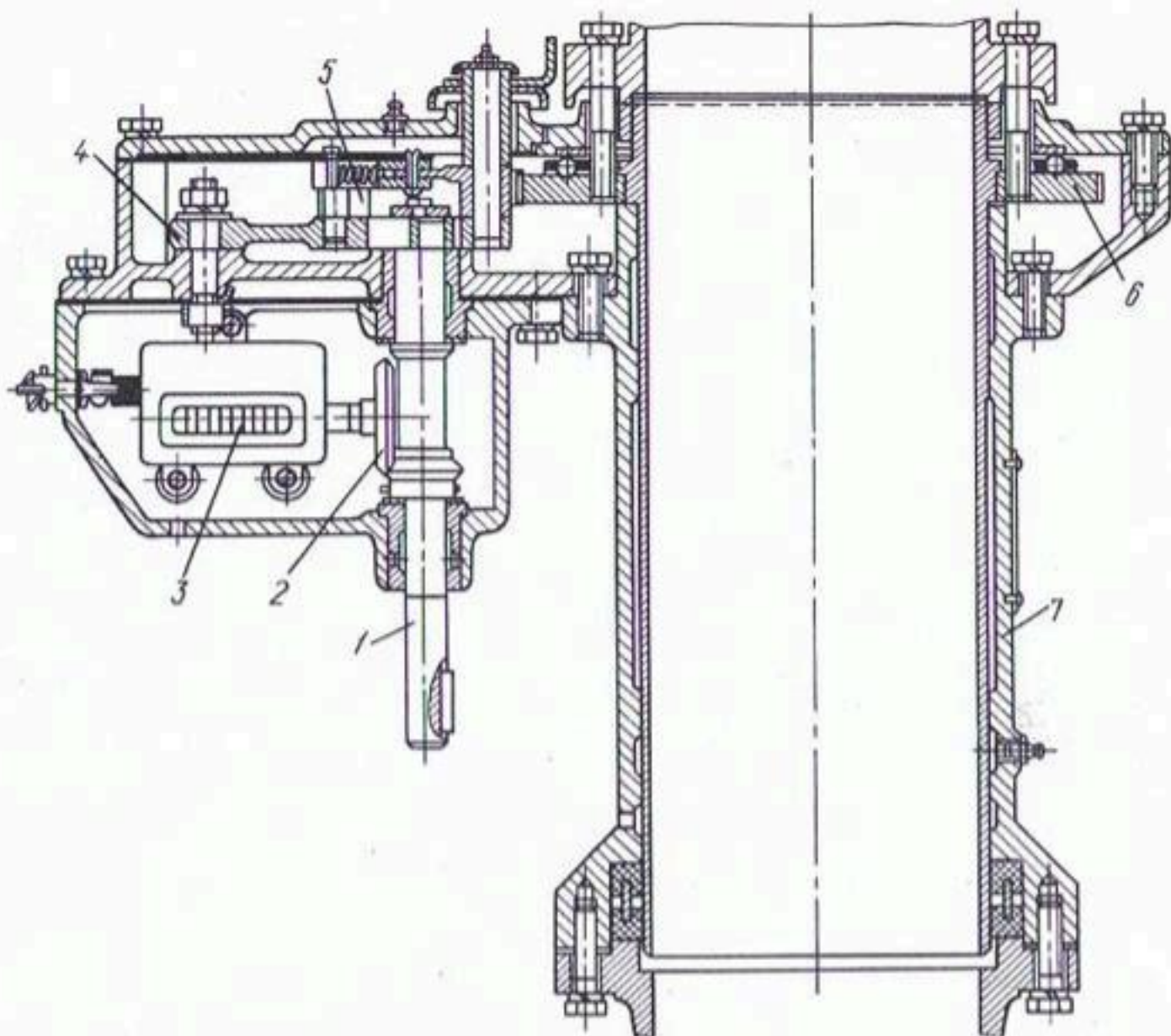
Рис. 3.24. Механизм поворота ствола машины ДДН-70:
