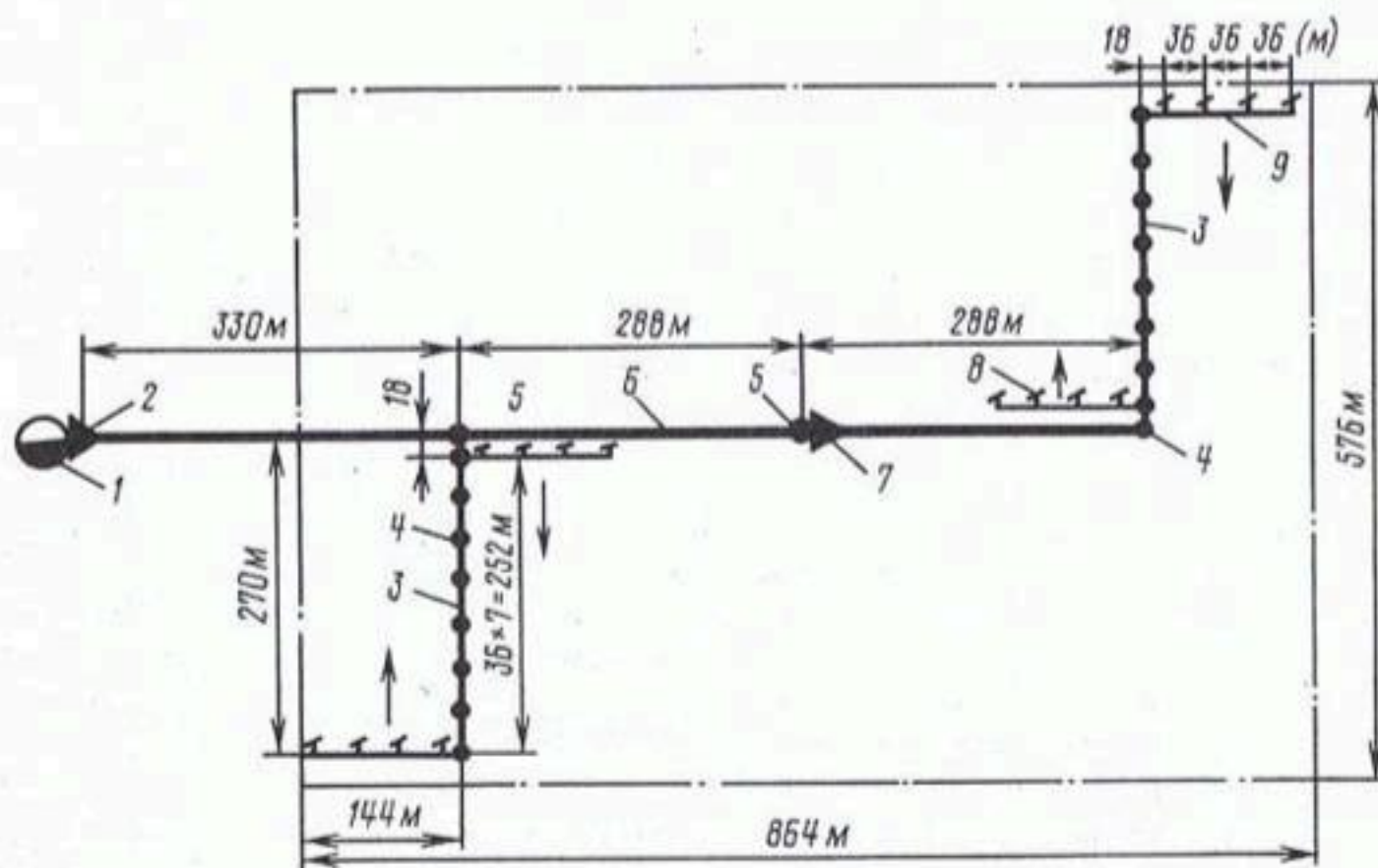
Рис. 3.29. Технологическая схема передвижного комплекта КИ-50:
