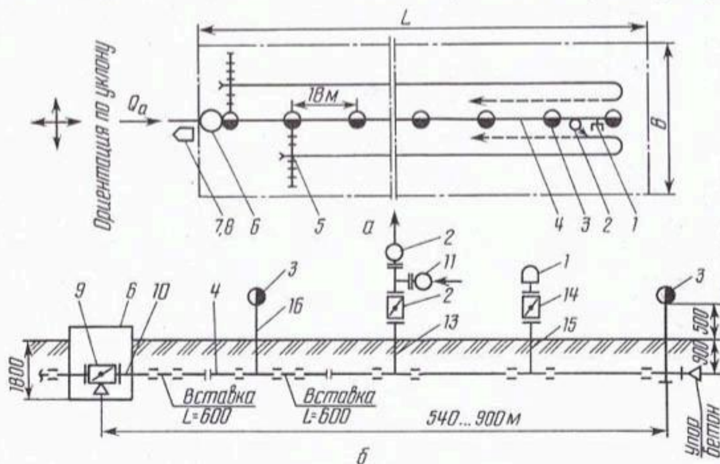
Рис. 3.8. Схема поливного модуля с машиной ДКШ-64 «Волжанка» (а) и его монтажа (б) (условные обозначения см. табл. 3.17)
