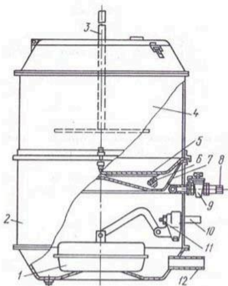
Рис. 3.50. Подкормщик к агрегату ДДА-100МА для внесения минеральных удобрений:
