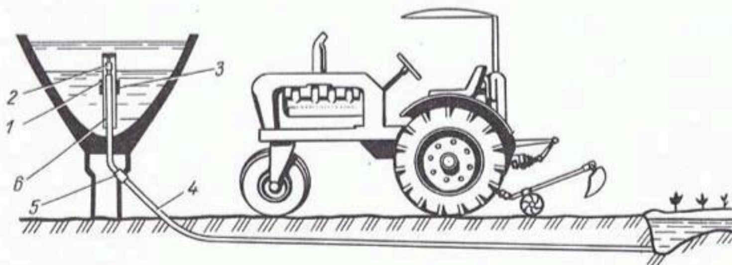
Рис. 2.20. Схема подачи воды из лотка в оголовки поливных борозд:
