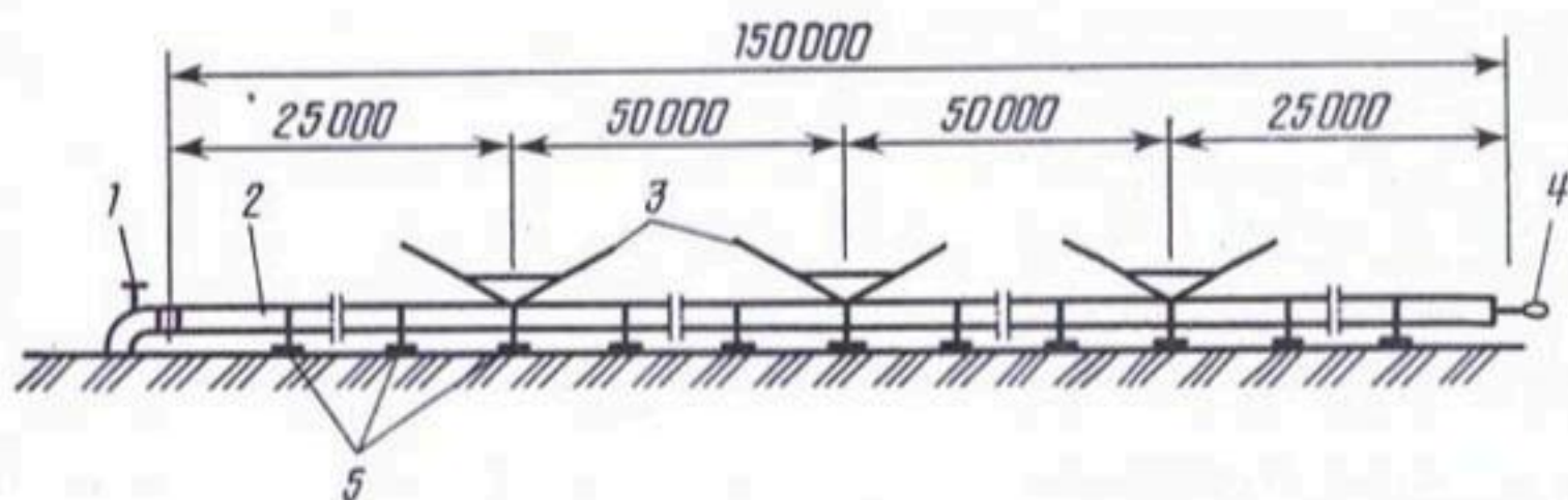
Рис. 3.17. Общий вид дождевального шлейфа ДШ-25/300:
