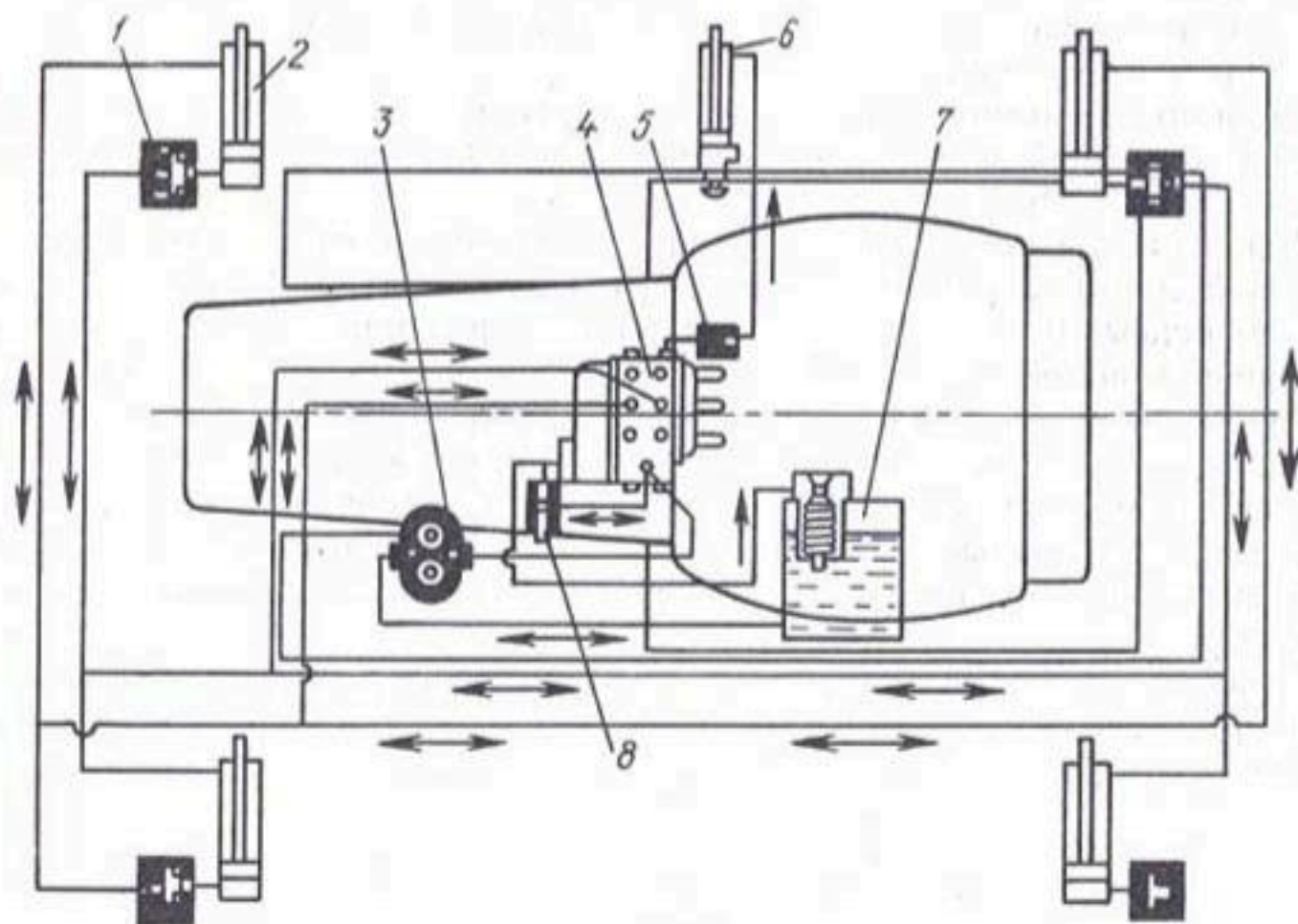
Рис. 3.51. Гидравлическая схема дождевального агрегата ДДА-100МА:
