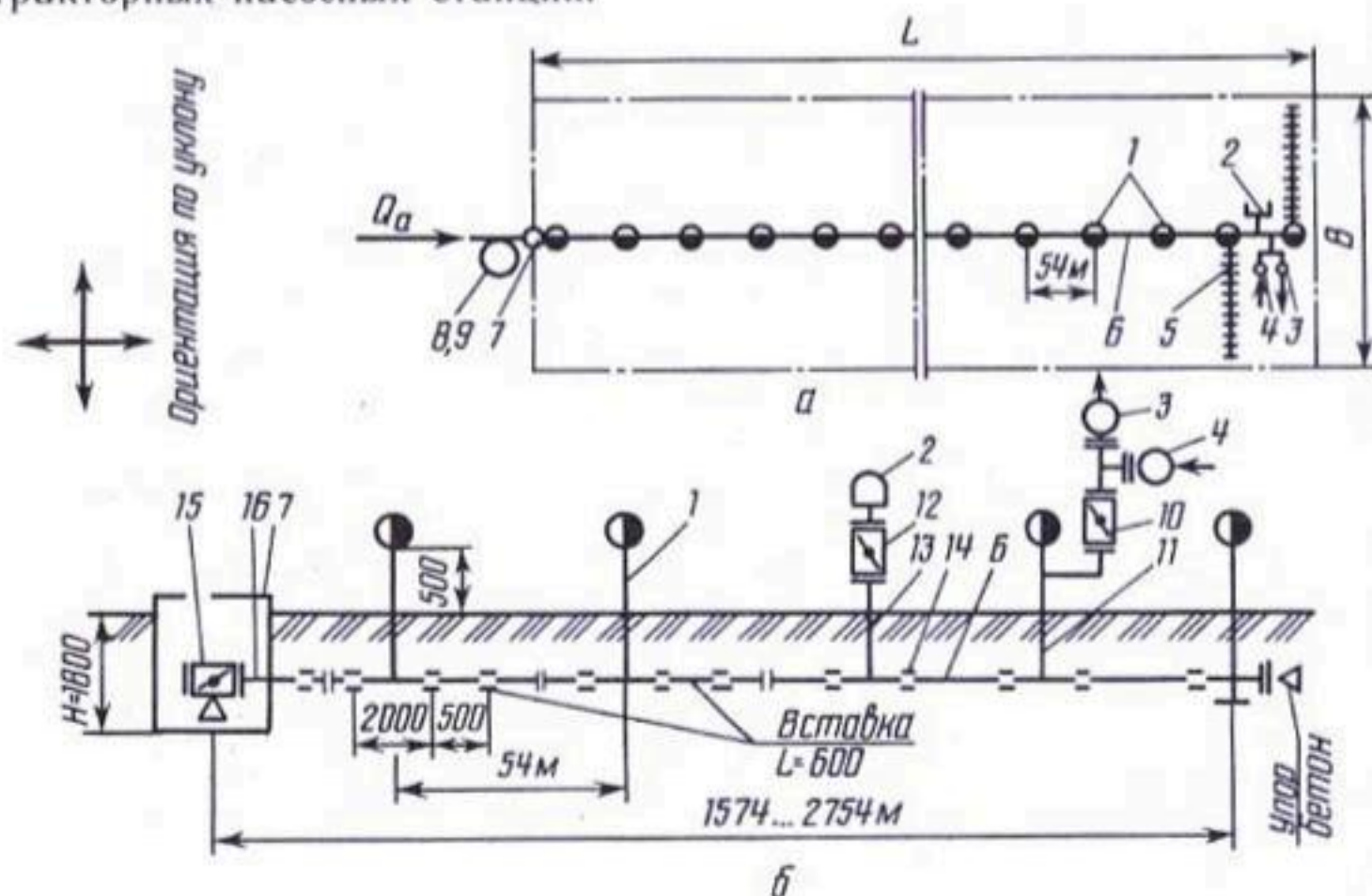
Рис. 3.21. Схема поливного модуля с машиной ДФ-120 «Днепр» (а) и его монтажа (б) (подвод воды к торцу участка, условные обозначения см. табл. 3.33)
