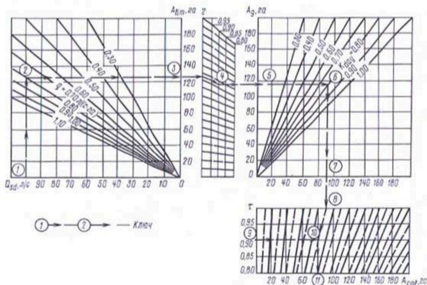
Рис. 3.57. Номограмма для определения сезонной нагрузки на дождевальные машины и установки:
