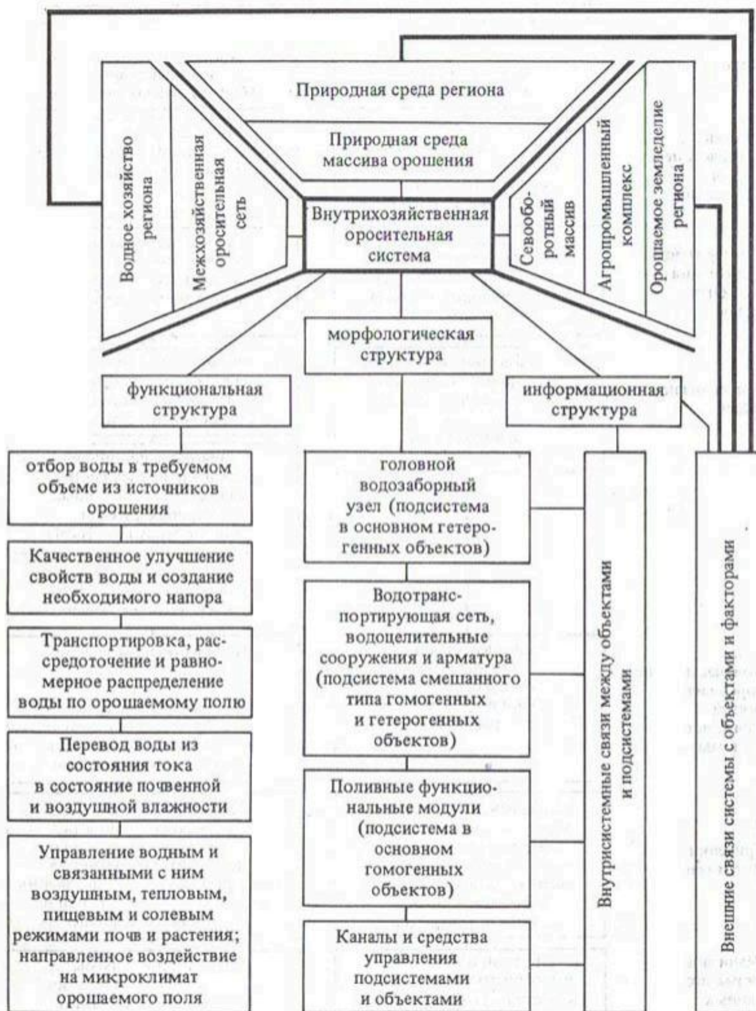
Рис. 1.3. Оросительная система (структурный анализ)
