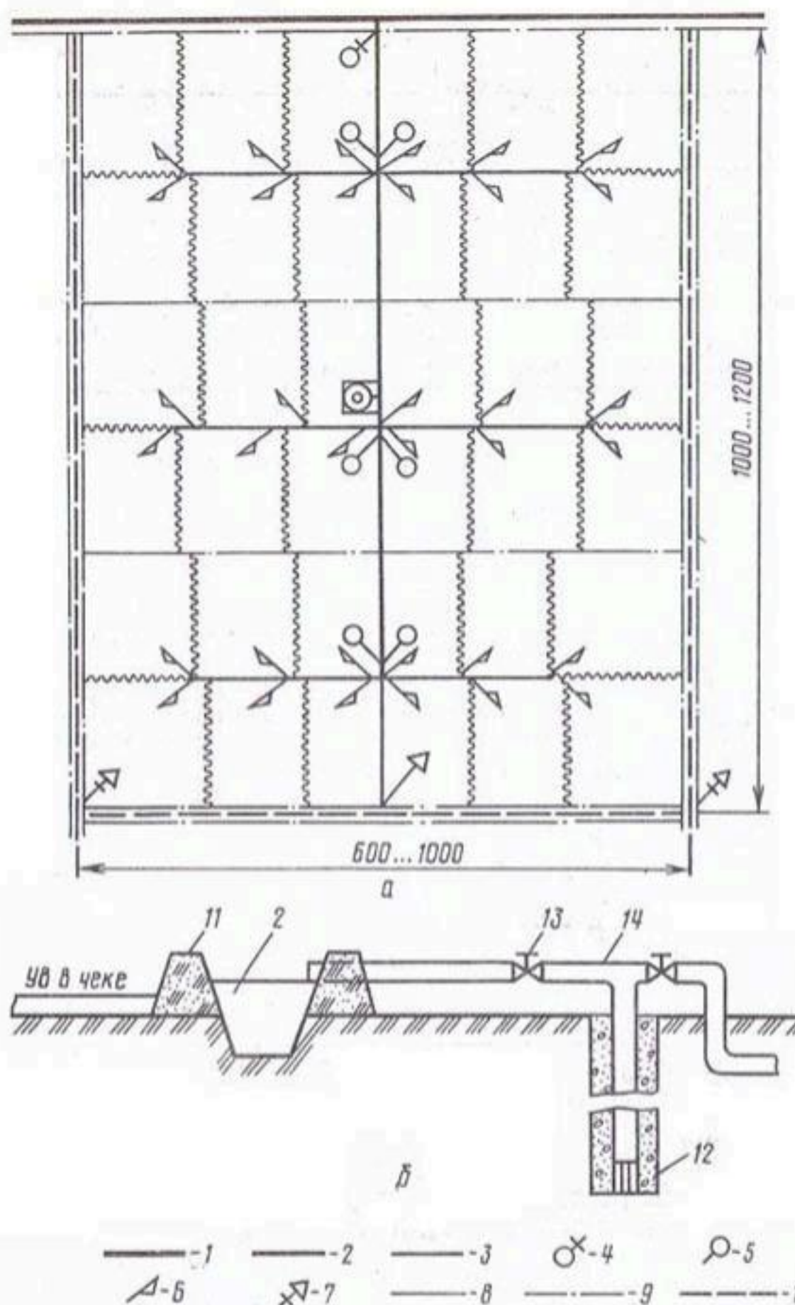
Рис. 2.25. Схема рисовой системы с вертикальным дренажом:
