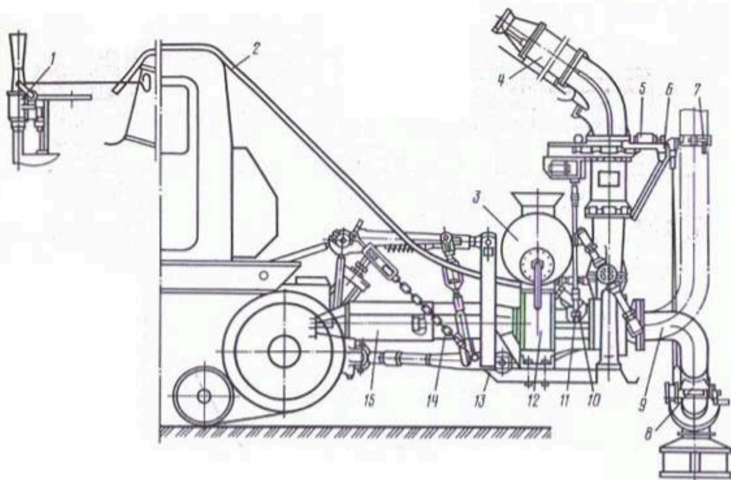
Рис. 3.22. Навесная дождевальная дальнеструйная машина ДДН-70:
