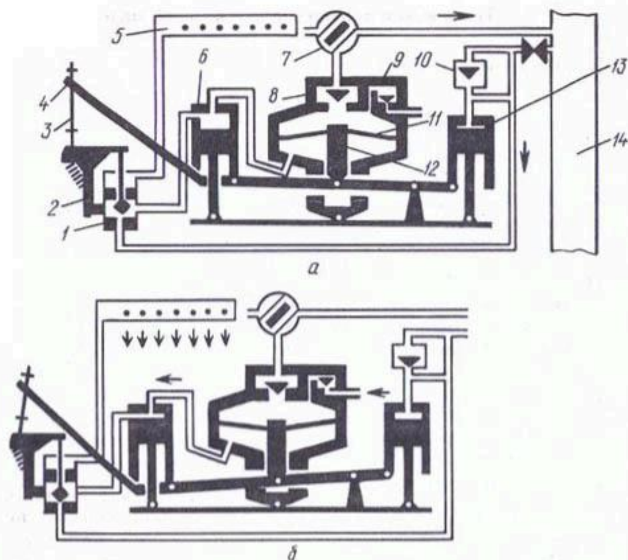
Рис. 3.37. Принципиальная схема работы насоса-дозатора:
