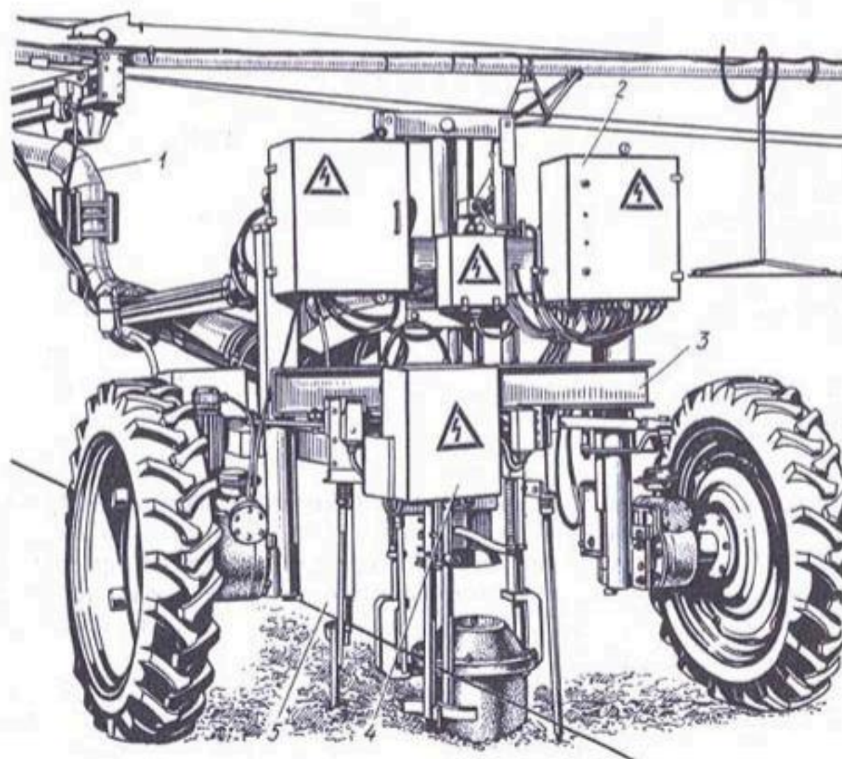
Рис. 3.54. Водозаборно-присоединительное устройство машины «Таврия»:
