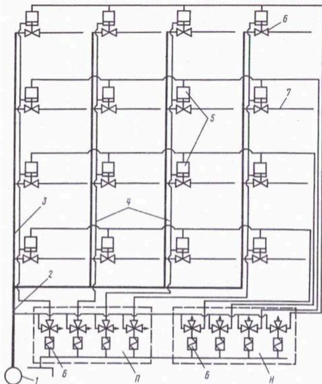
Рис. 4.7. Матричная схема дистанционного управления гидроприводными задвижками:
