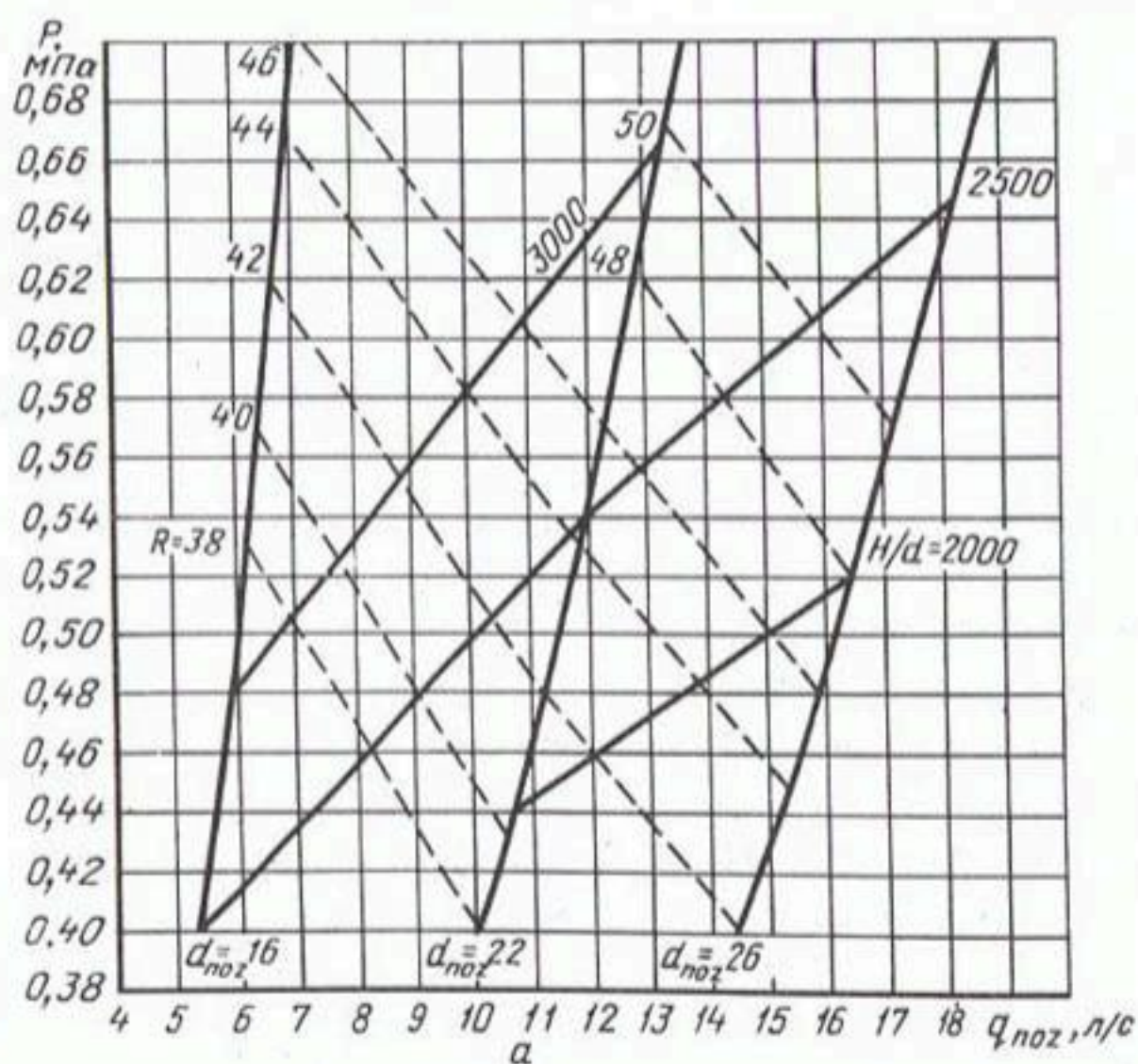
Рис. 3.5. Дальнейструйные дождевальные аппараты и их расходно-напорные характеристики:
