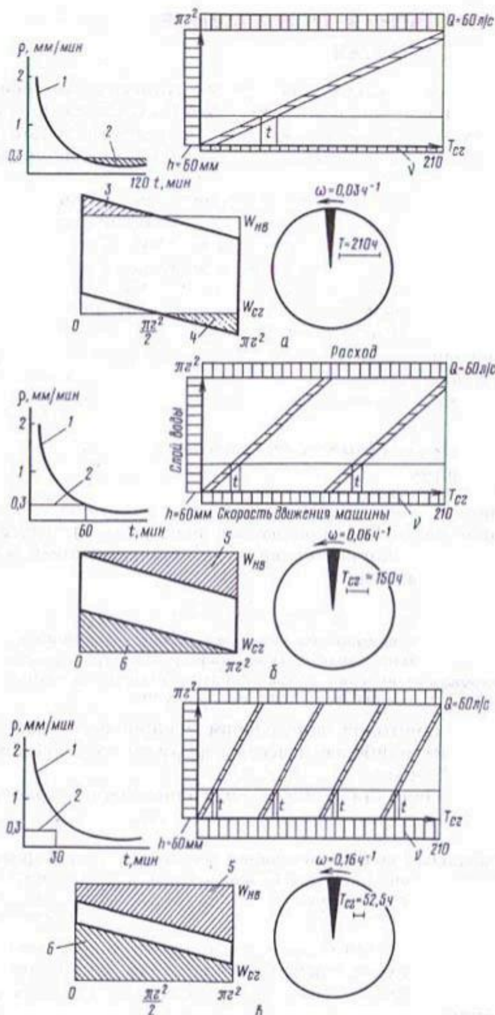
Рис. 1.19. Влияние технологий механизированного полива на параметры эксплуатационного режима орошения на примере использования дождевальная машины кругового действия ДМУ-Б463-60 при поливной норме 600 м³/га:
