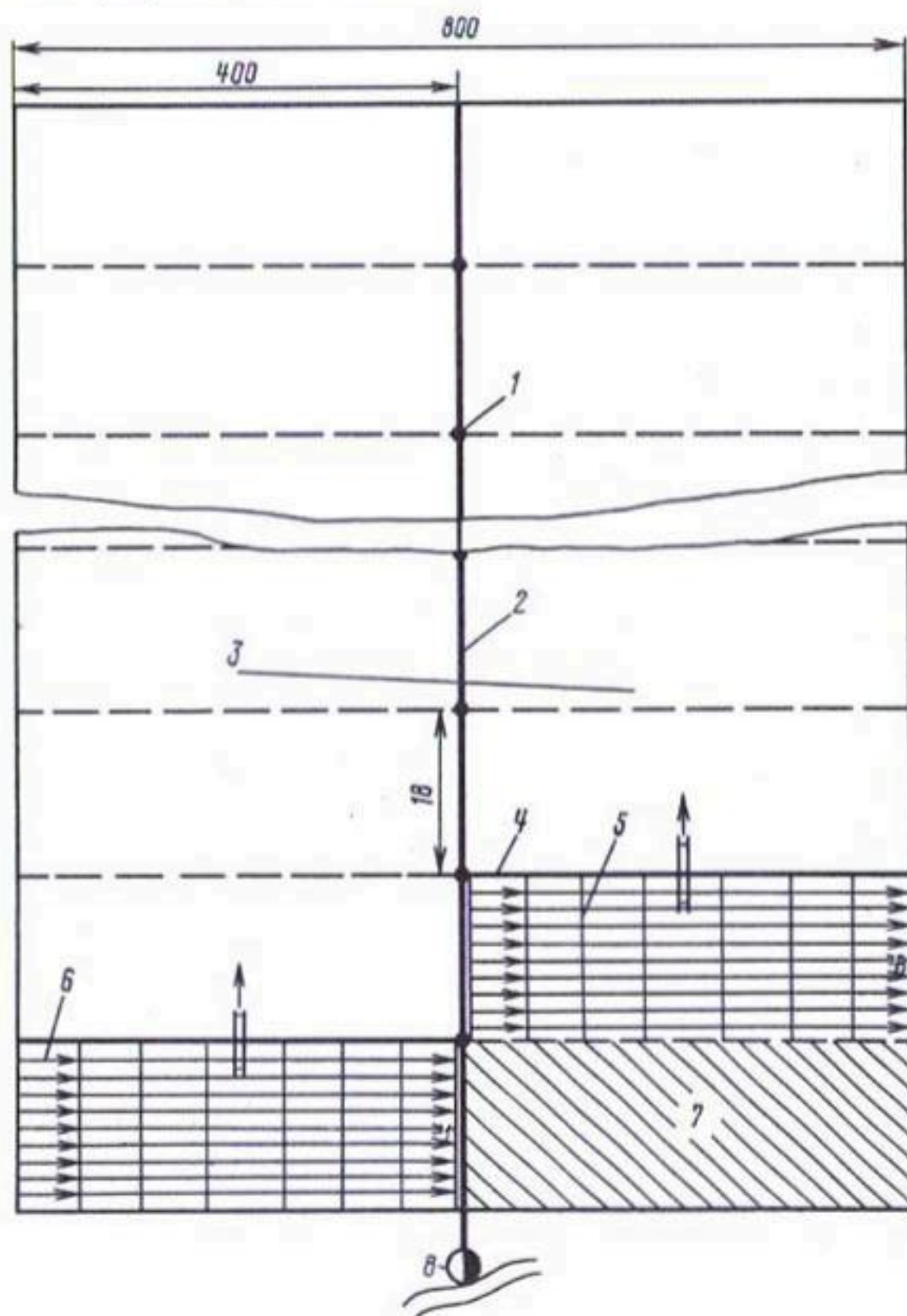
Рис. 2.14. Технологическая схема полива ТКП-90:
