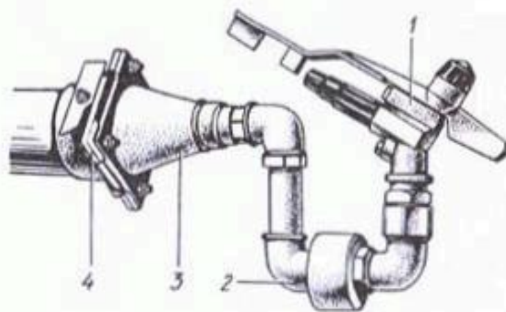
Рис. 3.15. Механизм самоустановки концевой дождевальной вставки машины ДКН-80:
