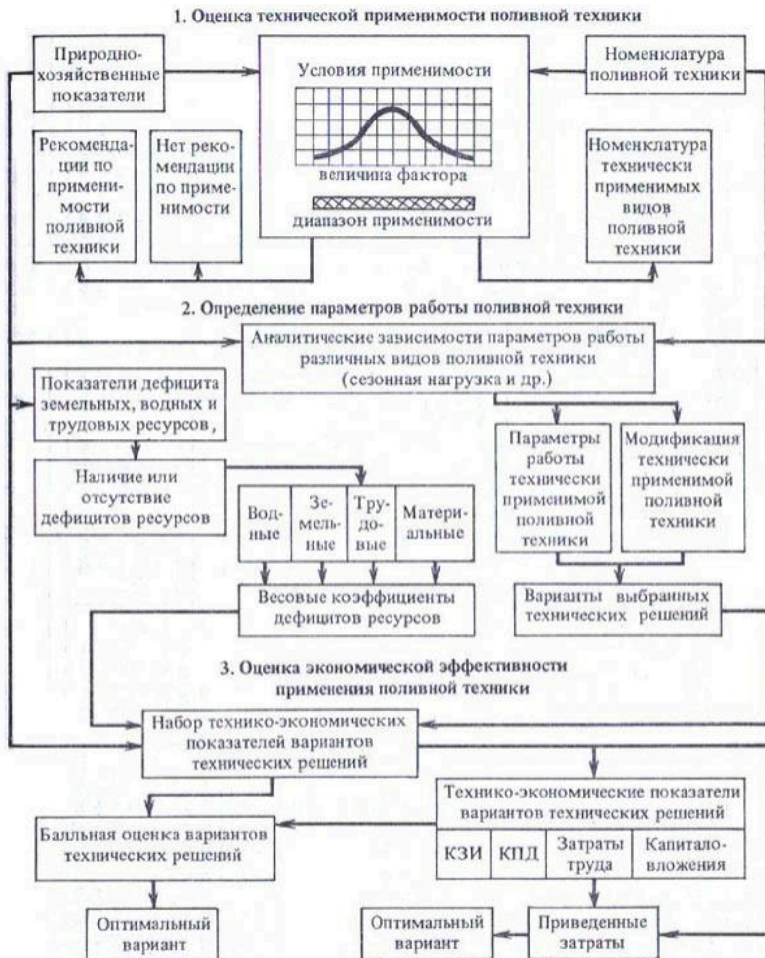
Рис. 1.11. Принципиальная схема оценки применимости при помощи ЭВМ поливной техники в конкретных природно-хозяйственных условиях
