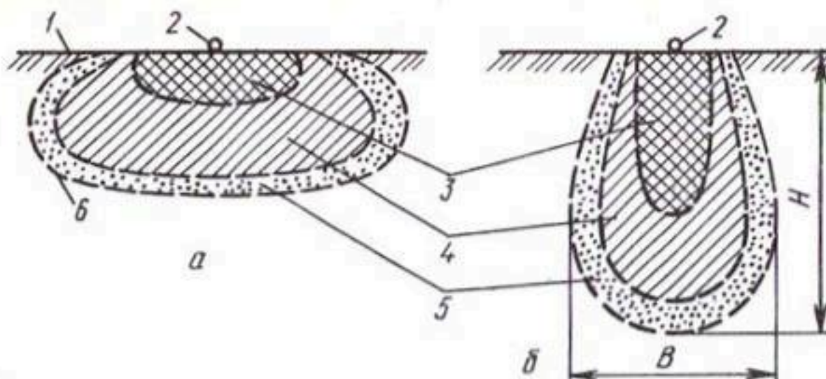
Рис. 4.9. Характерные контуры увлажнения почвы при капельном орошении: a — на тяжелых по механическому составу почвах; б — на легких по механическому составу почвах; 1 — поверхность почвы; 2 — капельный микроводовыпуск; 3, 4, 5 — зоны переувлажненной, нормально увлажненной и частично увлажненной почвы; 6 — контуры зон увлажнения
