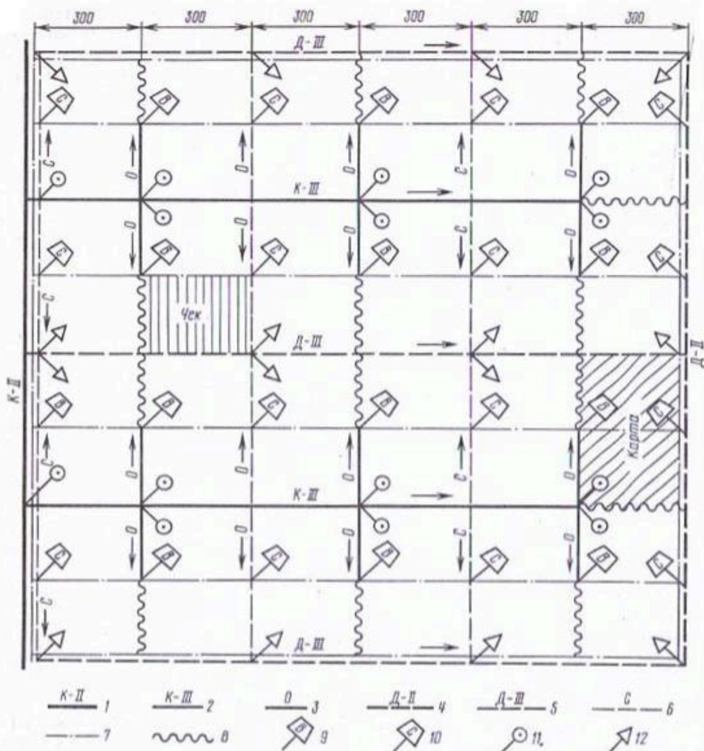
Рис. 2.24. Схема рисовой оросительной системы «Кубанская»:
