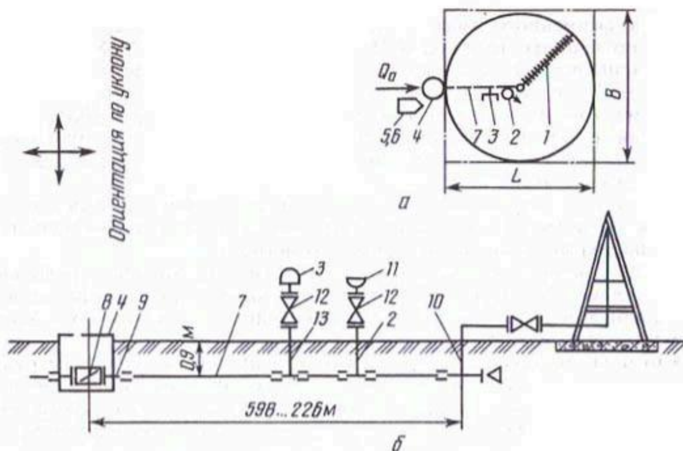
Рис. 3.41. Схема модульного участка с использованием машины «Кубань-ЛК-1» (а) и его монтажа (б) (условные обозначения см. табл. 3.55)
