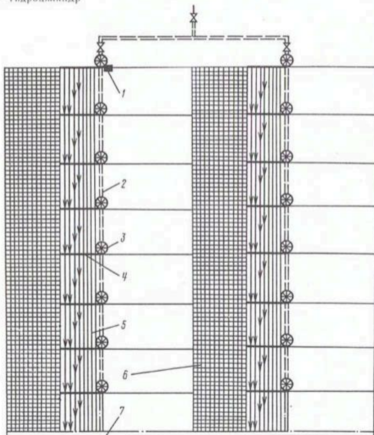
Рис. 2.16. Схема автоматизированной системы со шланговыми поливными устройствами АШУ-32: 1 — генератор импульсов; 2 — оросительный трубопровод; 3 — АШУ-32; 4 — шланг поливной; 5 — поливные борозды; 6 — политая площадь; 7 — канал сбросной
