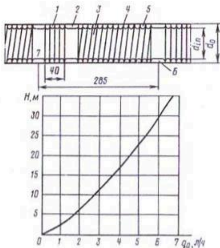
Рис. 4.3. Поливной трубопровод «Аква-Дроп» (а) и его расходно-напорная характеристика (б):
