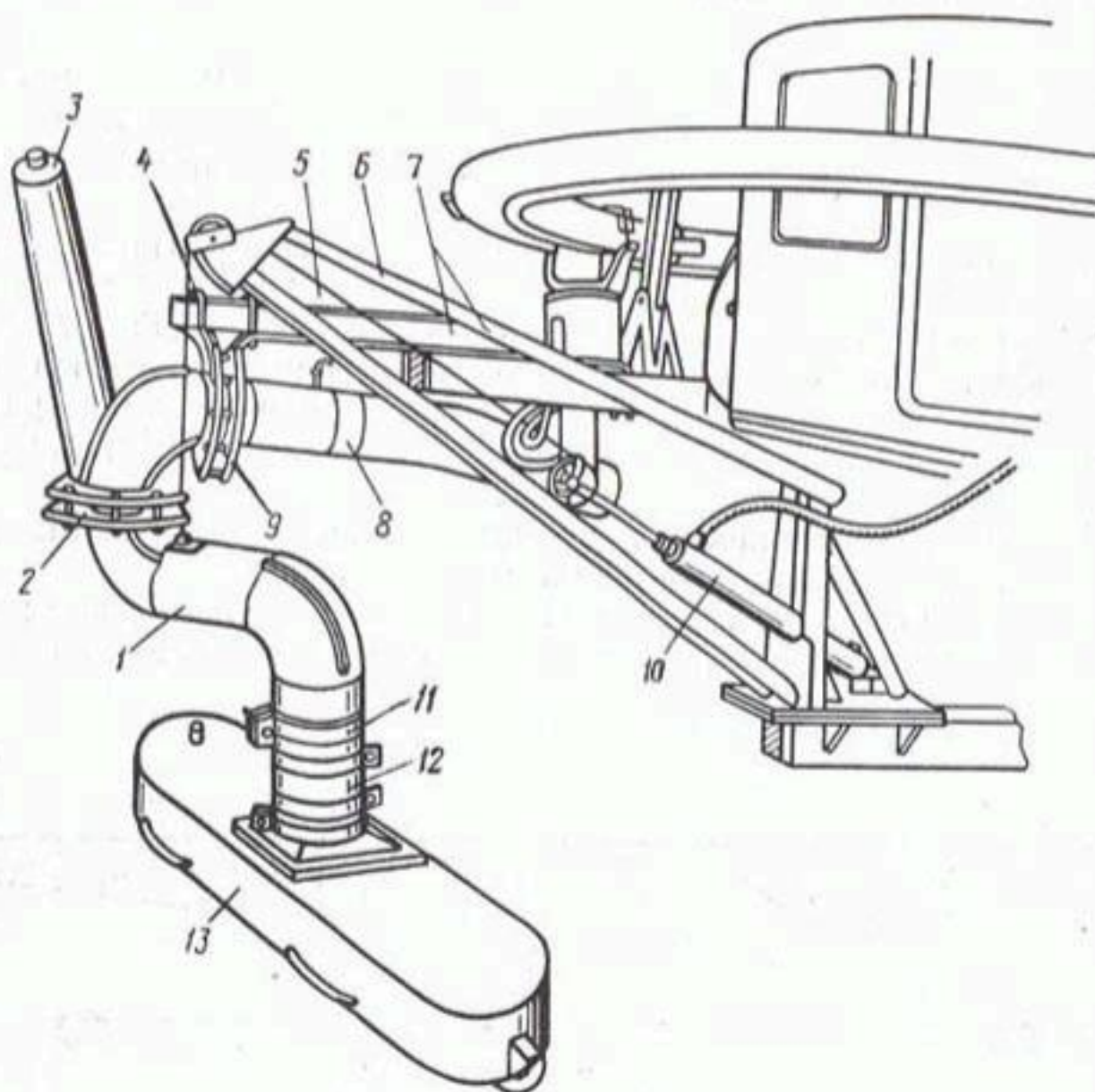
Рис. 3.49. Всасывающая линия:
