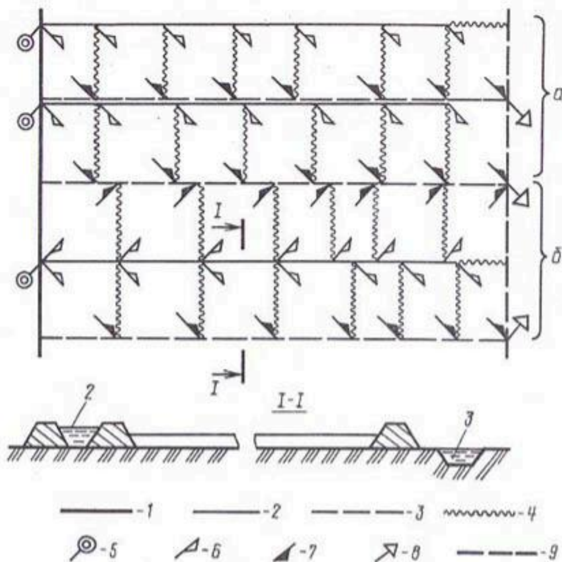
Рис. 2.21. Схема карты краснодарского типа:
