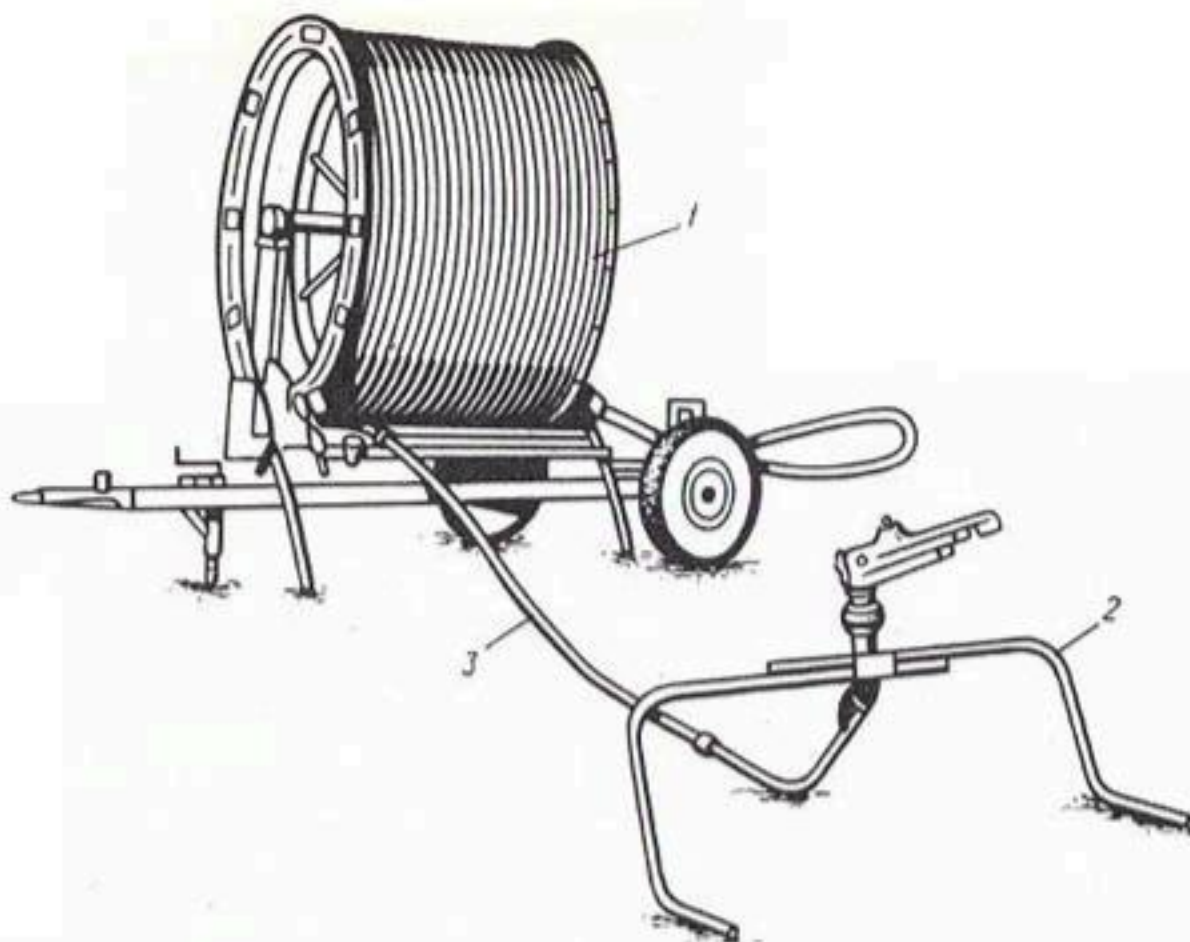
Рис. 3.31. Общий вид дождевального оборудования РЗТ-75: 1 — шасси с намоточным устройством; 2 — салазки с дождевальным аппаратом; 3 — полиэтиленовый шланг
