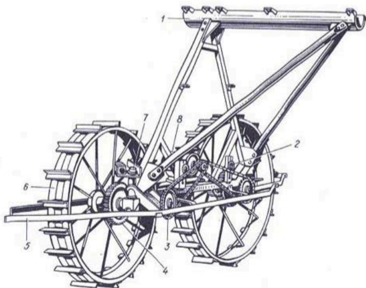
Рис. 3.20. Опорная тележка машины ДФ-120 «Днепр»: 1 — желоб; 2 — натяжная звездочка; 3, 4 — цепная и зубчатая передачи; 5 — стеблеотвод; 6 — колесо; 7 — ось; 8 — горизонтальный мотор-редуктор
