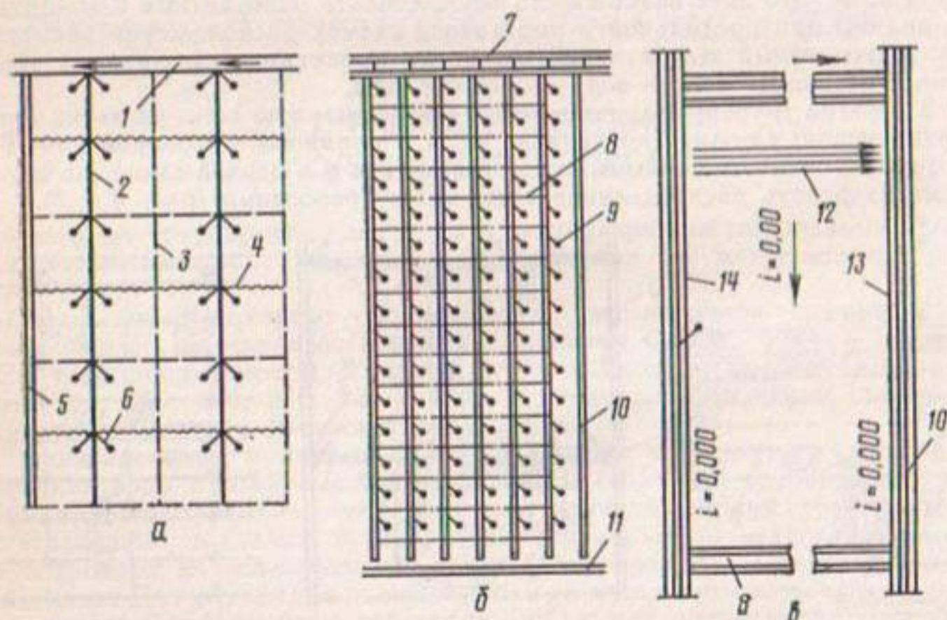
Рис. 4.5. Схемы сети для полива по постоянным участкам при очень малых уклонах (0,0005. . . 0,0003):
