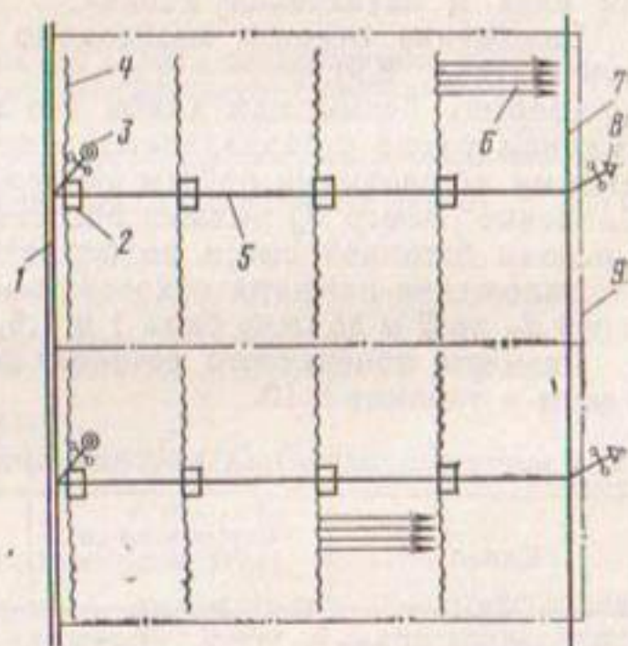
Рис. 8.7. Организация территории и схема оросительной сети при поливе по бороздам с применением агрегата ППА-165У:
