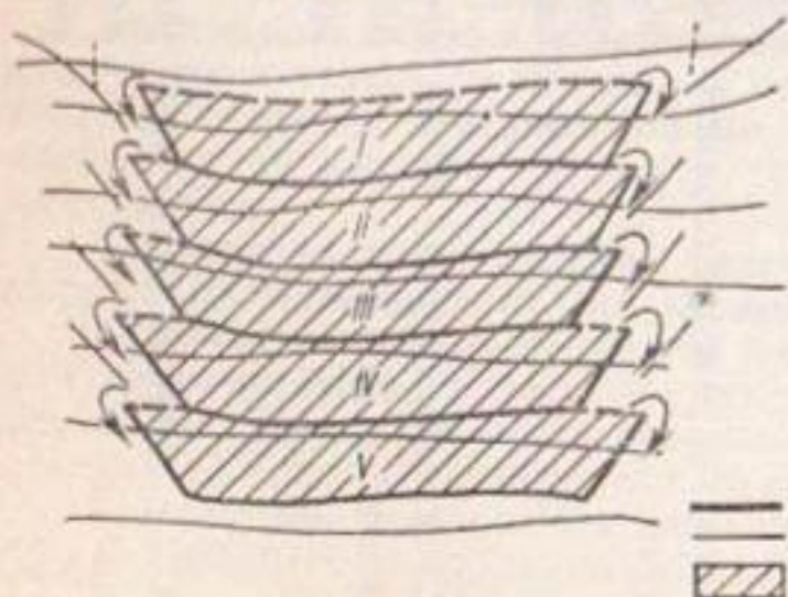
Рис. 10.2. Система мелкоярусных лиманов, устроенная на пологом склоне:
