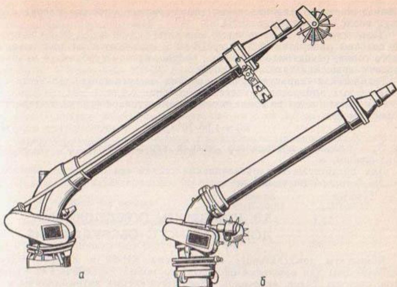
Рис. 5.12. Дальнеструйные дождевальные аппараты ДД-50 (а) и ДД-80 (б)
