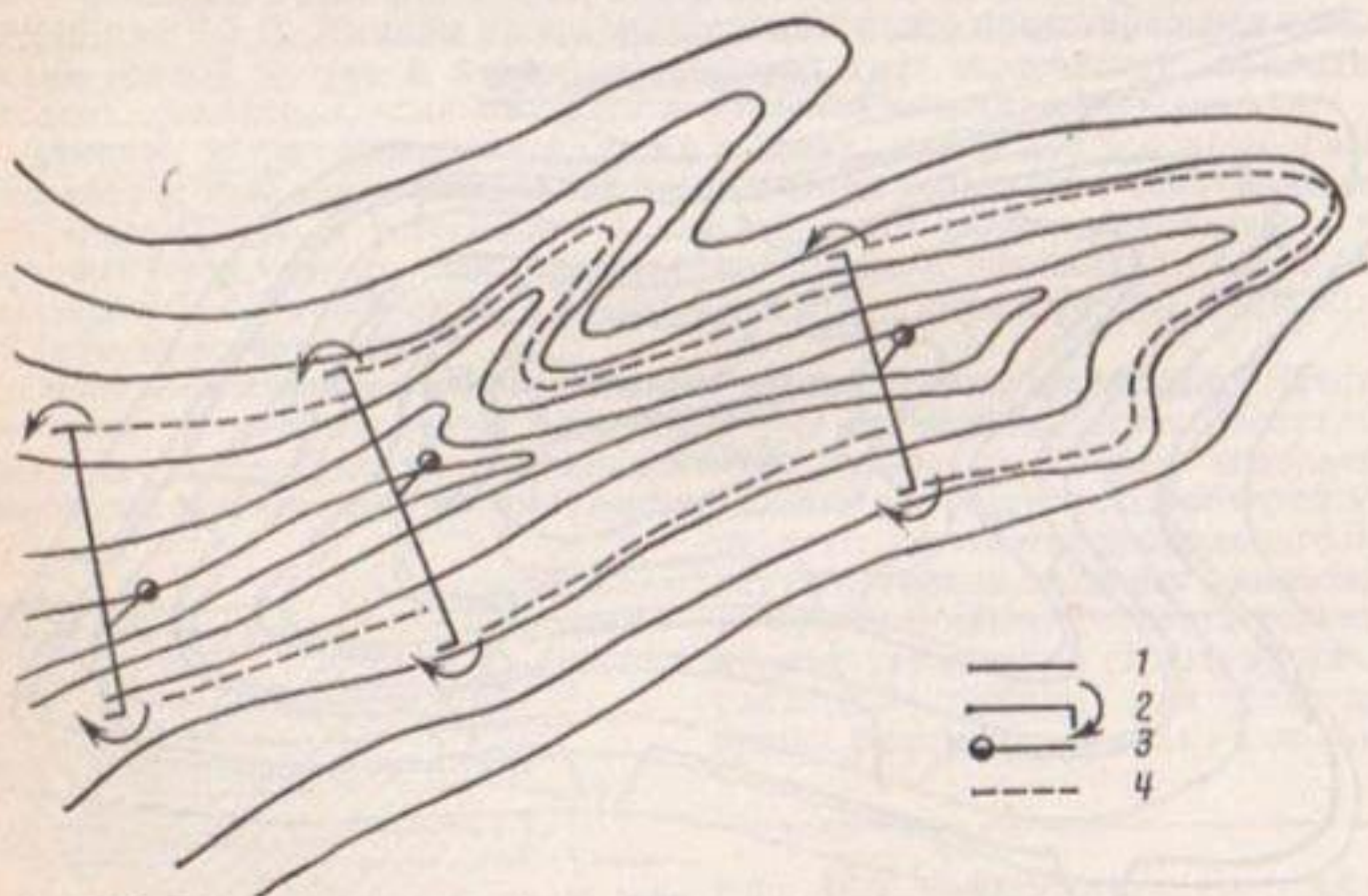
Рис. 10.5. Система ярусных лиманов глубокого затопления, устраиваемая на протяжинах:
