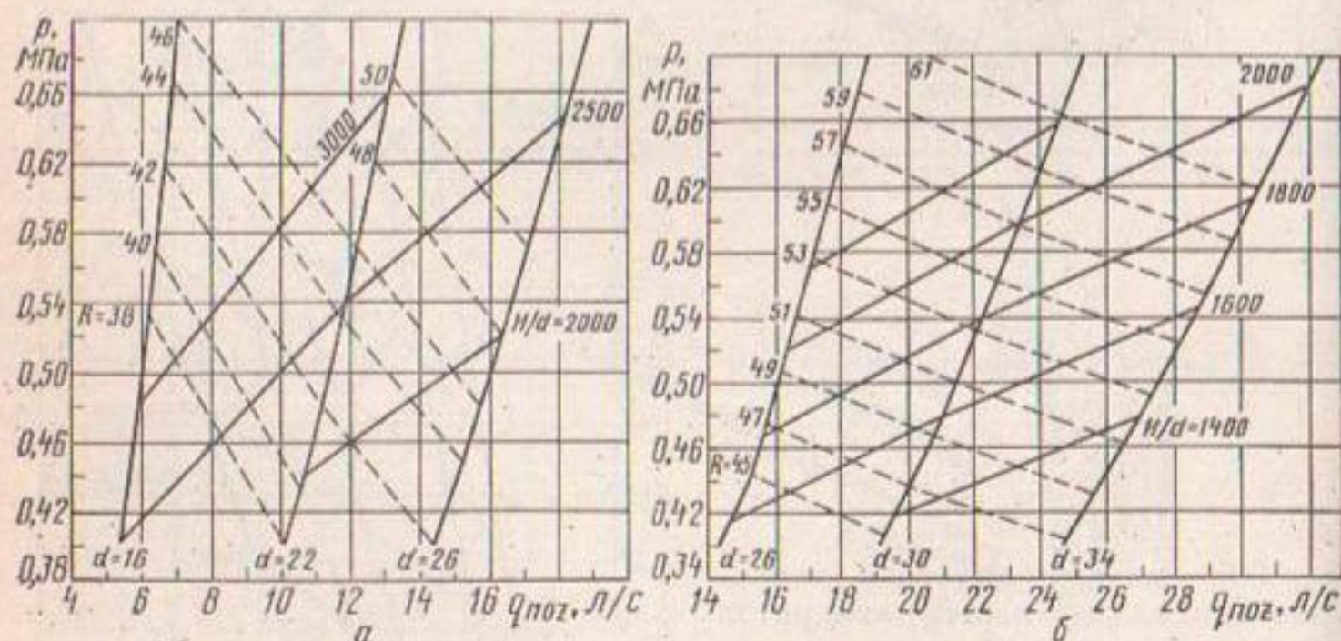
Рис. 5.11. Расходно-напорная характеристика дальнеструйных дождевальных аппаратов:
