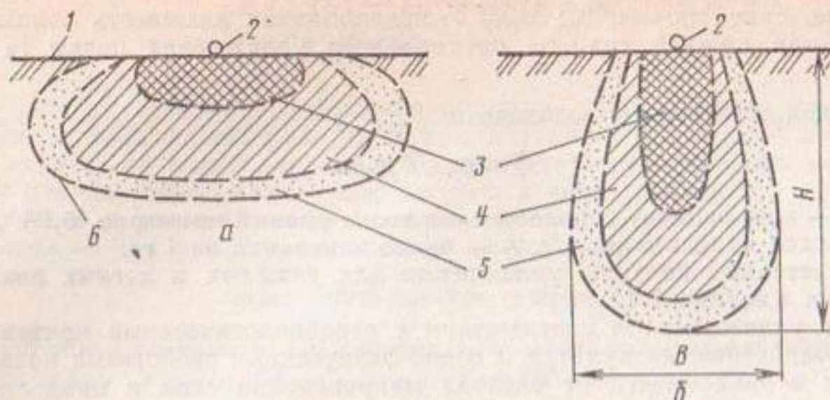
Рис. 7.12. Характерные контуры увлажнения при капельном орошении: а — на тяжелых по механическому составу почвах; б — на легких по механическому составу почвах; 1 — поверхность почвы; 2 — капельный микроводовыпуск; 3 — очаг переувлажненной почвы; 4 — очаг нормально увлажненной почвы; 5 — очаг частично увлажненной почвы; 6 — граница распространения увлажнения
