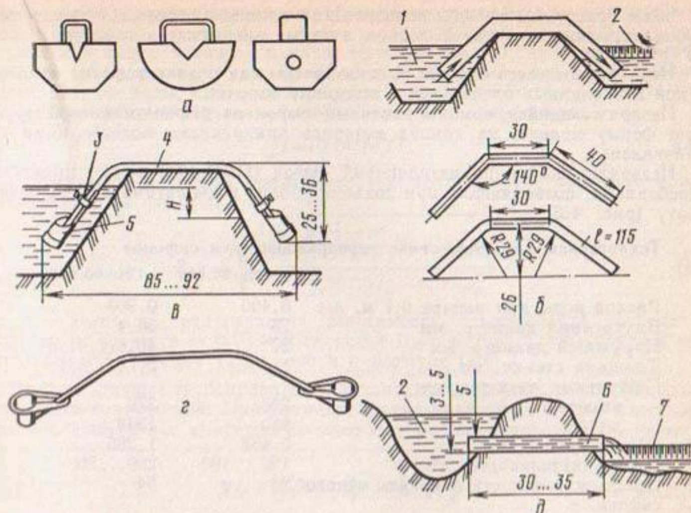
Рис. 4.2. Поливная арматура:
