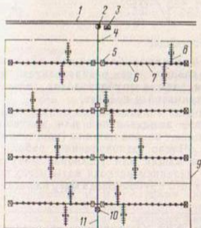
Рис. 8.20. Организация территории и схема оросительной сети при использовании дождевальных машин ДКШ-64 «Волжанка»; ДКГ-80 «Ока» и ДКН-80:
