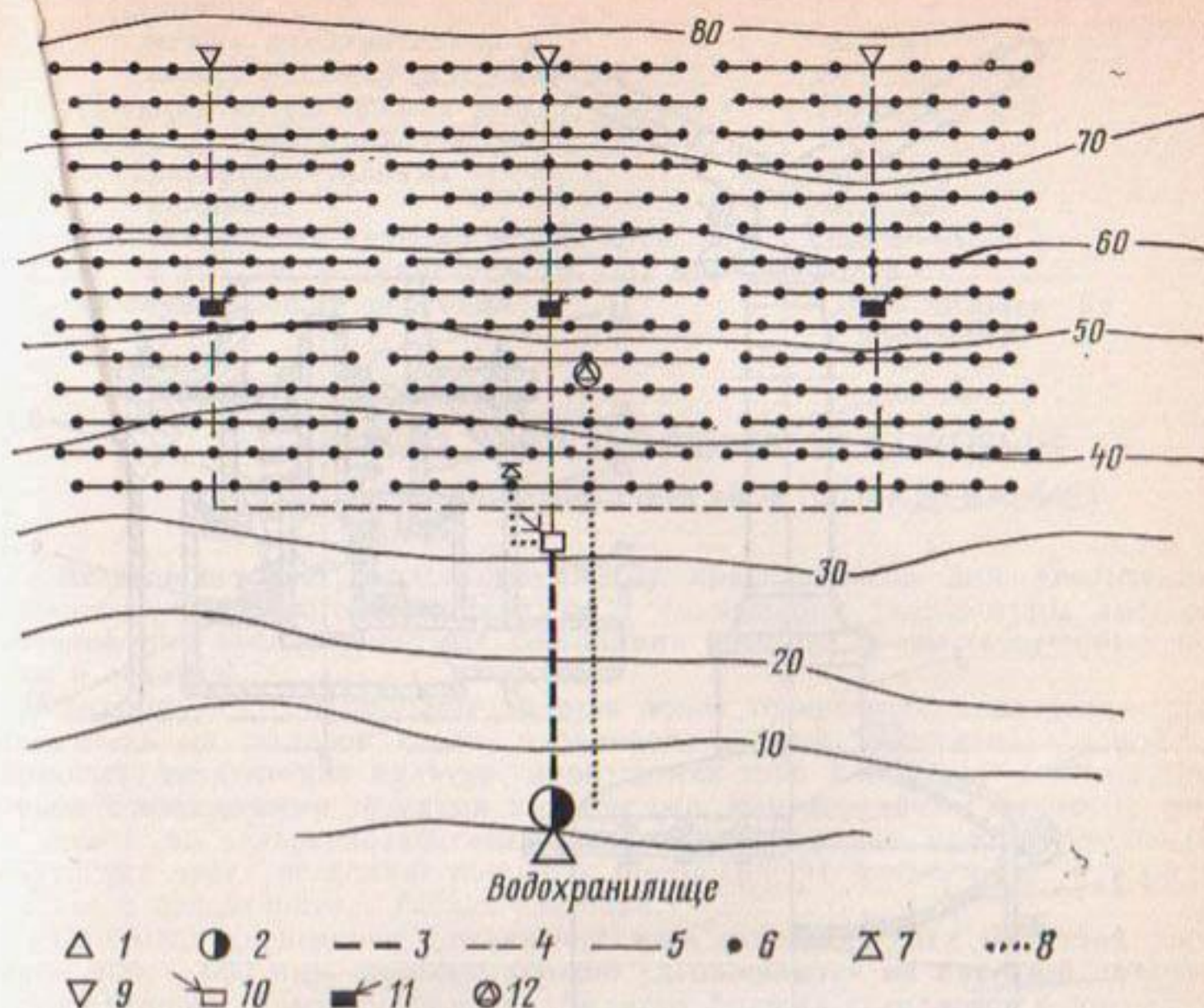
Рис. 5.33. Принципиальная схема системы синхронного импульсного дождевания:
