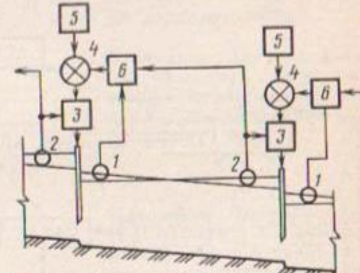
Рис. 14.6. Схема регулирования объемов воды в открытом канале:
