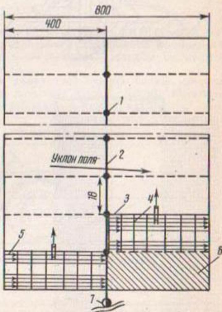
Рис. 4.11. Муфта с поливным шлейфом колесного трубопровода ТКП-90
