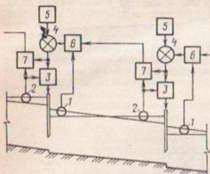
Рис. 14.7. Схема регулирования объемов воды в открытом канале при последовательном суммировании:
