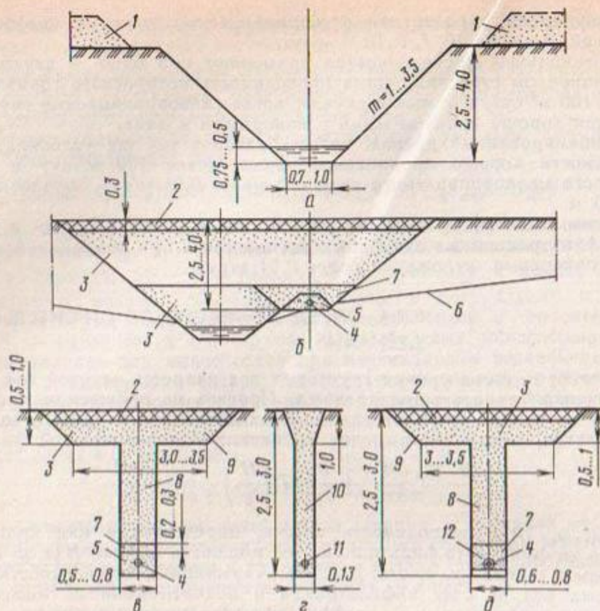
Рис. 8.28. Поперечные сечения дрена:
