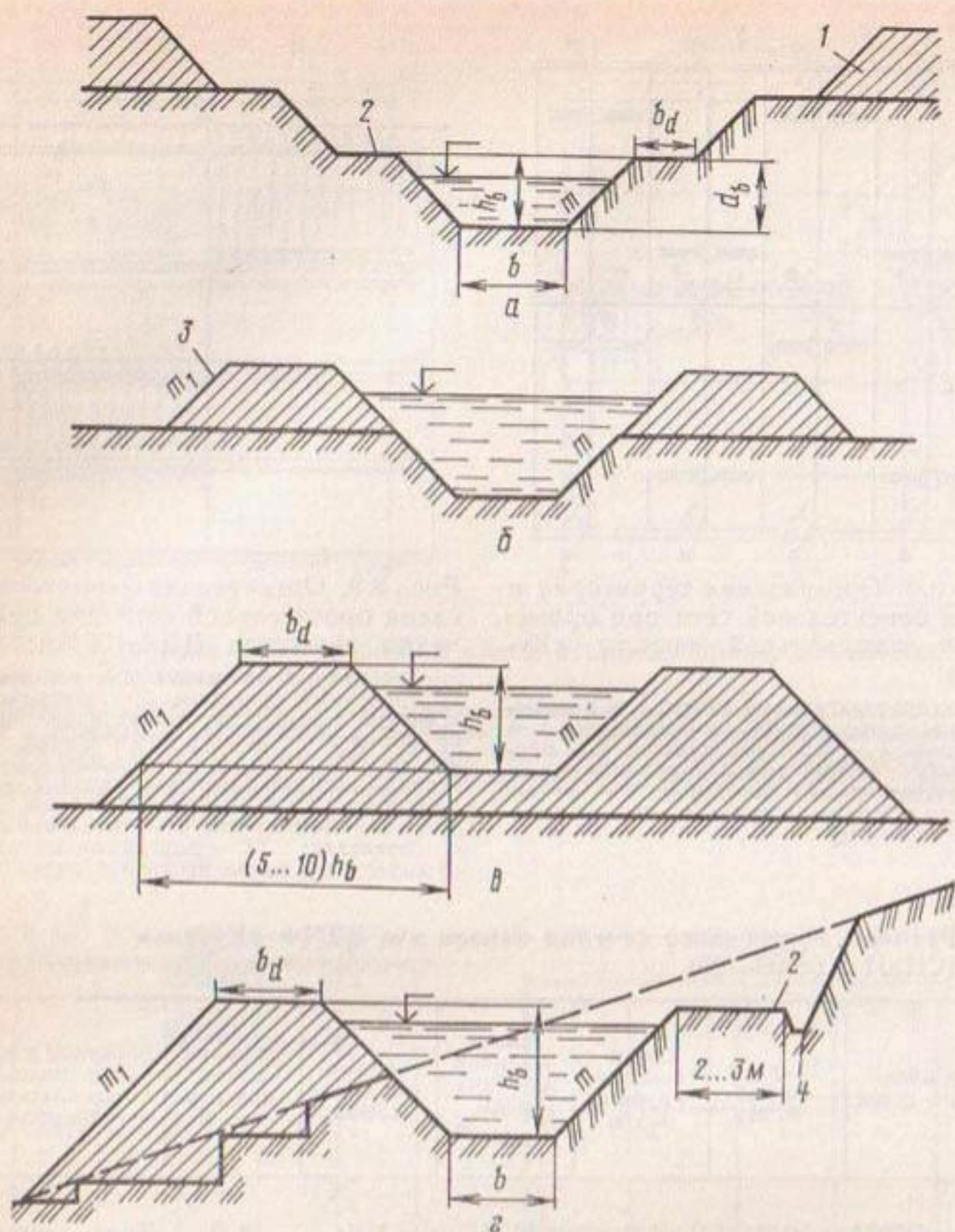
Рис. 8.10. Конструкции каналов:
