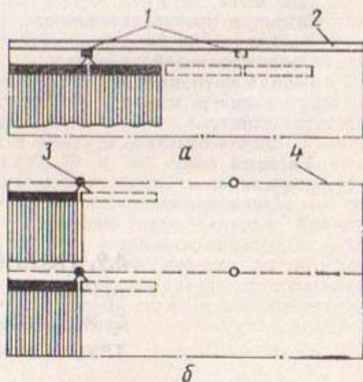
Рис. 4.10. Полив АПШ-1:
