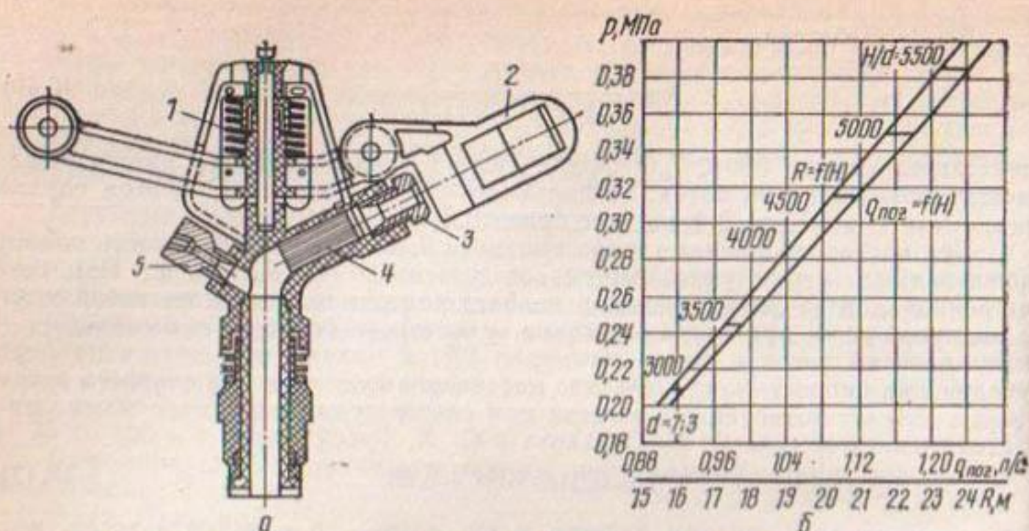
Рис. 5.6. Среднеструйный дождевальнй аппарат ДКШ-64.00.060 (а) и его расходно-напорная характеристика (б):
