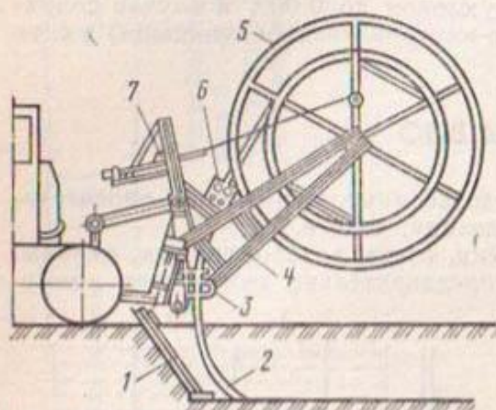
Рис. 6.7. Схема НБУ-ПТ:
