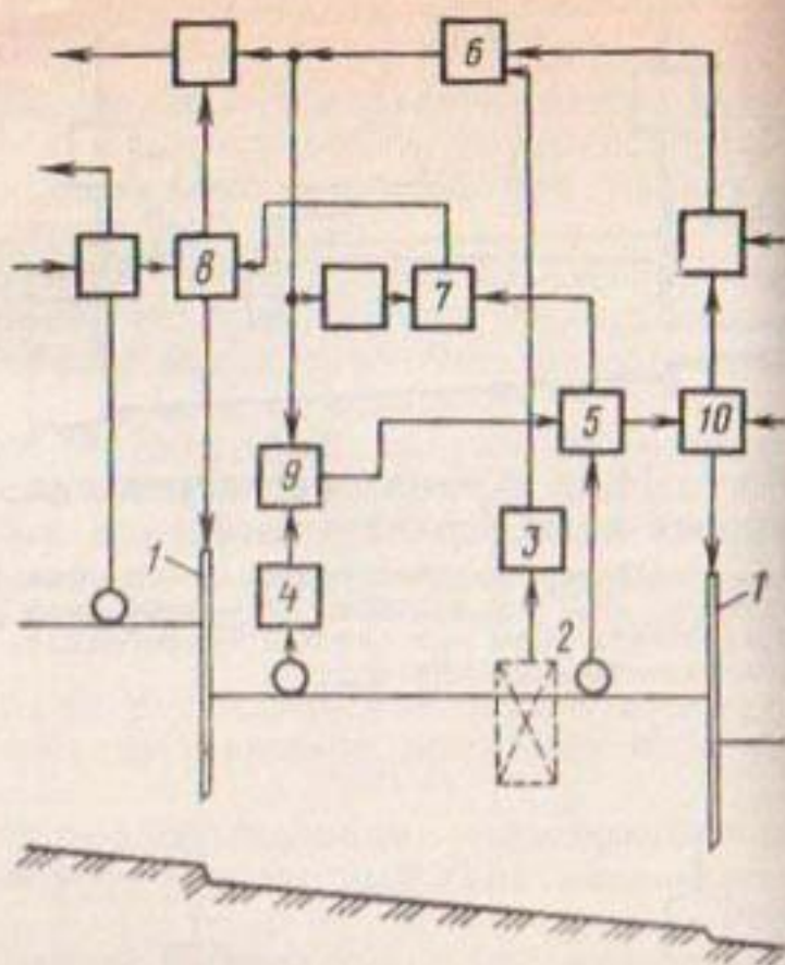
Рис. 14.8. Схема регулирования уровней воды с перекрестными обратными связями:
