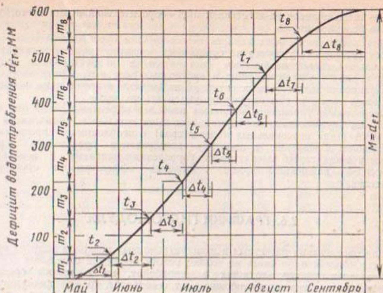
Рис. 2.3. Графоаналитический расчет режима орошения сахарной свеклы: m — поливная норма, мм; \Delta t — межполивный период в днях; t — средняя дата полива; M — оросительная норма, мм
