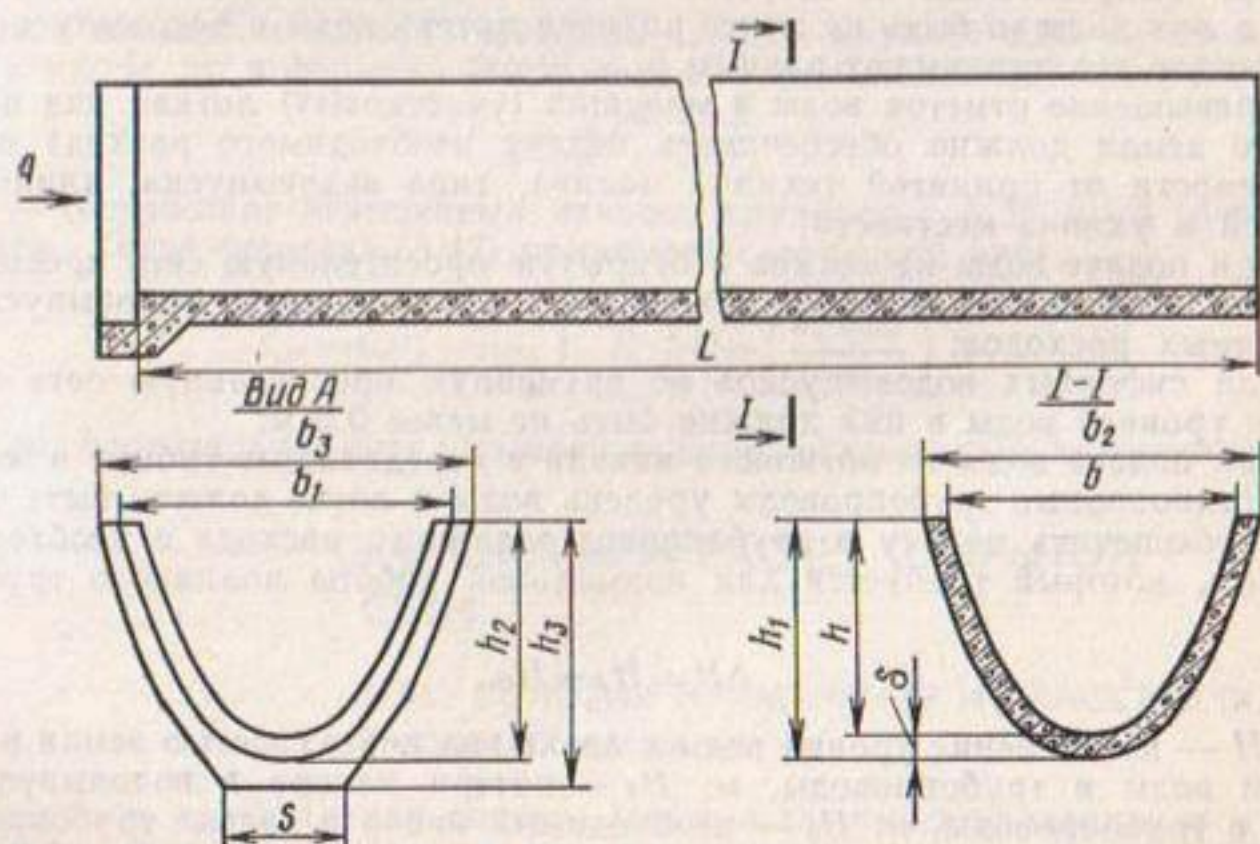
Рис. 8.12. Конструкции лотков
