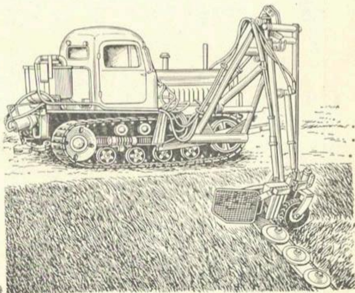
Рис. 7.6. Мелиоративная косилка К-48Б.
