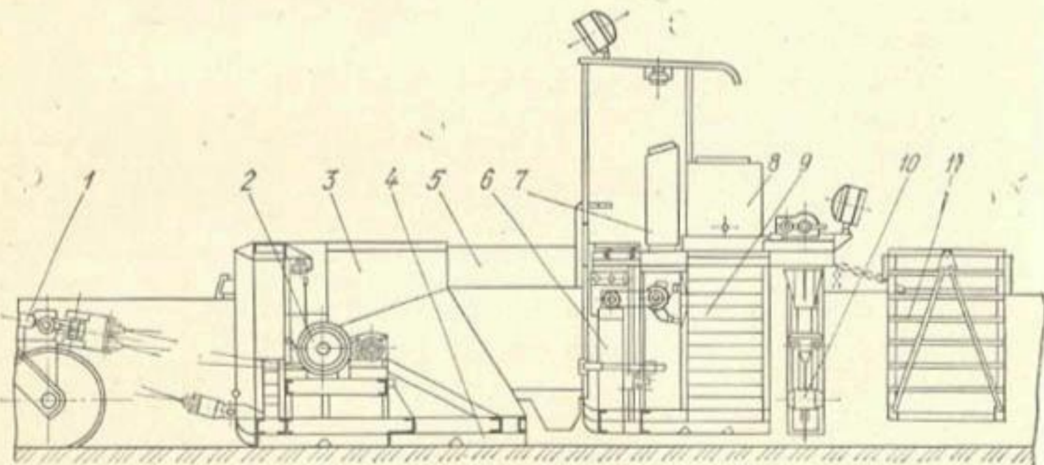
Рис. 2.26. Схема виброформы:
