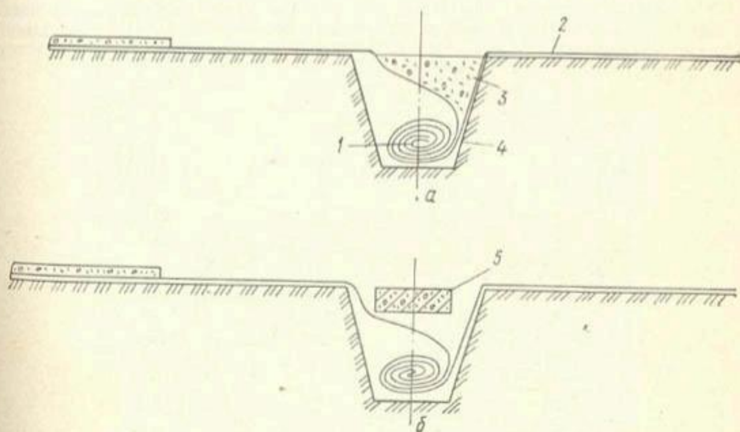
Рис. 2.9. Схемы устройства стыков пленочных экранов:
