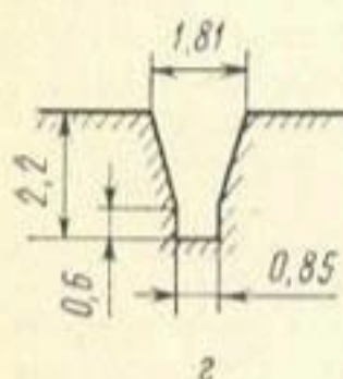
Рис. 2.23. Профили выемок, образуемых роторными траншейными экскаваторами:
