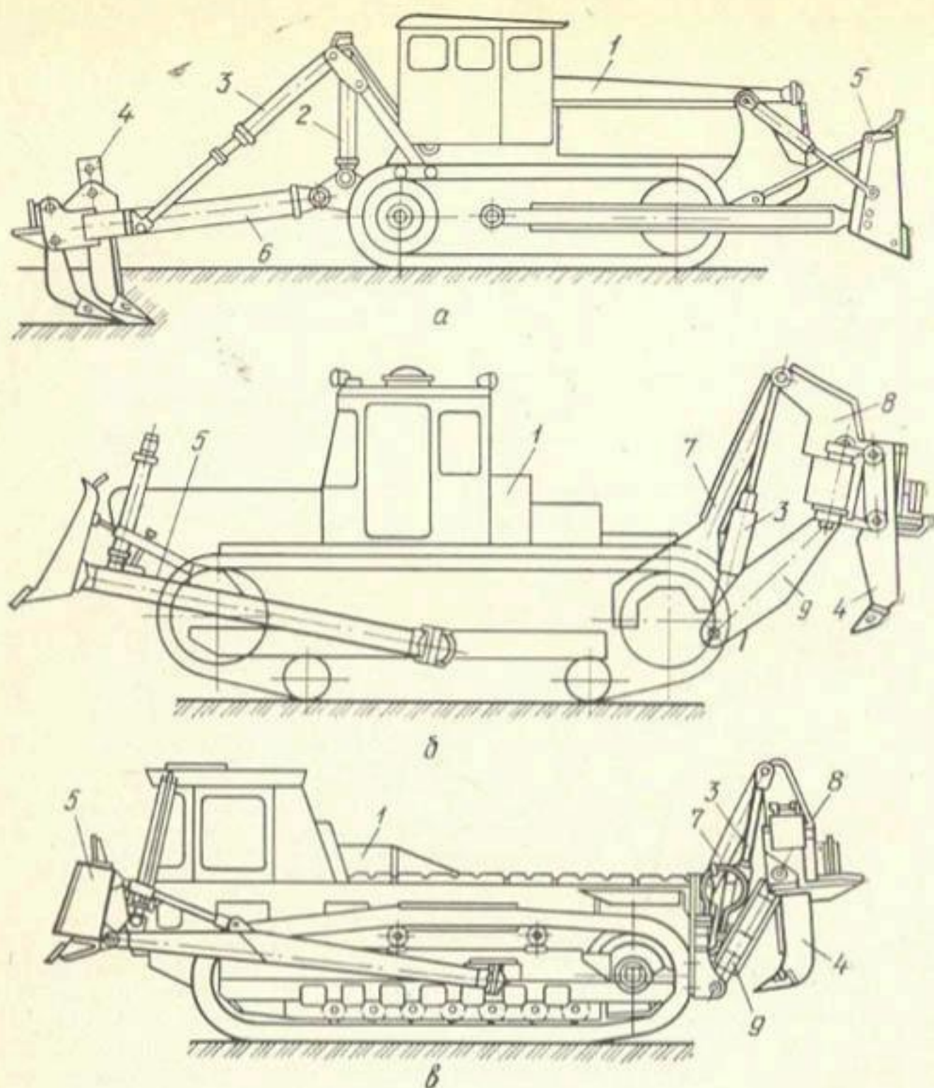
Рис. 5.13. Навесные рыхлители:
