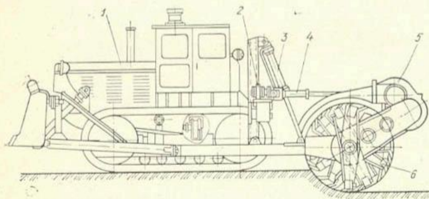
Рис. 5.18. Землеройно-фрезерная машина:
