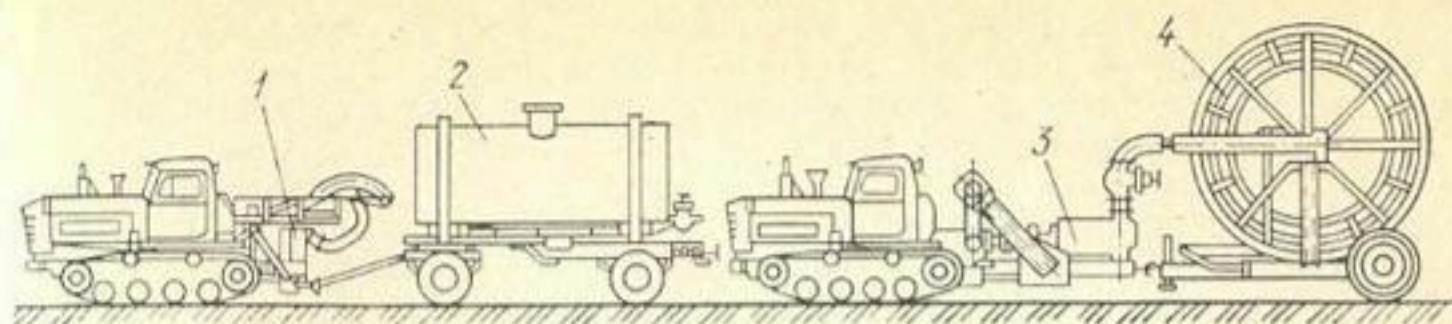
Рис. 7.7. Машина для промывки дрен ПДТ-125:
