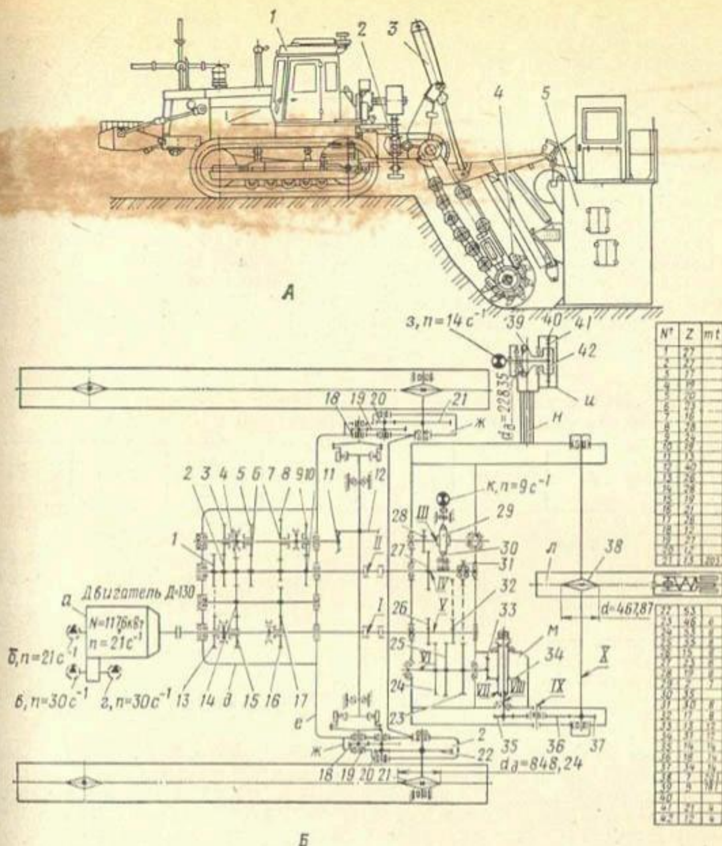
Рис. 5.21. Экскаватор-дреноукладчик ЭТЦ-20б:
