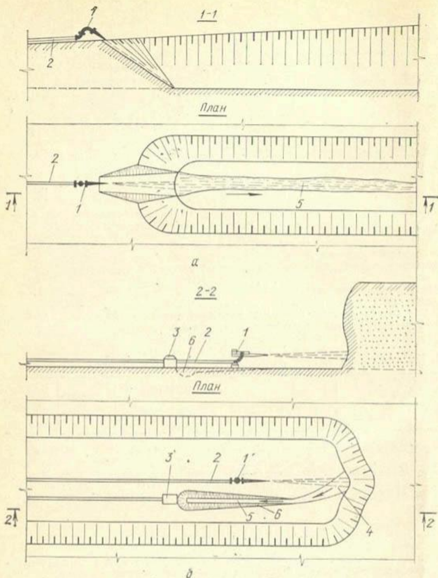
Рис. 2.3. Схемы гидромониторной разработки грунта разрывом попутного (а) и встречного (б) забоя:
