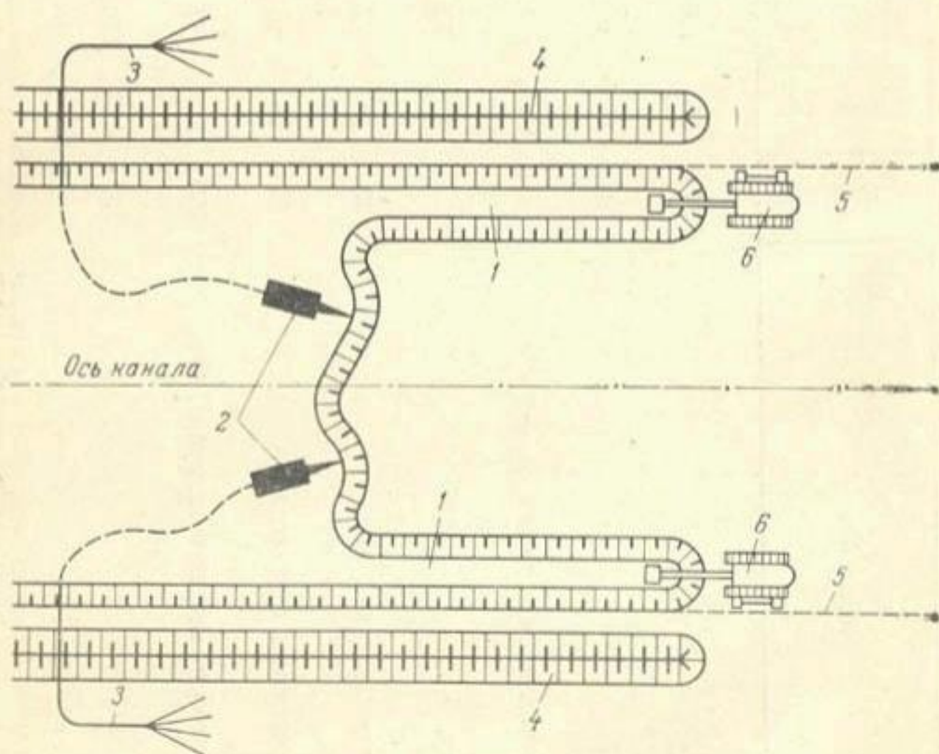
Рис. 2.5. Схема комбинированной разработки канала земснарядами и экскаваторами:
