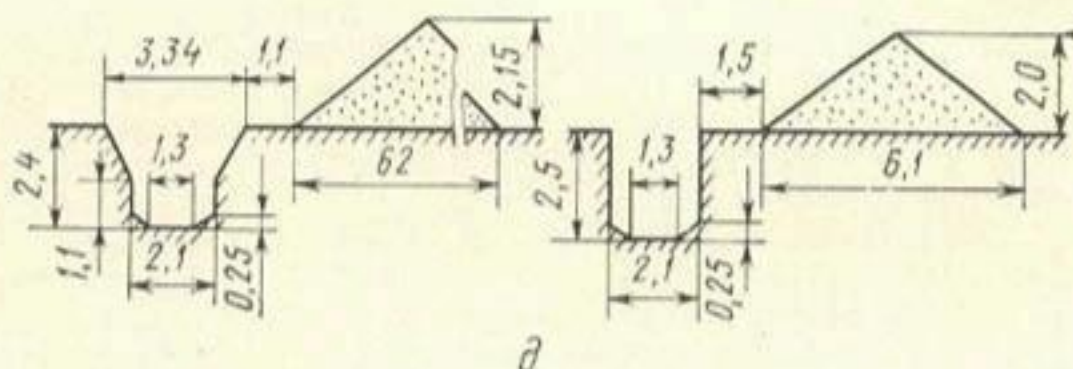
Рис. 2.23. Профили выемок, образуемых роторными траншейными экскаваторами:
