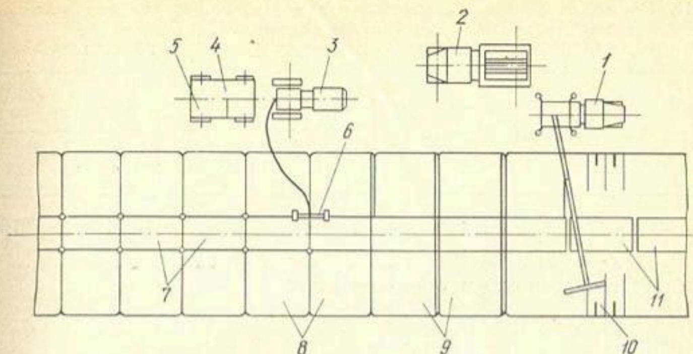
Рис. 2.7. Схема монтажа сборных облицовок оросительных каналов с обжатыми швами на гидроизоляционных прокладках:
