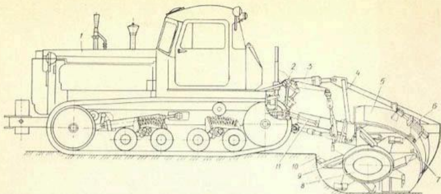
Рис. 2.18. Схема плужно-роторного каналокопателя МК-17:
