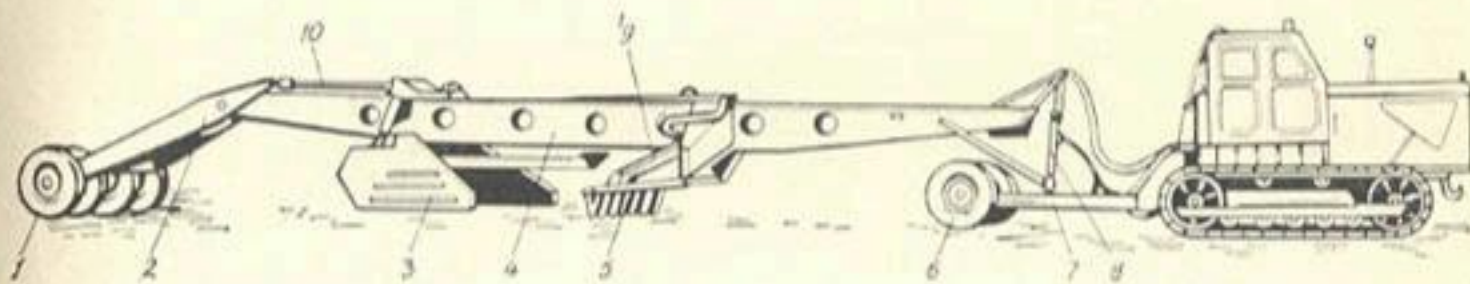
Рис. 4.7. Планировщик ДЗ-602:
