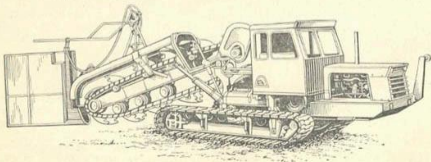
Рис. 2.29. Экскаватор-дреноукладчик ЭТЦ-202А.
