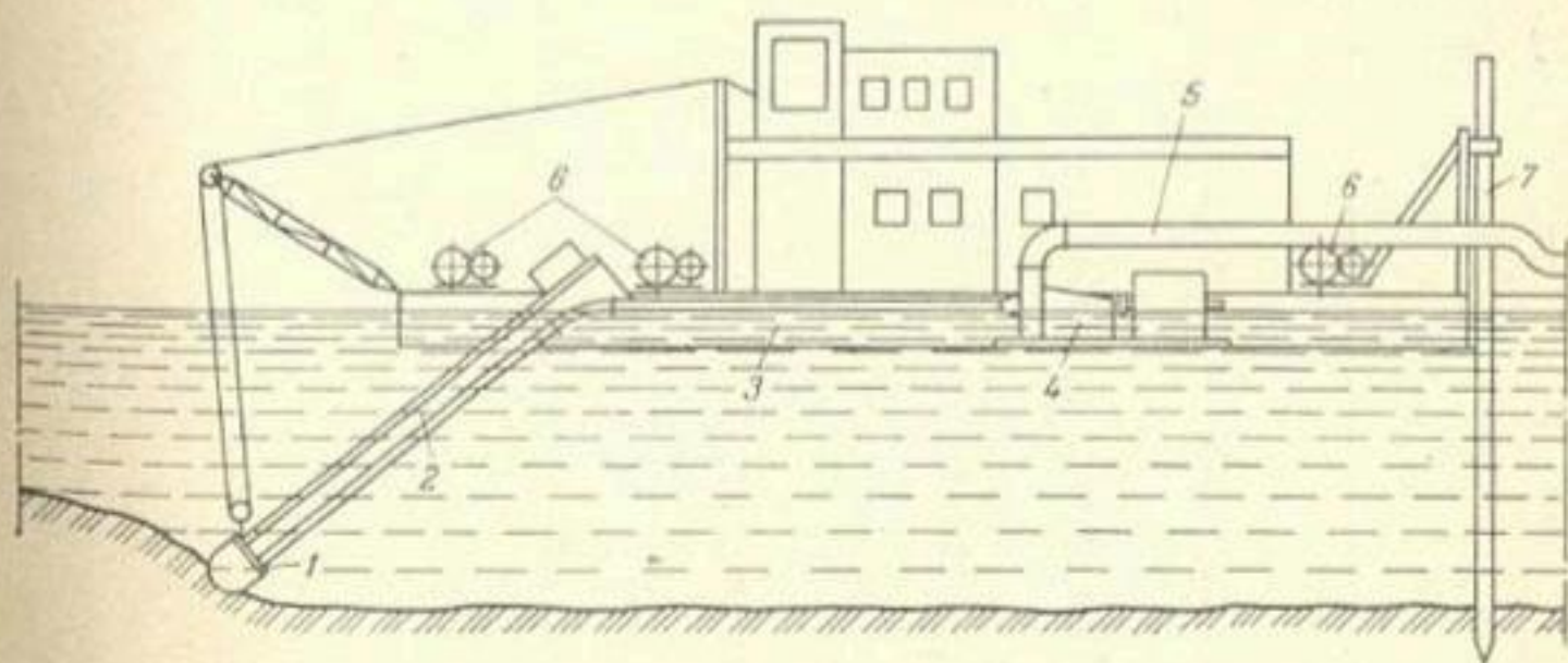
Рис. 2.4. Схема земснаряда.
