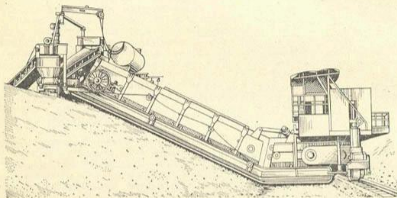
Рис. 2.28. Комплексы машин для облицовки монолитным бетоном каналов глубиной 3...5 м:
