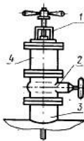
1 — сальниковый ввод; 2 — задвижка (затвор); 3 — патрубок; 4 — шлюзовая камера
