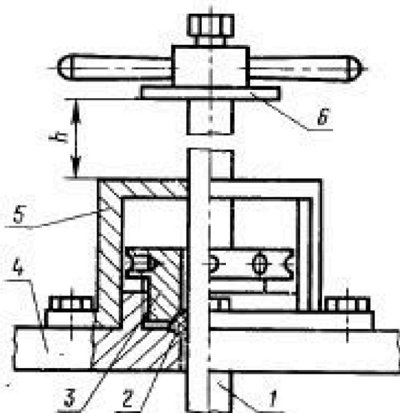
1 — штанга; 2 — набивка сальника; 3 — гайка; 4 — фланец; 5 — скоба; 6 — втулка
