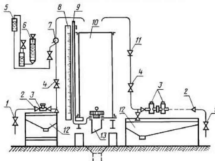
Принципиальная схема измерительной части поверочной установки для счетчиков с условным проходом от 15 до 25 мм
