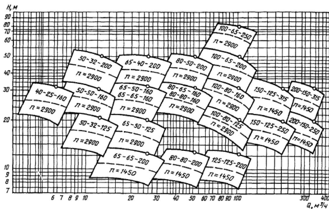
Рисунок 1 - Область работы центробежных консольных насосов.
