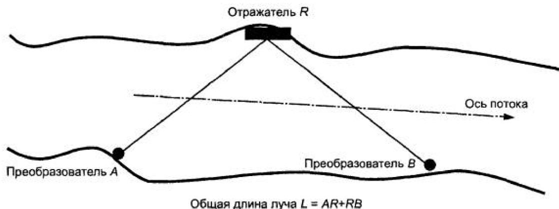
Рисунок 2 - Схема расположения преобразователей с отражением лучей
