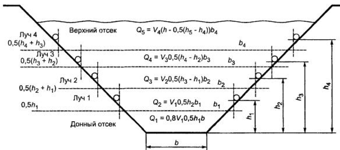
Рисунок 3 - Пример расчета расхода методом послойных сечений
