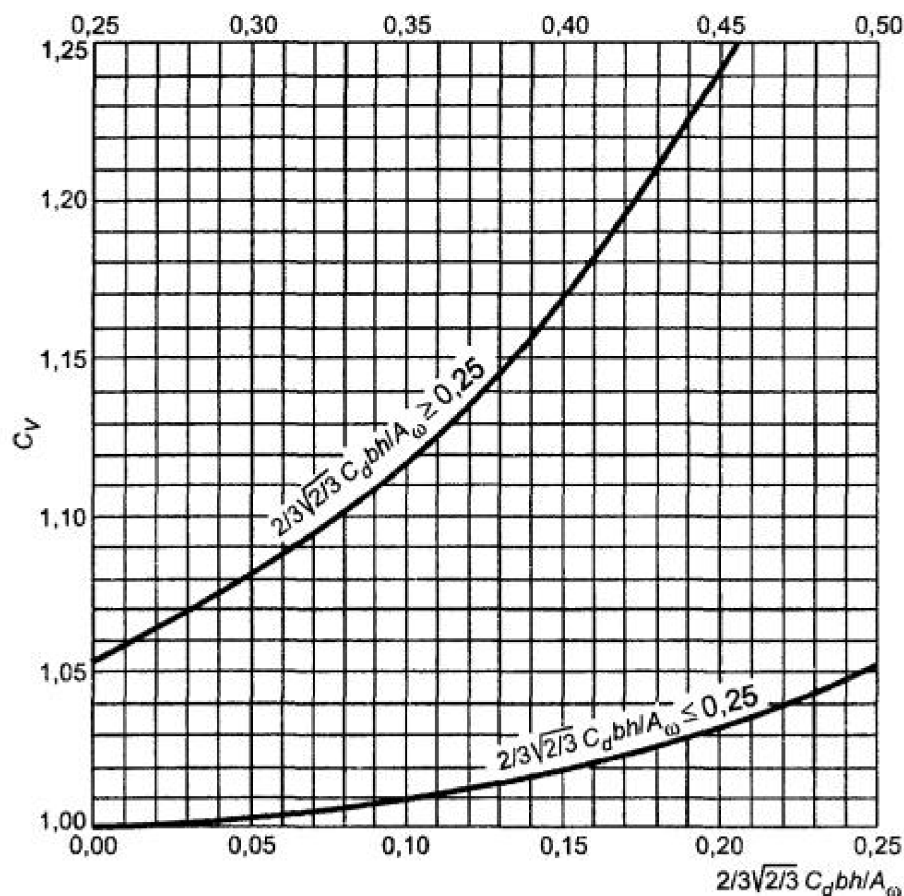
Рисунок 6 - Коэффициент скорости подхода потока C_v
