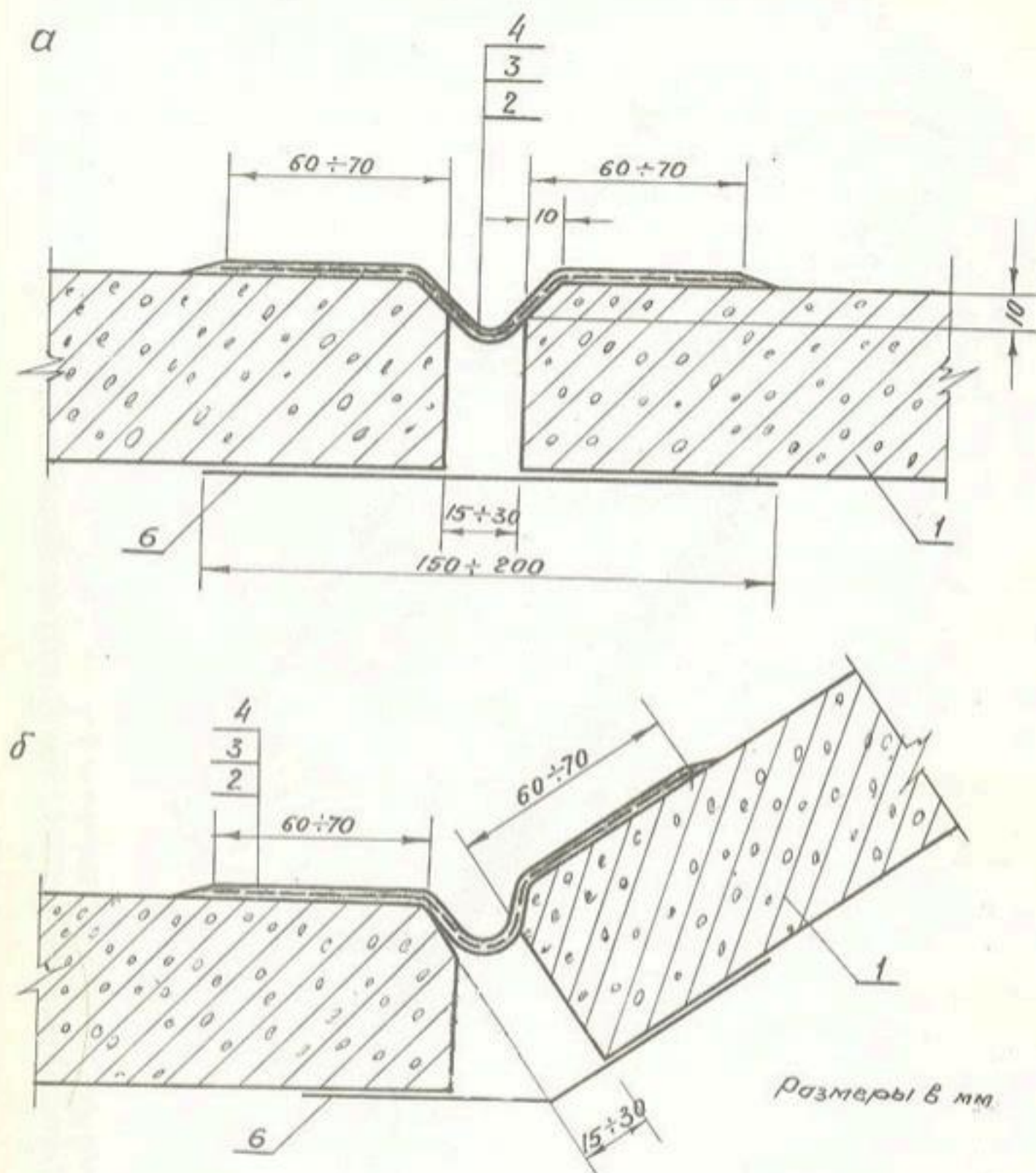
Рис.8. Герметизация стыка оклеечным стеклоэластиком: а - откосный и донный поперечные швы; б - донный продольный шов. 1-ж.б.плита; 2-приклеивающая эпоксидно-каучуковая мастика; 3-стеклоткань; 4-светотражающий эпоксидно-каучуковый состав; 5-подкладка (пергамин, толь или руберойд)
