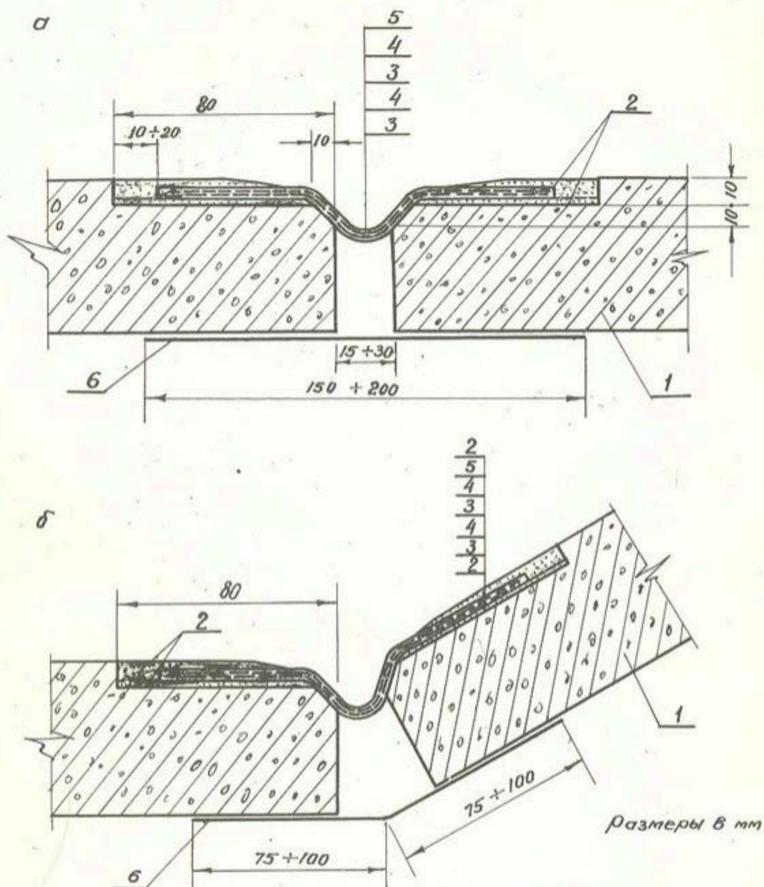
Рис.7. Герметизация стыка оклеечным стеклопластиком с пластрастровой подготовкой: а – откосный и донный поперечные швы; б – донный продольный шов. 1–ж.б. плита; 2–эпоксидно-песчаный пластрастр; 3–эпоксидный клей; 4–стеклоткань; 5–светоотражающий эпоксидный лак; 6–подкладка (пергамин, толь или руберойд)
