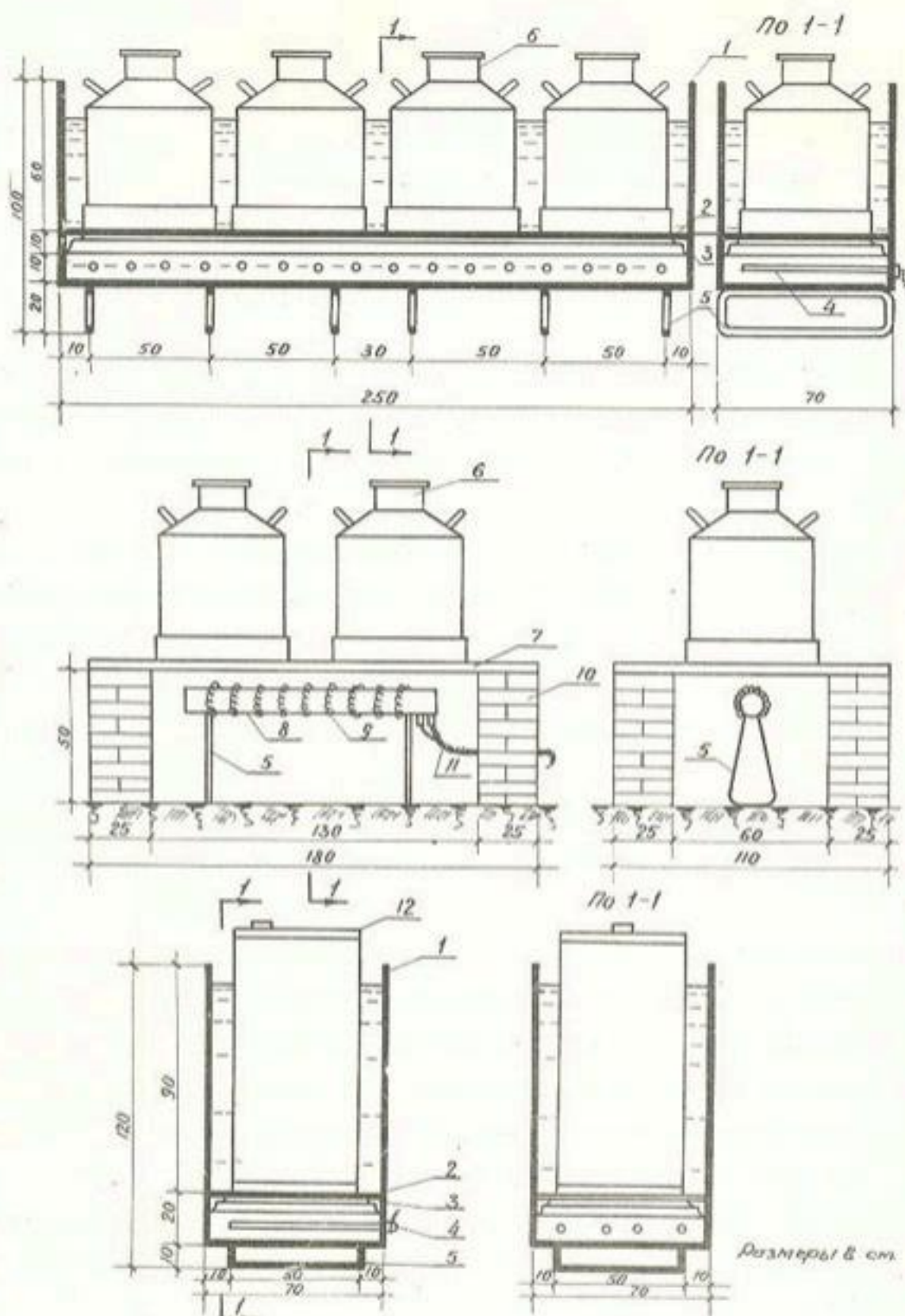
Рис. 27. Типы водяных и воздушных бань: 1—металлический корпус; 2—решетка; 3—опорный уголок 75x75; 4—теплоэлектронагреватель; 5—опора; 6—бидон со смолой; 7—асбоцементная плита толщиной 20 мм; 8—асбоцементная труба \phi=100 мм; 9—спираль; 10—кирпичная стенка; 11—кабель; 12—барабан со смолой
