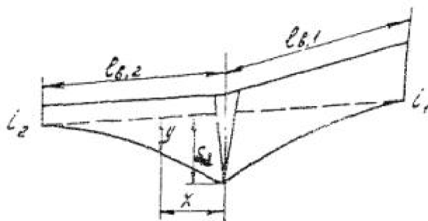
Черт. 10.1. Расчетная схема головных дрен
