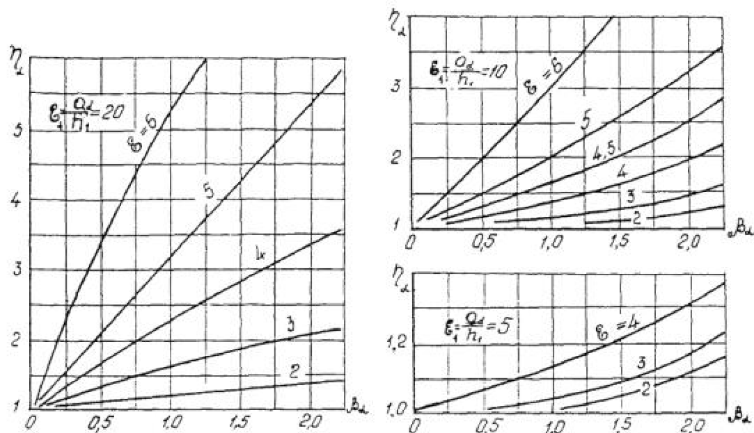
Черт. 8.11. Графики для определения коэффициента \eta_a
