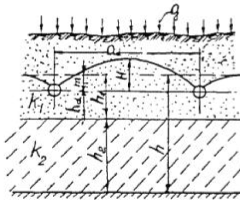
Черт. 8.2. Расчетная схема двухслойной толщ с дренажем в верхнем слое
