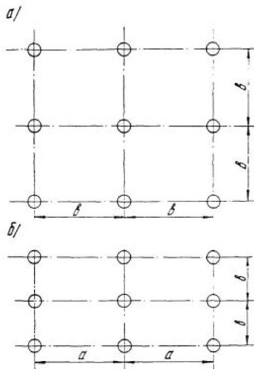
Черт. 12.1. Схемы размещения в плане систематического вертикального дренажа с равномерным (а) и неравномерным (б) шагом сетки
