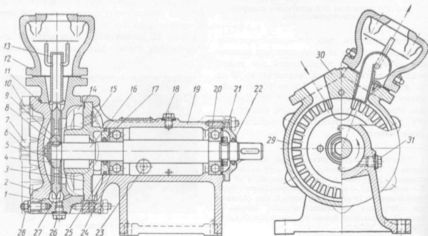
Вихревой насос типа В.
