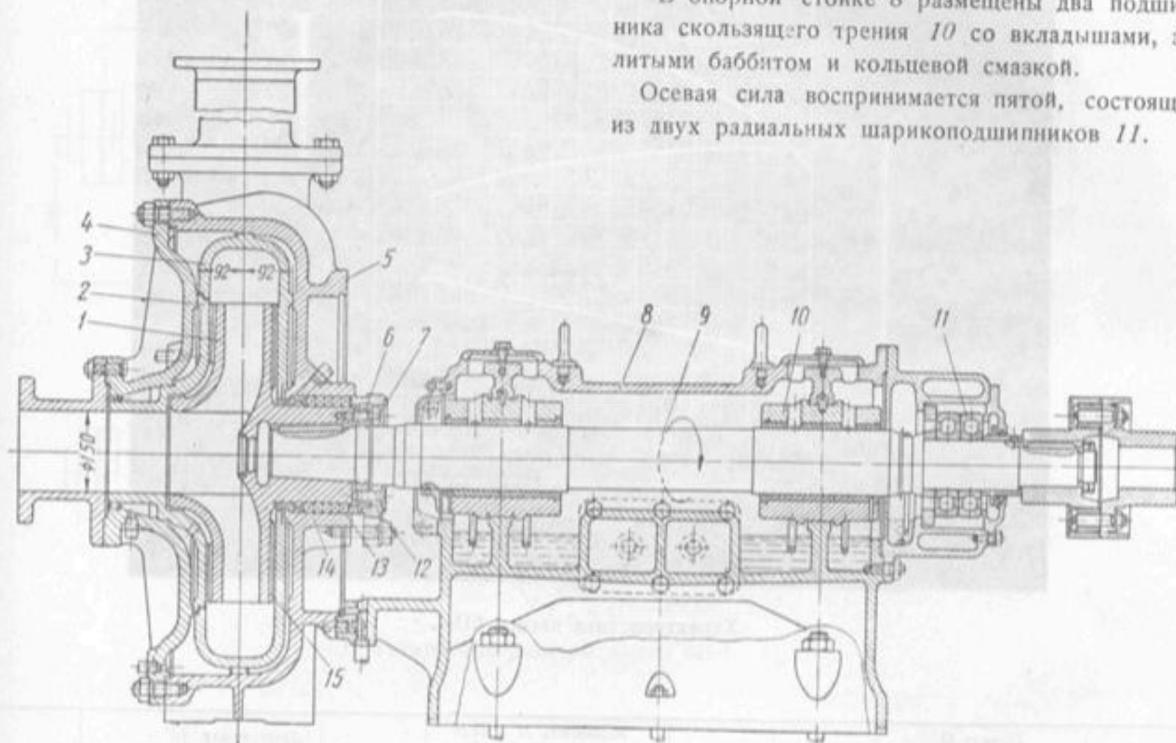
Насос 6П-7.
