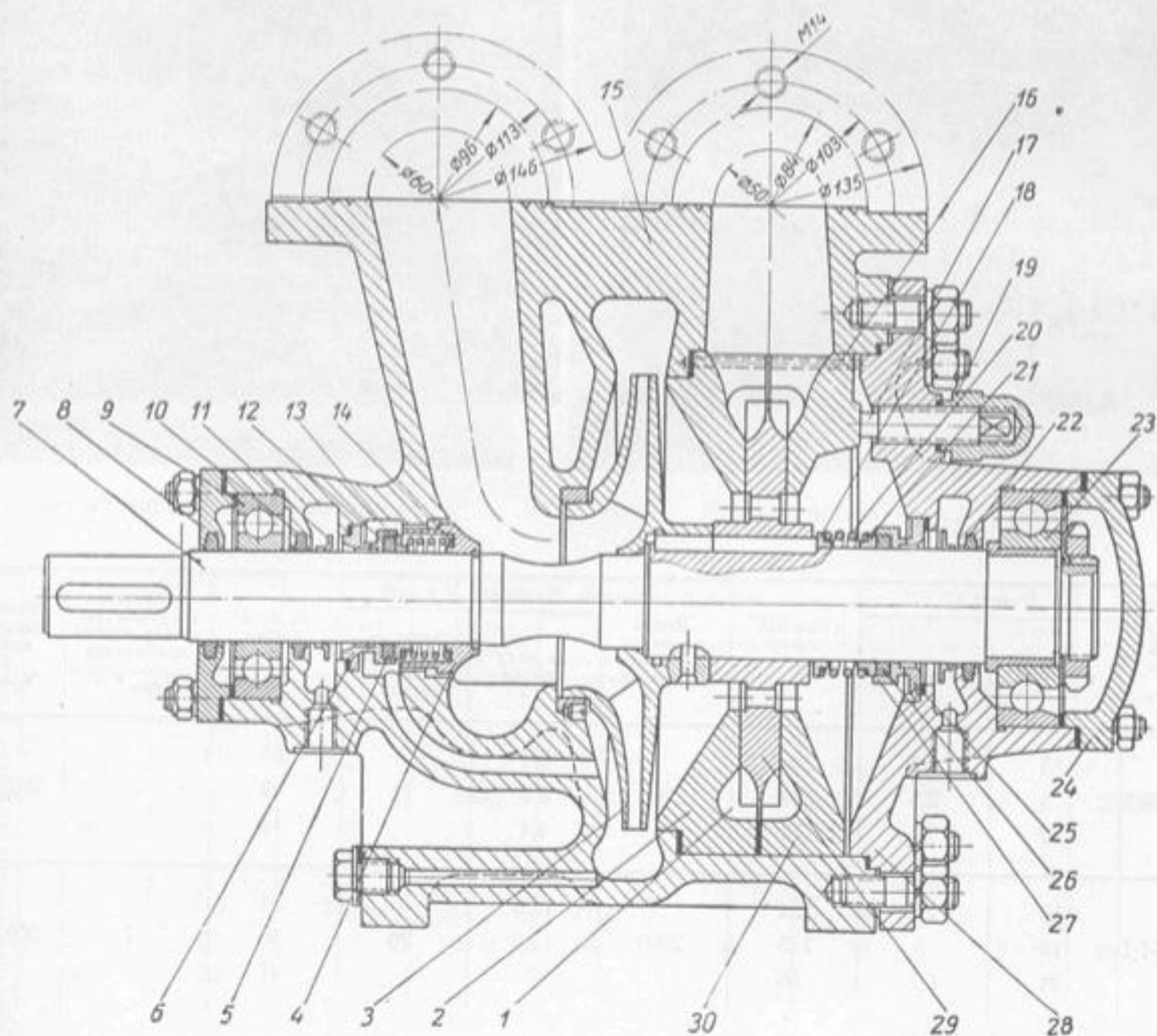
Насос 2,5ЦВ-1,5.
