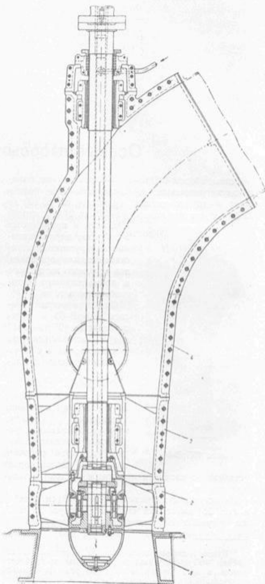
Насос 40ПрВ-60.
