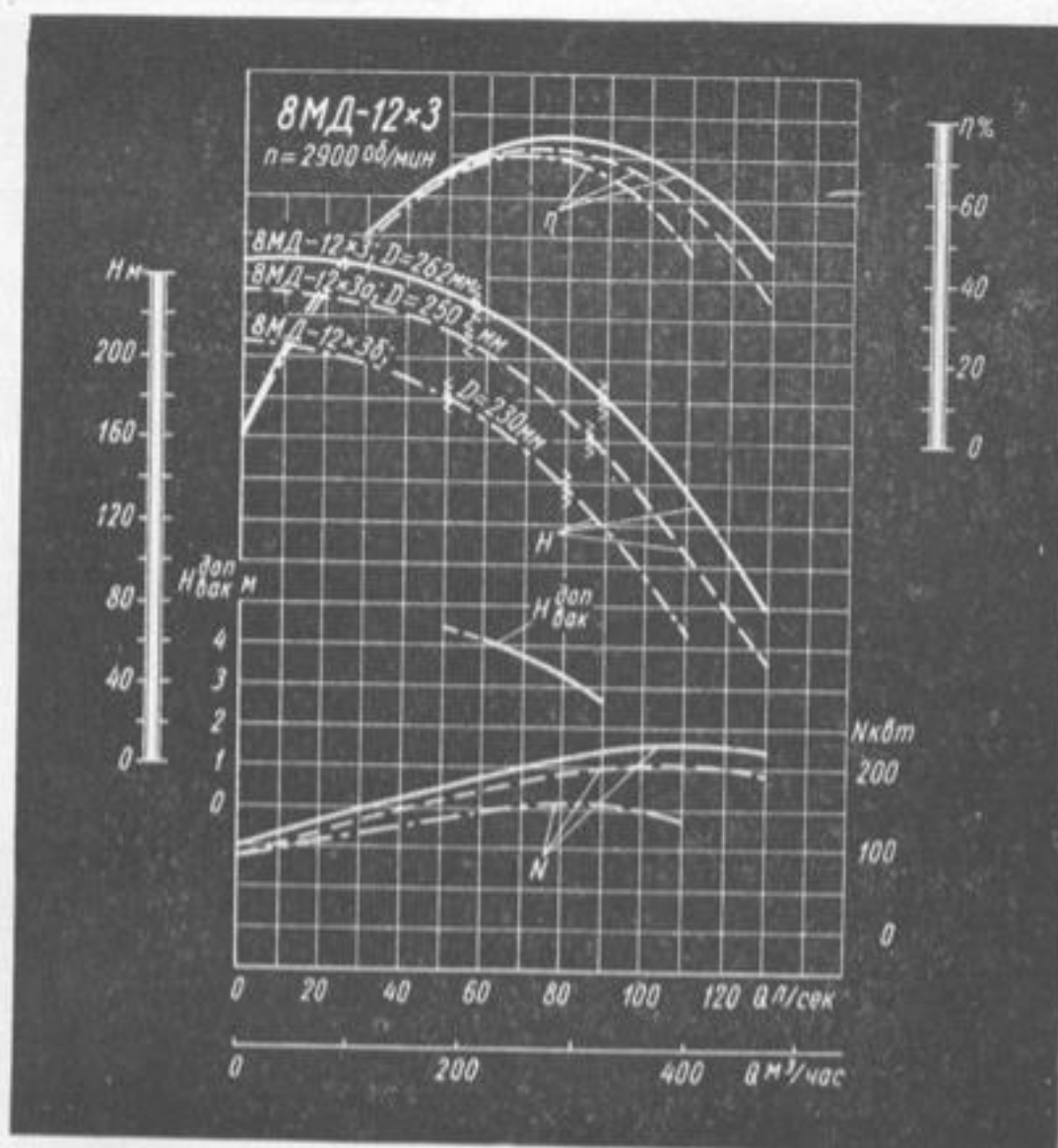
Характеристика насоса 8МД-12×3.
