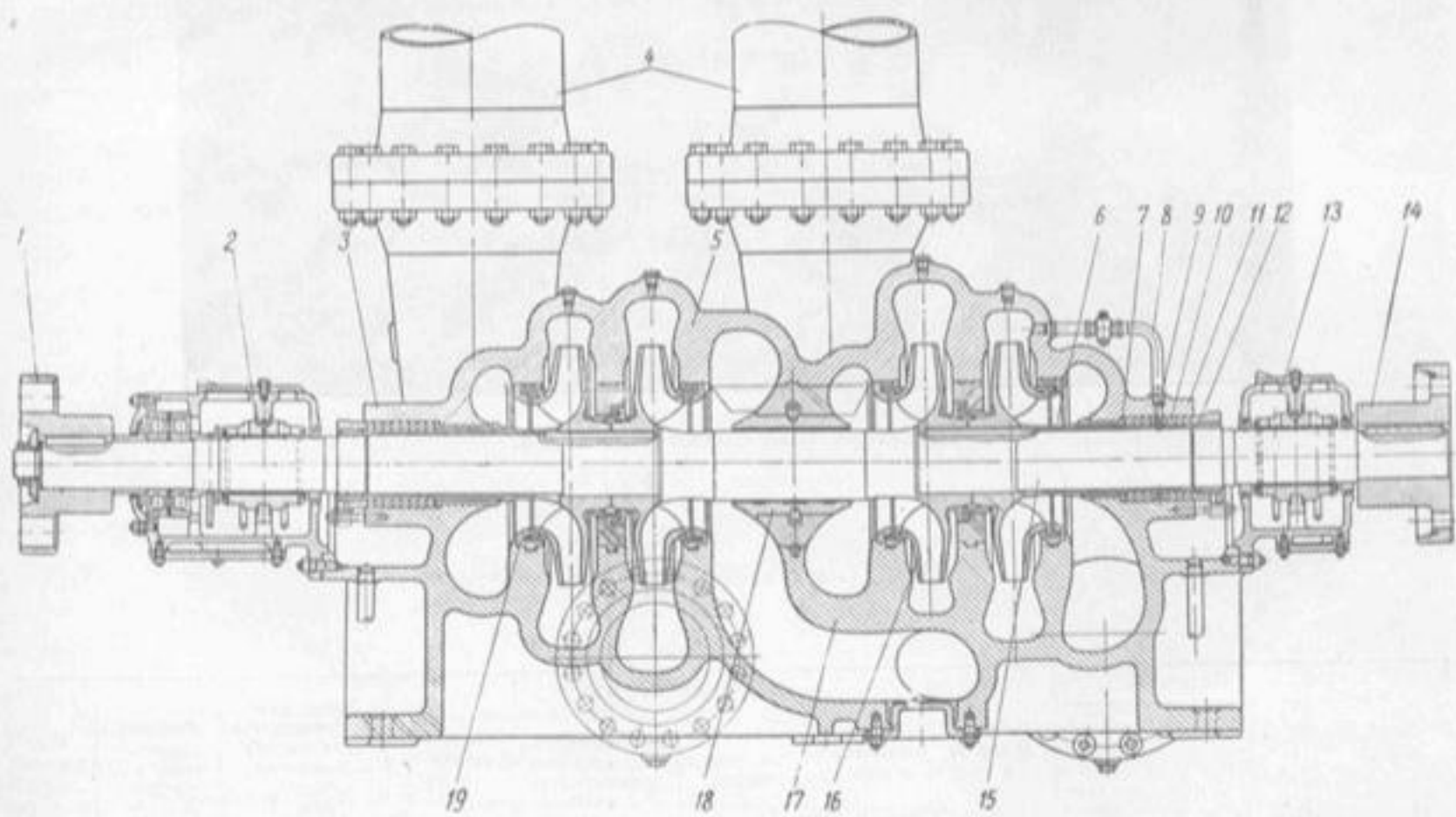
Насос 14М-12 × 4.
