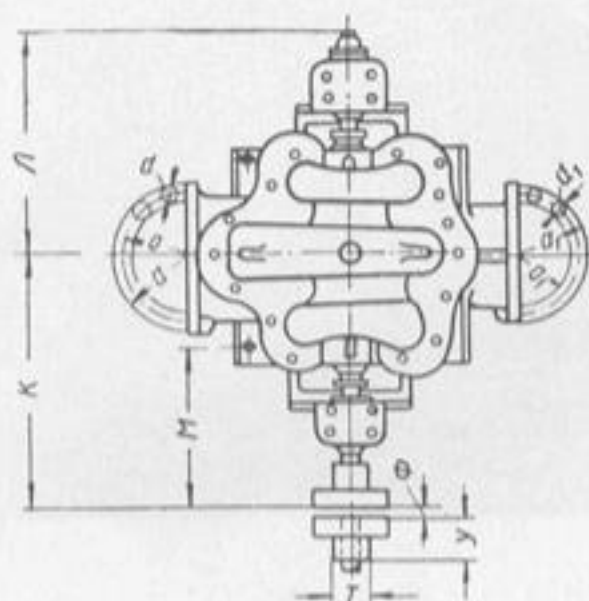
Габаритные размеры насосов типов НДв.
