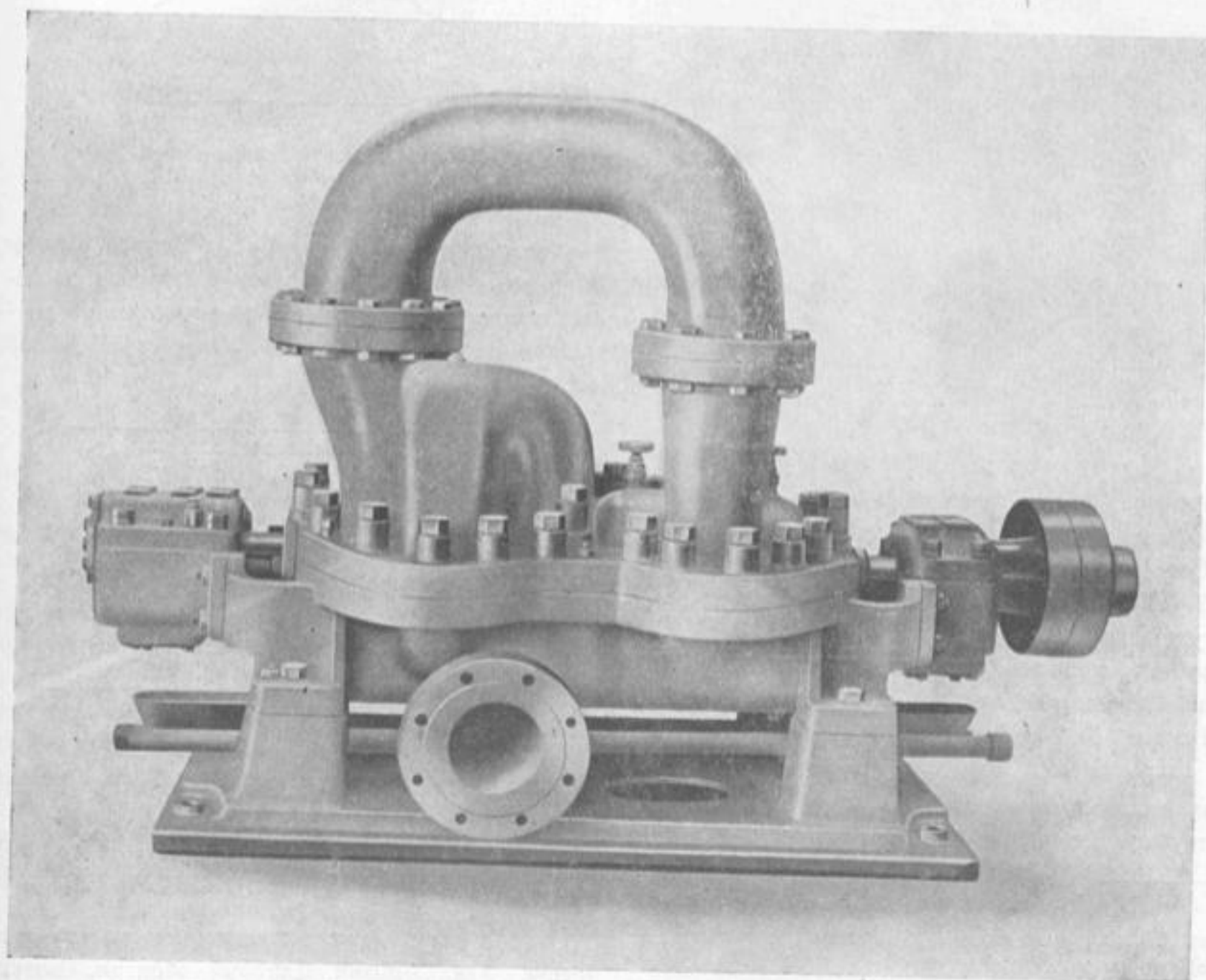
Насос 8МД-12×3.
