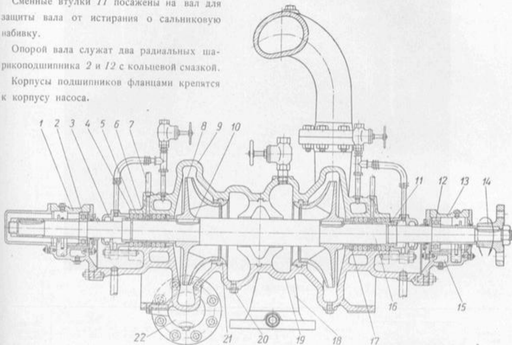
Насос 5Кс-5 × 2.
