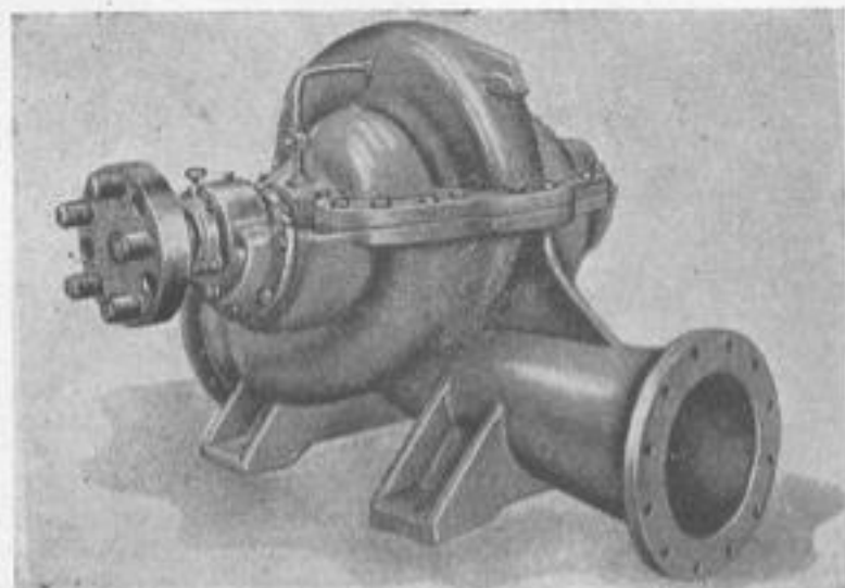
Насос 8НДв.
