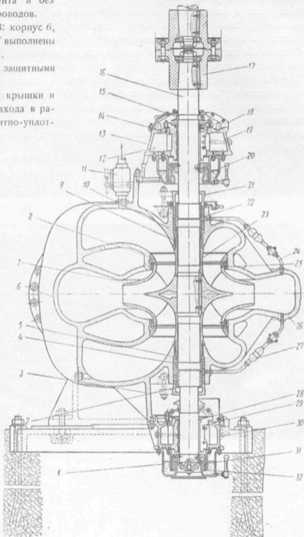
Насос 24НДсВ.
