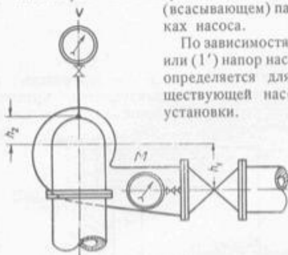
Фиг. 2. Схема установки насоса с манометром и вакуумметром.
