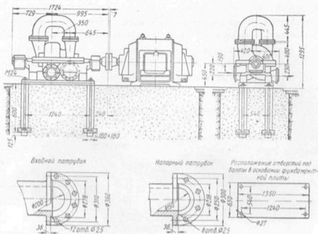
Габаритные размеры насоса 8МД-12×3.
