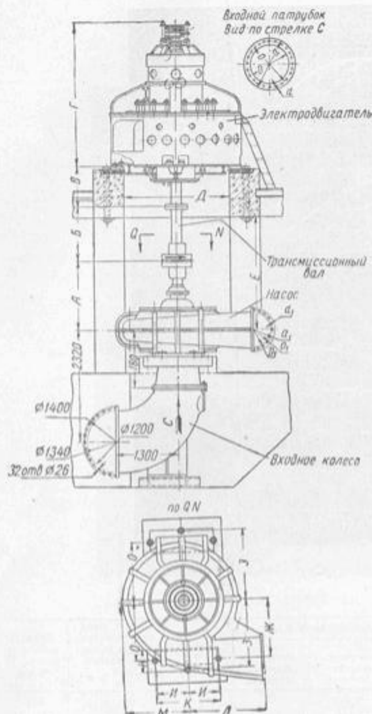
Установочный чертеж насосов типа В.
