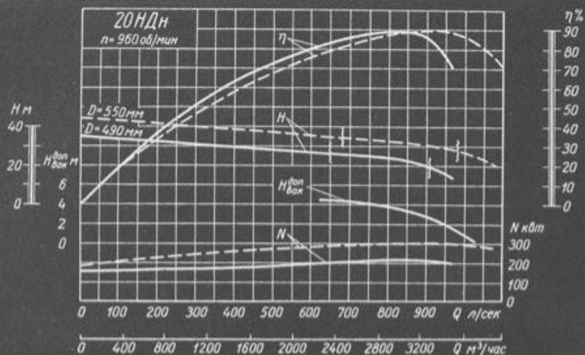
Характеристика насоса 20НДн ( n = 960 \text{ об/мин} ).
