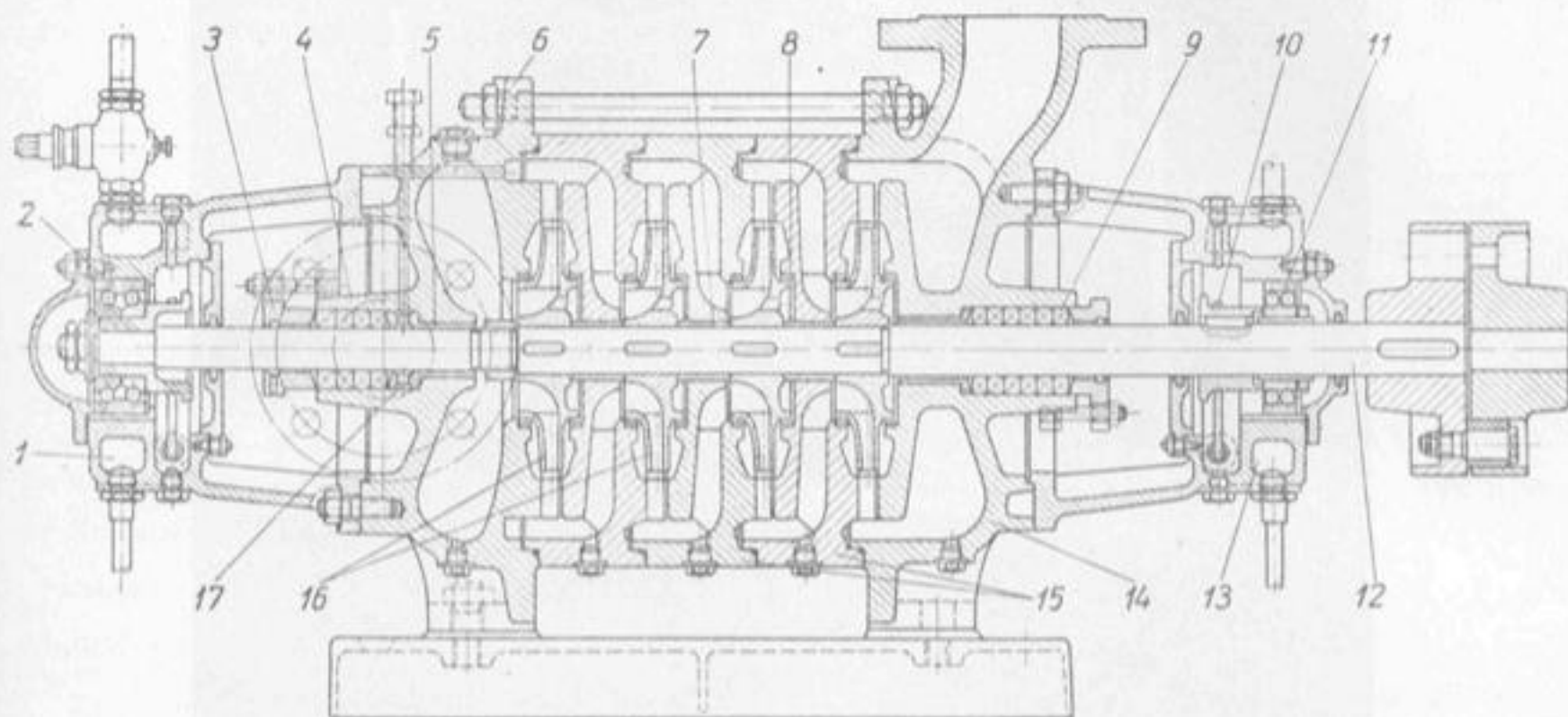
Насос 3НМГ × 4.
