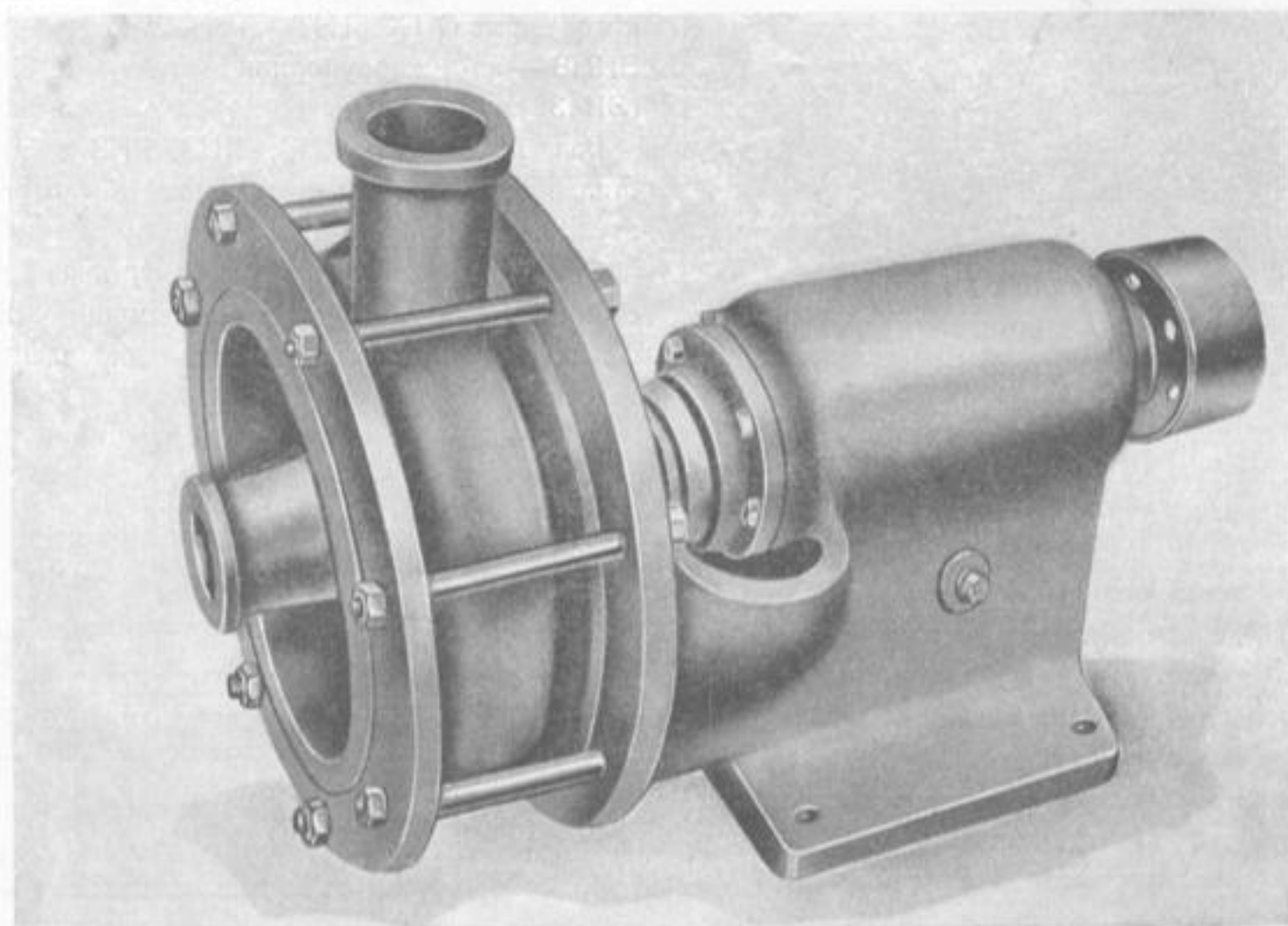
Насос КНЗ.
