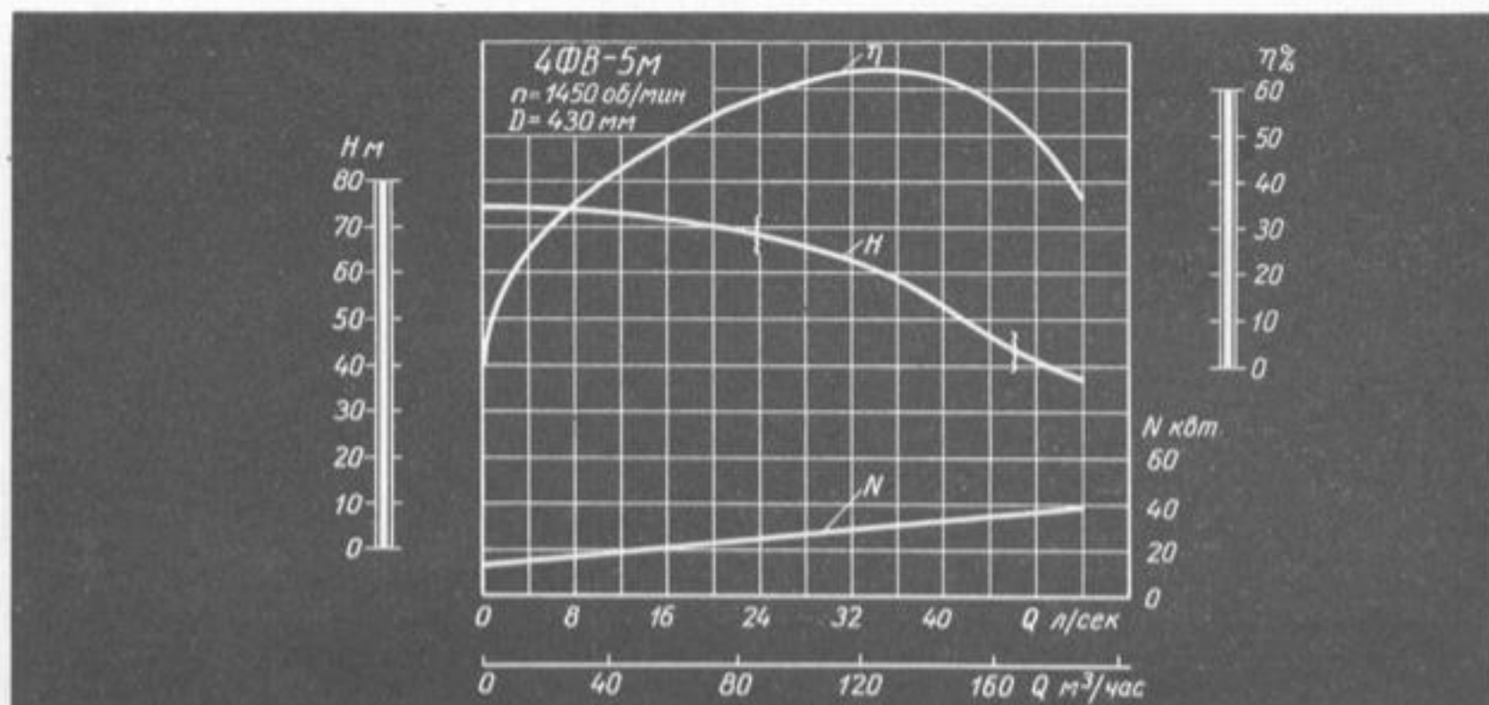
Характеристика насоса 4ФВ-5м.
