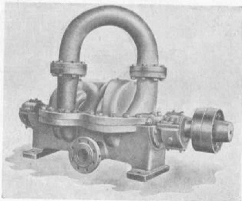
Насос 3В-200 × 4.
