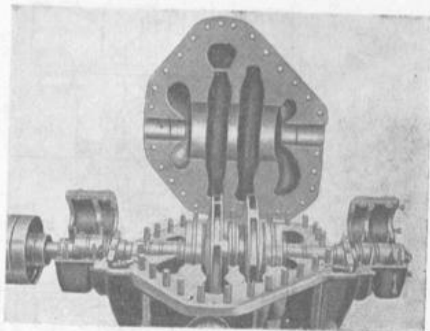
Насос 10HMK \times 2 с приподнятой крышкой.
