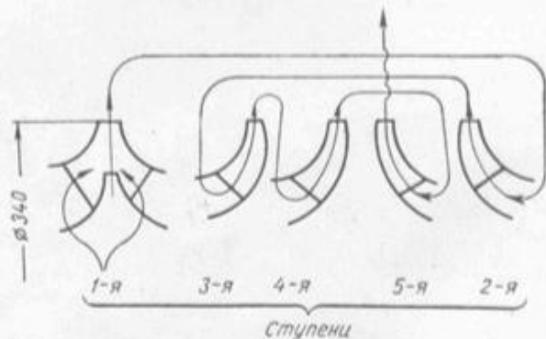
Схема движения потока в пятиступенчатом насосе типа МД.
