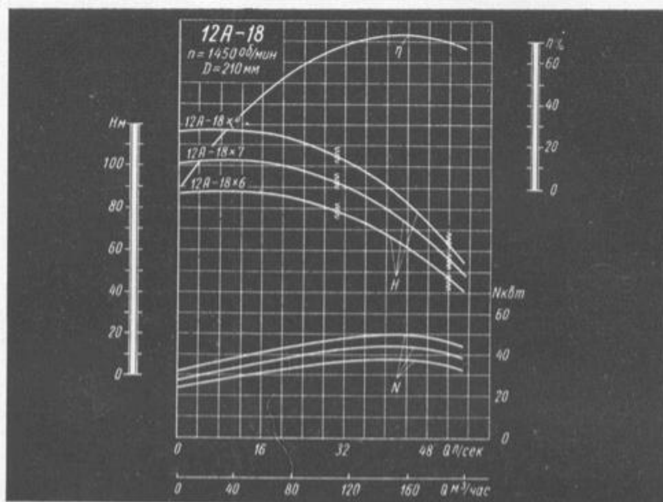
Характеристика насосов 12A-18×6, 12A-18×7 и 12A-18×8.
