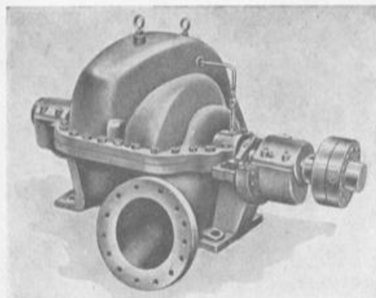
Насос 10НМК×2.
