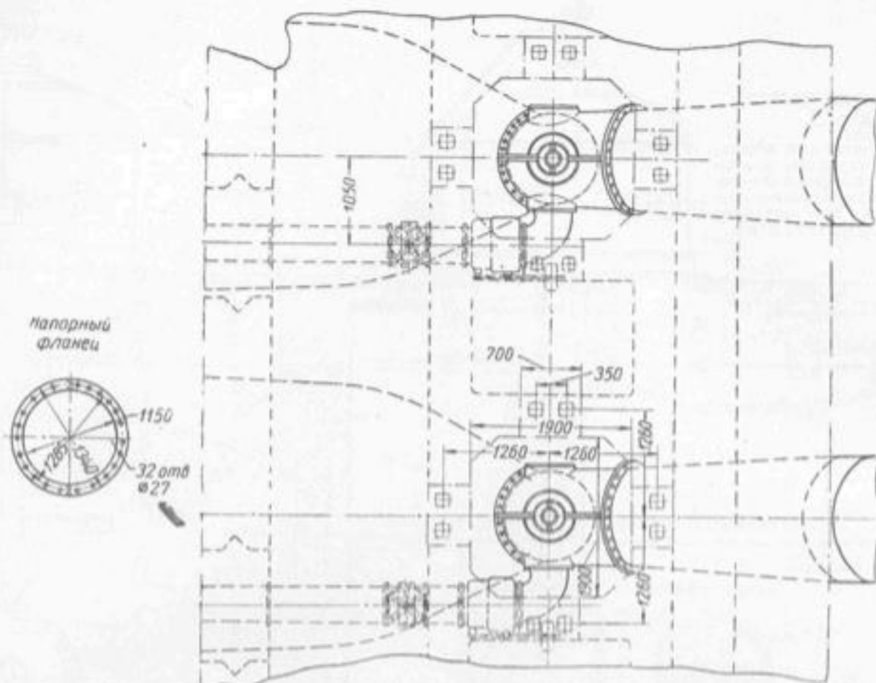
Схема установки насоса 40PrB-50x2. Вид сверху.
