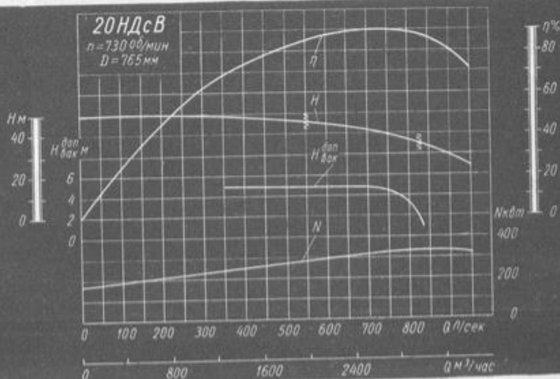
Характеристика насоса 20НДсВ ( n = 730 \text{ об/мин} ).
