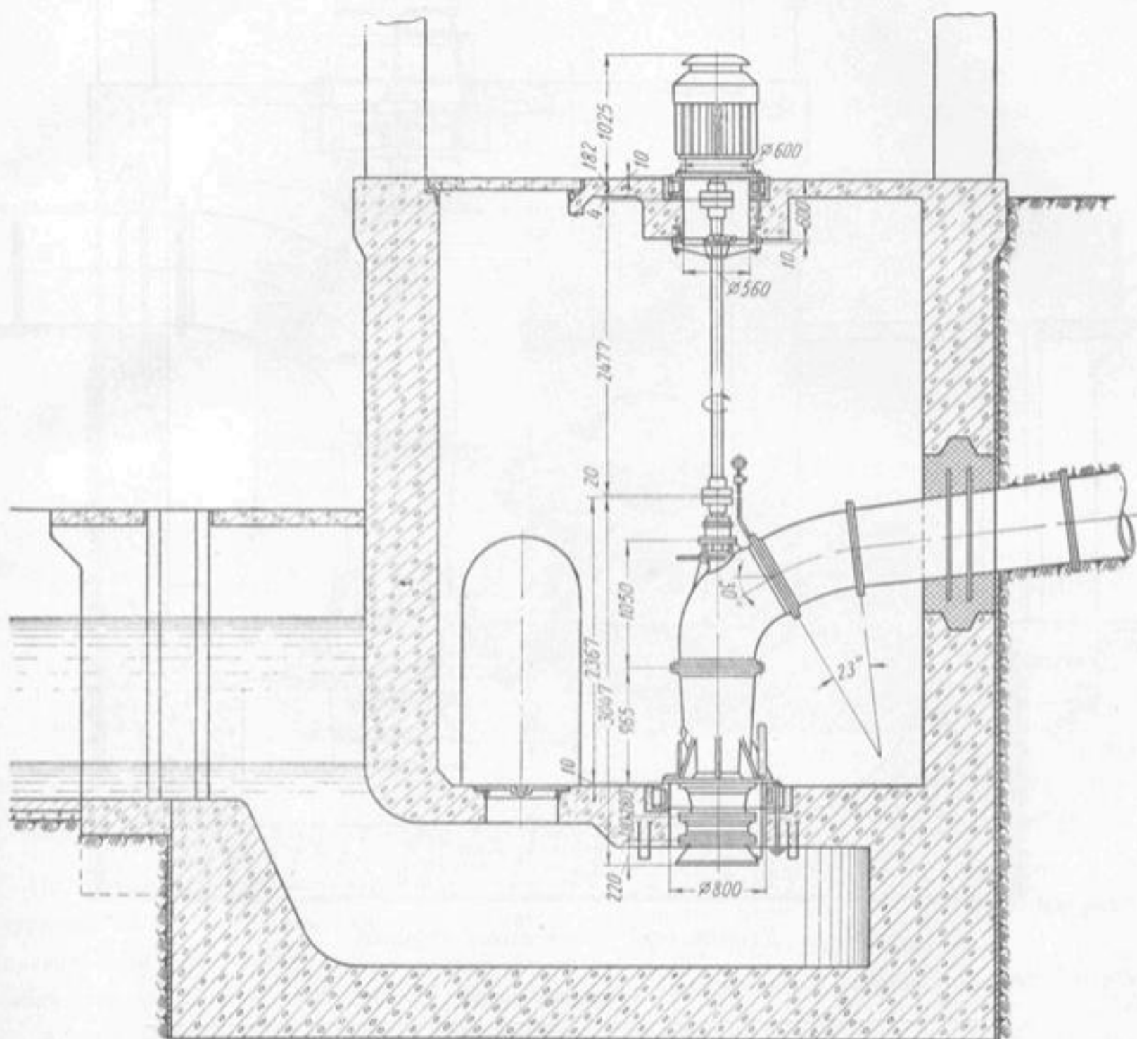
Установочный чертеж насоса 20PrB-60.
