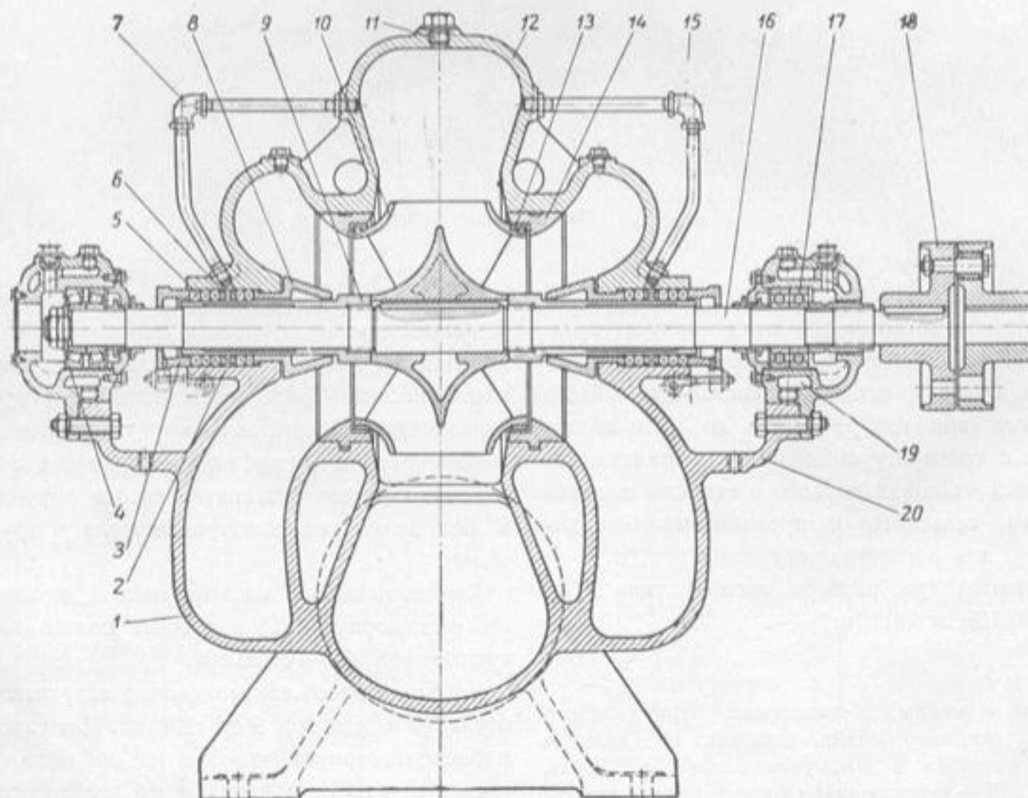
Насос 16НДи.
