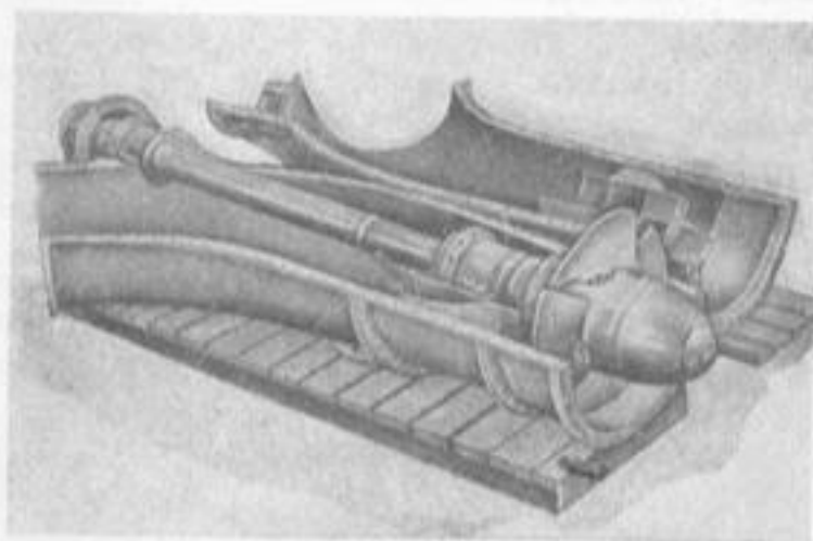
Насос 40ПрВ-60 с откинутой крышкой.
