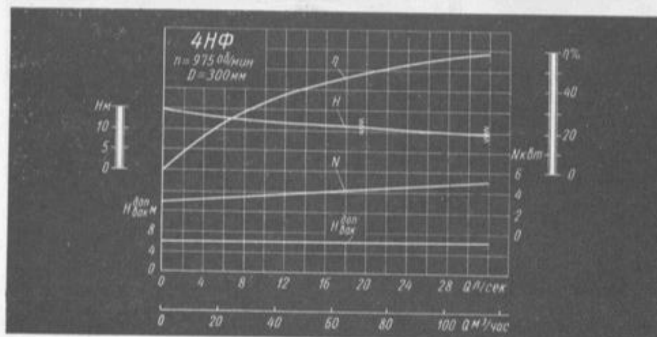
Характеристика насосов 4НФ ( n = 975 \text{ об/мин} ).
