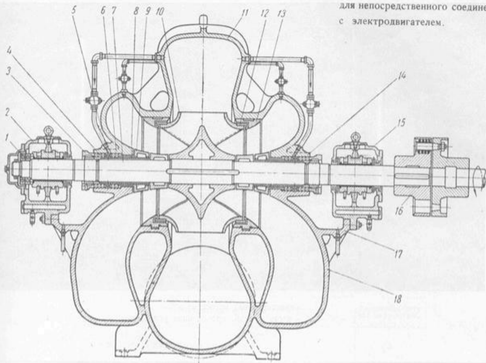
Насос 48Д-22.
