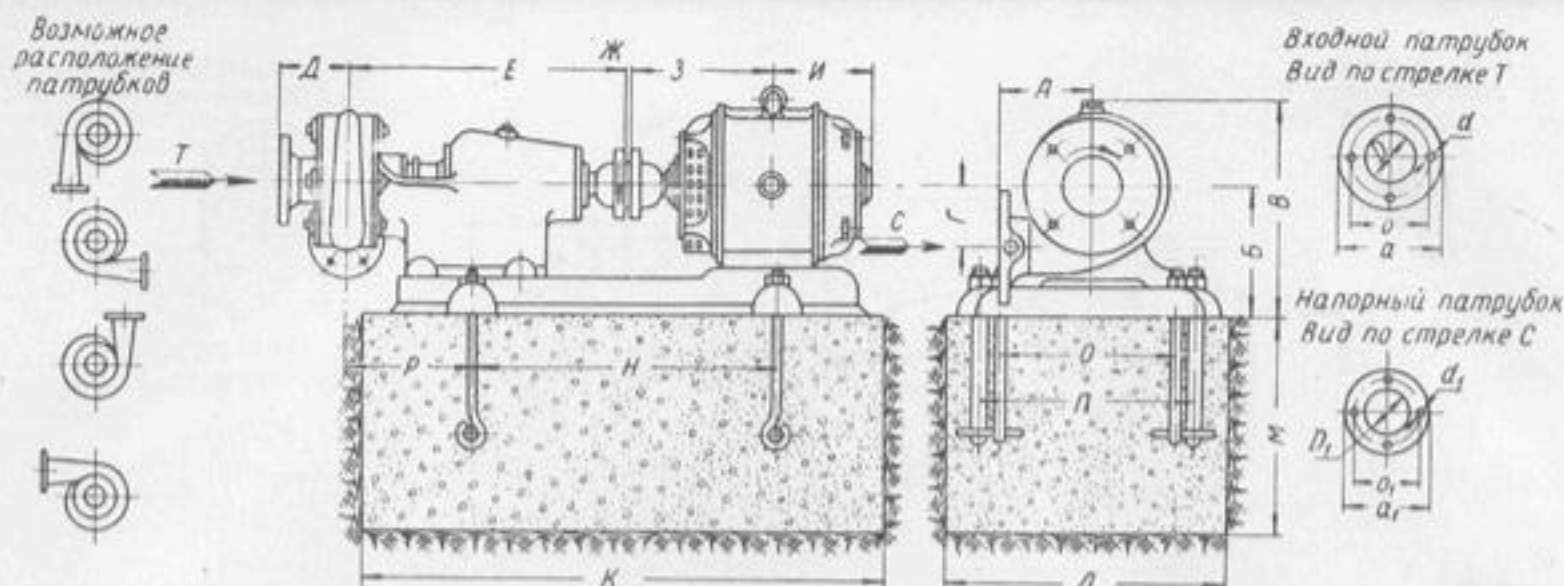
Габаритные размеры насосов типа К на опорных стойках 0-1, 0-2, 0-2а, 0-3, 0-3а с электродвигателем на общей фундаментной плите.
