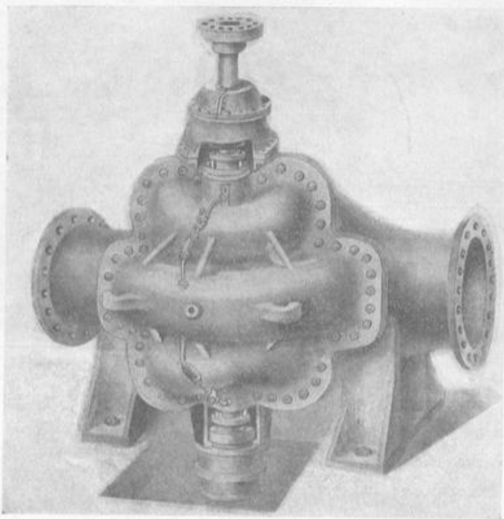
Насос 24НДсВ.
