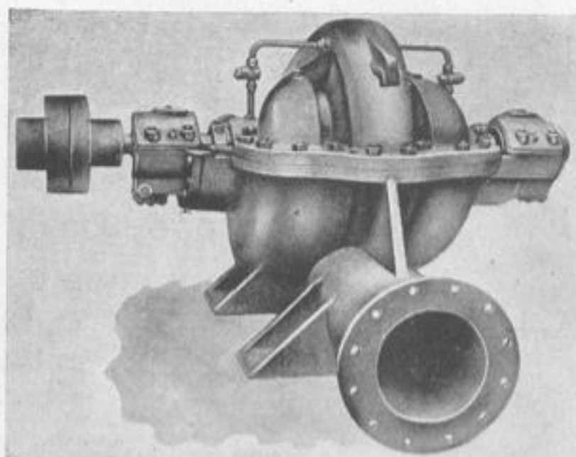
Насос 20НДс.
