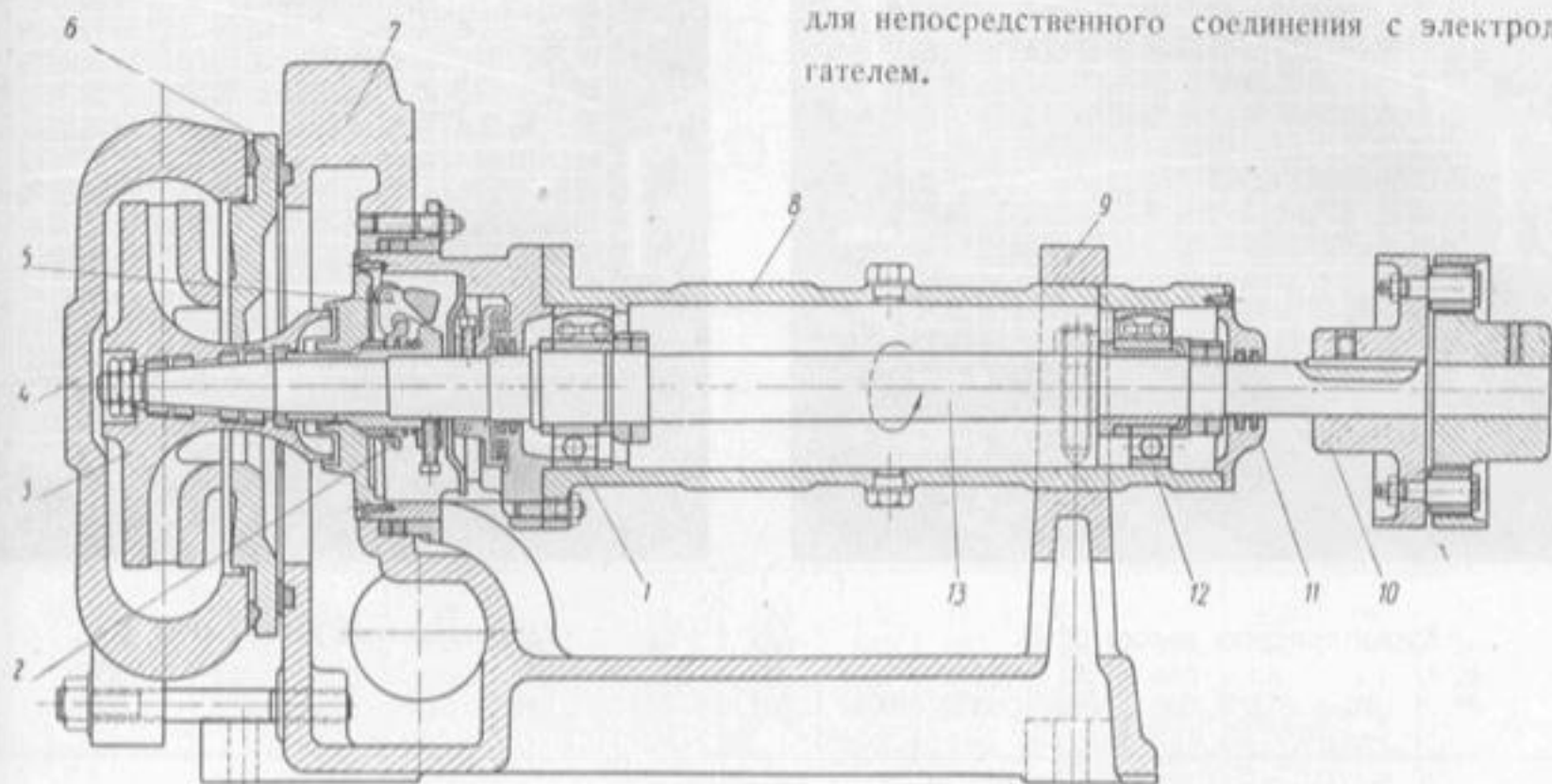
Насос 6НП.
