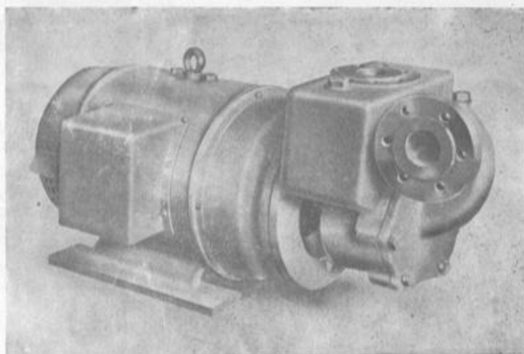
Насос ЭСН-1/1.
