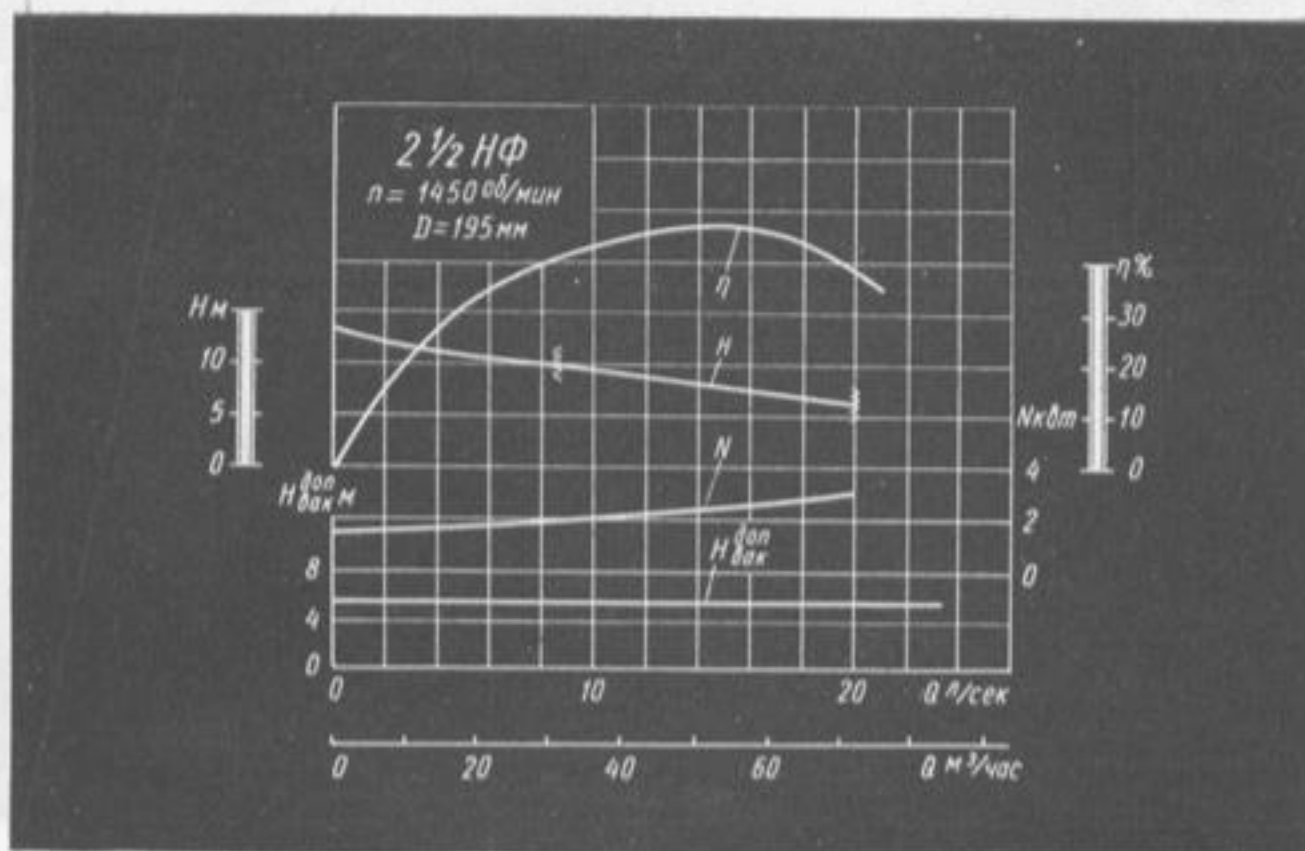
Характеристика насосов 2 \frac{1}{2} HF ( n = 1450 об/мин).
