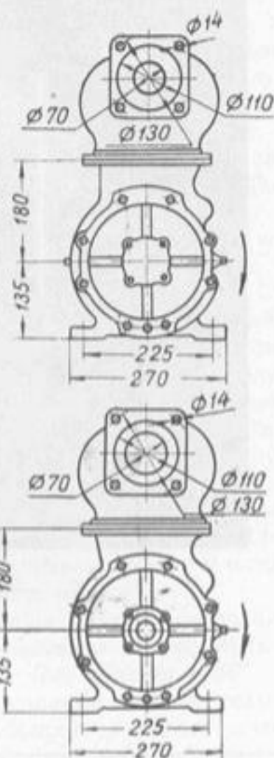
Насос левого вращения
