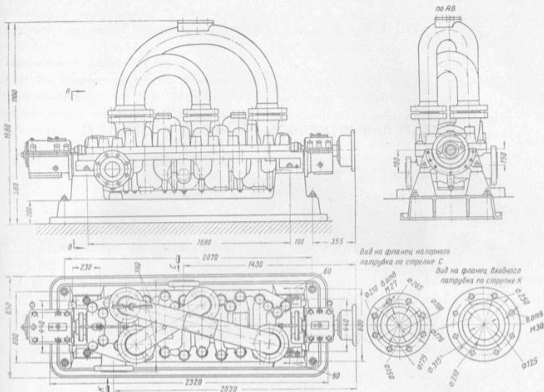
Габаритные размеры насоса 5М-7 × 8.
