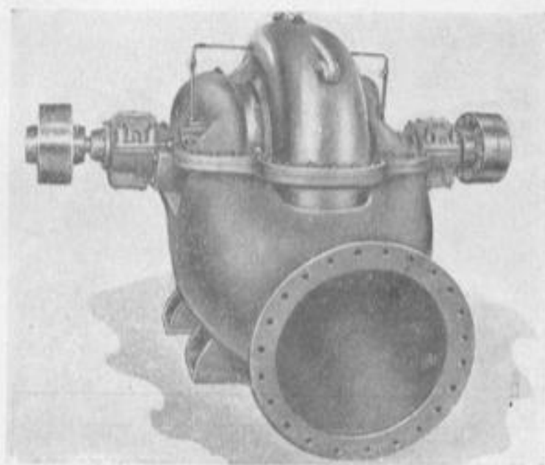
Насос 32Д-19.
