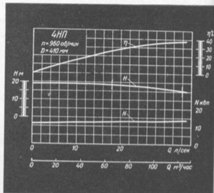
Характеристика насоса 4НП.
