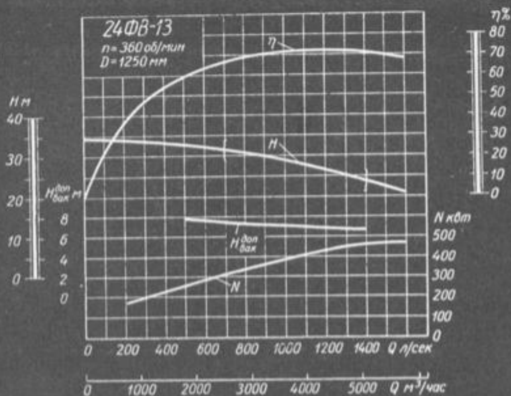
Характеристика насоса 24ФВ-13.
