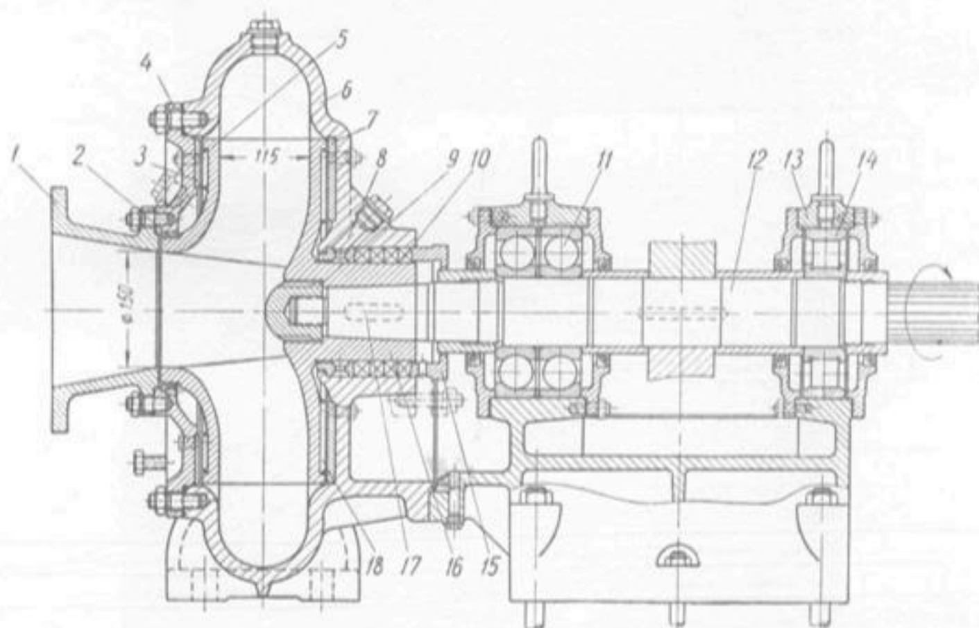
Землесос 6Р-11.
