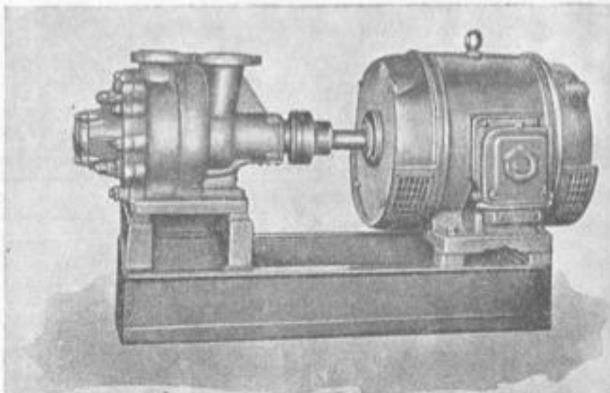
Насос 2,5ЦВ-1,5 на общей раме с электродвигателем.
