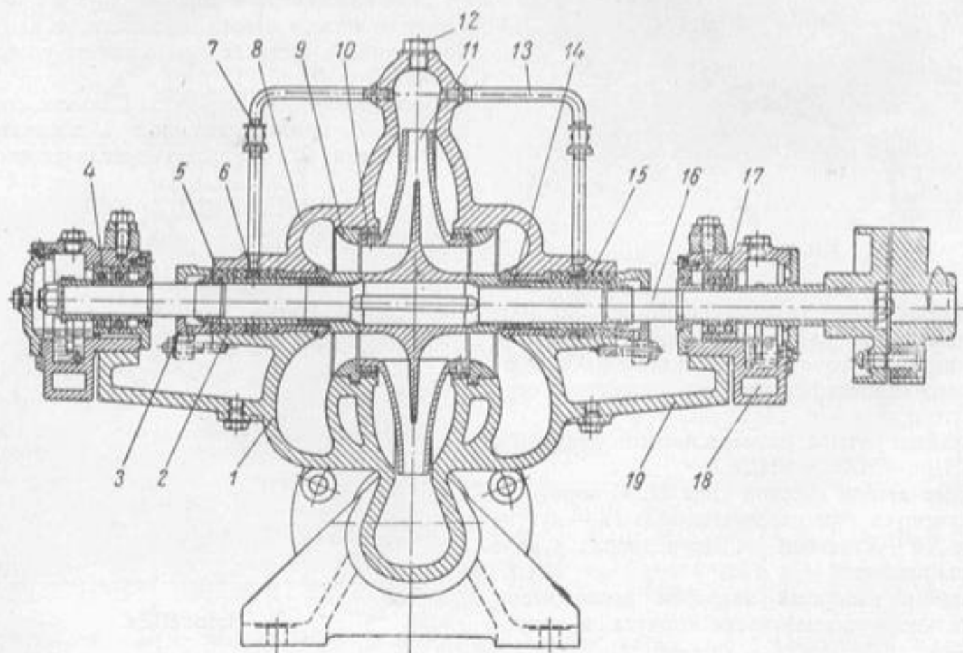
Насос 6НДв.
