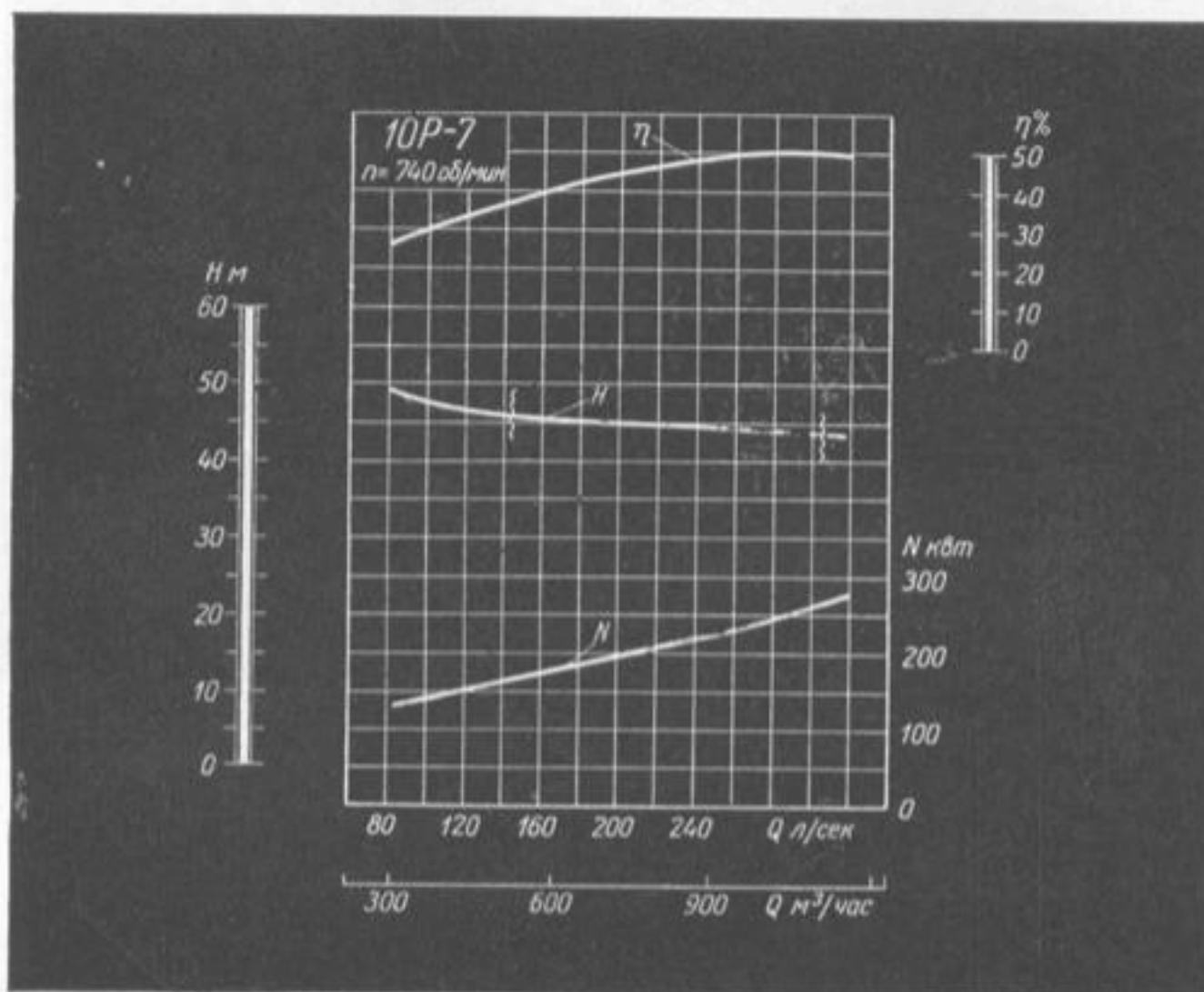
Характеристика землесоса 10Р-7.
