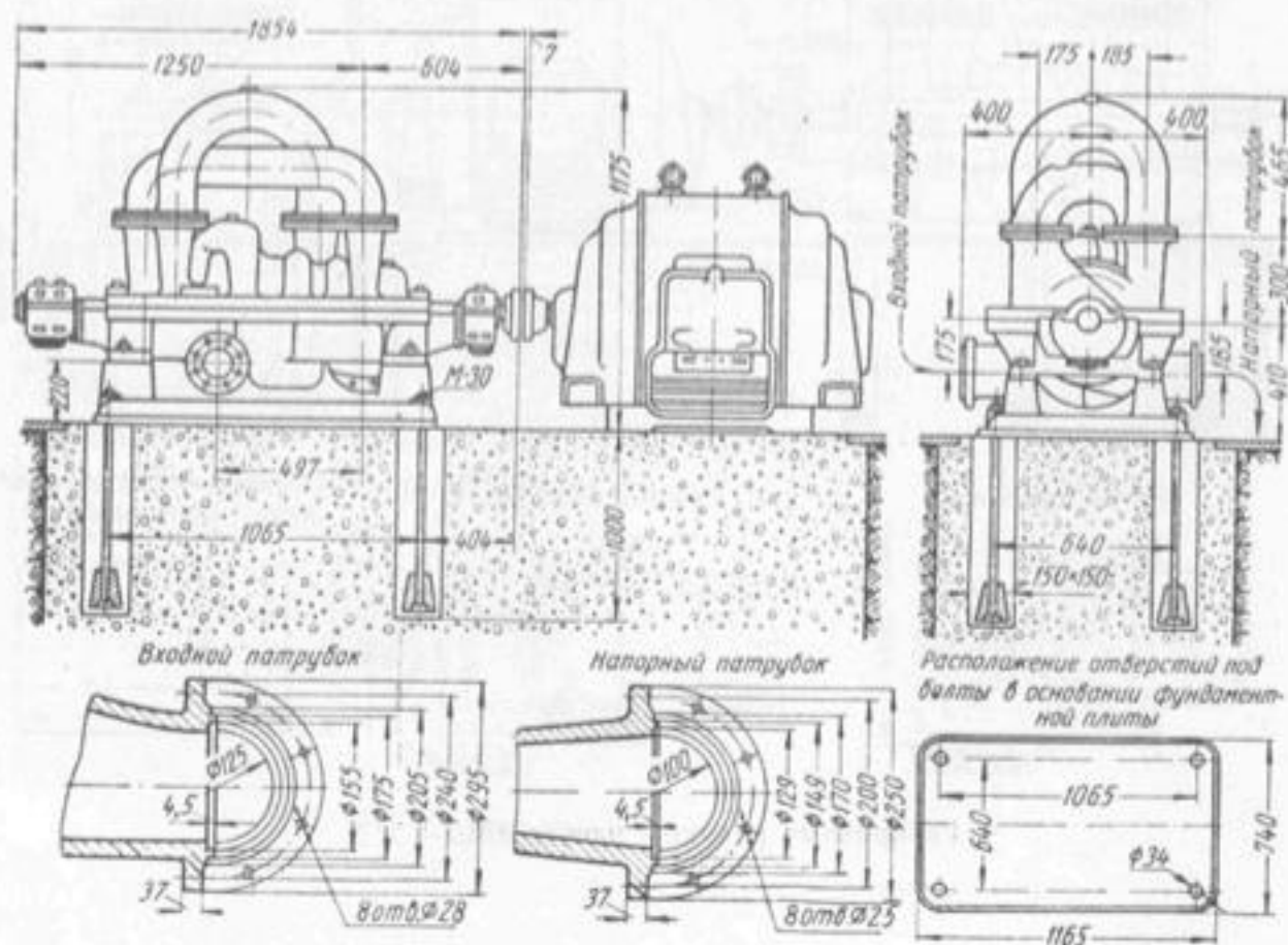
Габаритные размеры насоса 5МД-7 \times 5.
