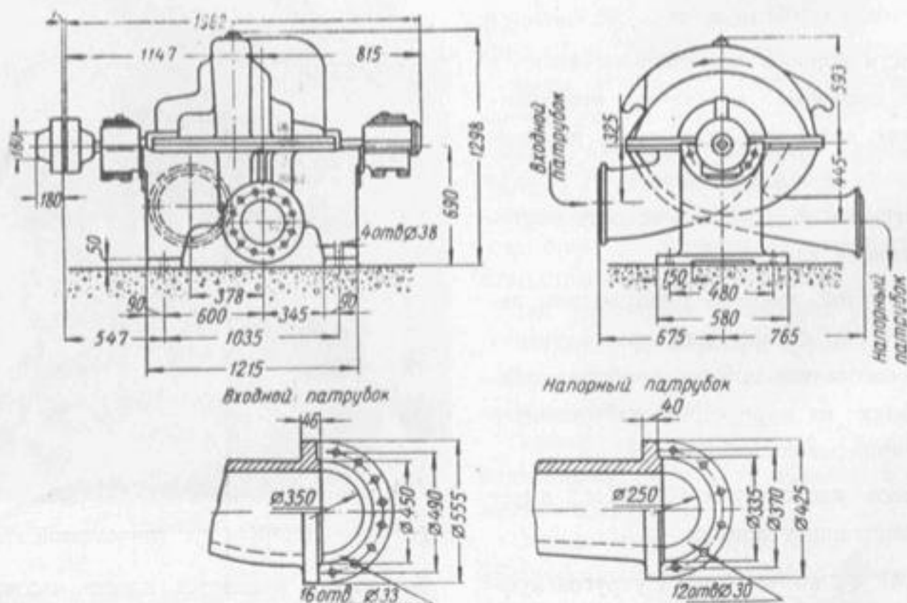
Габаритные размеры насоса 10НМК \times 2.
