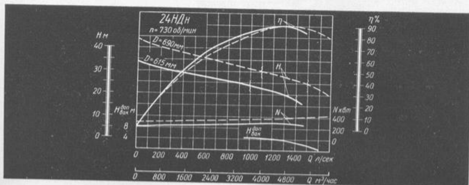
Характеристика насоса 24НДн (n = 730 об/мин).
