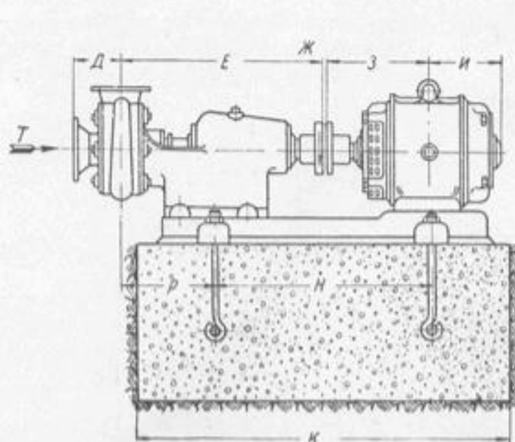
Габаритные размеры насосов типа К на опорных стойках 0-3 и 0-3а с электродвигателем на общей фундаментной плите.
