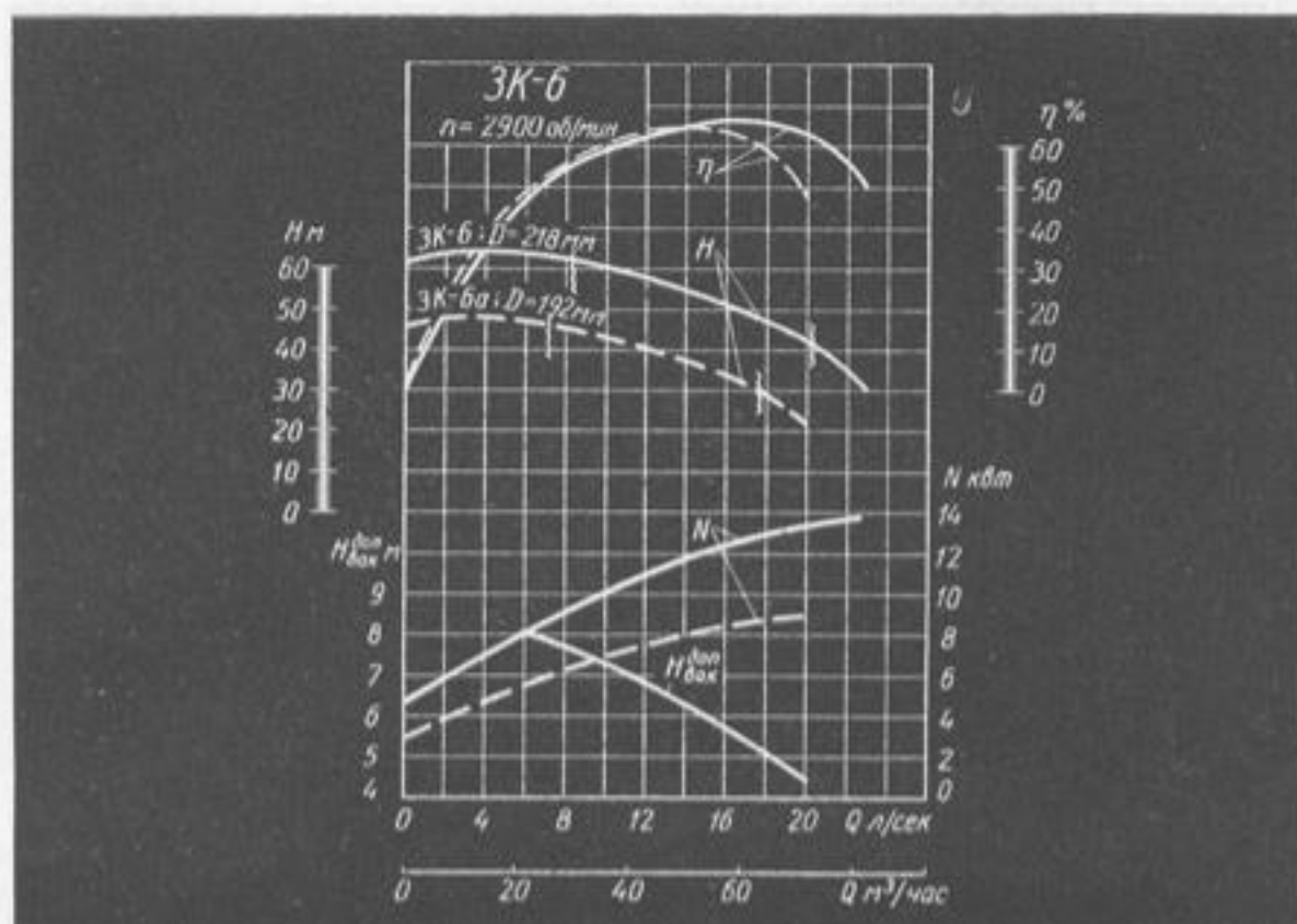
Характеристика насоса 3K-6.
