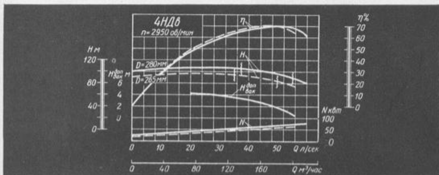
Характеристика насоса 4НДв ( n = 2950 \text{ об/мин} ).
