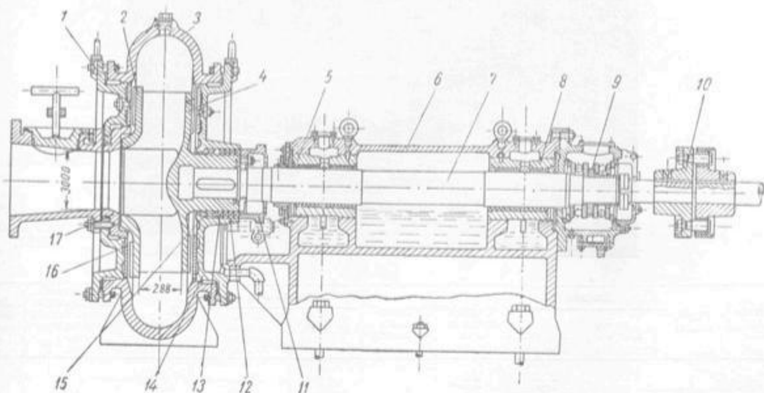
Насос 12НЗ36.
