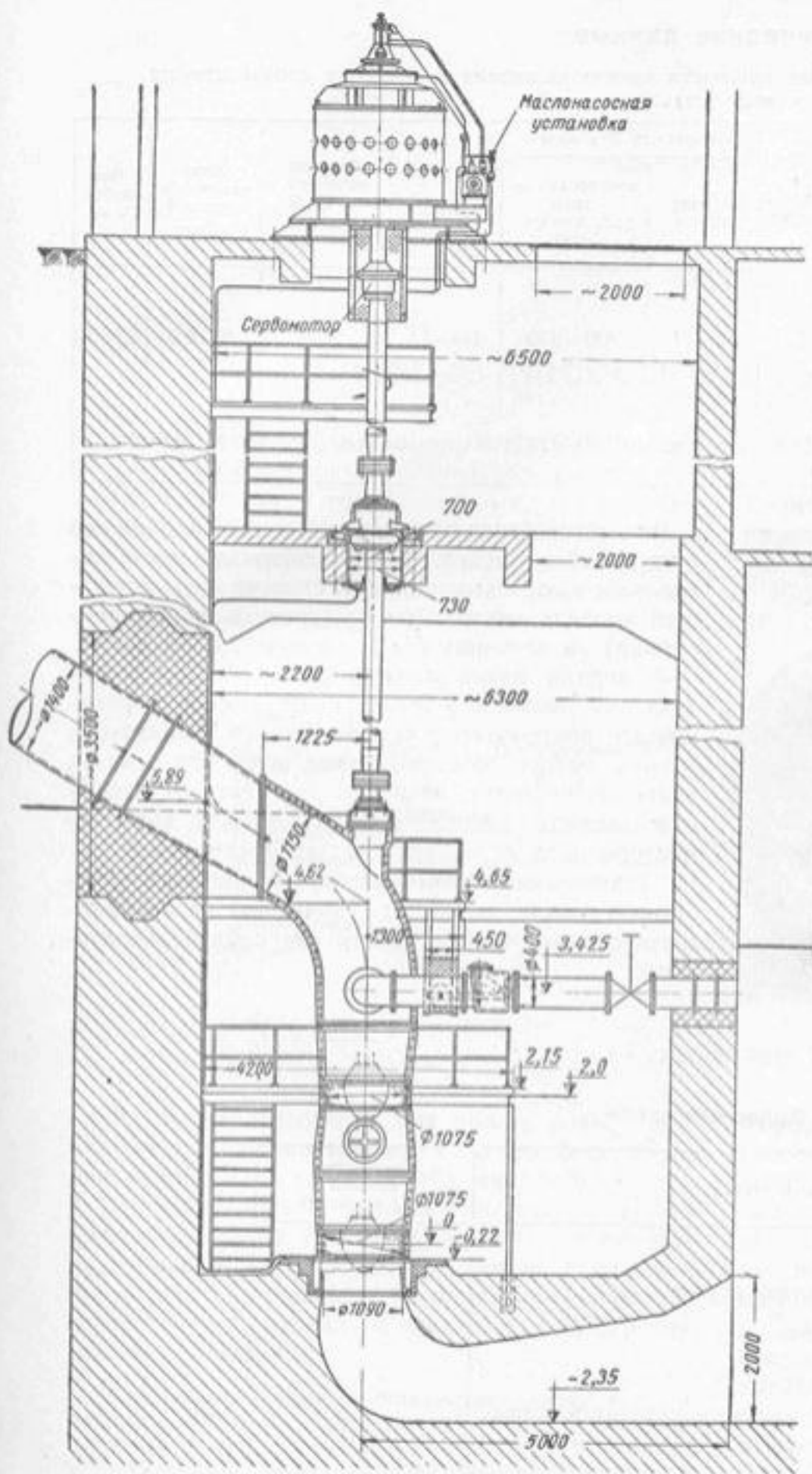
Схема установки насоса 48ПрВ-58 \times 2.
