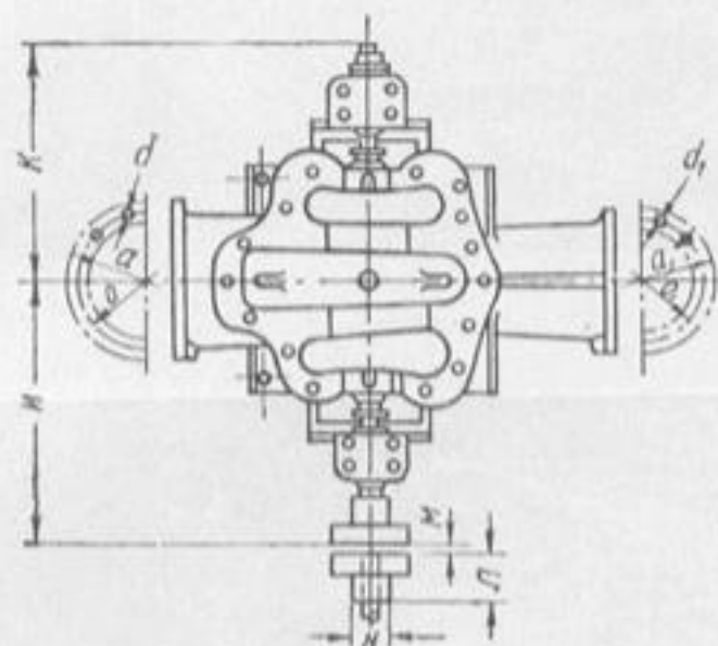
Габаритные размеры насосов типа НДи
