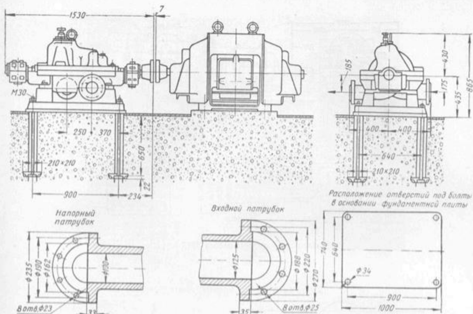
Габаритные размеры насоса 5МД-7 \times 3.
