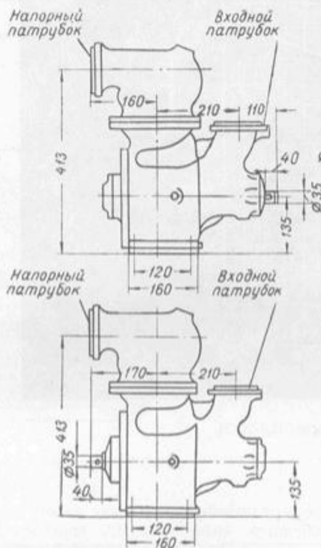
Габаритные размеры насоса СЦЛ-20-24.
