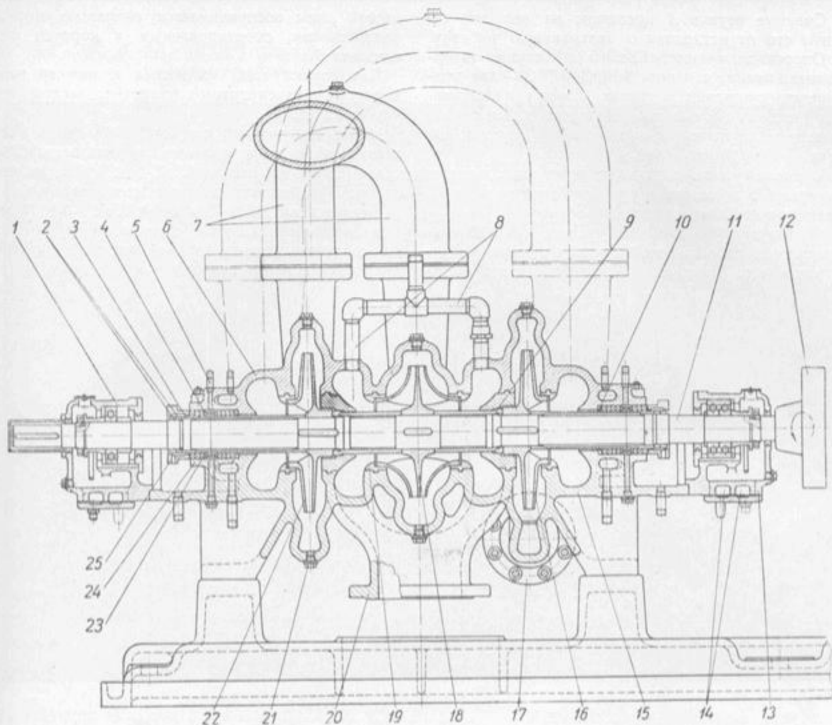
Насос 8КсД-5 × 3.
