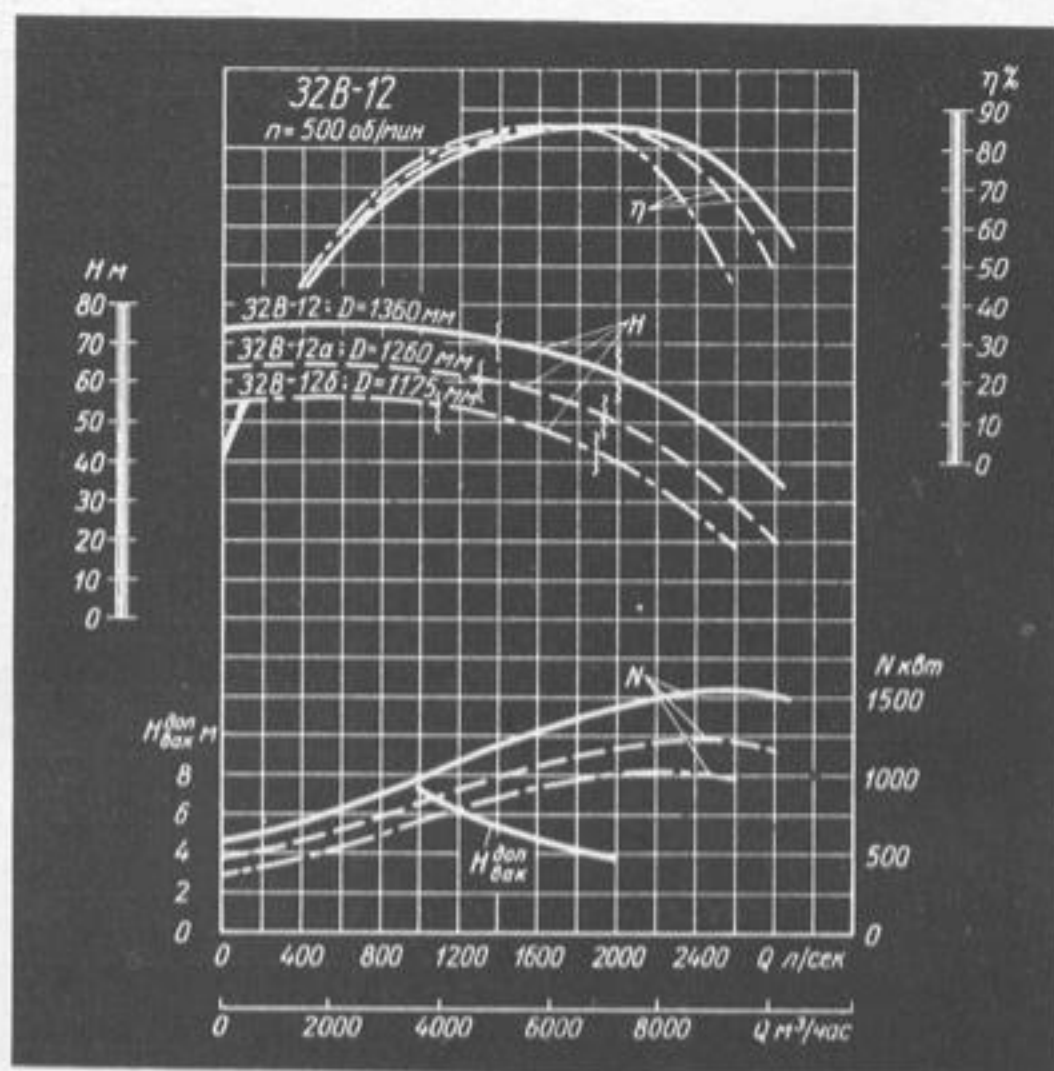
Характеристика насоса 32В-12.
