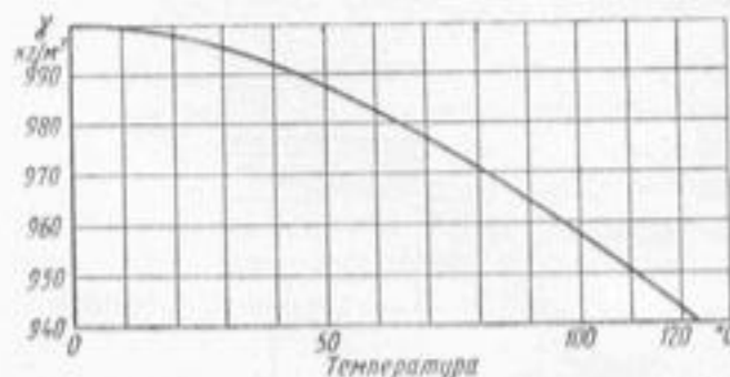
Фиг. 8. Зависимость удельного веса воды от температуры.
