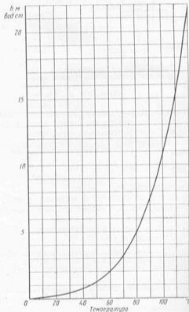
Фиг. 9. Зависимость давления насыщенного водяного пара от температуры, выраженная в м вод. ст. соответствующей температуры.
