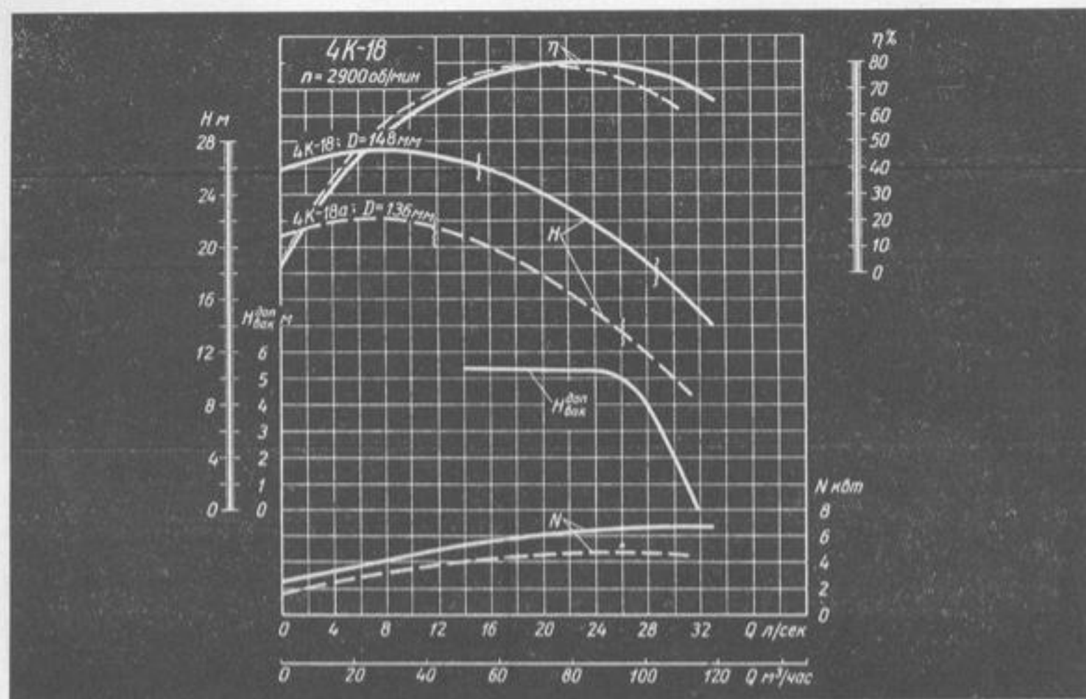
Характеристика насоса 4K-18.
