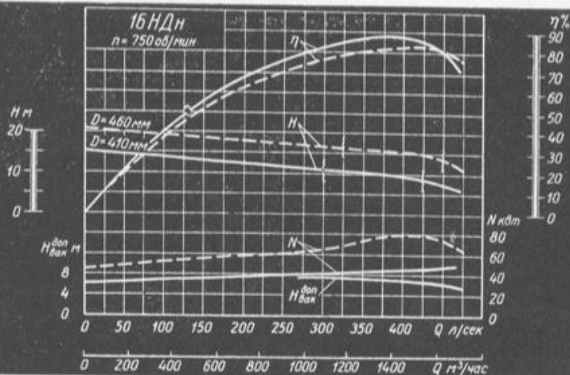
Характеристика насоса 16НДи (n = 750 об/мин).
