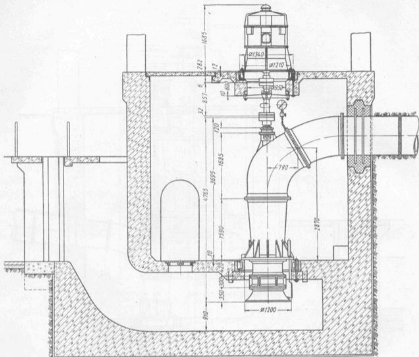
Установочный чертеж насоса 30PrB-60.
