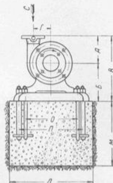
Габаритные размеры насосов типа К на опорных стойках 0-3 и 0-3а с электродвигателем на общей фундаментной плите.
