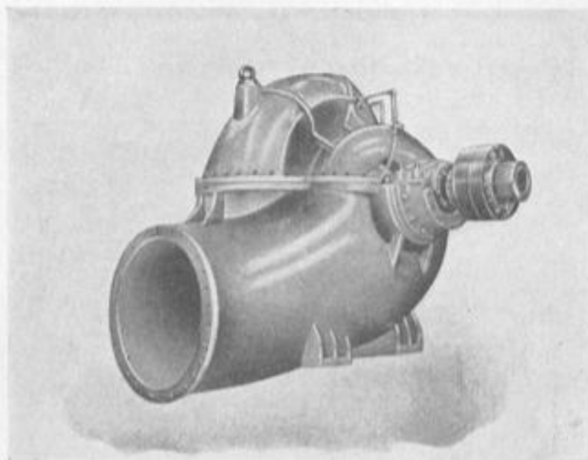
Насос 48Д-22.
