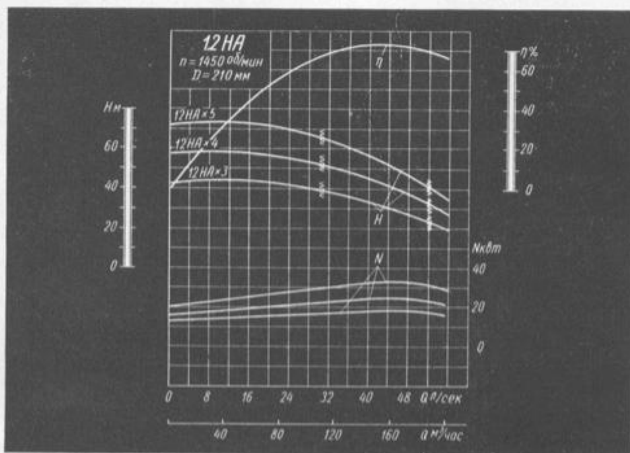
Характеристика насосов 12HA × 3, 12HA × 4 и 12HA × 5.
