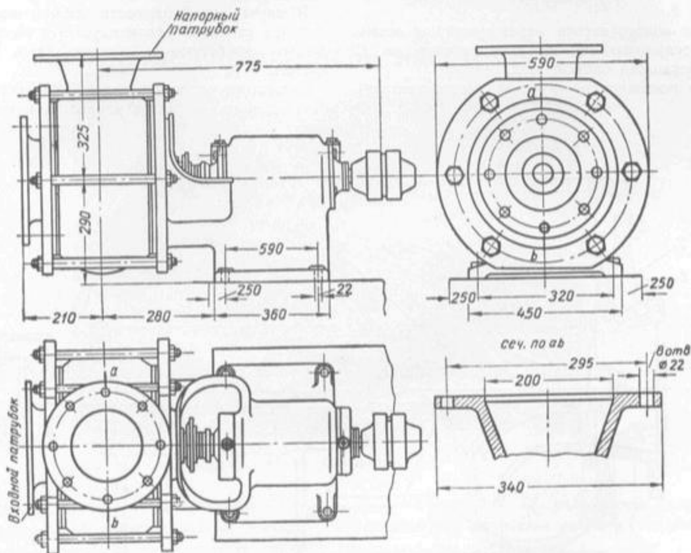
Насос ЭХМ-20/35 — 20/28.
