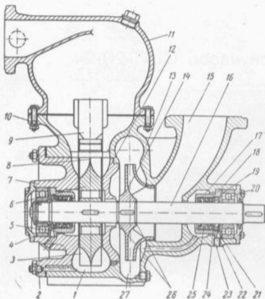
Насос СЦЛ-20-24.
