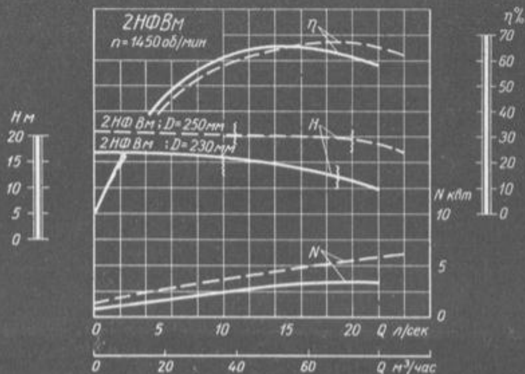
Характеристика насоса 2НФВм.
