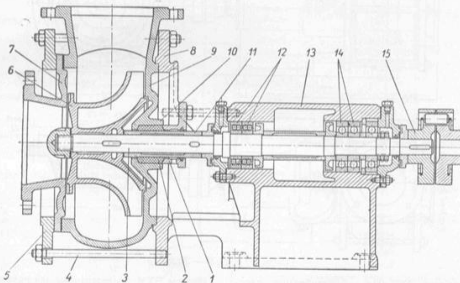
Насос ЭХМ-20/35.
