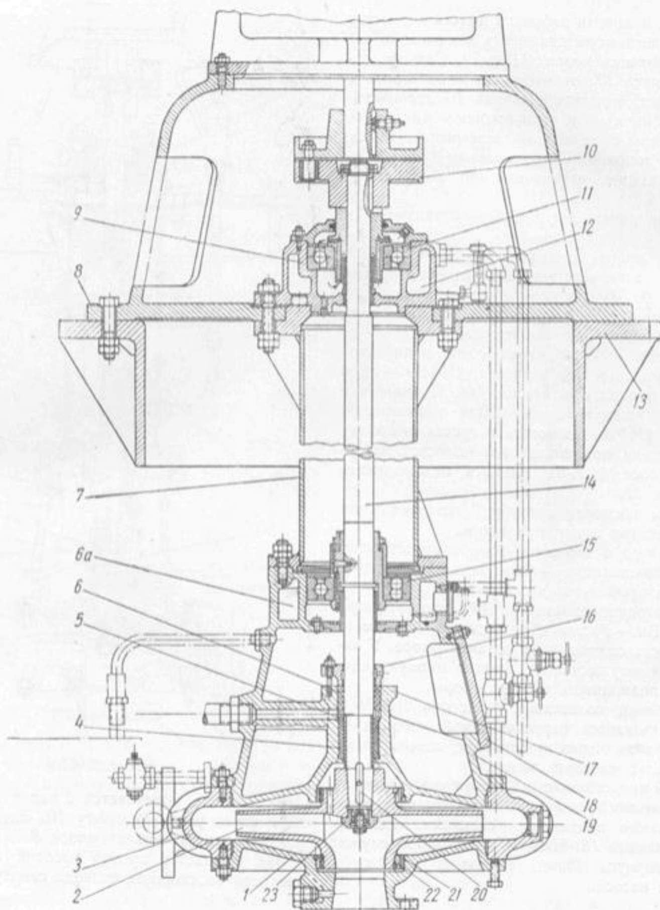
Насос 4ΦВ-5М.
