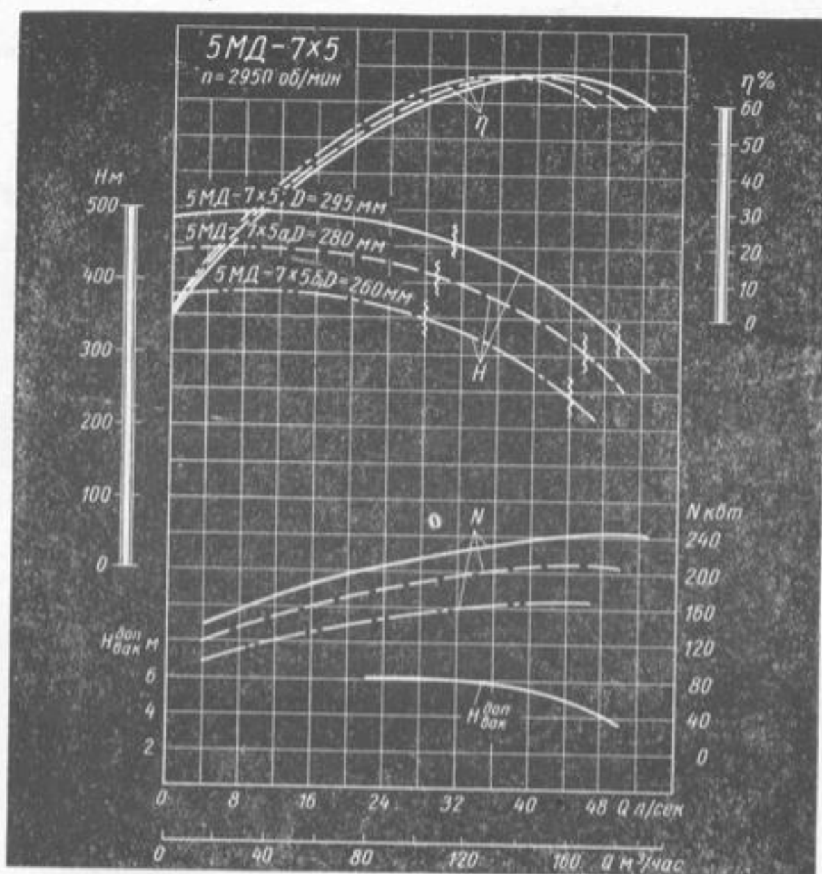
Характеристика насоса 5МД-7х5.
