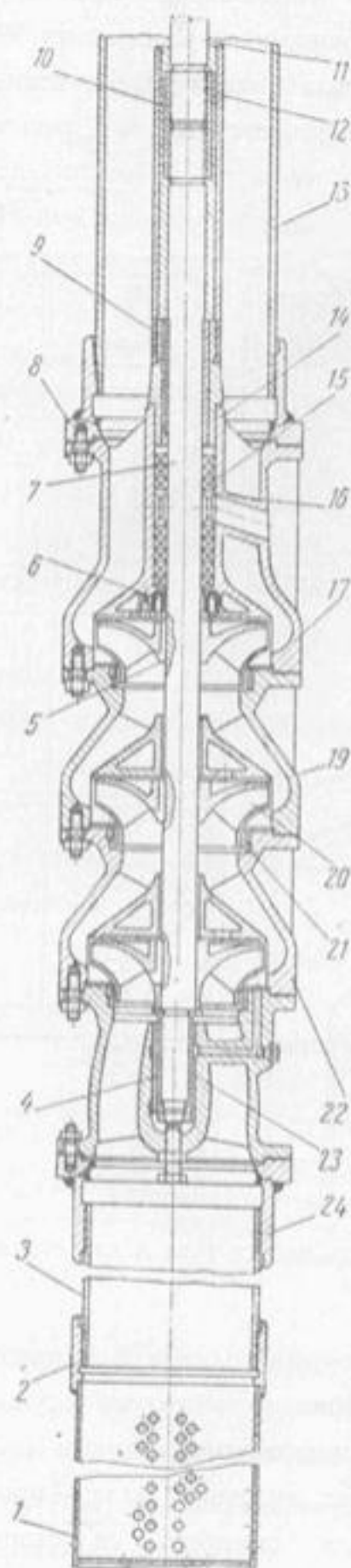
Артезианский насос 12HA \times 3.
