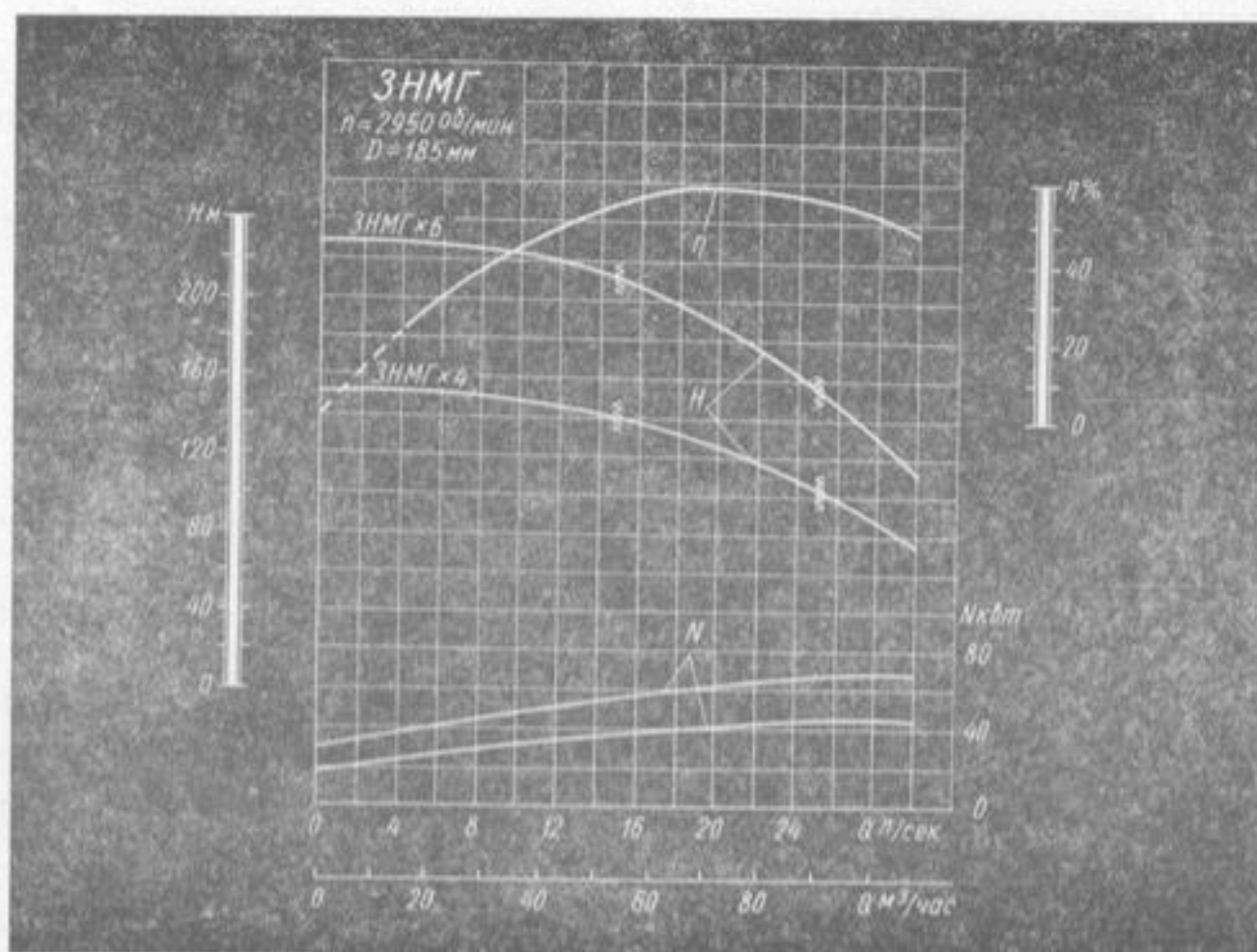
Характеристика насосов 3НМГ×4 и 3НМГ×6.
