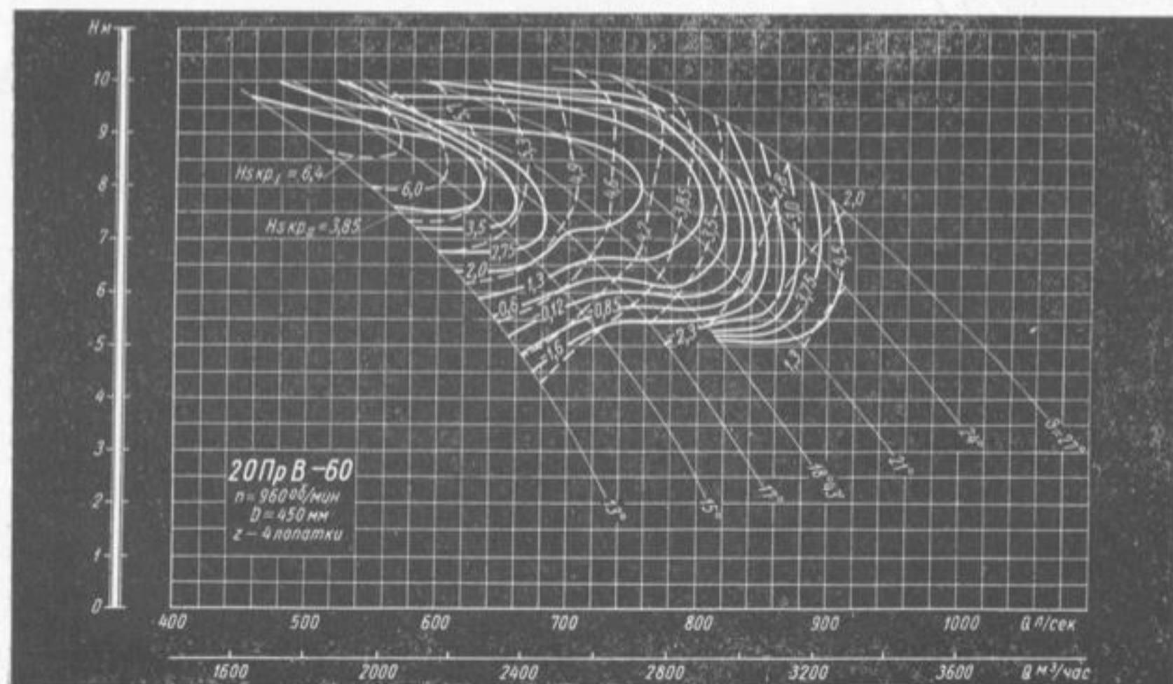
Характеристика высот всасывания насосов 20Пр-60 и 20ПрВ-60 ( n = 960 \text{ об/мин} ).
