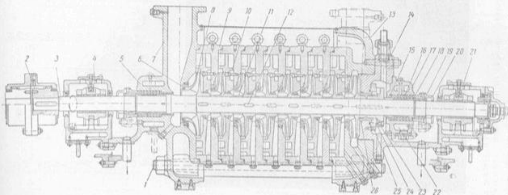
Насос 4П-5X8.
