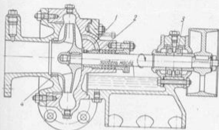
Насос 3К-9 с опорой в виде втулки-грундбуксы.
