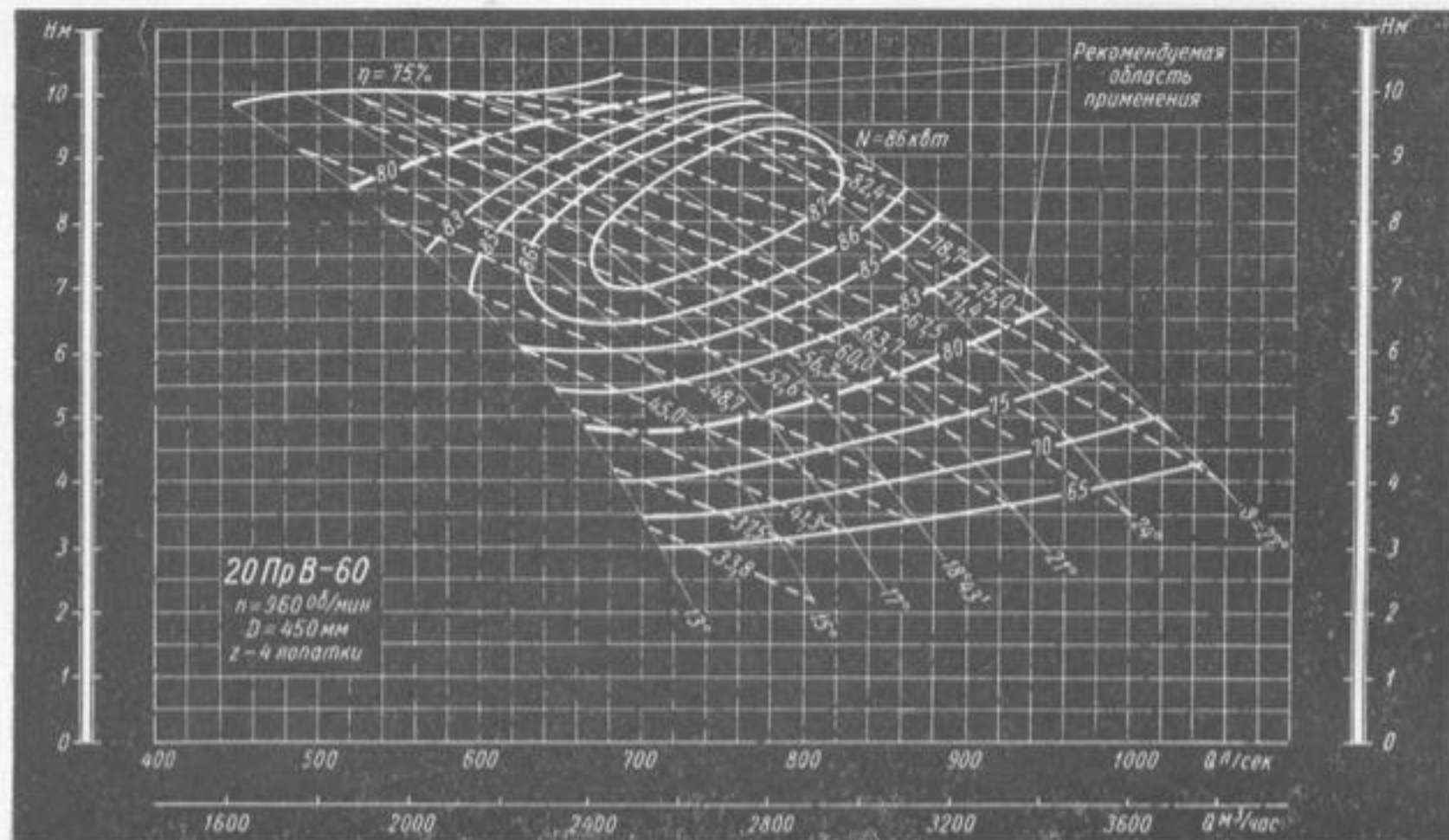
Характеристика насосов 20Пр-60 и 20ПрВ-60 ( n = 960 \text{ об/мин} ).
