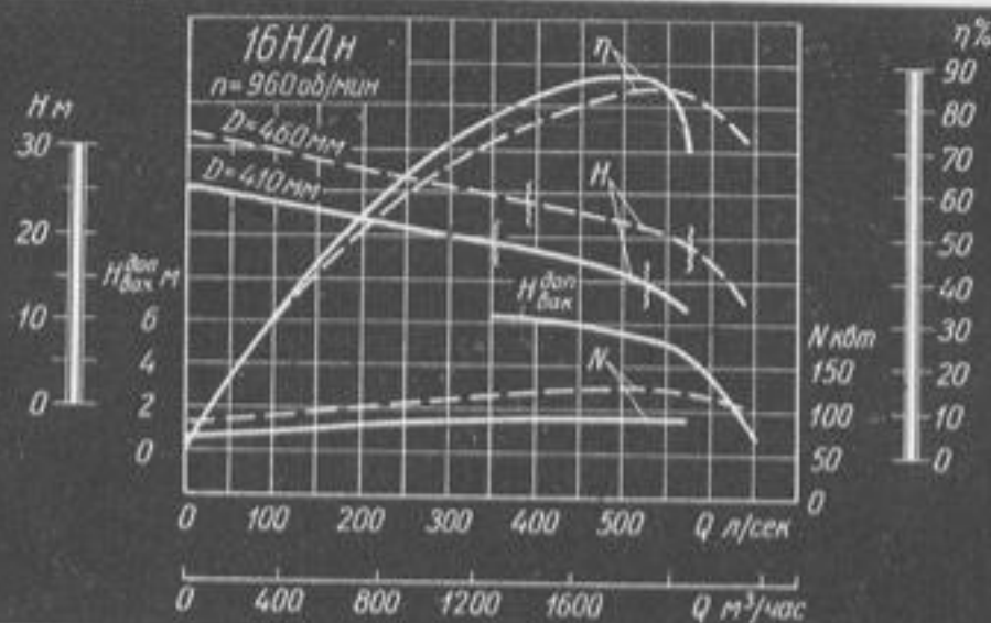
Характеристика насоса 16НДи (n = 960 об/мин).
