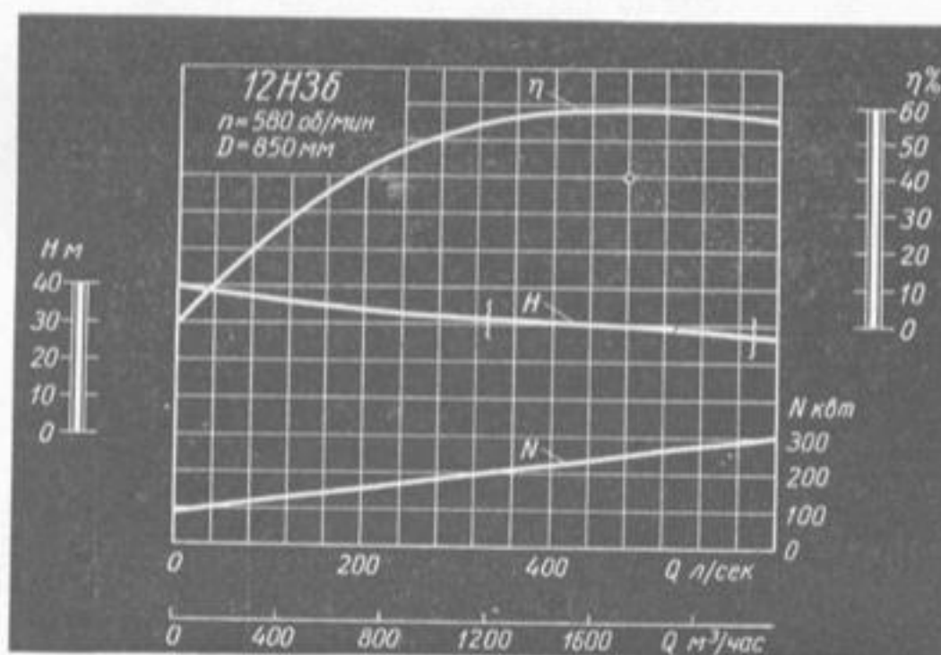
Характеристика насоса 12H36.
