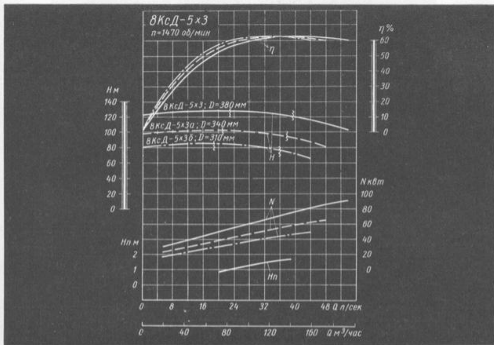
Характеристика насоса 8KcD-5x3.
