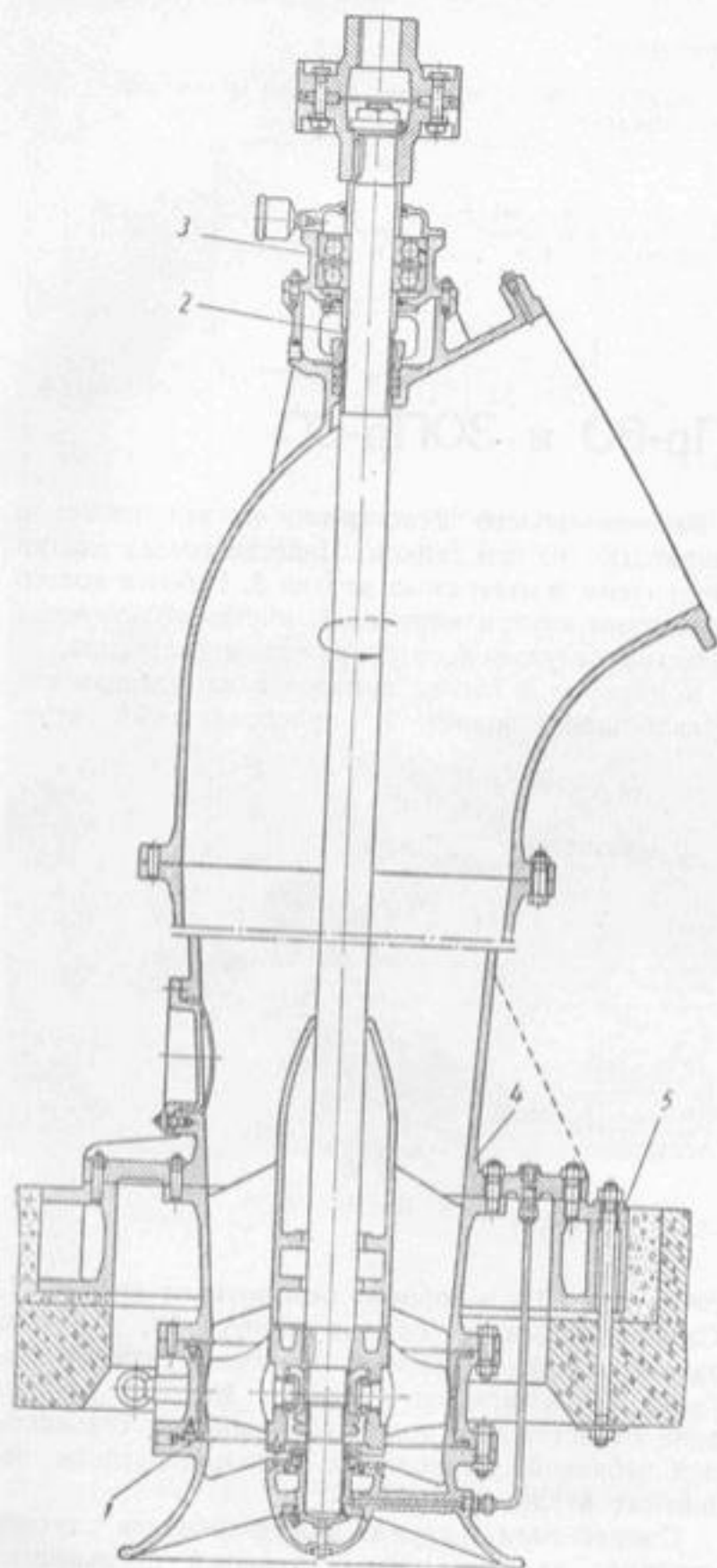
Вертикальный насос 30PrB-60.
