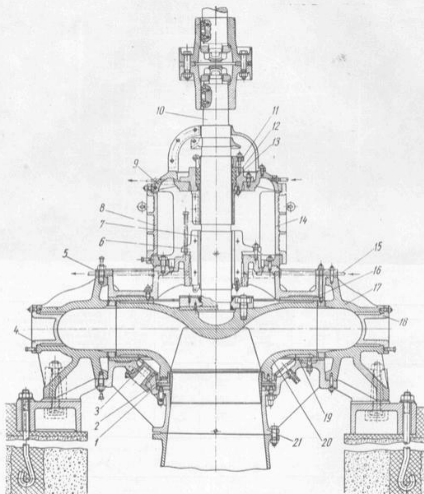
Насос 24ФВ-13.
