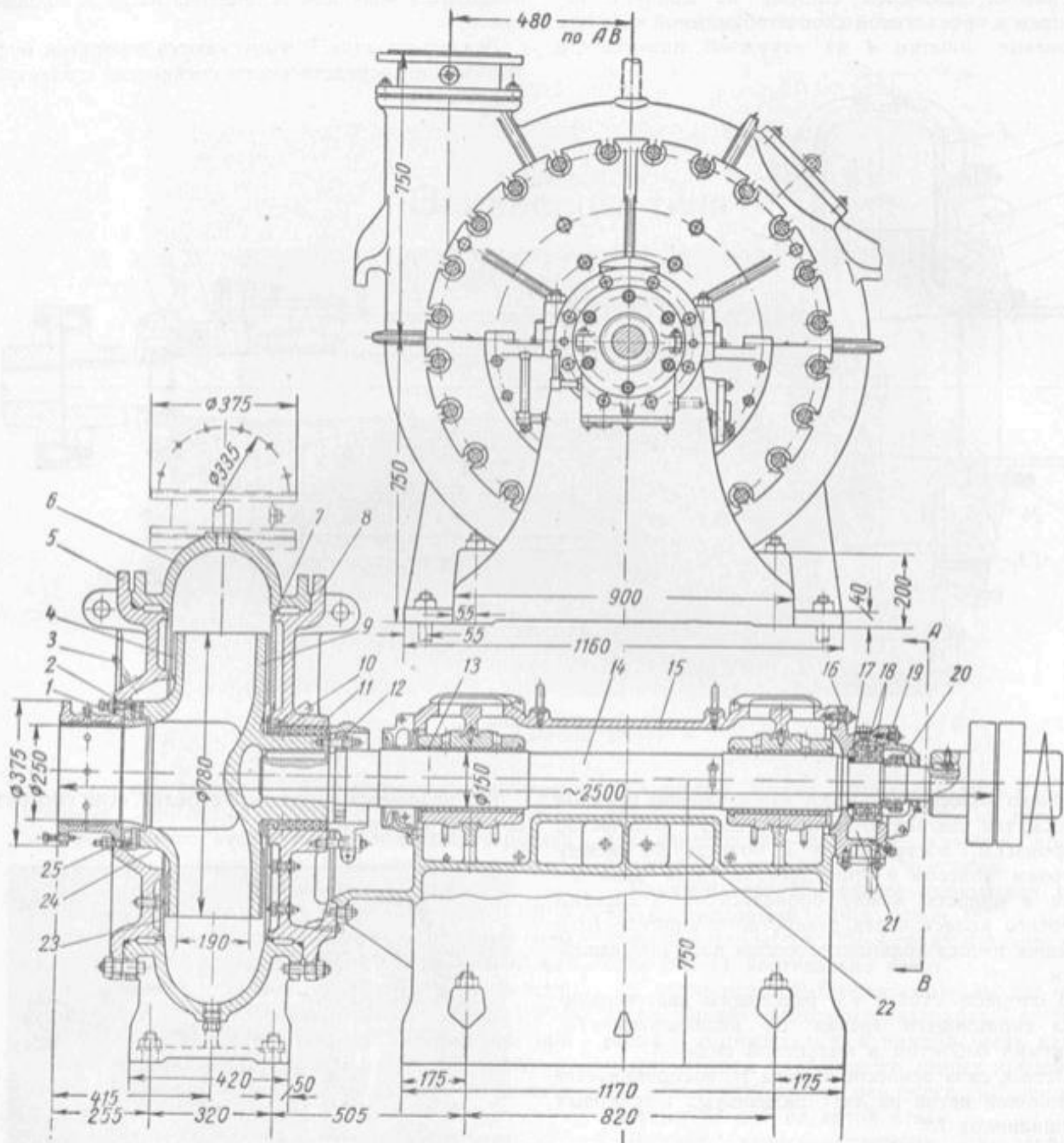
Землесос 10P-7.
