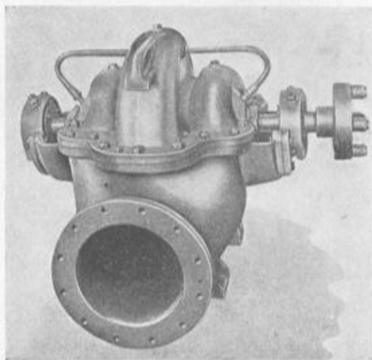
Насос 12Д-19.
