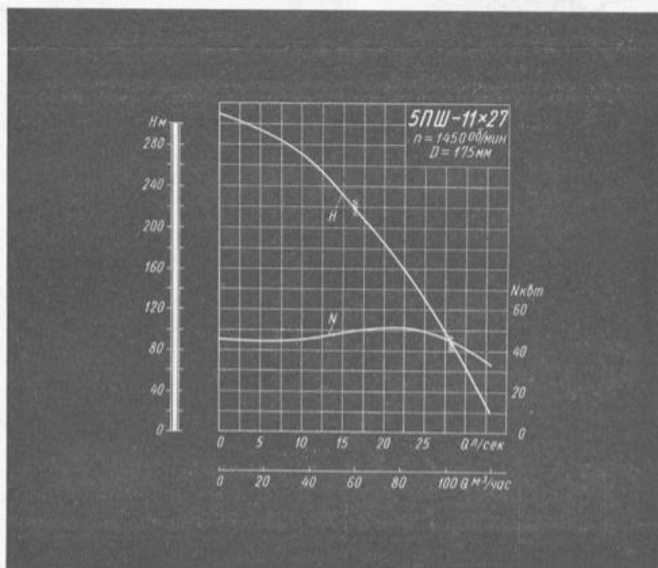
Характеристика насоса 5ПШ-11 × 27.
