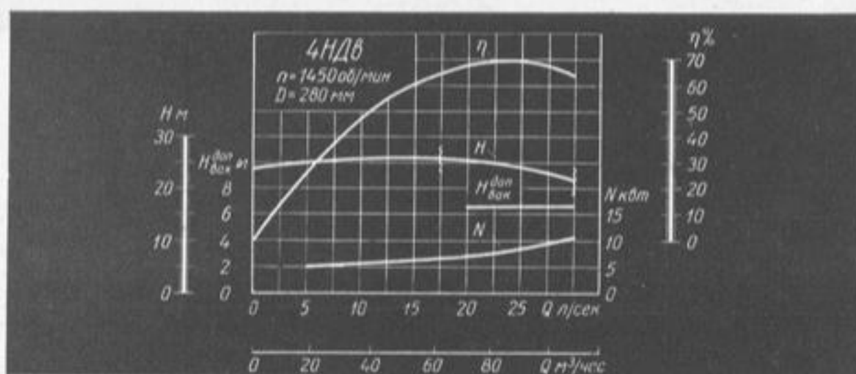
Характеристика насоса 4НДв ( n = 1450 \text{ об/мин} ).
