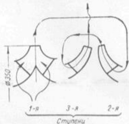
Схема движения потока в трех-ступенчатом насосе типа МД.
