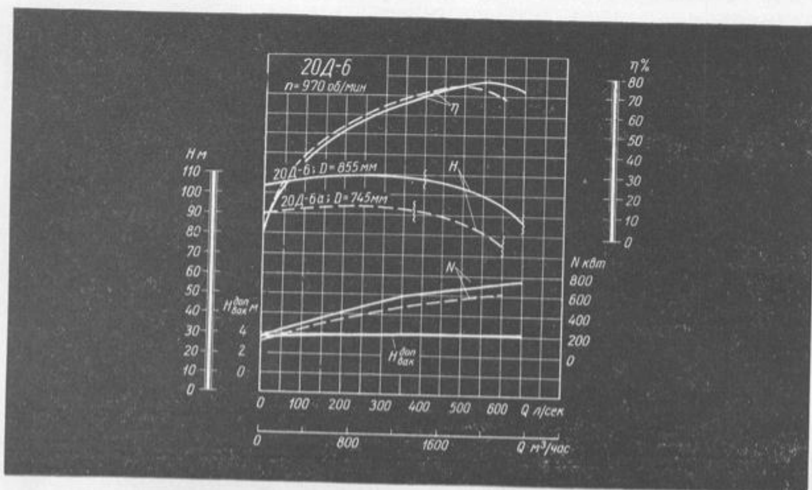
Характеристика насоса 20Д-6.
