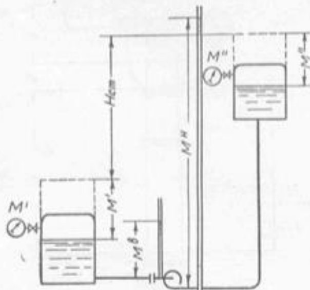
Фиг. 3. Схема установки насоса с закрытыми резервуарами (уровни находятся под давлением выше атмосферного).
