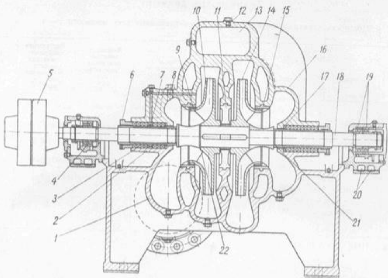
Насос 10HMK \times 2.
