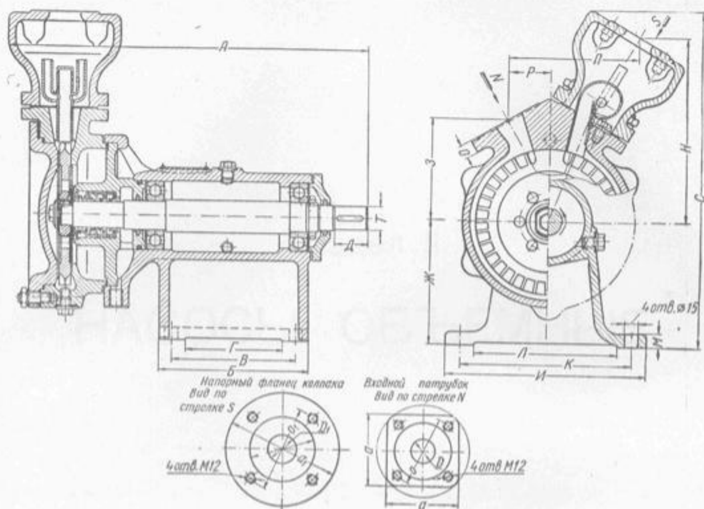
Общий вид и габаритные размеры насосов типа ВС.
