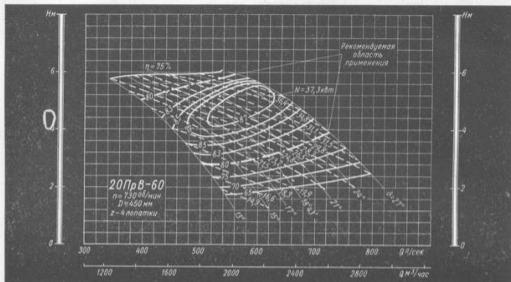
Е. Характеристика насосов 20Pr-60 и 20PrB-60 ( n = 730 \text{ об/мин} ).
