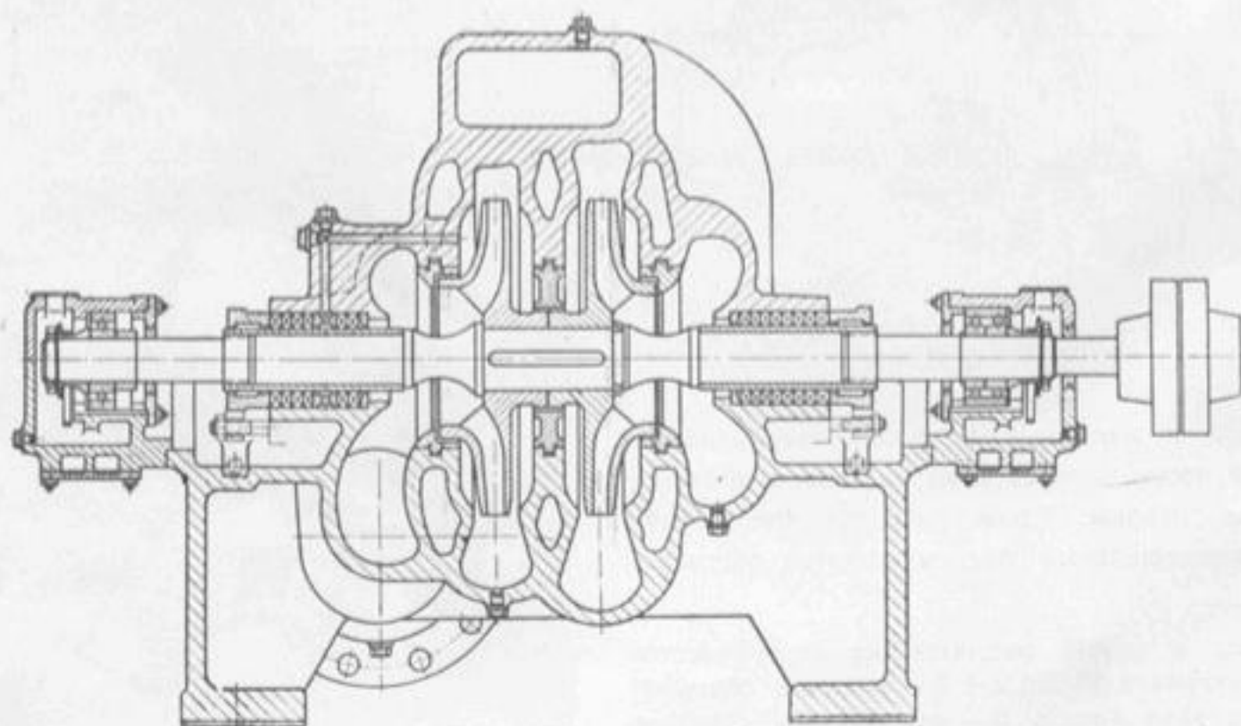
Hacoc 3B-200×2.
