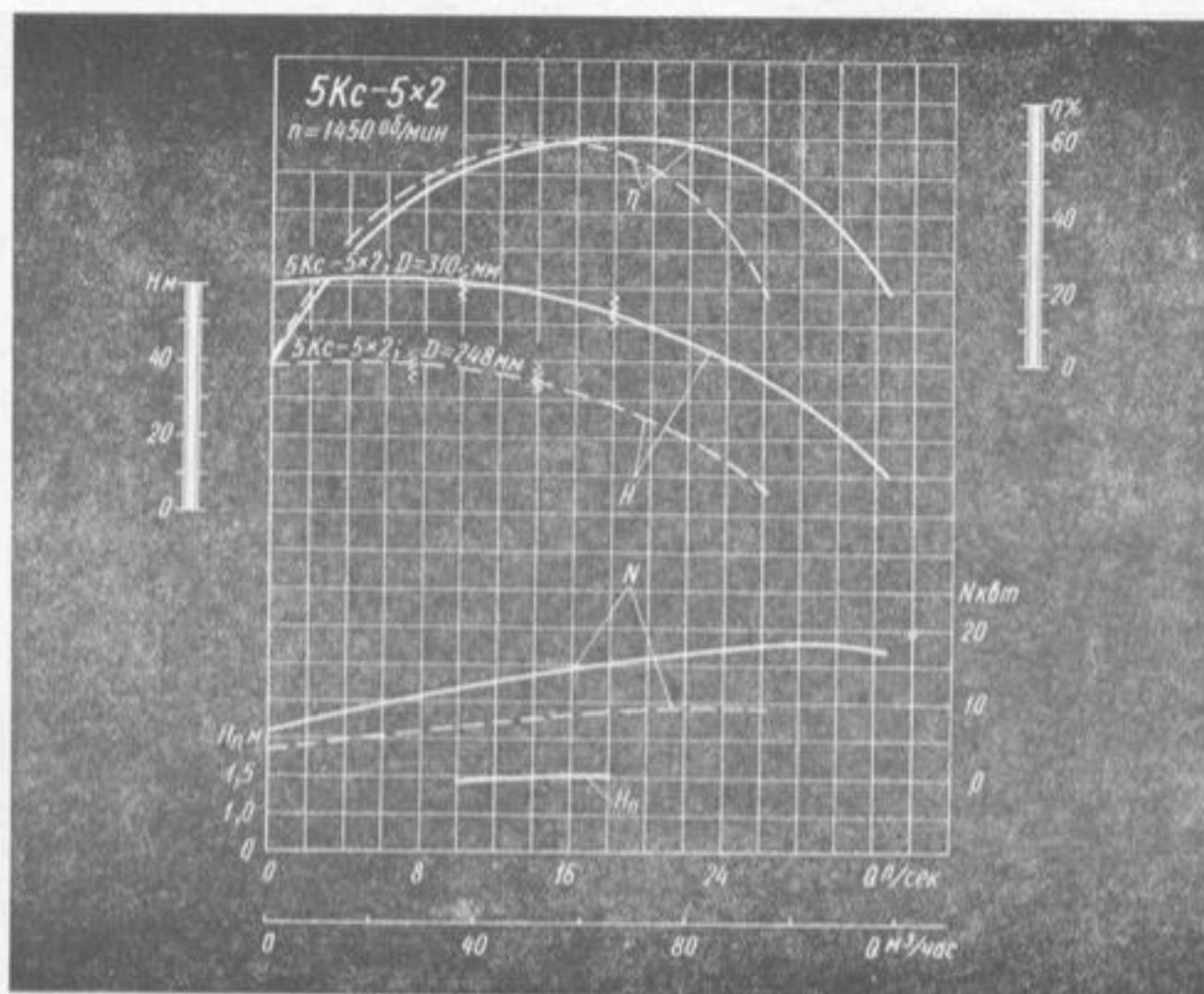
Характеристика насоса 5Кс-5 × 2.
