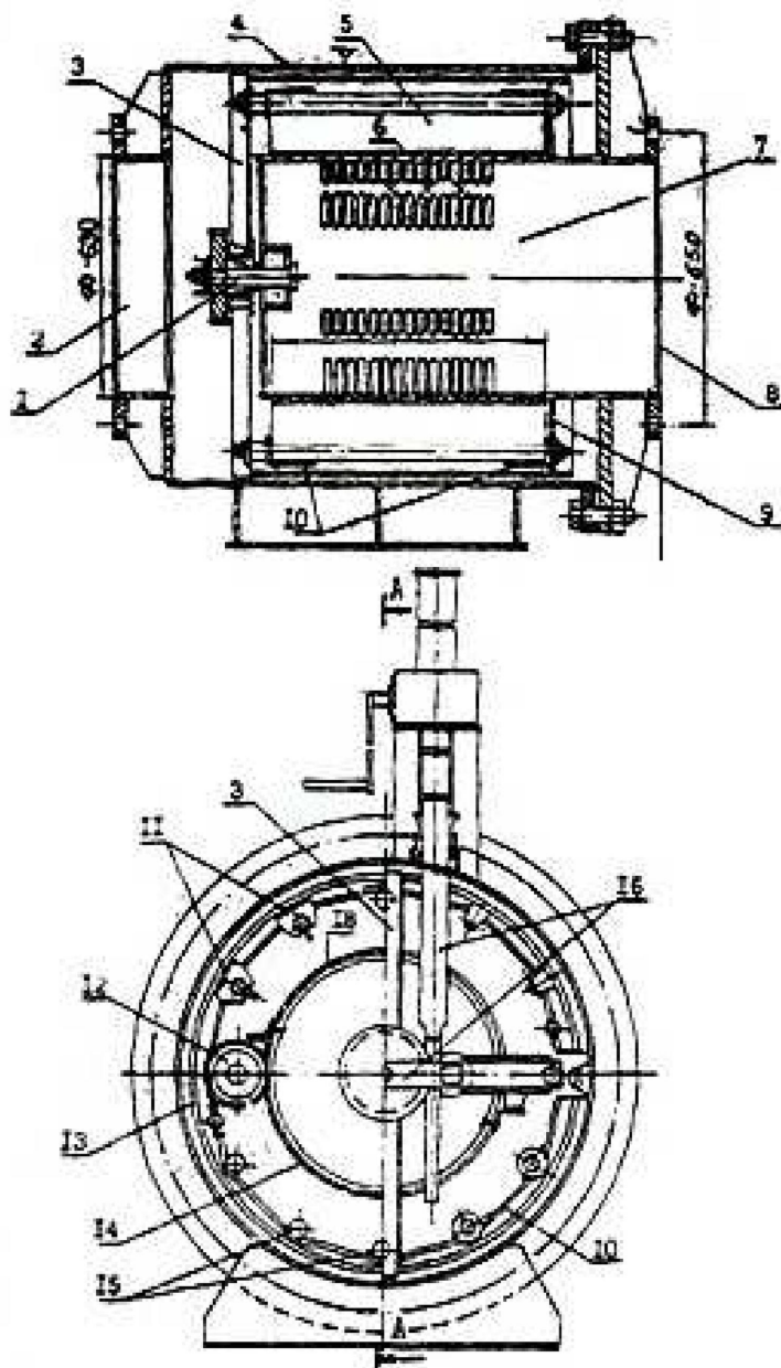
Рисунок 1 - Запорно-регулирующее устройство:
