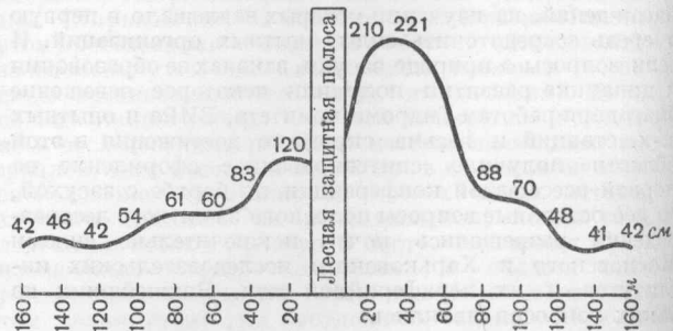
8. Огложение снега в лесных защитных полосах. Однородная полоса из вяза. Наблюдение зимы 1933 г. Тимашевский участок.
