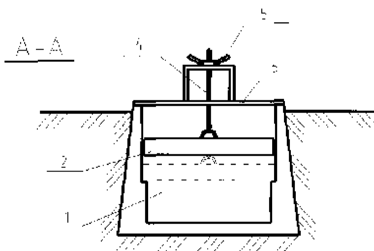
Рисунок 4 – Разрез по A-A рисунка 3
