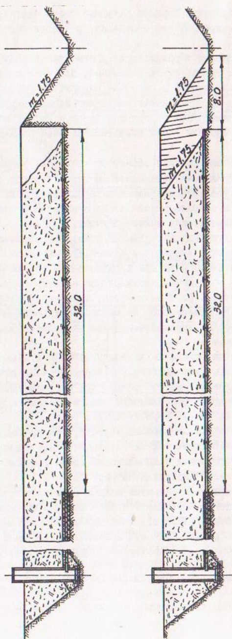
Рис. 3. Технология этажности подсоединения тушиковых дрен к коллектору.
