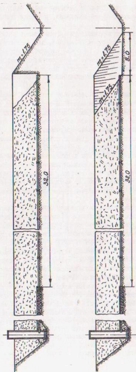
Рис. 3. Технология этапности подсоединения тушиковых дрен к коллектору.
