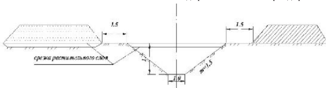
Рисунок 1 - Проектный поперечный профиль картый сброса рисовой системы ОПХ «Караултинский»
