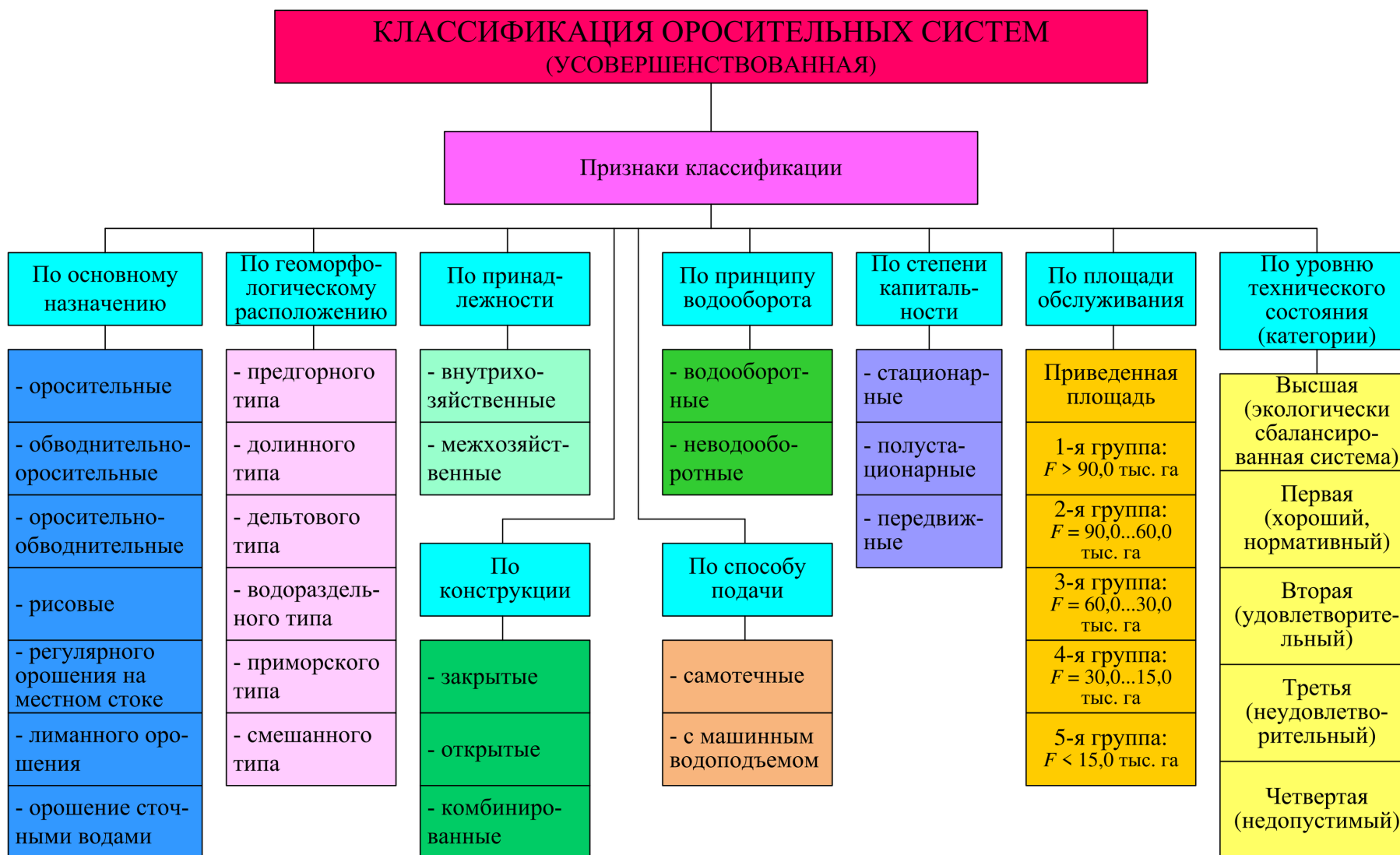
Рисунок 1 – Классификация оросительных систем
