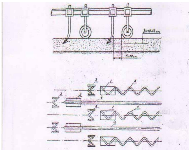
Рис.2. Схема установки катков – борозделов КБ-1 на культиваторе КРХ-4:
