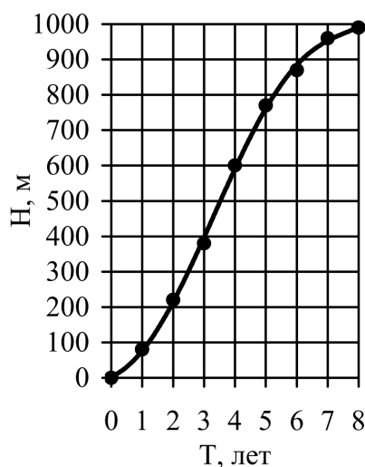
Рис.1. Зависимость необходимого напора воды H для размыва илистых отложений от времени T их нахождения в дренах при эксплуатации по существующей технологии
