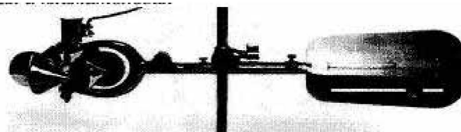
Рис. 8. Вертушка Прайса USGS TYPE AA MODEL 6200 (Rickly Hydrological Company, США) (по [12; 19])
