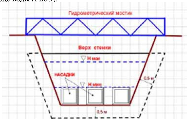
Рис.9. Водомерное устройство типа «СНС»
