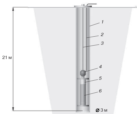
Рис. 9. Схема вертикального модуля на 500 кВт
