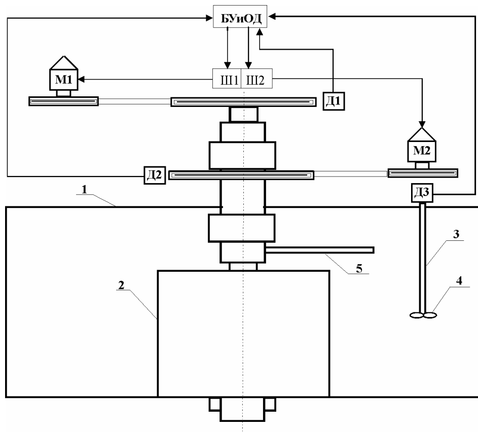
Рис. 4. Структурная схема УПИС.
