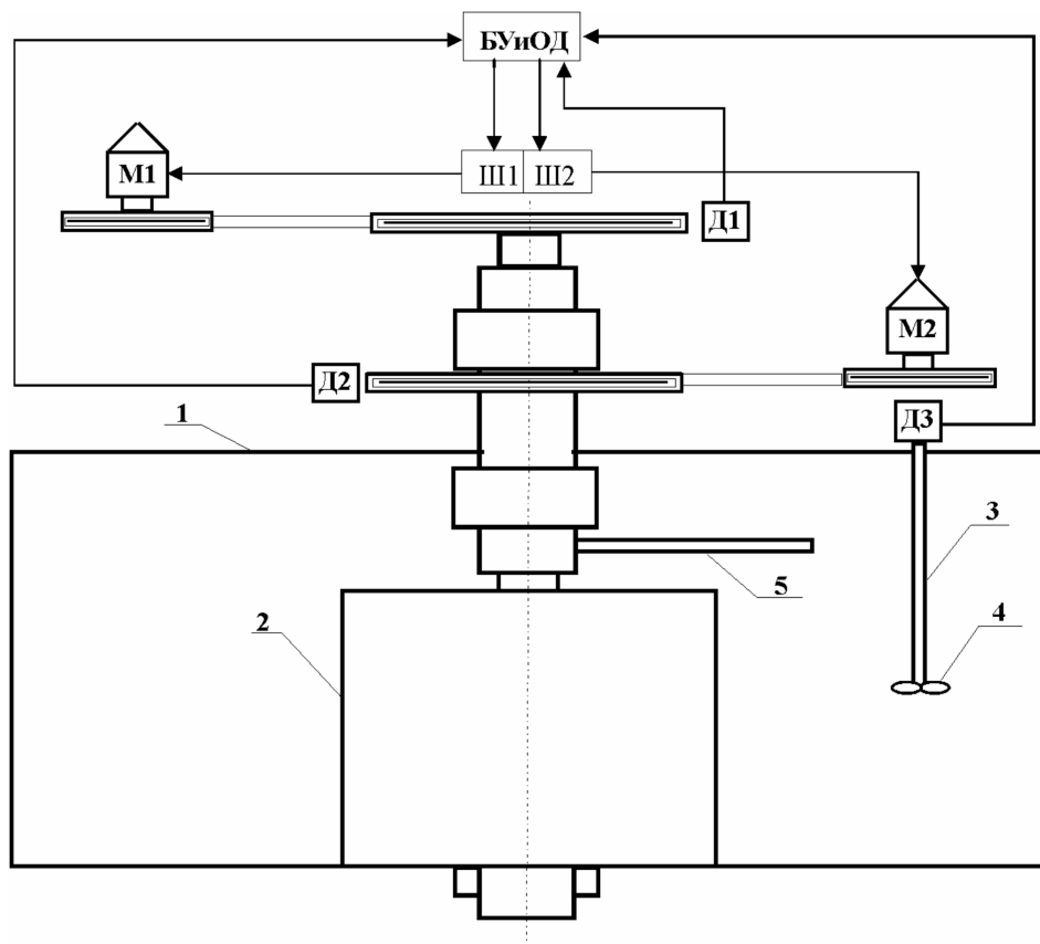
Рис. 4. Структурная схема УПИС.
