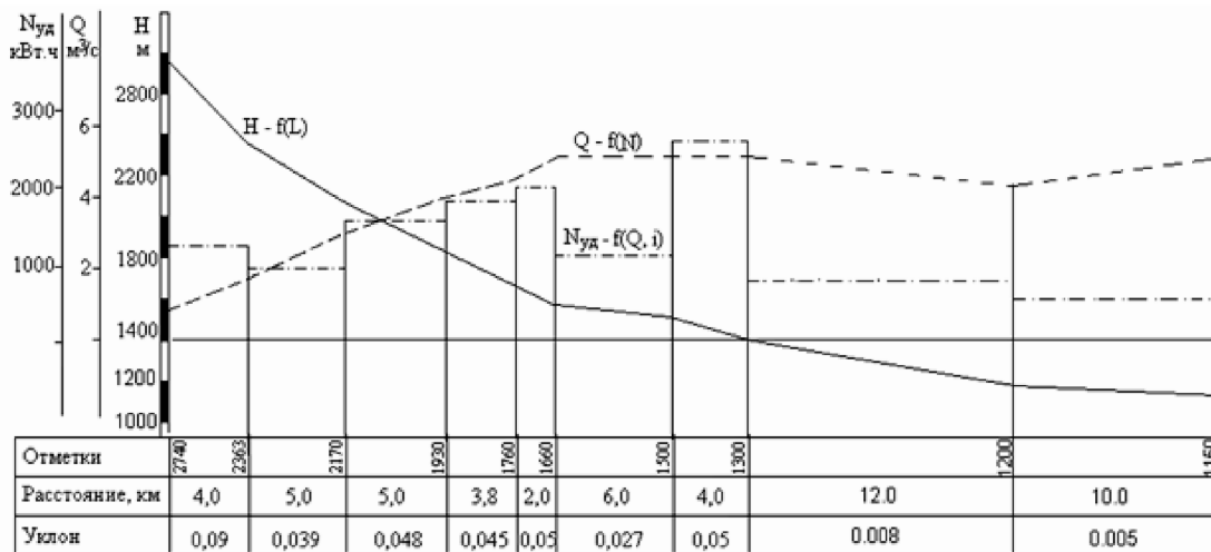
Рисунок 3 – Характерный продольный профиль горной реки Кыргызстана
