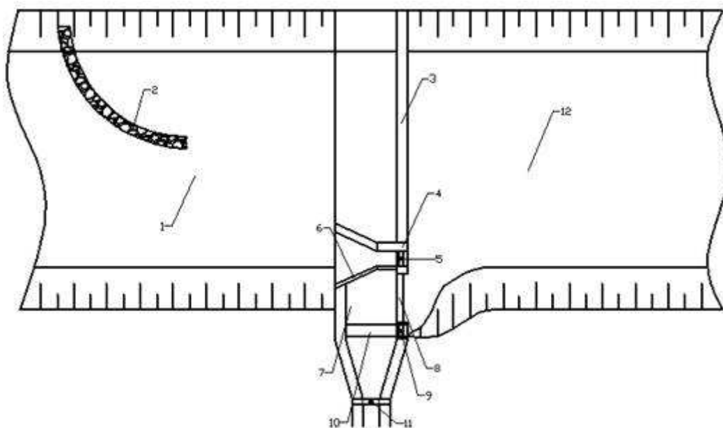
Рис. 1. Схема бесплотинного водозаборного сооружения для горных рек (БВСГР): 1 – подводящее русло; 2 – струнаправляющая шпора; 3 – поперечный речной уступ; 4 – промежуточные устои; 5 – затвор промывного тракта; 6 – ломанный в плане наносозащитный порог; 7 – водоприемная камера; 8 – катастрофический водослив; 9 – затвор промывной галереи водоприемной камеры; 10 – рыбозащитное устройство; 11 – затвор регулятор деривационного канала; 12 – отводящее русло
