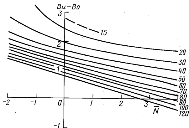
Рис. 2. Зависимость комплексного параметра тепло-влагообмена атмосферы с подстилающей поверхностью ( Bu-Bo ) от спутникового параметра облачности \bar{N}_{ис3} (цифры у линий — параметр V )
