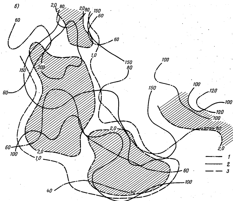
и параметра S (3) за сентябрь (а) и ноябрь (б) 1972 г.
