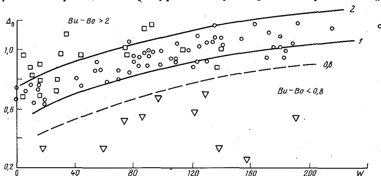
Рис. 3. Зависимость поправки \Delta_0 к максимально возможному испарению E_0 от параметра W , характеризующего комплексно соотношение предшествующего увлажнения почвы и осадков расчетного периода (цифры у линий — Bu - B_0 )
