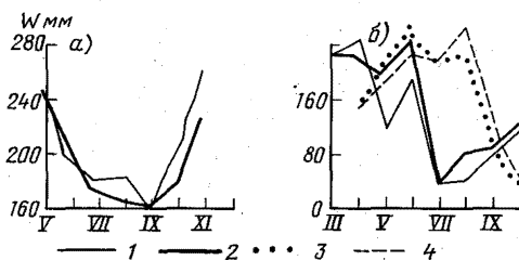
Рис. 4. Результаты расчетов влажности почвы и максимально возможного испарения по предложенному алгоритму для воднобалансовых участков агрометстанций Полтавы (а) и Нержина (б):
