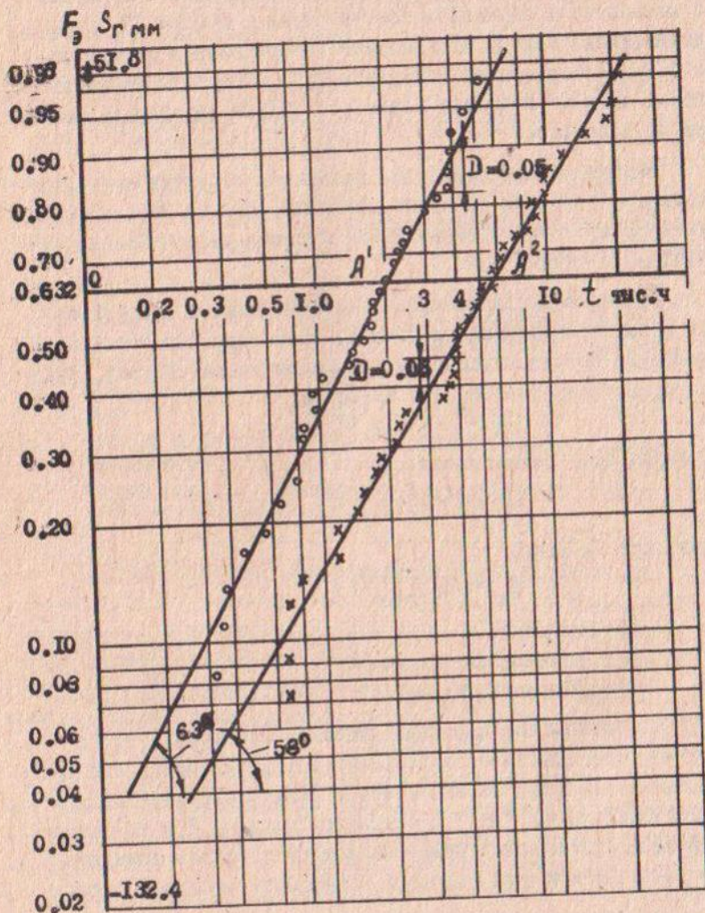
Рис. 1. Графики экспериментальных функций распределения наработки на отказ электронасоса ЭЦВ10-160-35Г: 1 - минерализация 4-8 г/л, пескование 0,1-0,3; 2 - минерализация 2-4 г/л, пескование до 0,01 г/л.
