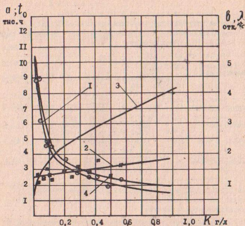
Рис.2. Зависимость показателей надежности и параметров закона распределения наработки на отказ электронасоса 29В12-255-30Г от пескования (минерализация 2-5 г/л):
