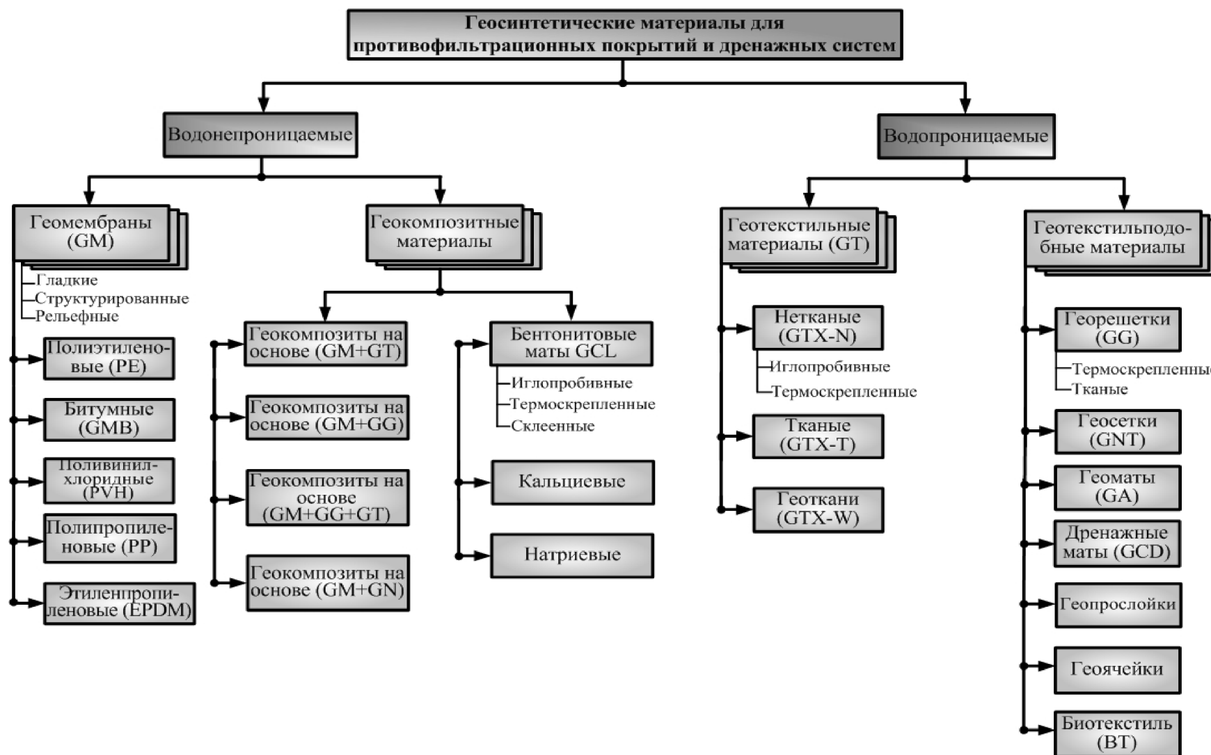
Рисунок 1 – Классификация геосинтетических материалов, применяемых в гидротехническом строительстве для противофильтрационных покрытий и дренажных систем
