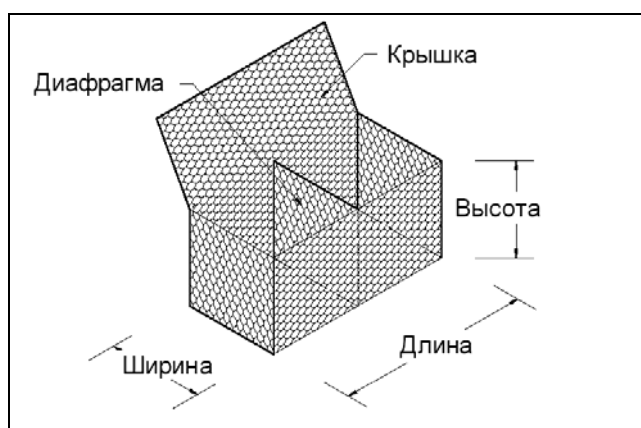
Рис. 2. Коробчатый габион
