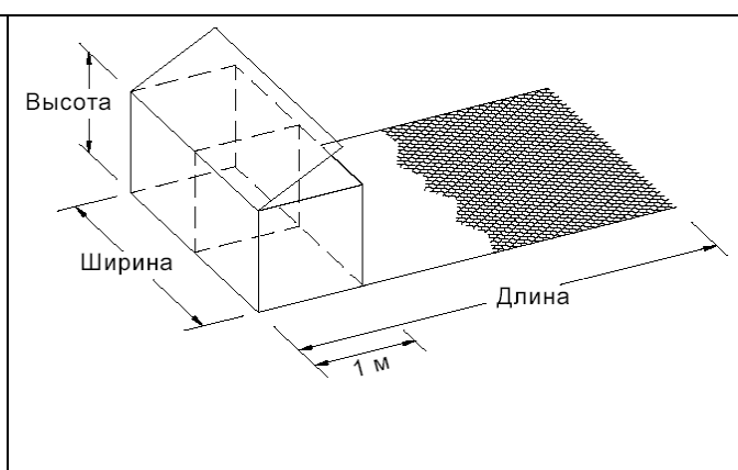
Рис. 3. Система Террамеш
