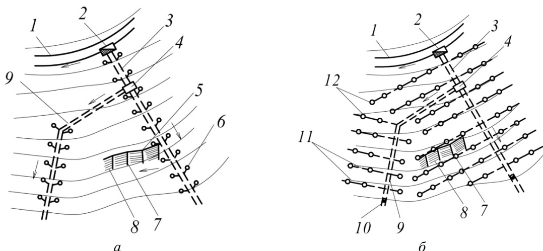
а – закрытая безнапорная; б – закрытая напорная; 1 – магистральный канал; 2 – шлюз-регулятор; 3 – распределитель I; 4 – вододельитель; 5 – временный ороситель; 6 – водовыпуск во временный ороситель; 7 – выводные борозды; 8 – поливные борозды; 9 – распределитель II; 10 – напороразгрузочное устройство; 11 – закрытый ороситель; 12 – водовыпуск в выводную борозду и гибкий шланг
