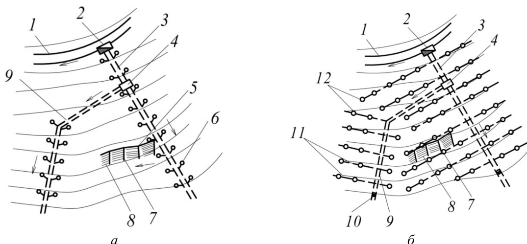
а – закрытая безнапорная; б – закрытая напорная; 1 – магистральный канал; 2 – шлюз-регулятор; 3 – распределитель I; 4 – вододелитель; 5 – временный ороситель; 6 – водовыпуск во временный ороситель; 7 – выводные борозды; 8 – поливные борозды; 9 – распределитель II; 10 – напороразгрузочное устройство; 11 – закрытый ороситель; 12 – водовыпуск в выводную борозду и гибкий шланг
