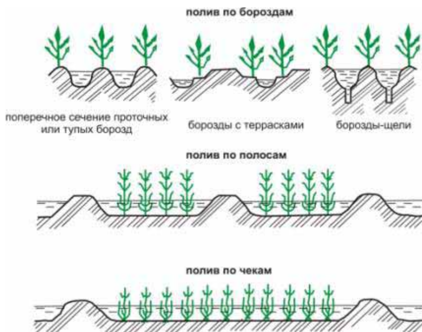
Рис. 1. Основные способы поверхностного способа полива
