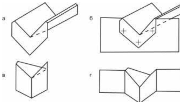
Рис. 7. Оголовки борозд: а- пластмассовый; б- пластмассовый с закрылками; в- из жести; г- из жести с закрылками
