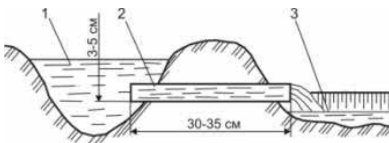
1- выводная борозда; 2- поливная трубка; 3- поливная борозда
