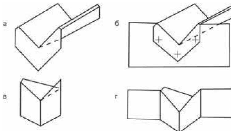
Рис. 7. Оголовки борозд: а- пластмассовый; б- пластмассовый с закрывками; в- из жести; г- из жести с закрывками
