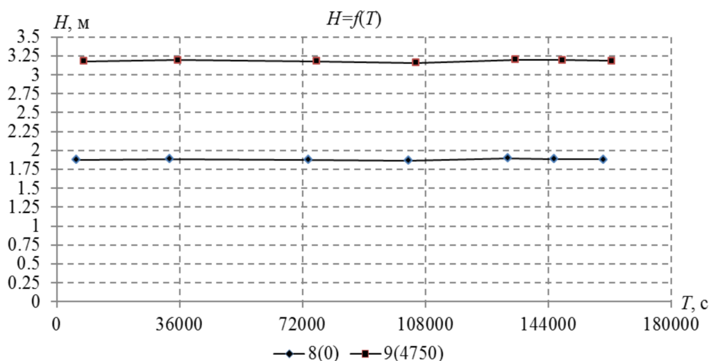
Рисунок 3 – Зависимость изменения уровней от времени в начальном створе 8-го и конечном створе 9-го бьефов для отбора расходов воды 98 % обеспеченности при наличии регуляторов уровней по нижнему и верхнему бьефам сооружений (регулирование с перетекающими объемами)
