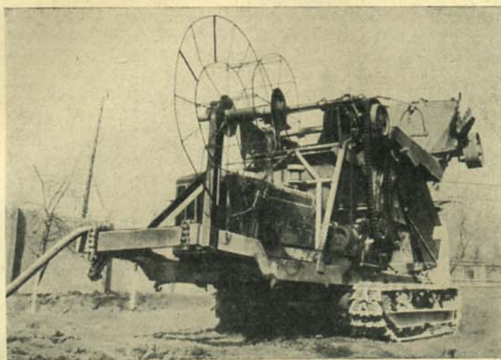
Рис. 6. Щелевой дренаж-укладчик ДШ-251 конструкции САННИРИ для строительства пластмассового дренажа. Отдел организации и механизации водохозяйственных работ
