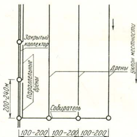
Продольная схема расположения дренажной сети
