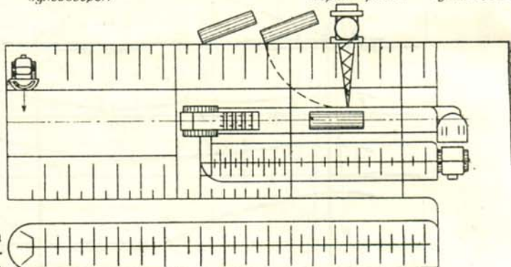
Схема производства работ по устройству закрытого коллектора
