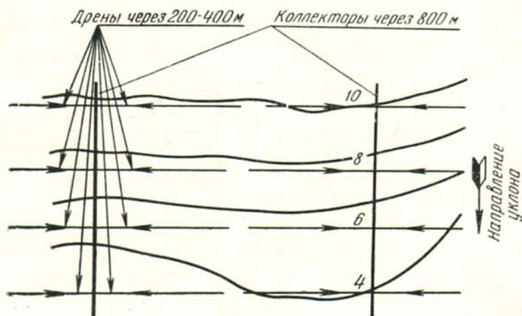
4 Поперечная схема расположения дренажной сети
