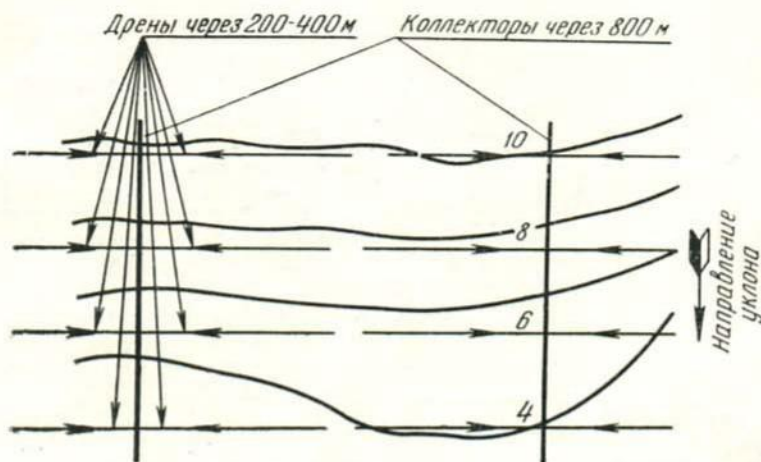
4 Поперечная схема расположения дренажной сети
