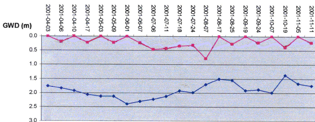
Рис. 5. Динамика глубины залегания грунтовых вод (GWD) и коэффициента «покрытия» орошаемой площади поливами(IAC) для участка дренируемого дренай - УД-3 (2001)
