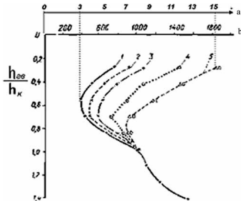
Рис. 3. Оптимизация мелиоративного режима по сумме приведенных затрат учетом воды и урожая: 1 — C = 1 г/л; 2 — C = 2 г/л; 3 — C = 3 г/л; 5 — C = 15 г/л.
