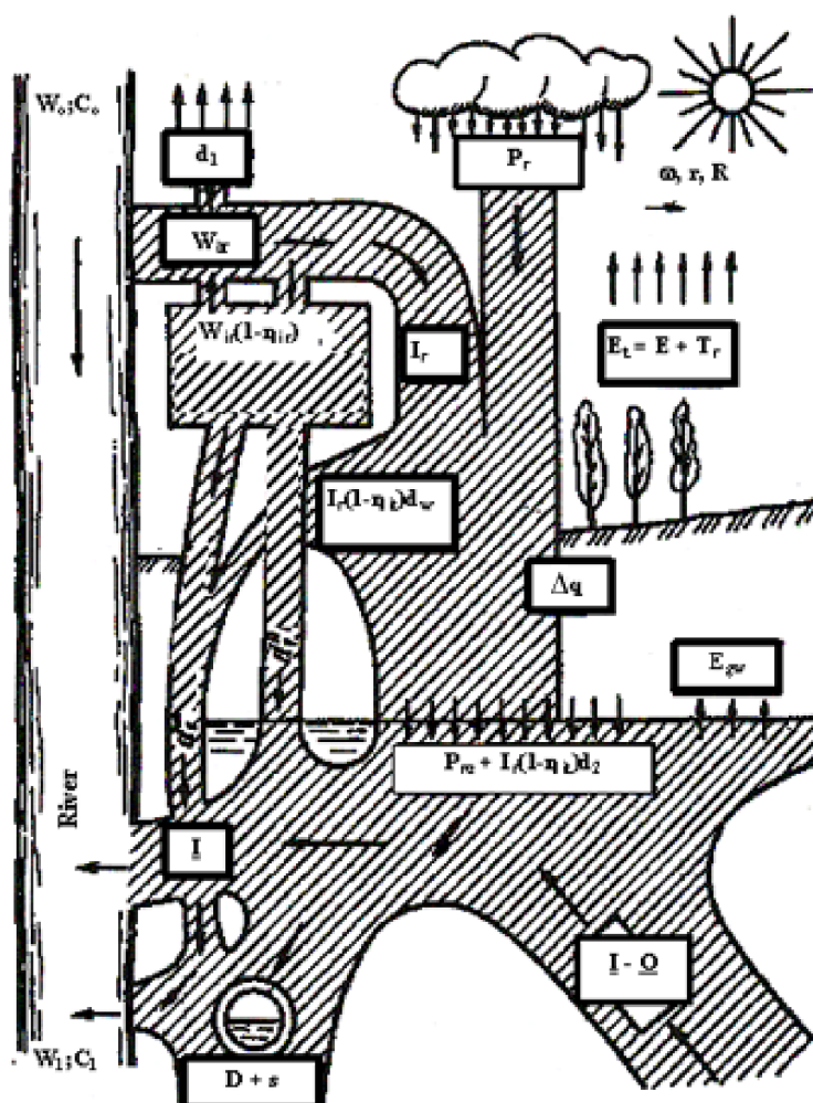
Рис.2. Взаимодействие орошения и дренажа в оросительных системах
