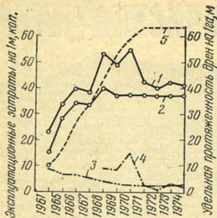
Рис. 2. Изменение удельной протяженности дренажа и затрат на его содержание: 1 — всего эксплуатационных затрат, в том числе: 2 — амортизационные отчисления, 3 — содержание штата, 4 — промывка дрен и очистка колодцев, 5 — рост удельной протяженности дренажа на 1 га.
