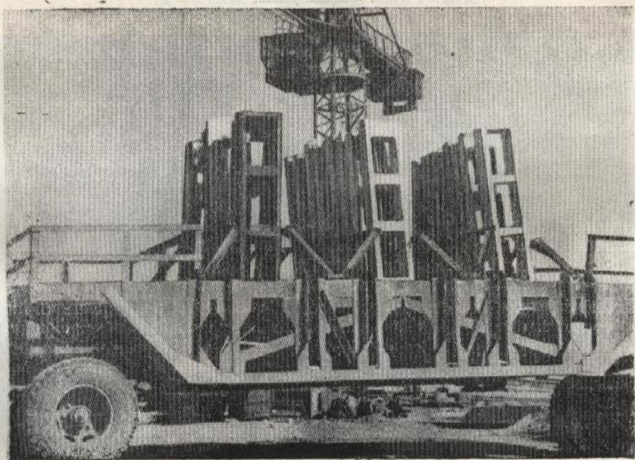
Рис. 4. Контейнер стойковоза для перевозки стоек, совмещенных с седлами.
